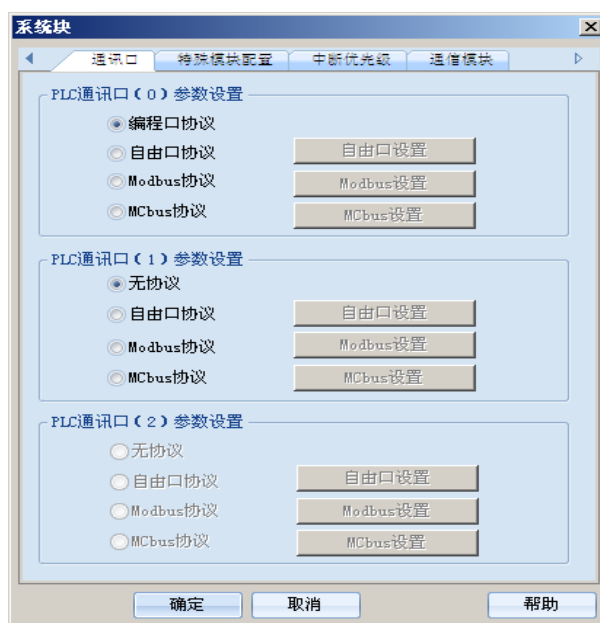
图2-9 设置通讯口
