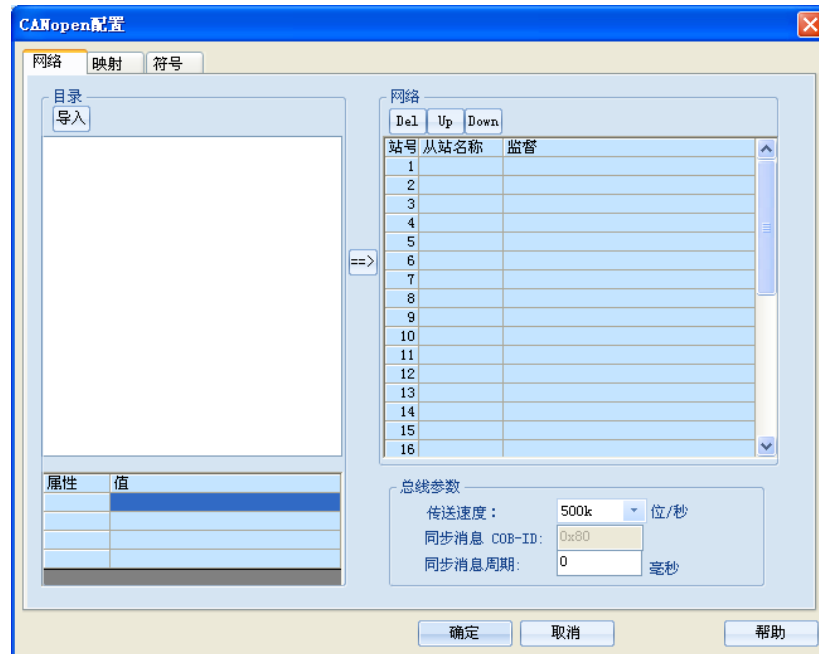
图2-14 CANOPEN 模块配置
