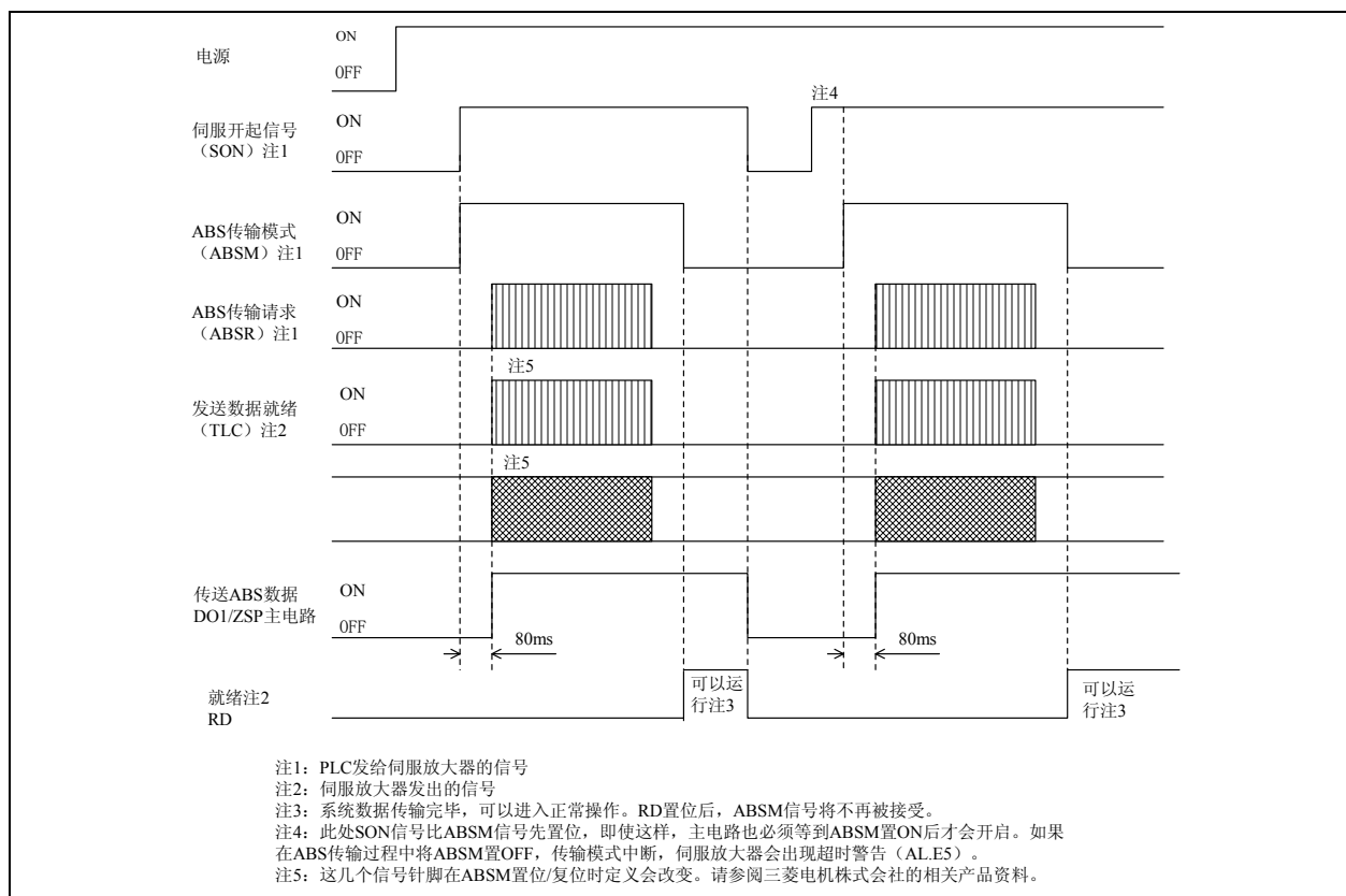
时序图
