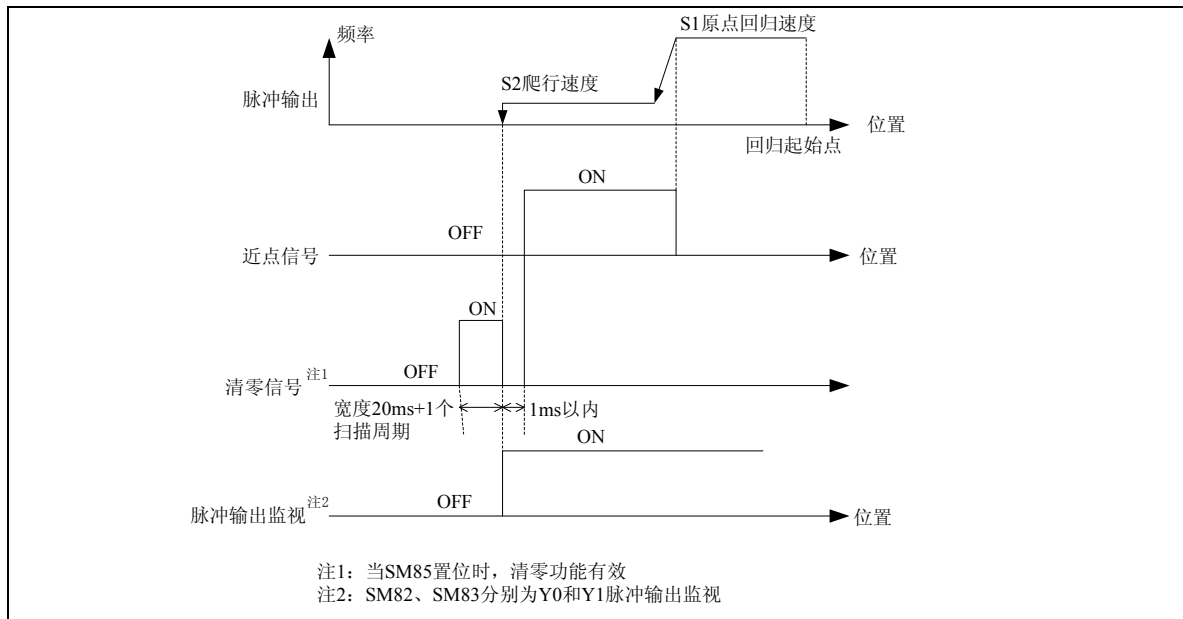
时序图
