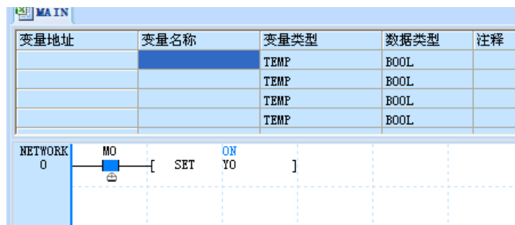
图2-24 被强制软元件的锁标记
