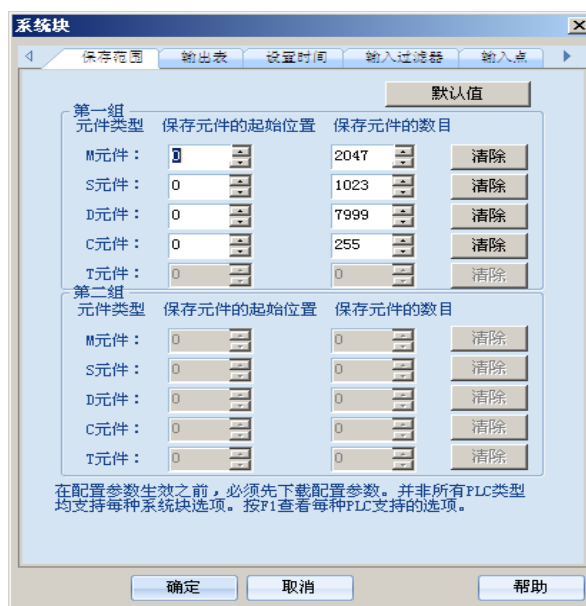
图2-2 设定保存范围
