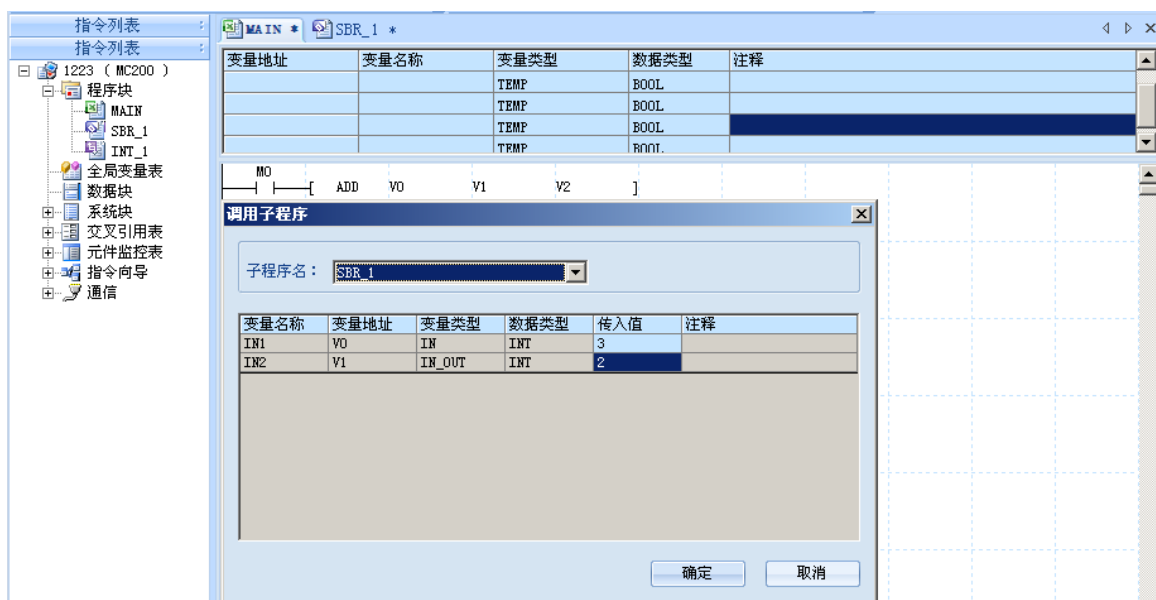
图4-13 调用子程序
