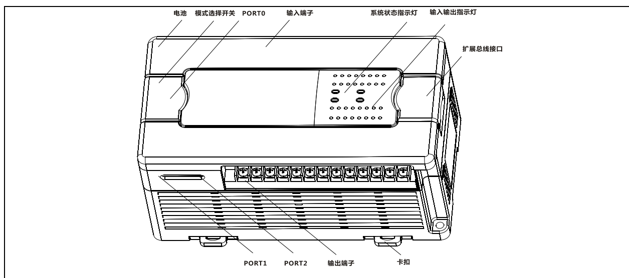
图1-4 MC280 系列主模块的外形结构与部件布局
