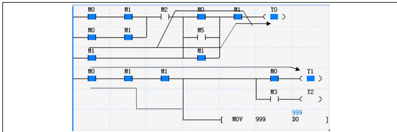
图4-2 能流传递及能流的驱动作用
