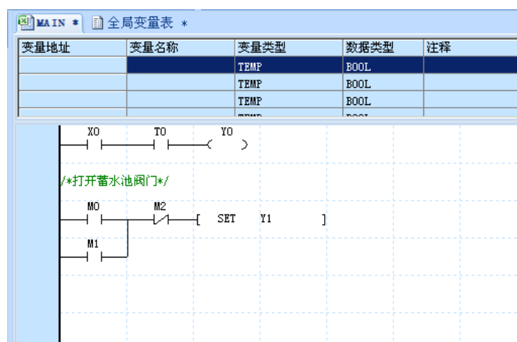
图4-8 未选中符号编址的状态
