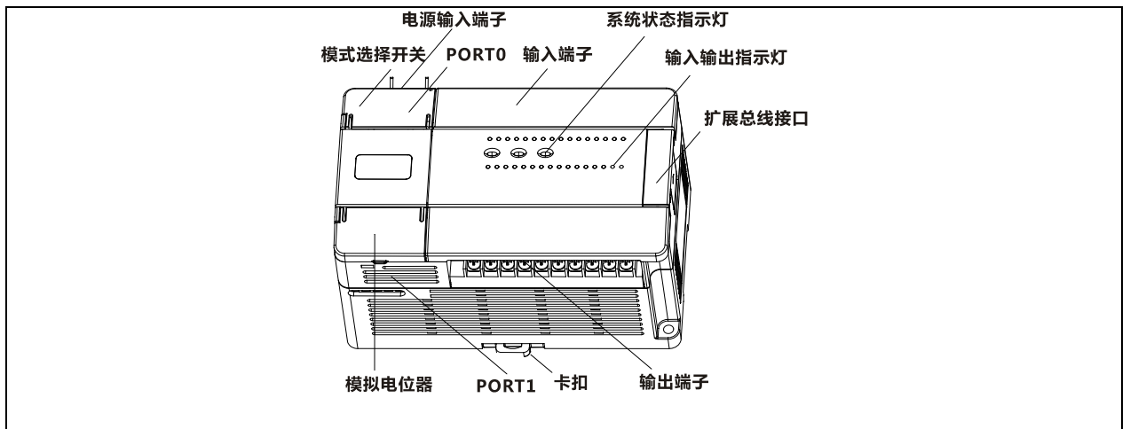
图1-2 MC100 系列主模块外形结构
