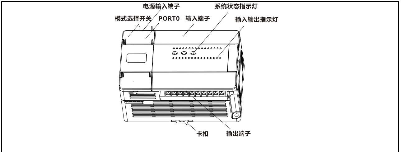
图1-1 MC80 系列主模块外形结构
