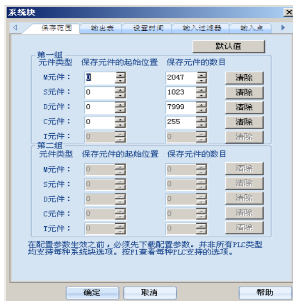
图2-3 配置保存元件地址范围
