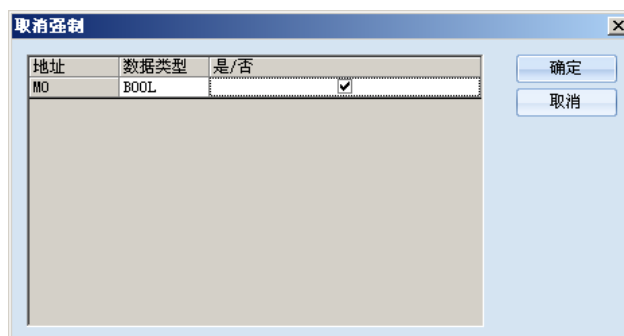
图2-25 取消强制对话框
