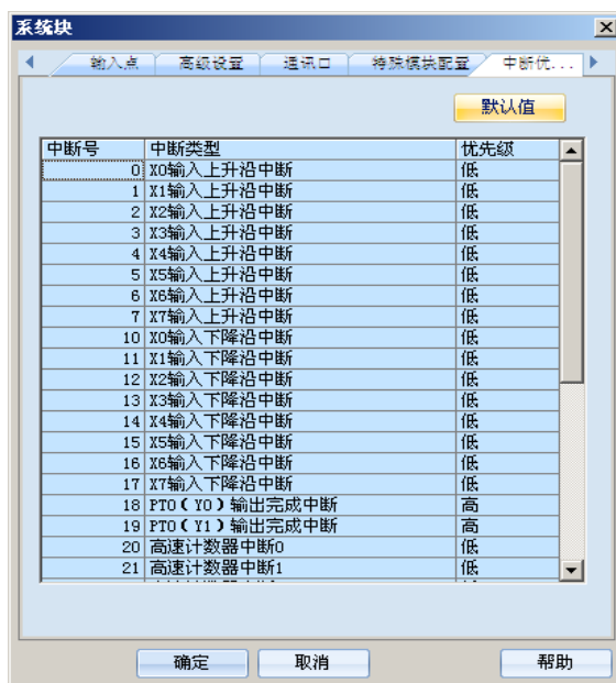
图2-12 设置中断优先级
