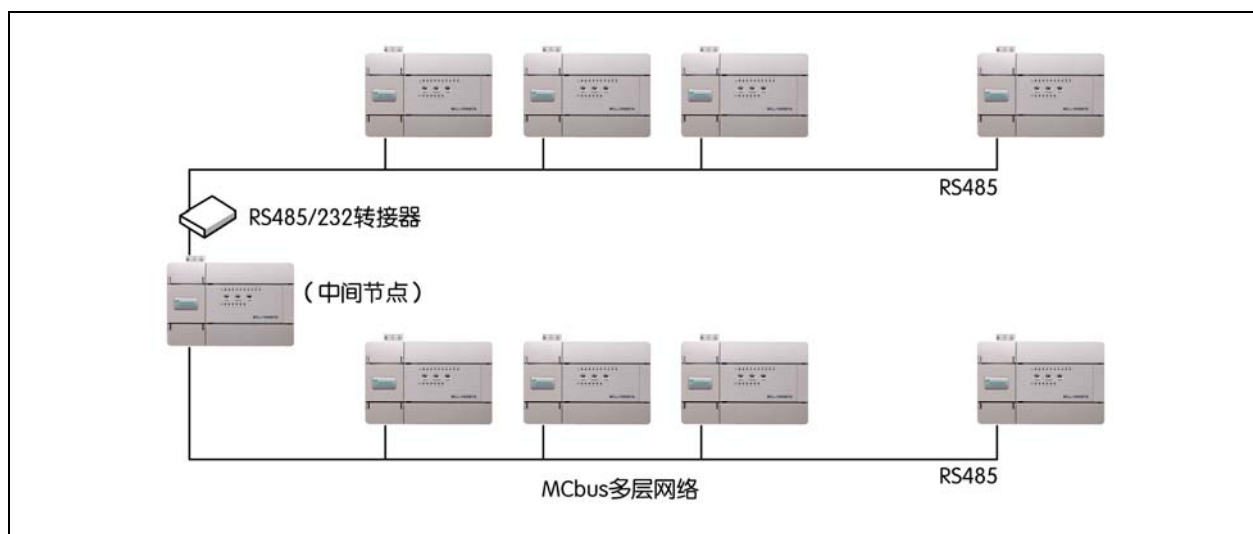
图10-8 MCbus 多层网络
