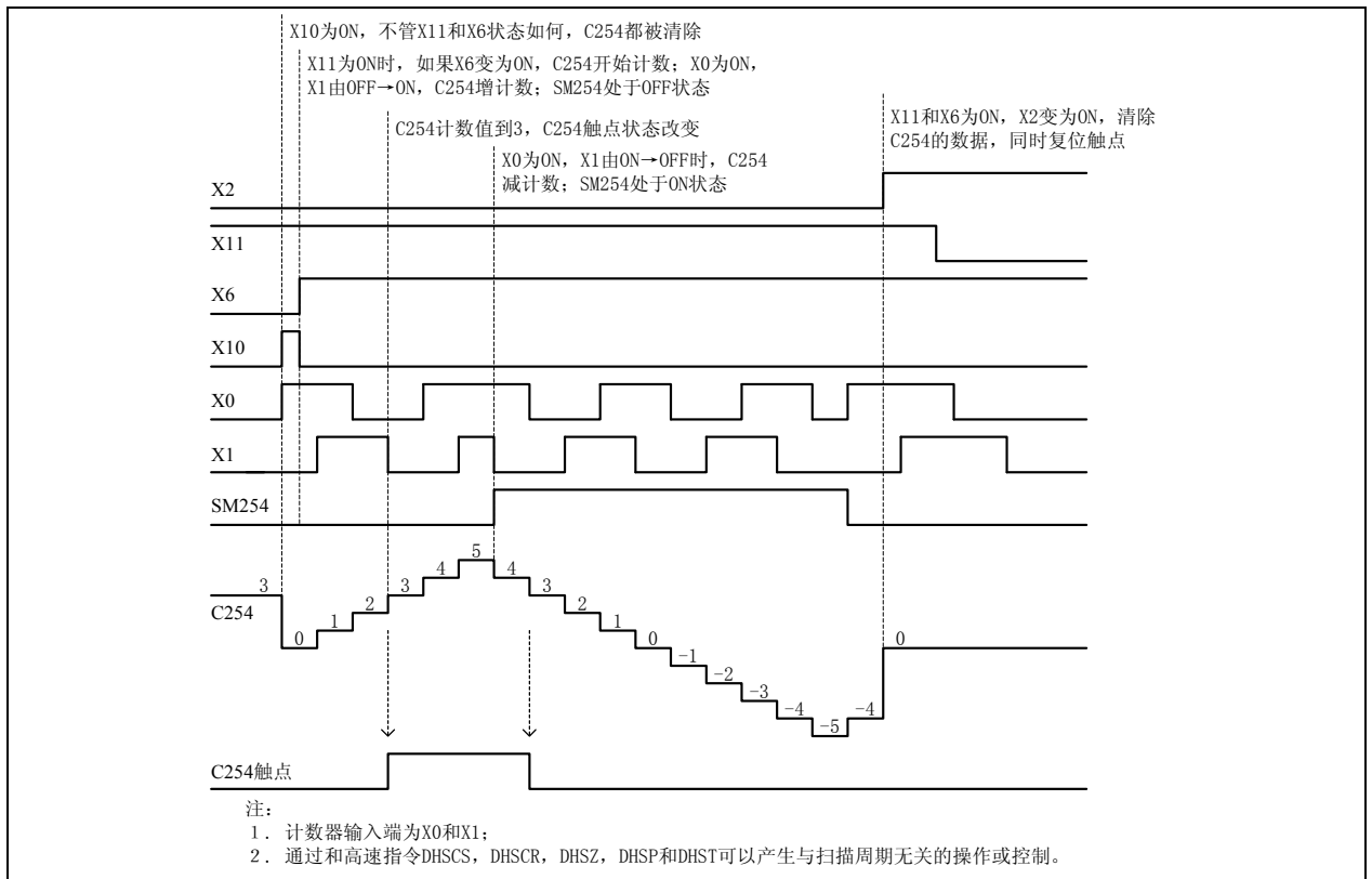
动作示例如下所示程序中触点的时序操作图:
