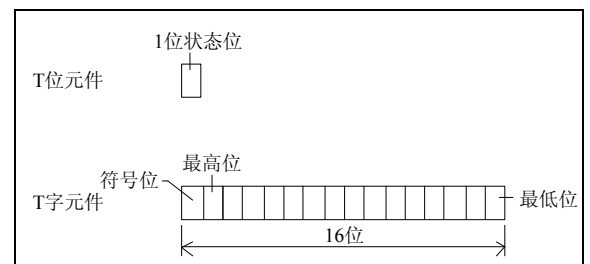
图3-3 T元件
