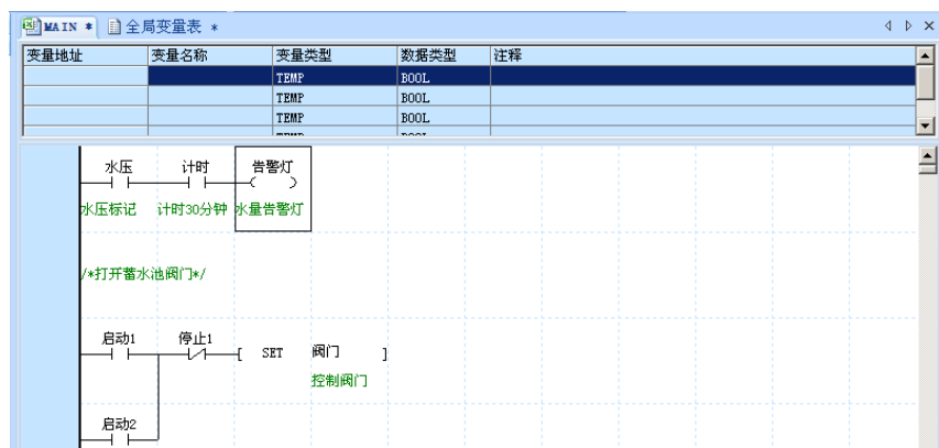
图4-10 显示元件注释时的梯形图程序
