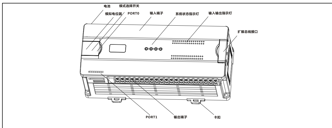
图1-3 MC200 系列主模块的外形结构与部件布局
