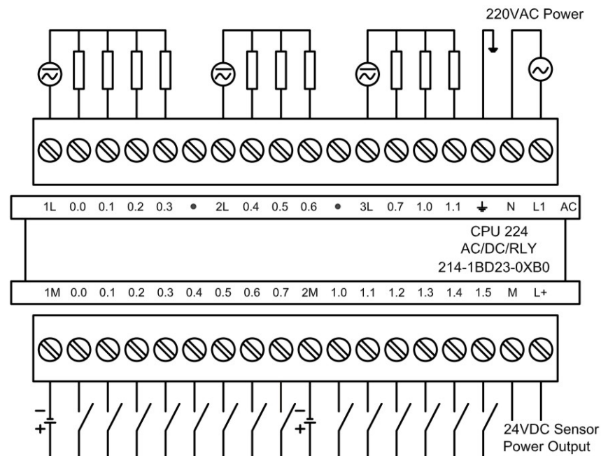
图3: CPU224 AC/DC/RLY接线图
