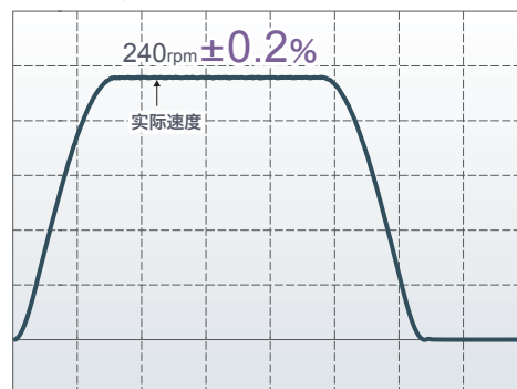
■ 匀速旋转时的速度波形
