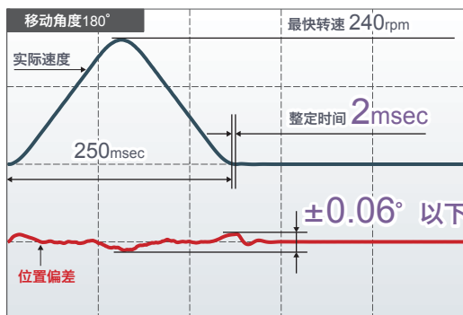
■ 定位时的速度波形
