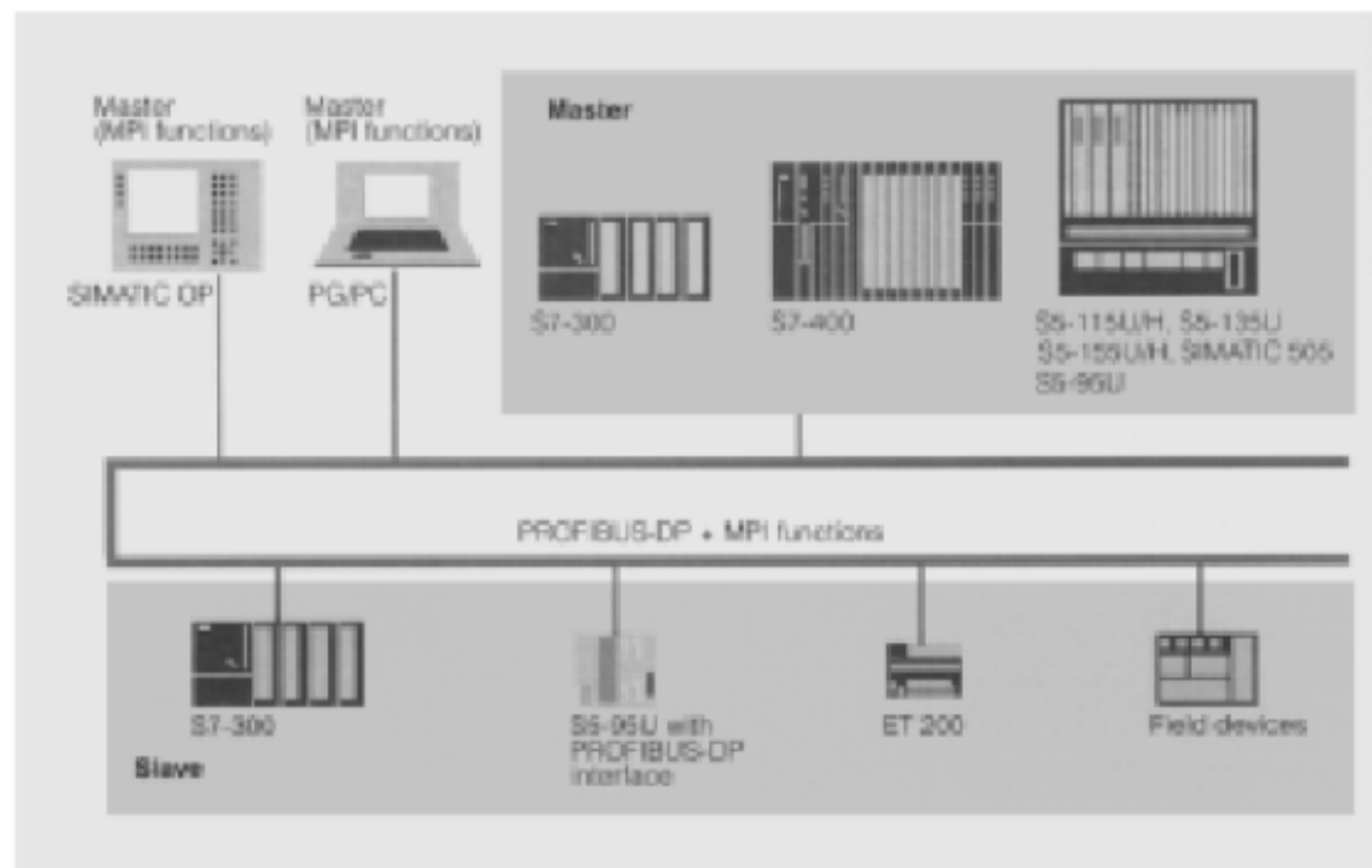
图 4 应用 PROFIBUS-DP 总线系统的联网
