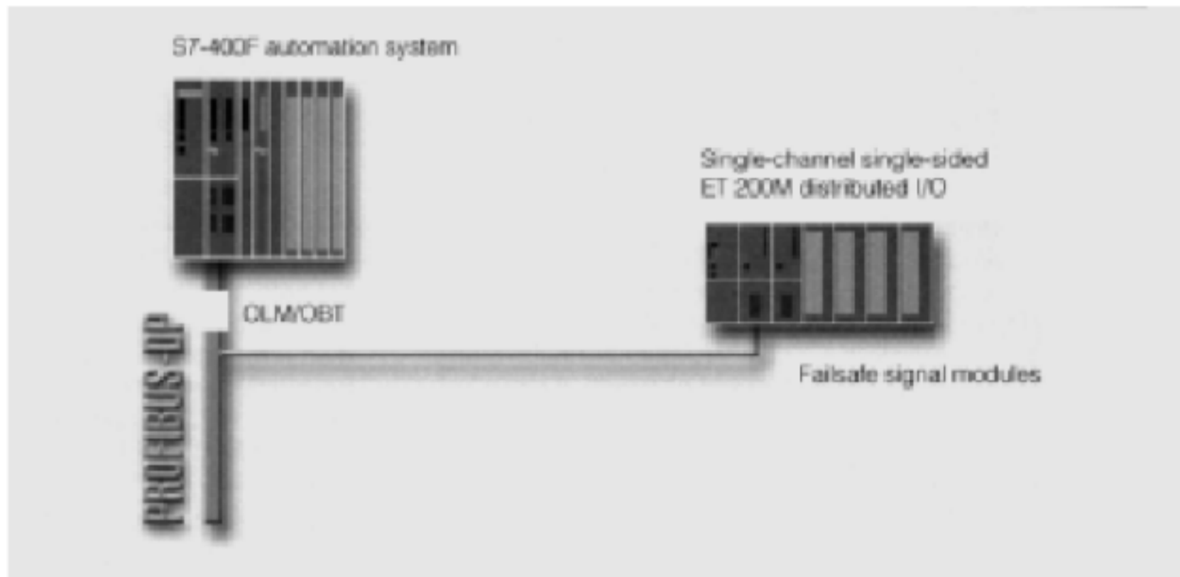
图 13 单通道单边 I/O 的配置
