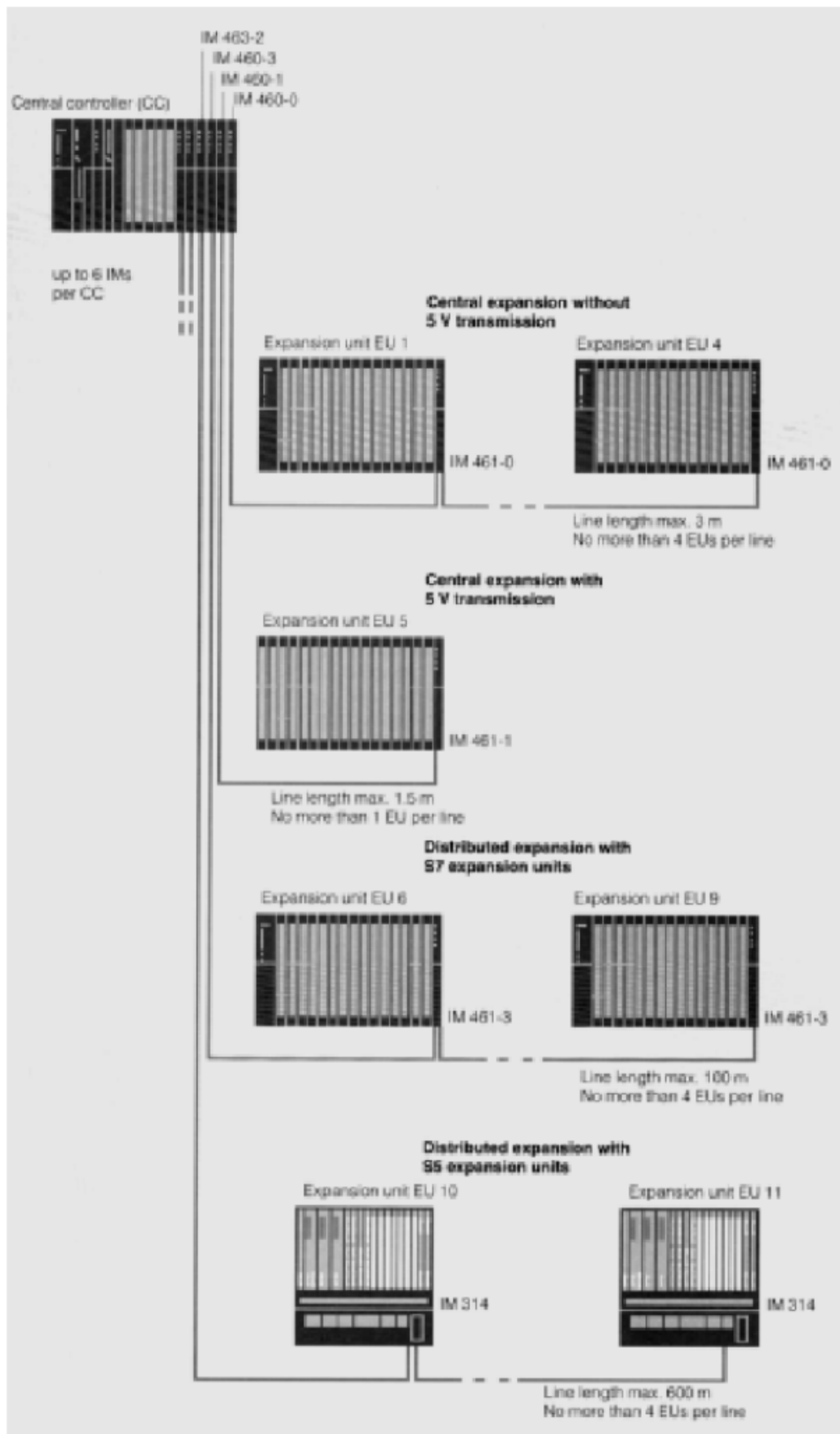
图 3 S7-400 可能的扩展型式
