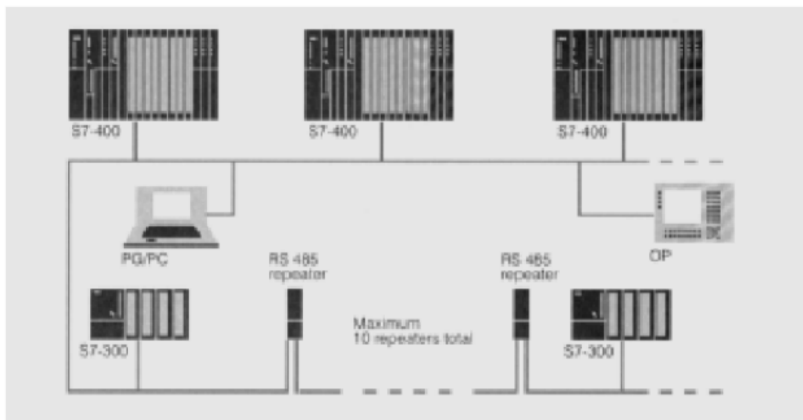
图 5 典型的带 MPI 接口的通讯配置
