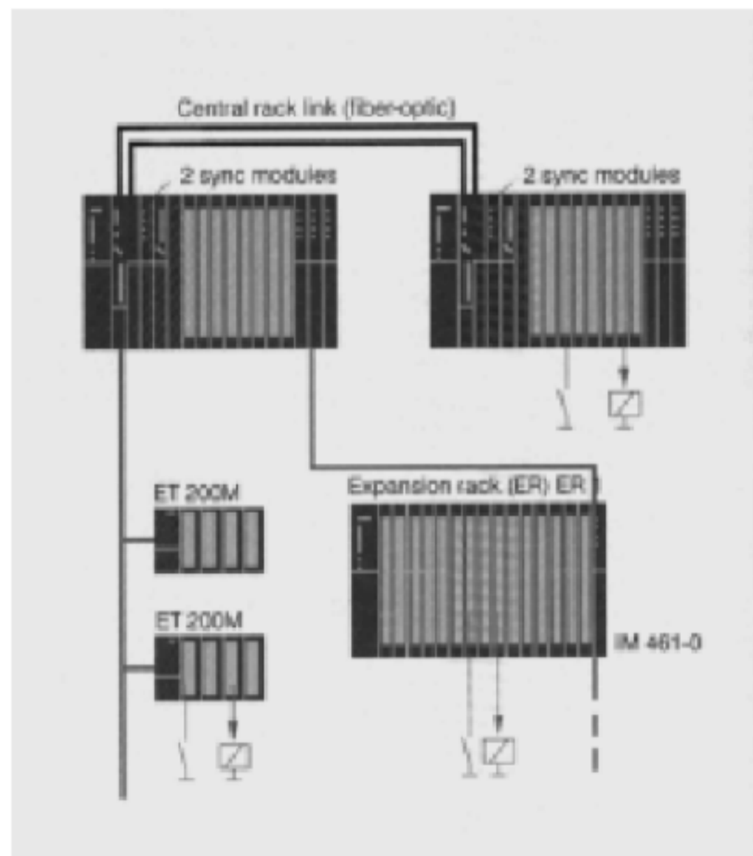
图 9 单边配置 (常规的可用性)
