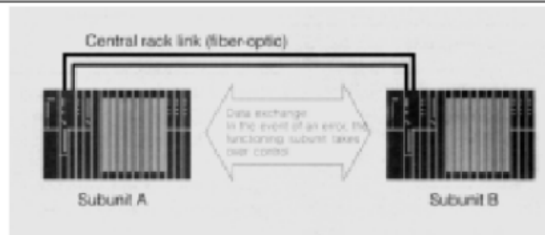
图 11 S7-400H 的工作原理
