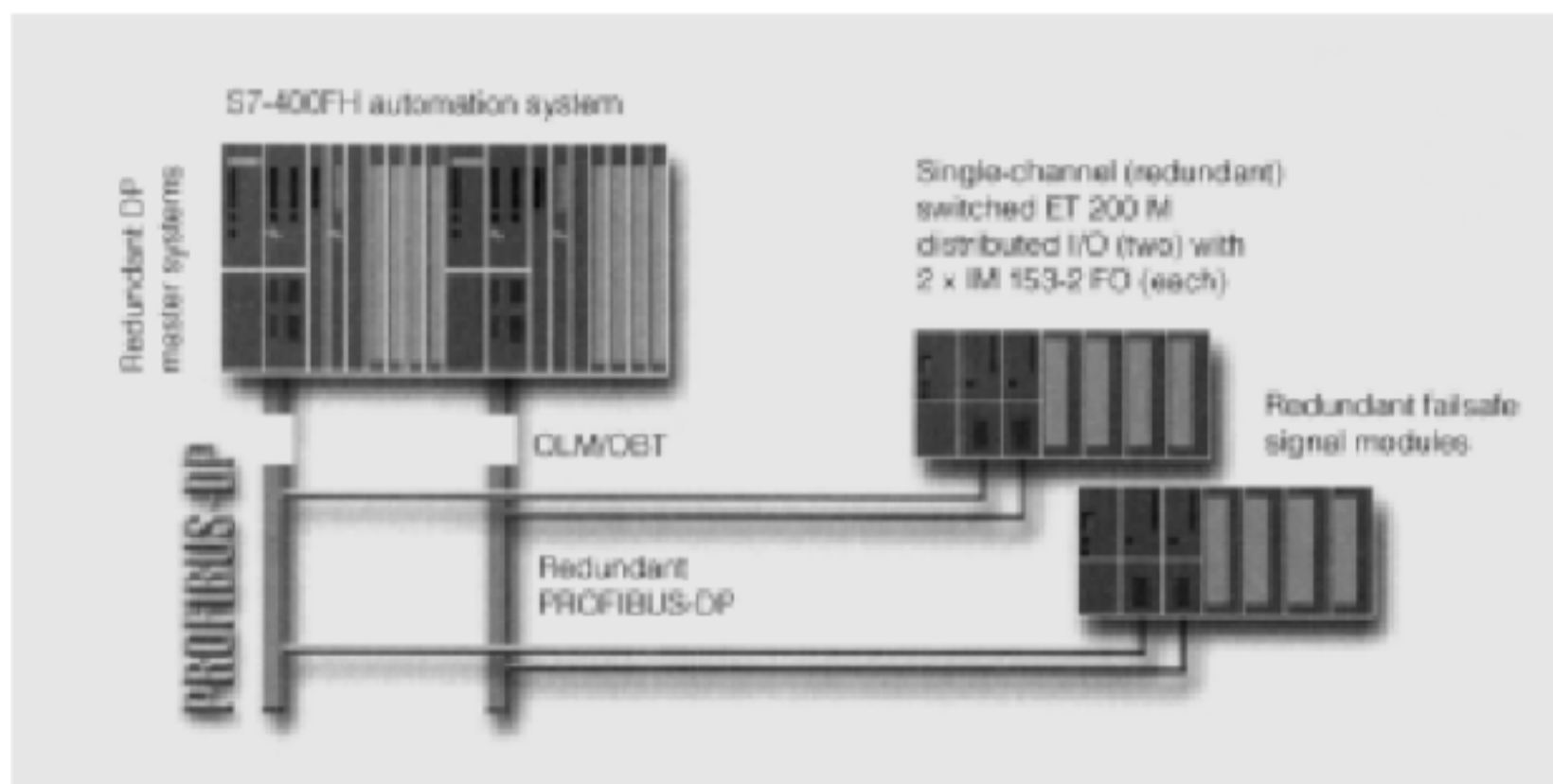
图 15 冗余切换式 I/O 的配置
