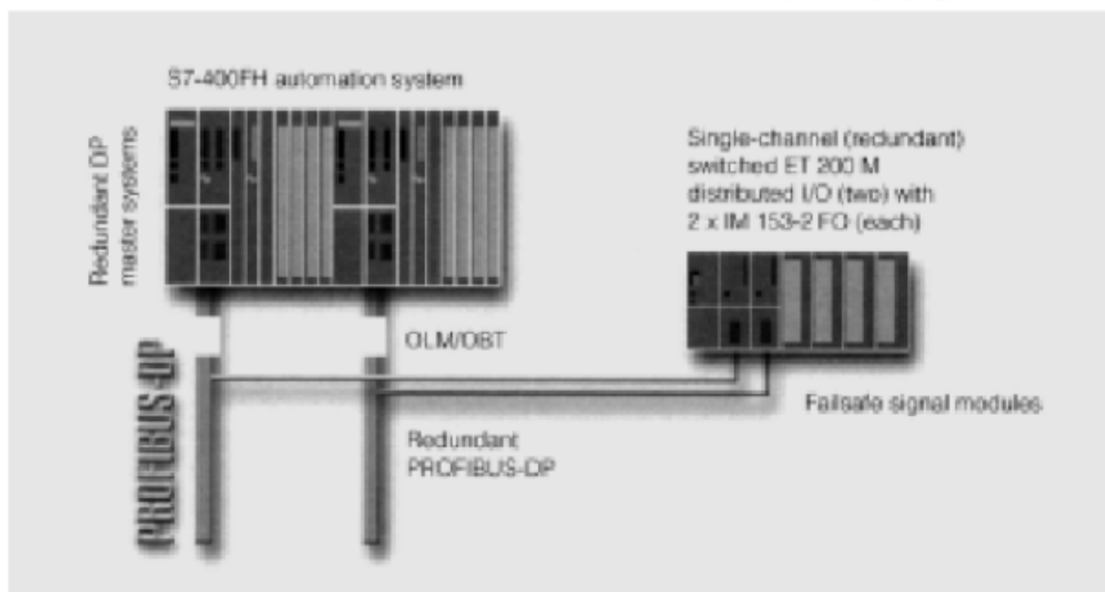
图 14 单通道、切换式 I/O 的配置
