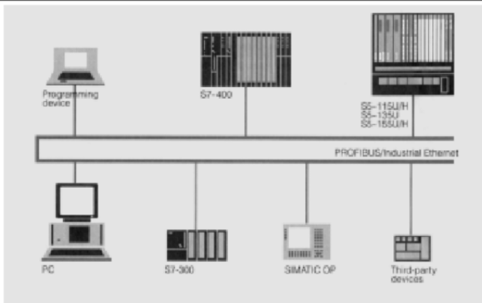
图 7 使用 PROFIBUS 或工业以太网的联网
