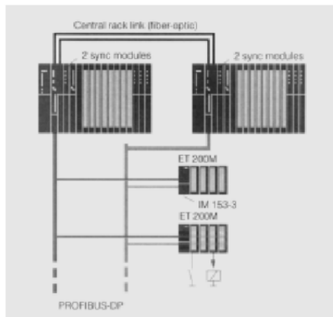
图 10 切换式配置
