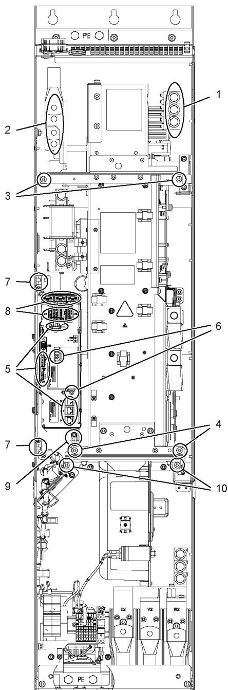
图 8-5 更换 FX 型调节型电源模块和电机模块的功率单元
