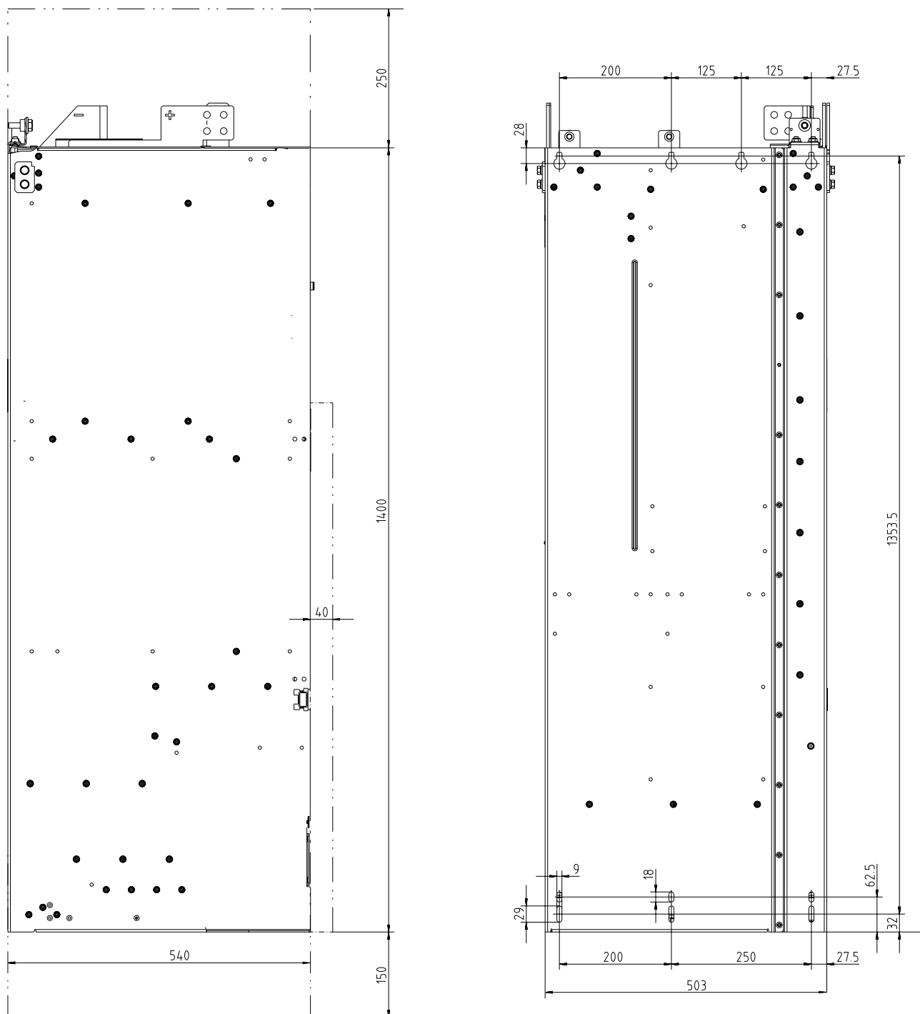
图 4-8 HX 型电机模块的外形尺寸图 侧视图和背视图
