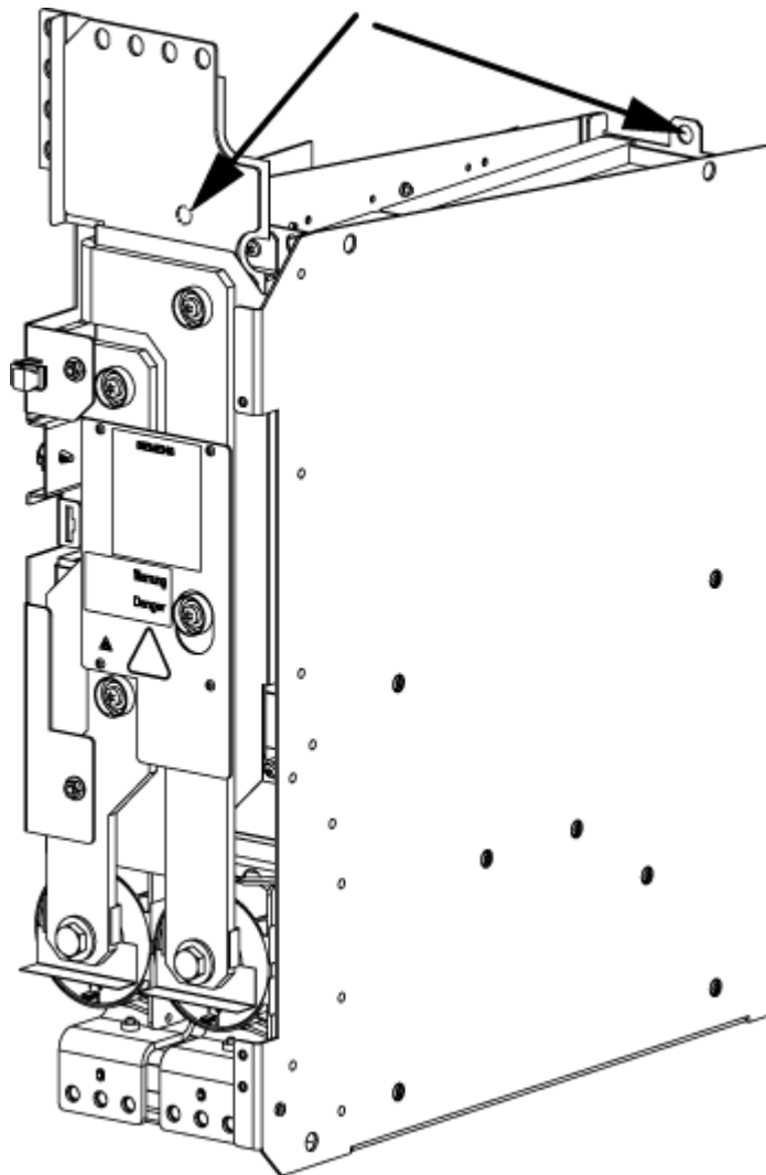
图 8-3 功率单元（HX, JX 型）上的吊孔
