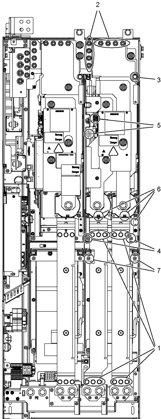
图 8-8 更换 HX 型非调节型/调节型电源模块和电机模块的右侧功率单元
