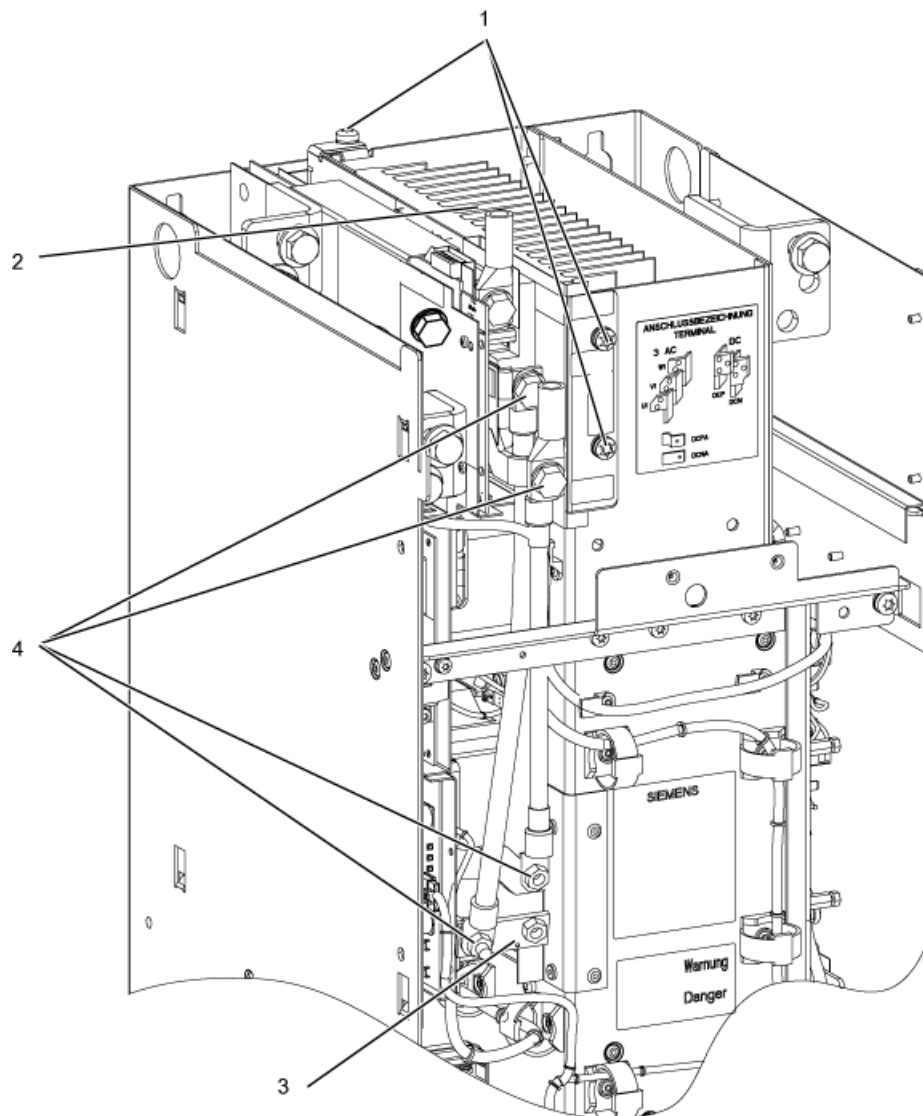
图 5-12 将制动模块安装到 FB 型基本型电源模块中
