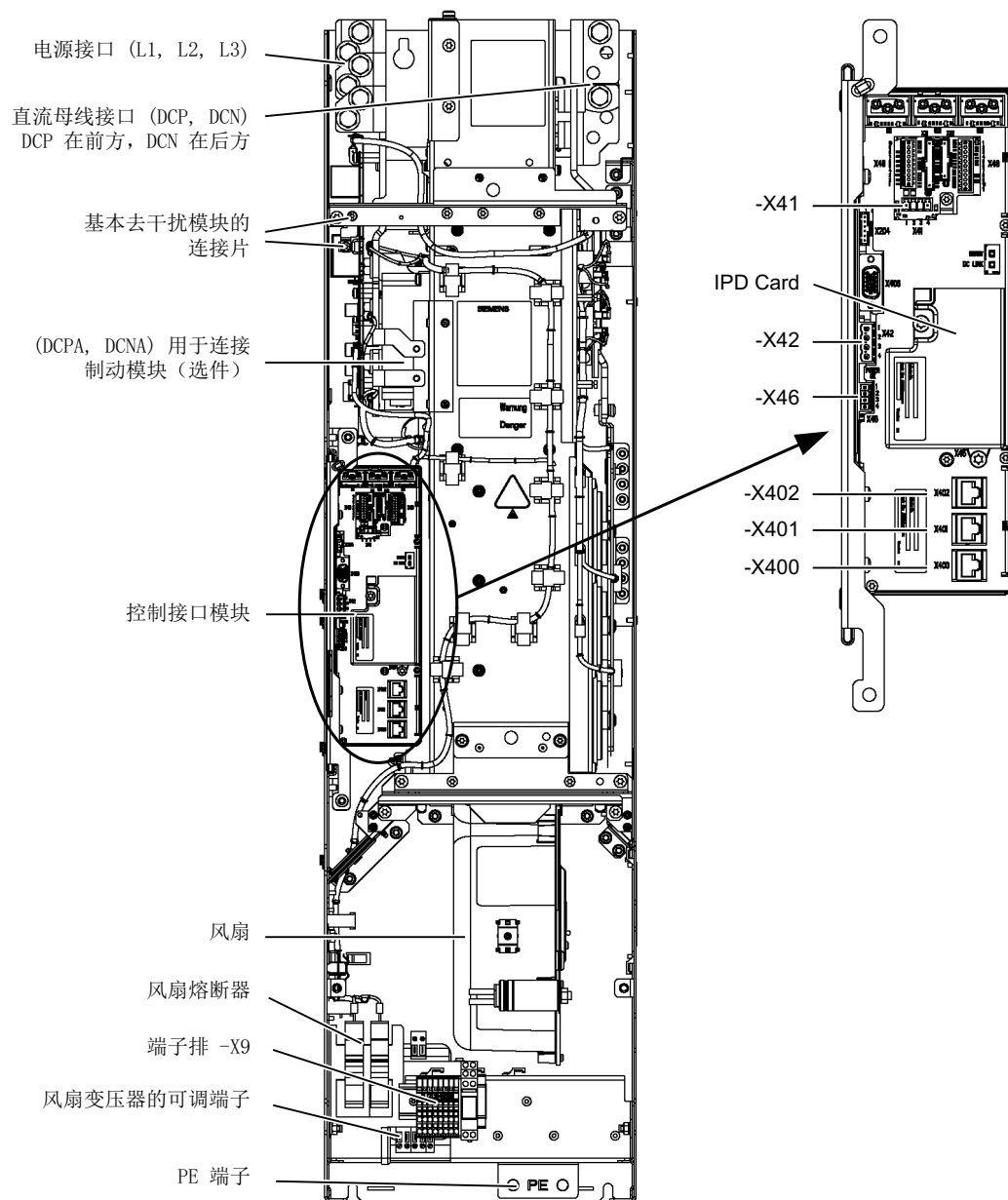
图 3-1 FB 型基本型电源模块
