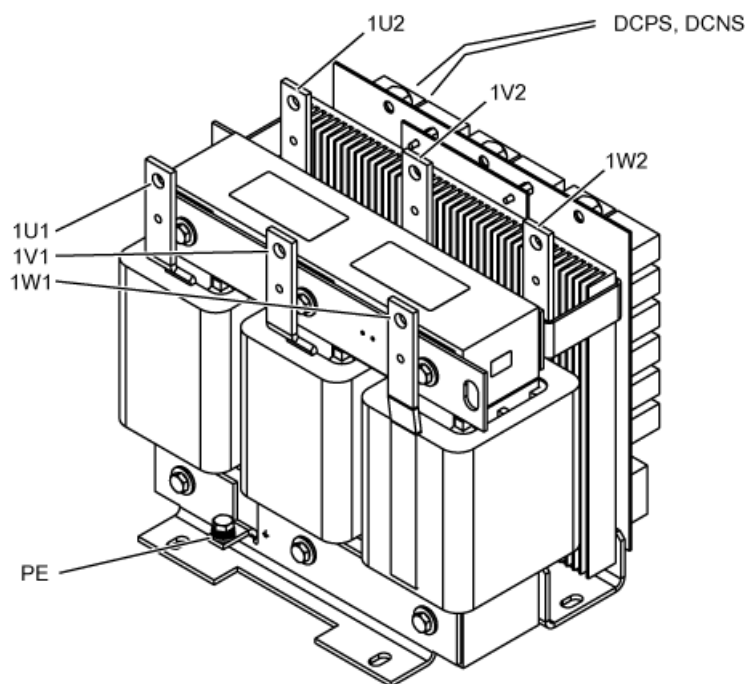
图 6-14 带有电压峰值限制器的紧凑型 du/dt 滤波器的接口一览，类型 2
