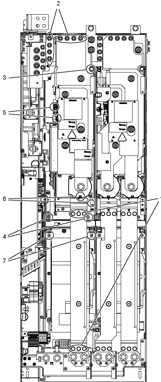
图 8-7 更换 HX 型非调节型/调节型电源模块和电机模块的左侧功率单元
