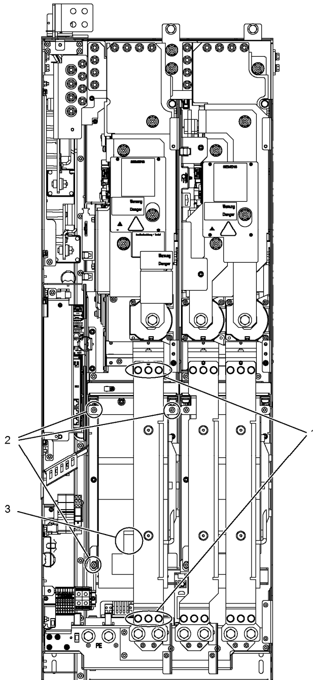
图 8-19 更换 HX 型非调节型/调节型电源模块、电机模块、左侧功率单元的风扇
