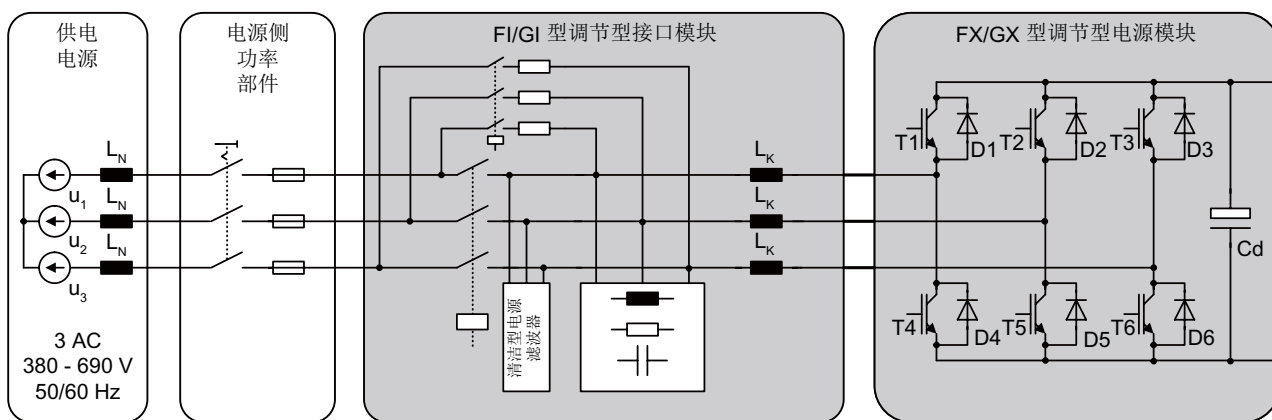
图 3-27 调节型电源 F1/FX 和 G1/GX 型的概览
