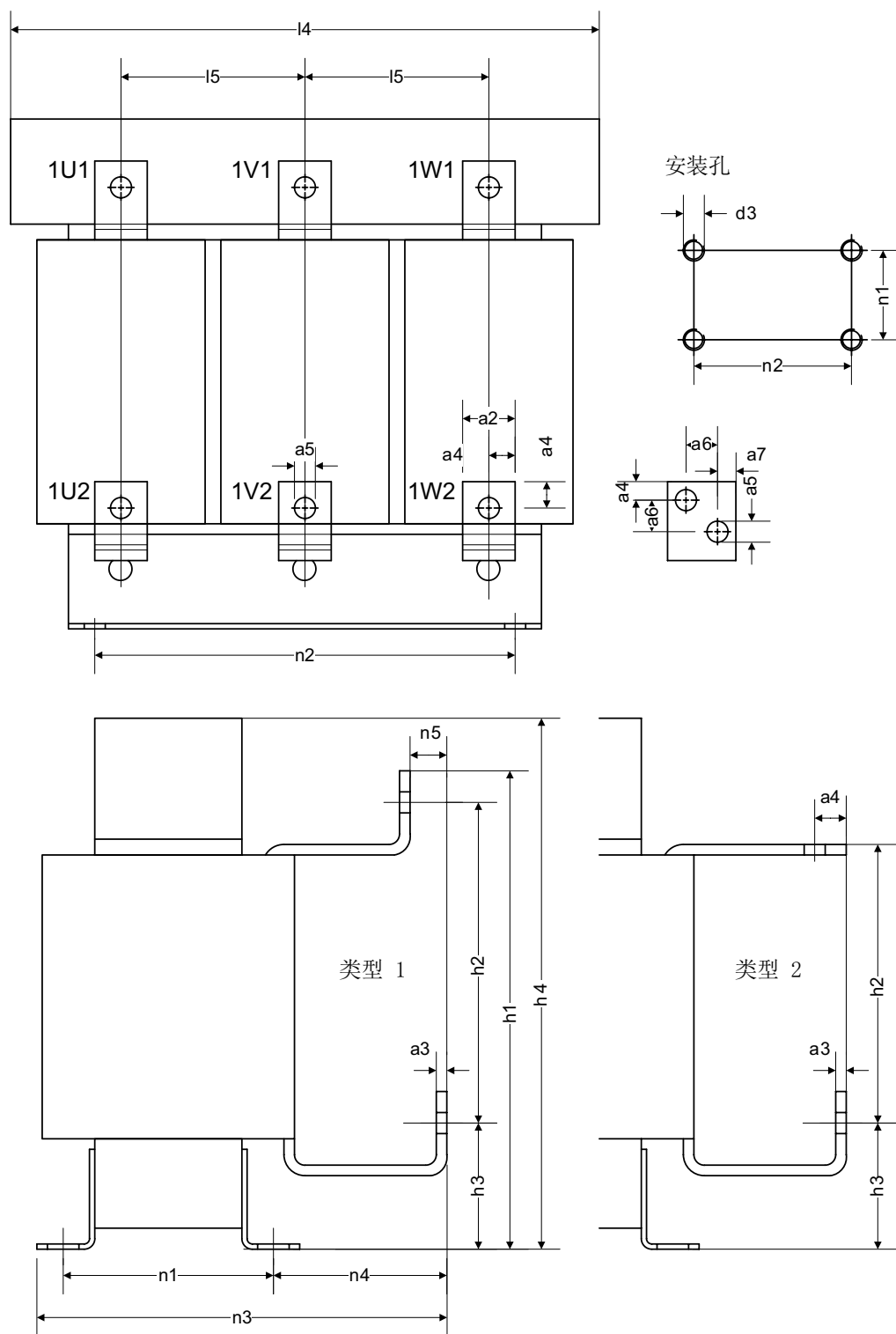
图 6-3 电机电抗器的外形尺寸图
