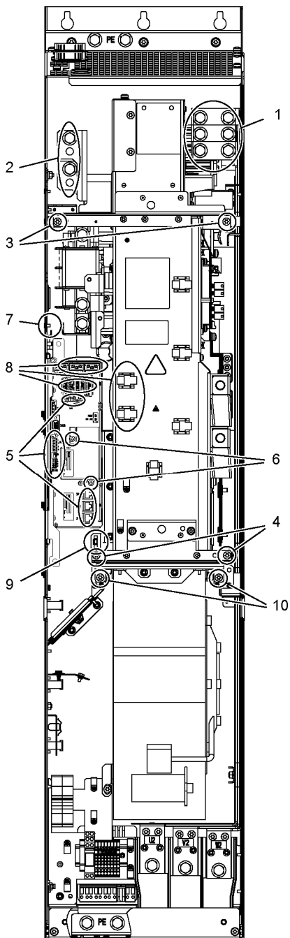
图 8-6 更换 GX 型非调节型/调节型电源模块和电机模块的功率单元
