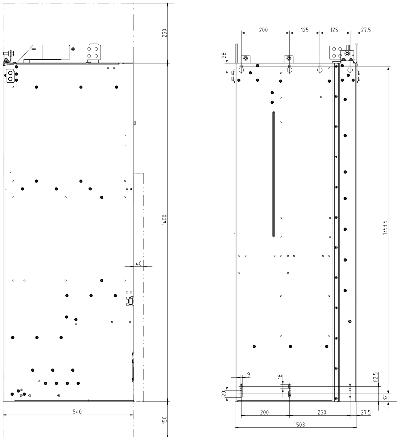
图 3-19 HX 型非调节型电源模块的外形尺寸图 侧视图和背视图
