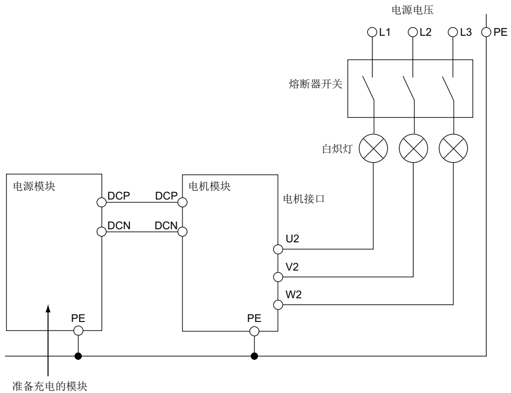
图 8-30 电源模块的充电回路
