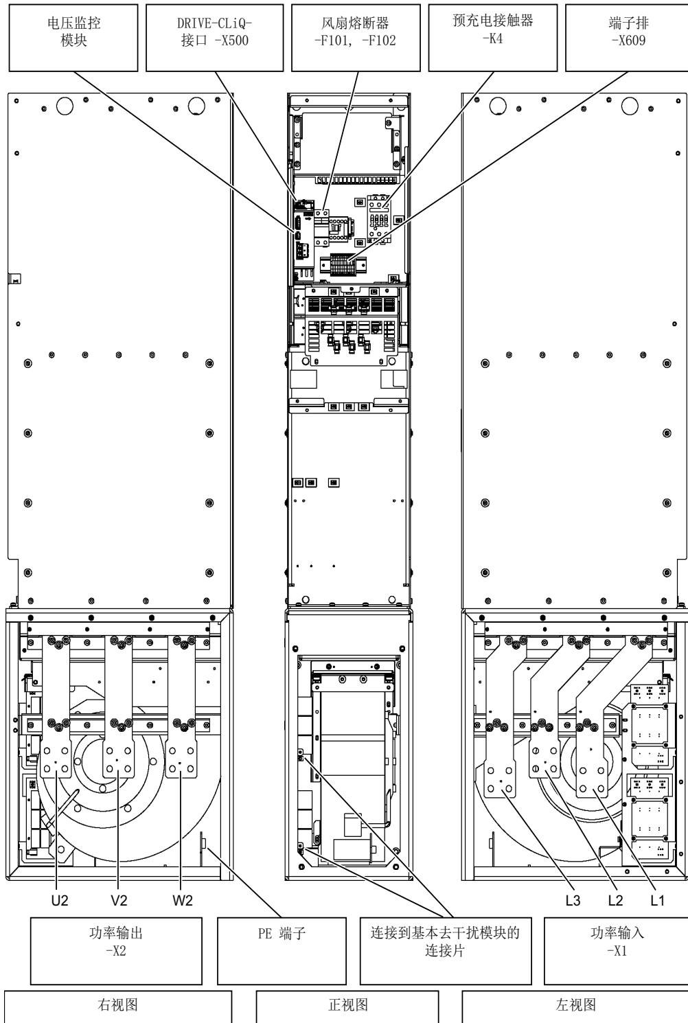
图 2-12 HI 型调节型接口模块的接口概览
