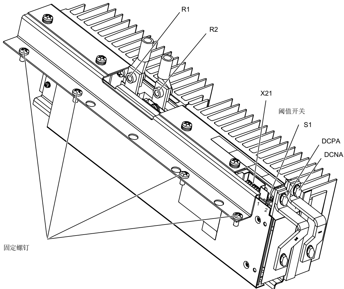
图 5-4 制动模块，用于 HX / JX 型非调节型/调节型电源模块/电机模块
