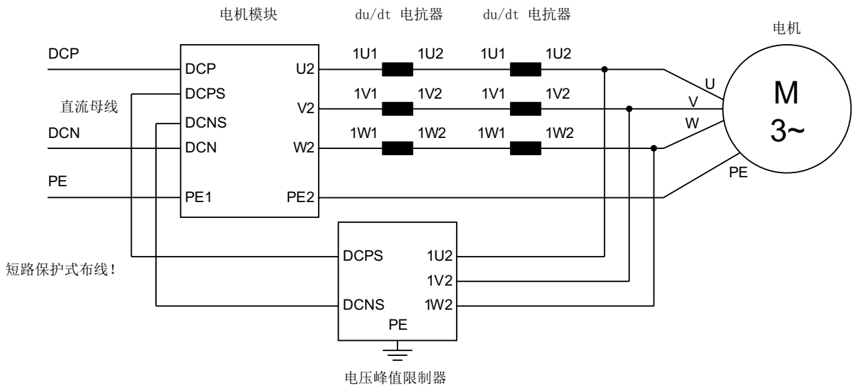
图 6-8 连接带有电压峰值限制器、两个 du/dt 电抗器的 du/dt 滤波器
