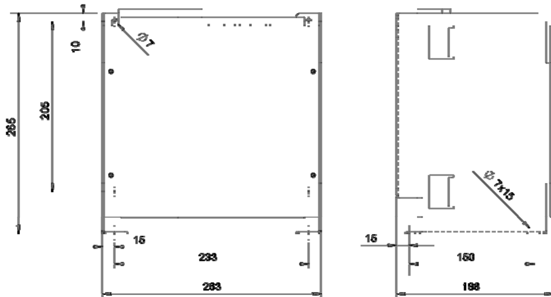
图 6-10 1 类电压峰值限制器的外形尺寸图
