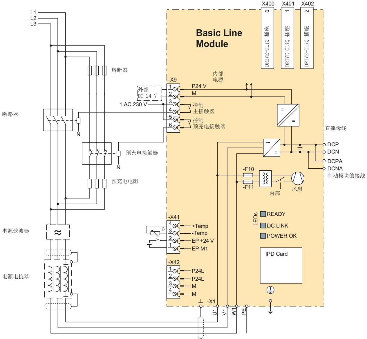
图 3-4 GD 型基本型电源模块的接线示例
