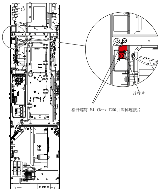
图 3-8 取出 FB 型调节型接口模块中的基本去干扰模块的连接片
