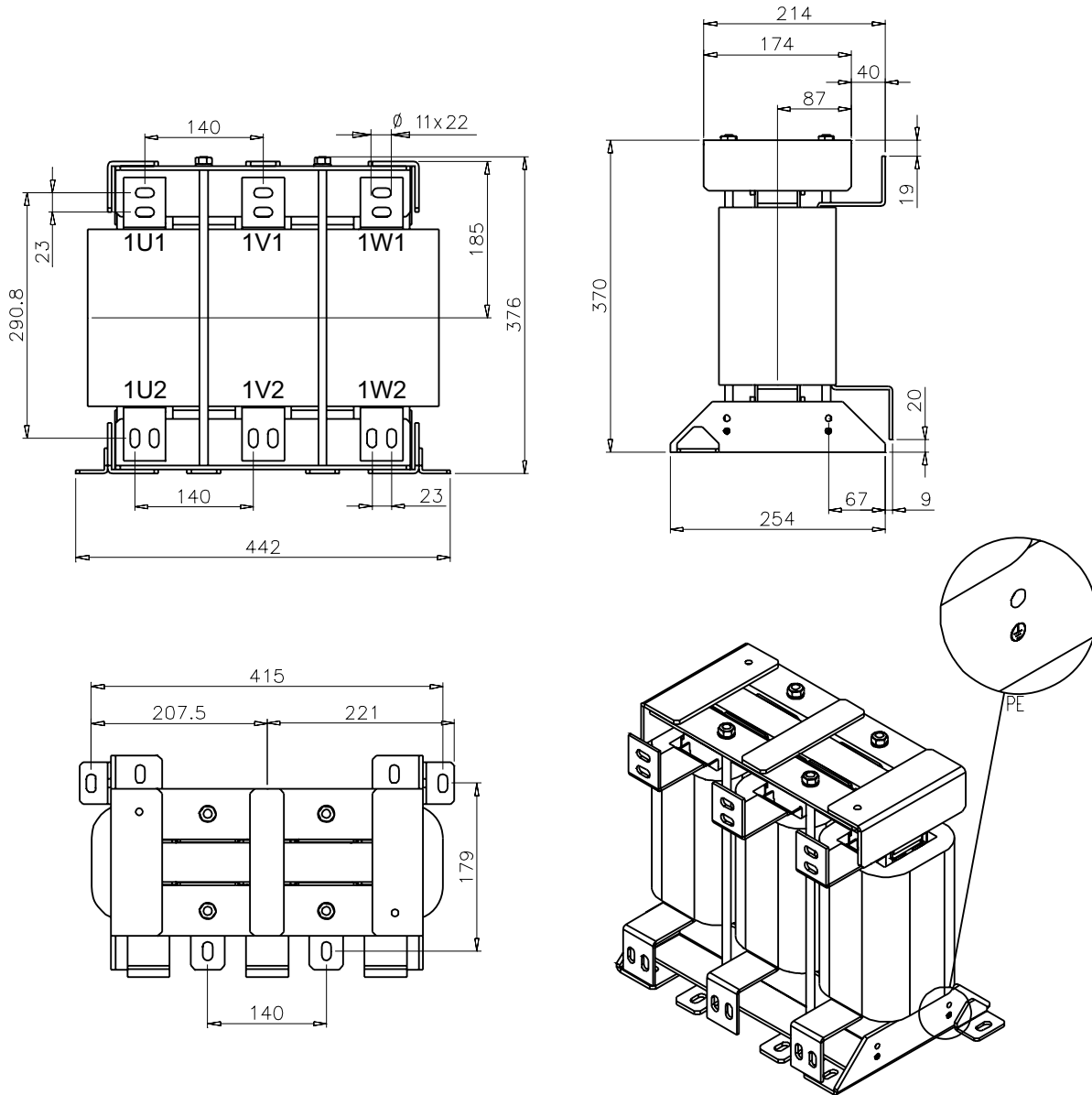
图 2-5 电源电抗器 6SL3000-0EE38-8AA0 的外形尺寸图，所有尺寸以 mm 为单位
