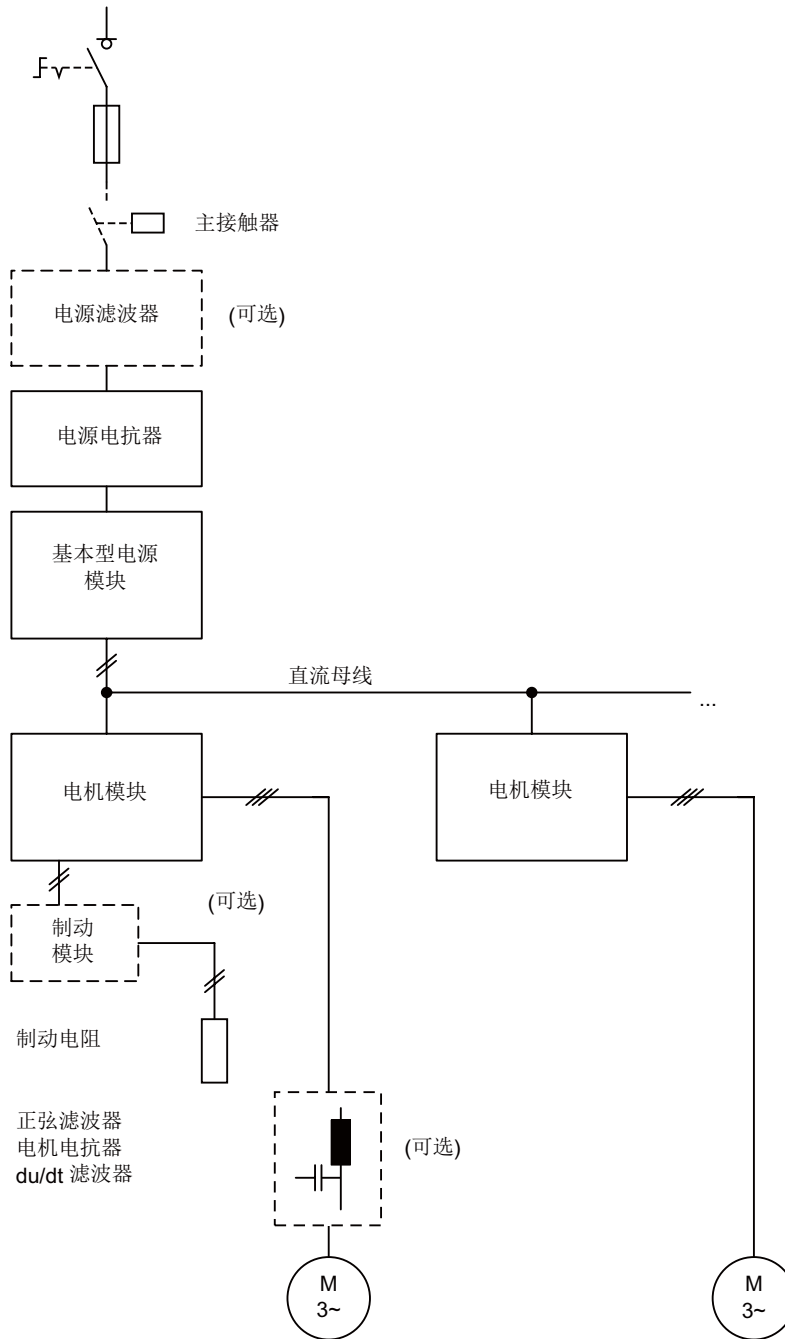
图 1-6 SINAMICS S120 和非受控型电源模块组成的驱动系统的基本结构
