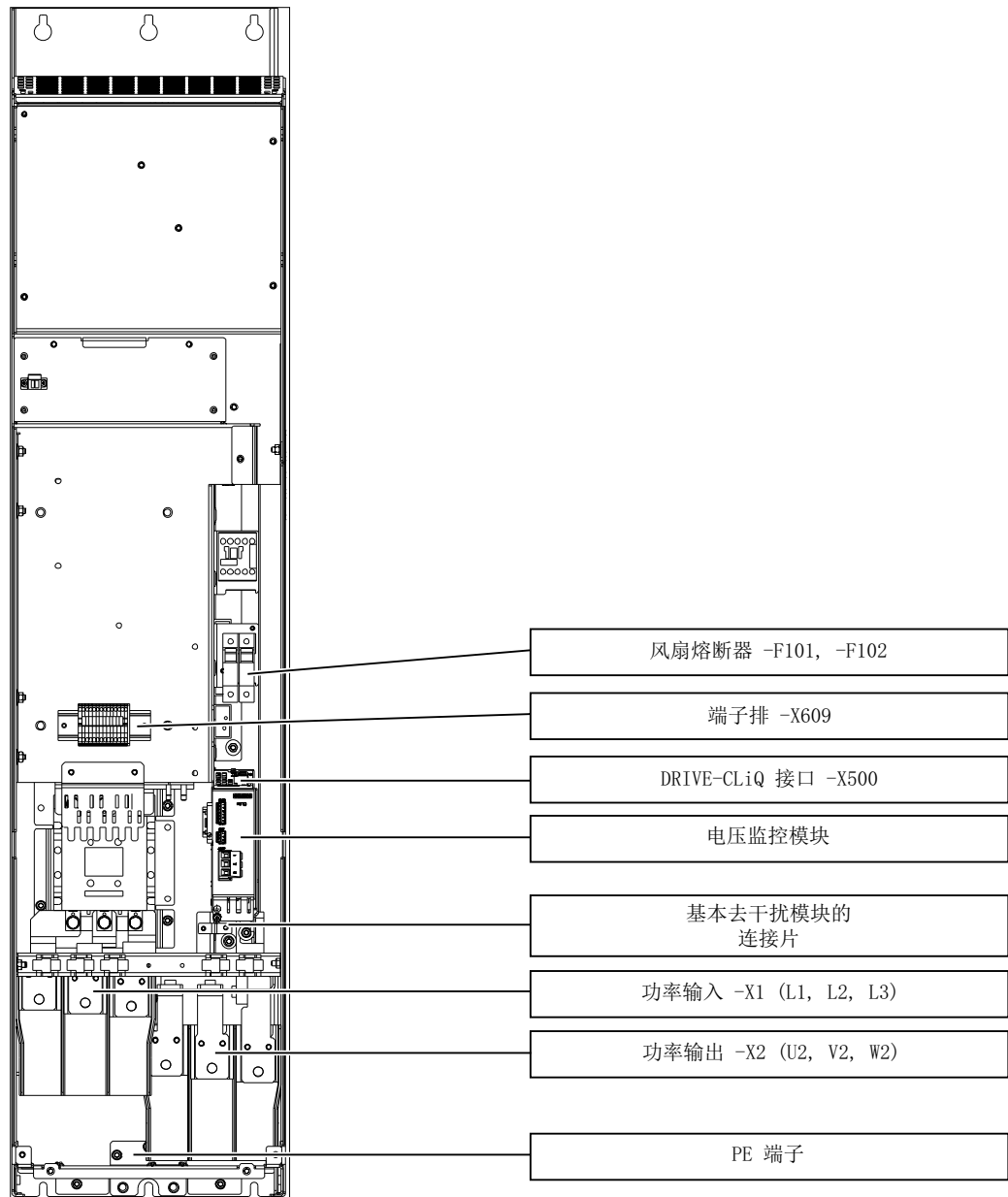
图 2-10 FI 型调节型接口模块的接口概览
