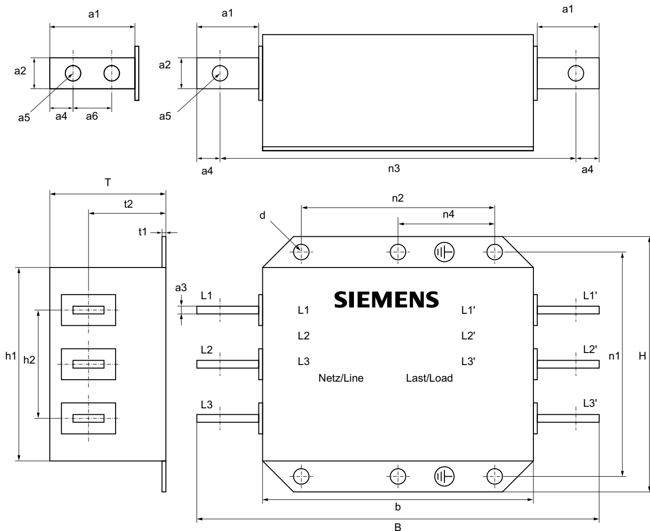
图 2-1 和基本型电源模块配套的电源滤波器的外形尺寸图
