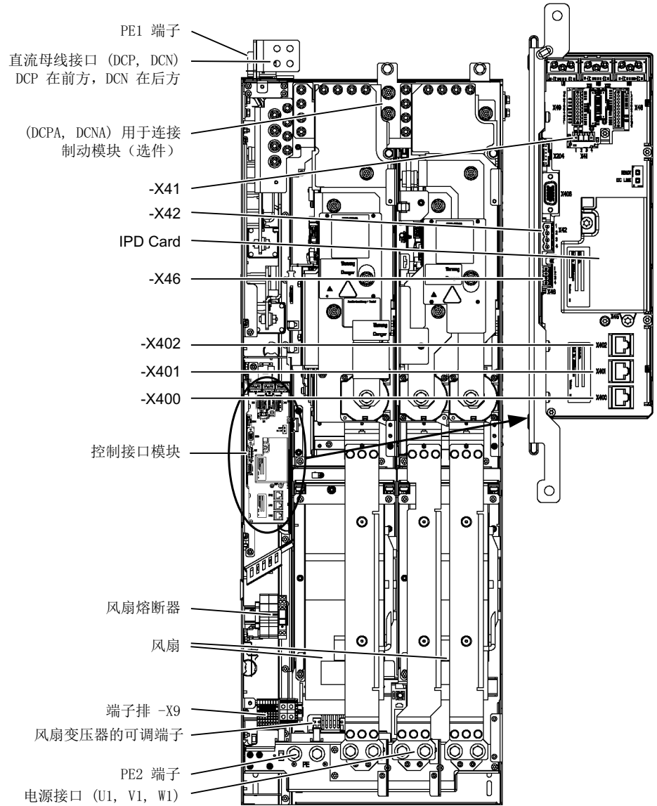
图 3-31 HX 型调节型电源模块
