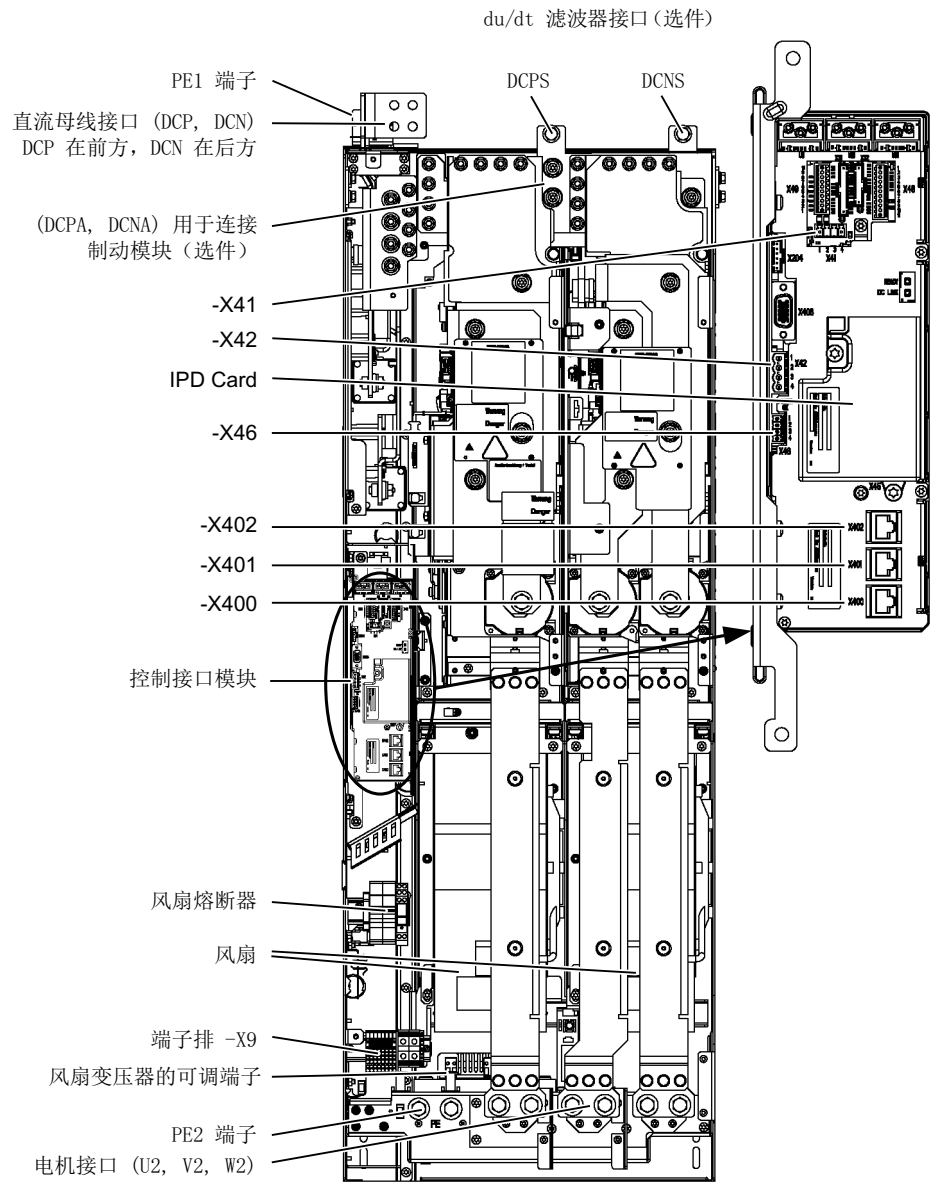
图 4-3 电机模块，HX 型
