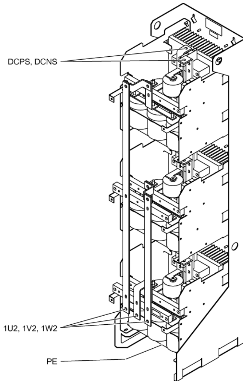
图 6-6 3 类电压峰值限制器的接口概览
