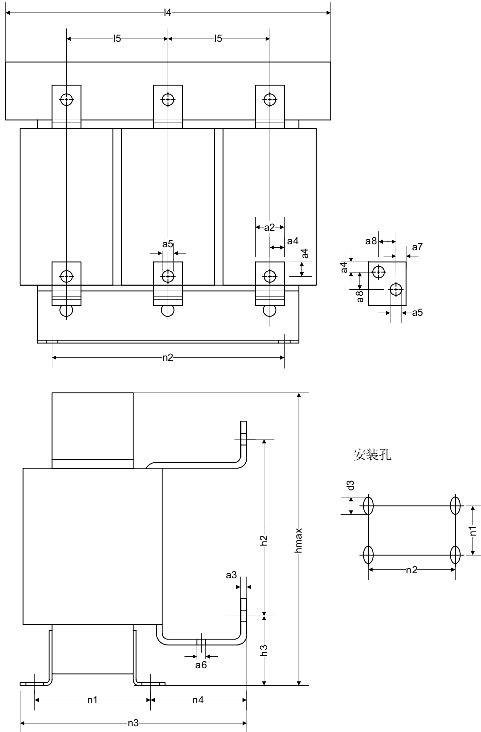
图 6-9 du/dt 电抗器的外形尺寸图
