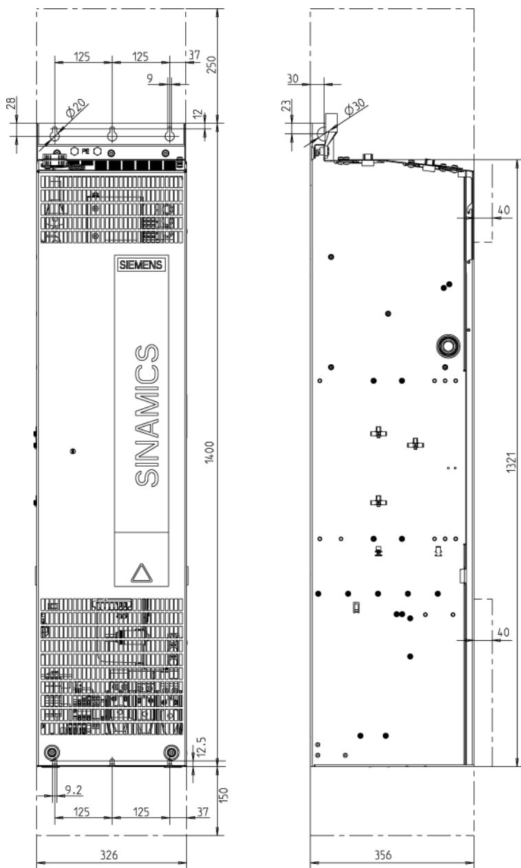
图 3-34 FX 型调节型电源模块的外形尺寸图 正视图和侧视图
