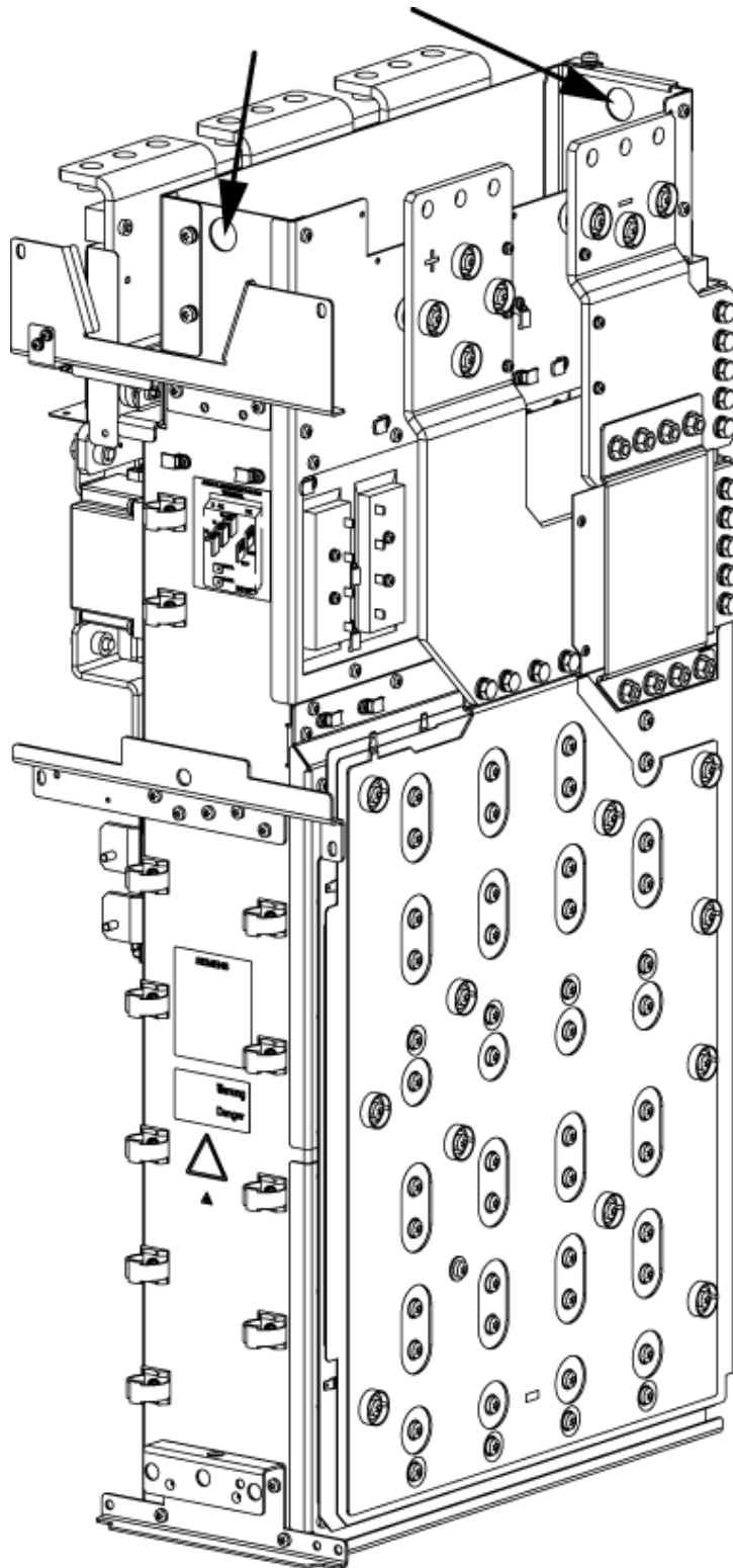
图 8-4 GB、GD 型功率单元上的吊孔
