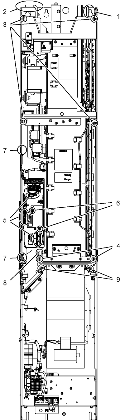
图 8-11 更换 GB、GD 型基本型电源模块的功率单元
