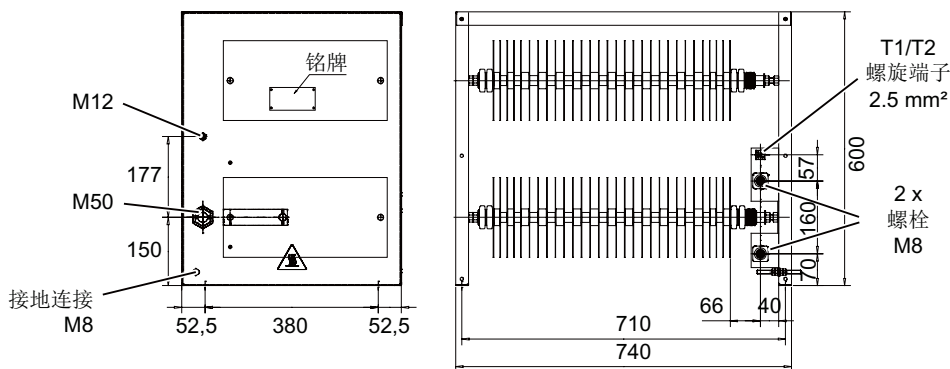
图 5-14 制动电阻 25 kW / 125 kW 的外形尺寸图
