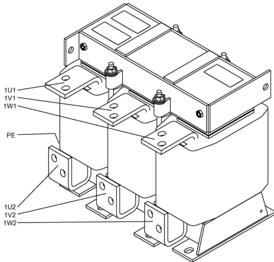
图 6-16 带有电压峰值限制器的紧凑型 du/dt 滤波器的接口一览，类型 4： du/dt 电抗器
