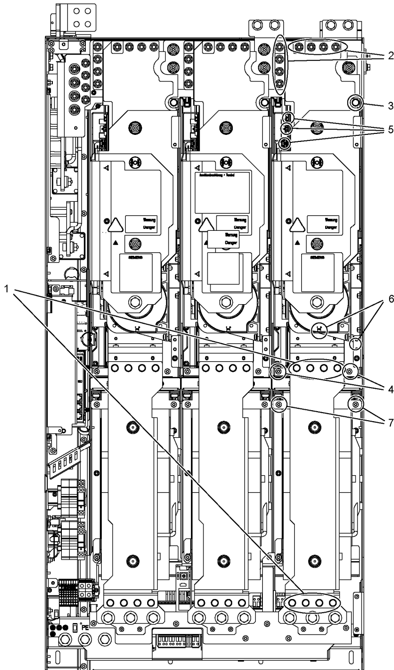
图 8-9 更换 JX 型非调节型/调节型电源模块和电机模块的功率单元
