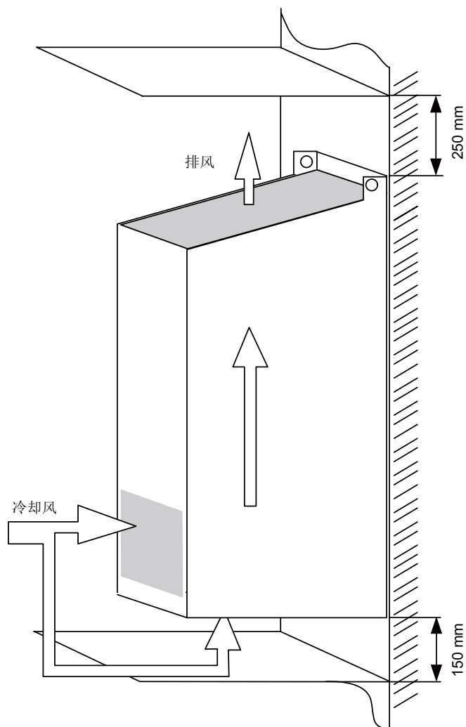
图 7-1 FI, GI 型调节型接口模块的通风
