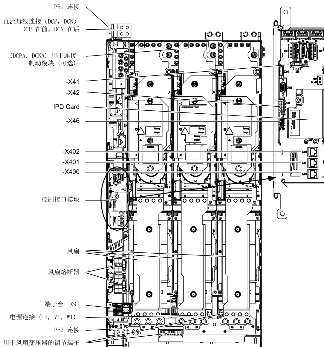
图 3-32 JX 型调节型电源模块
