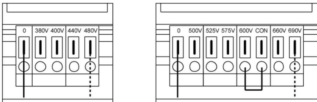
图 3-25 风扇变压器的可调端子(3 AC 380 到 480 V / 3 AC 500 到 690 V)
