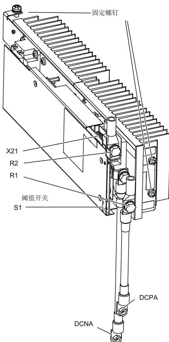
图 5-3 制动模块，用于 GX 型非调节型/调节型电源模块/电机模块和 GB、GD 型基本型电源模块
