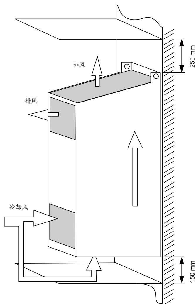
图 7-3 FX, GX 型非调节型/调节型电源模块和电机模块的通风
