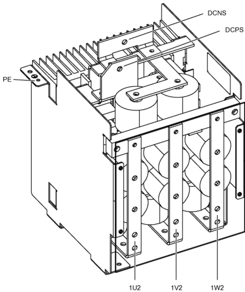
图 6-17 带有电压峰值限制器的紧凑型 du/dt 滤波器的接口一览，类型 4：电压峰值限制器
