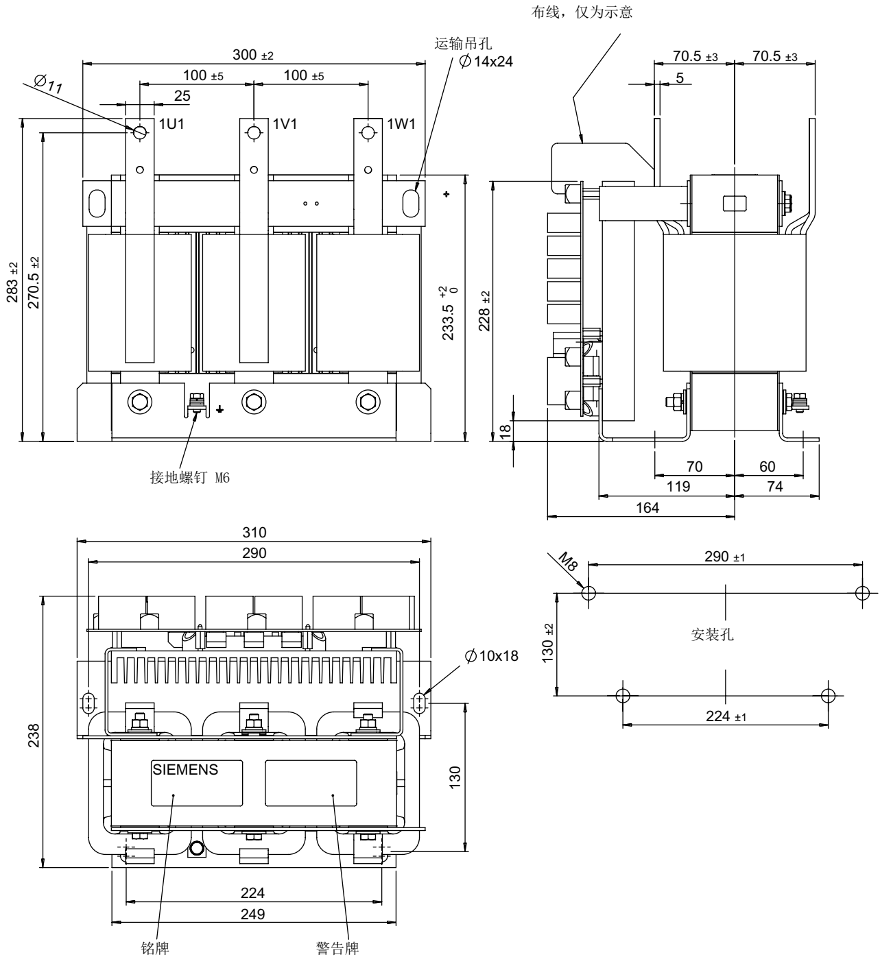
图 6-20 带有电压峰值限制器的紧凑型 du/dt 滤波器的尺寸图，类型 1
