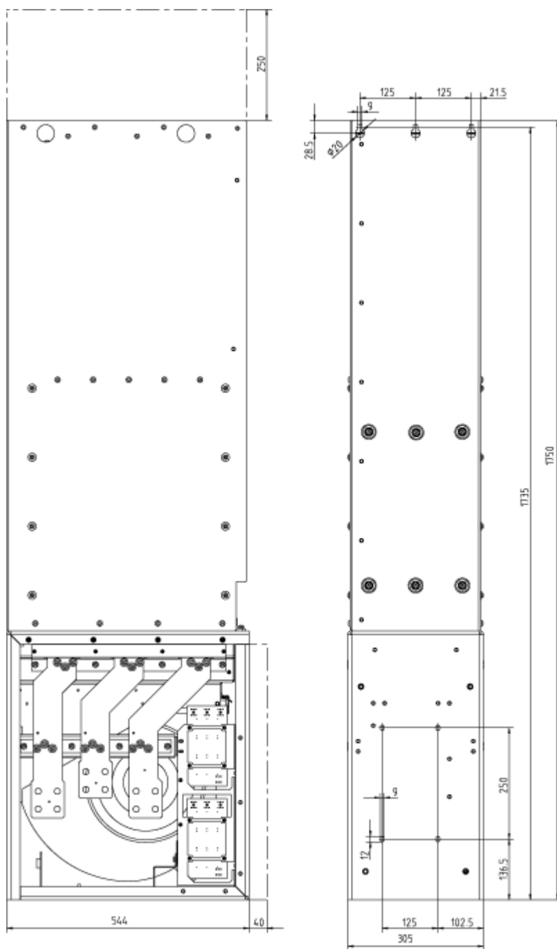
图 2-19 HI 型调节型接口模块的外形尺寸图。侧视图和背视图
