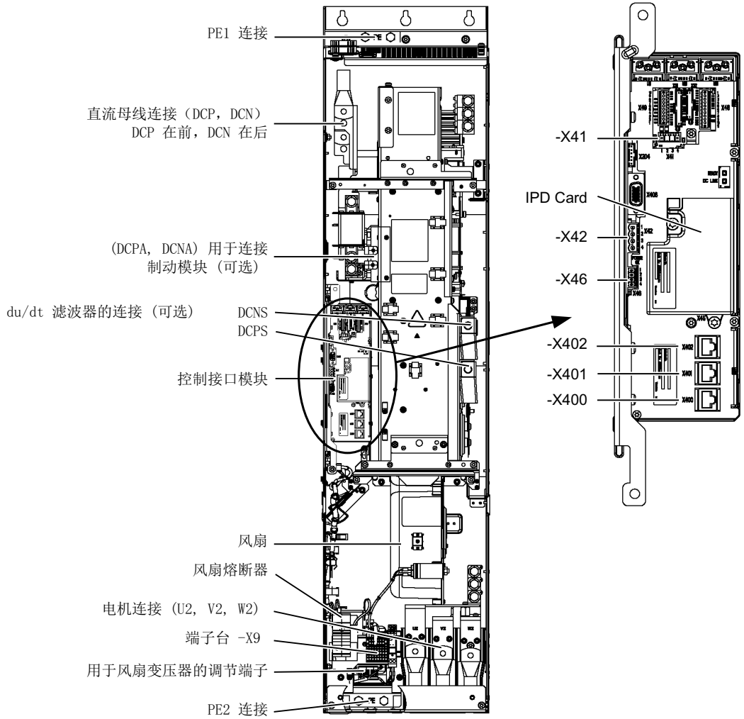
图 4-1 电机模块, FX 型
