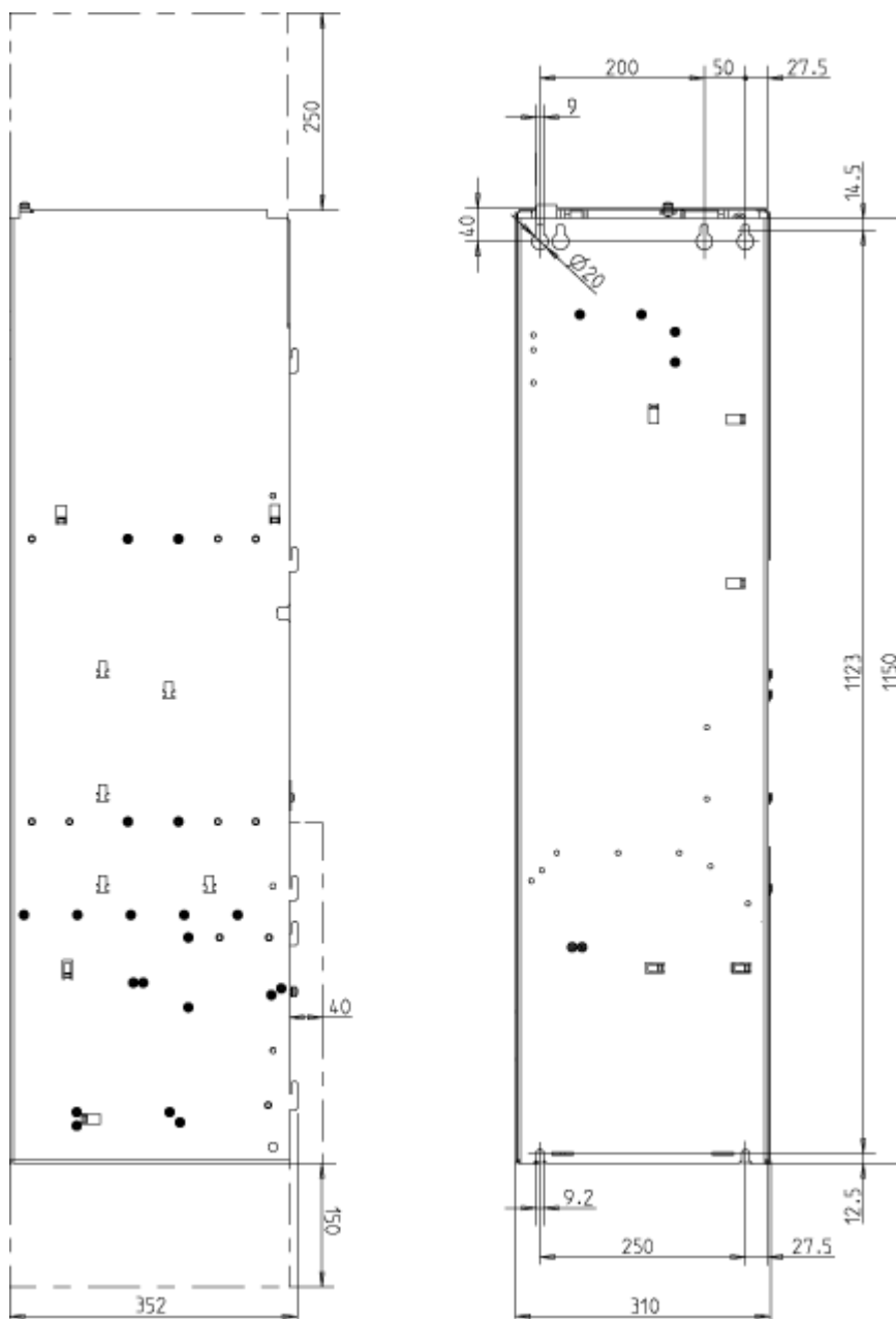
图 3-5 FB 型基本型电源模块，侧视图和背视图
