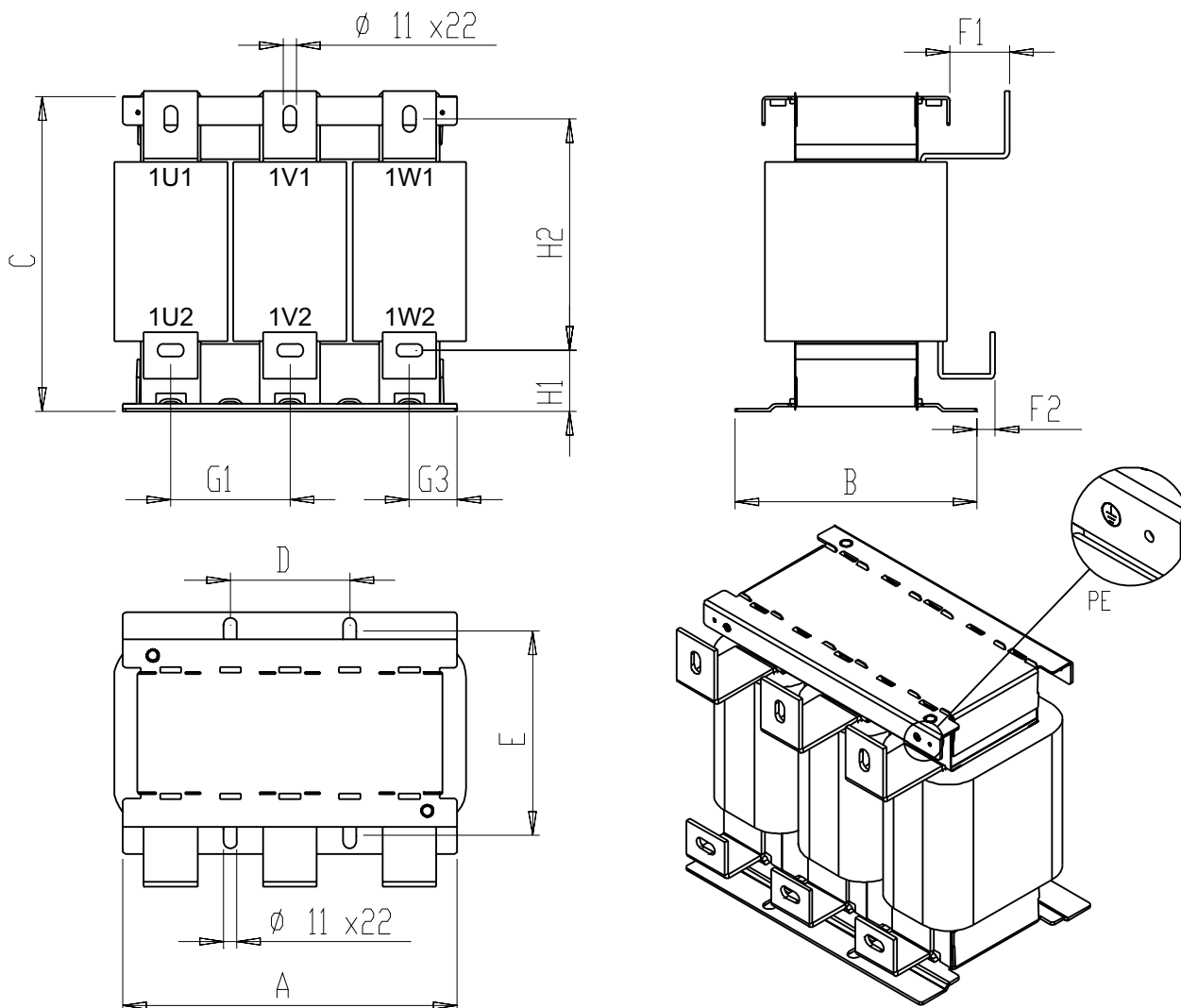
图 2-4 电源电抗器 6SL3000-0EE36-2AA0 的外形尺寸图
