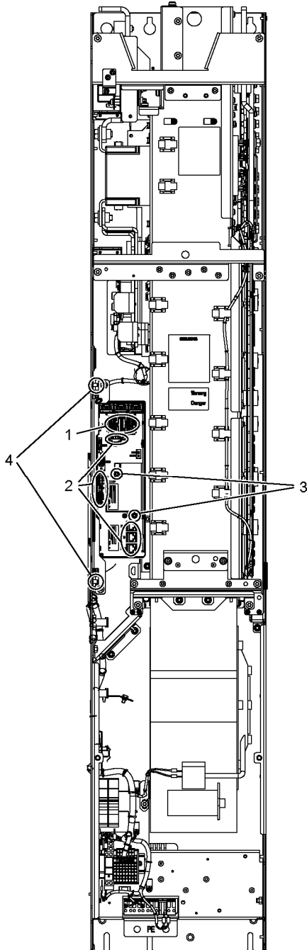
图 8-17 更换 GB、GD 型基本型电源模块的控制接口模块
