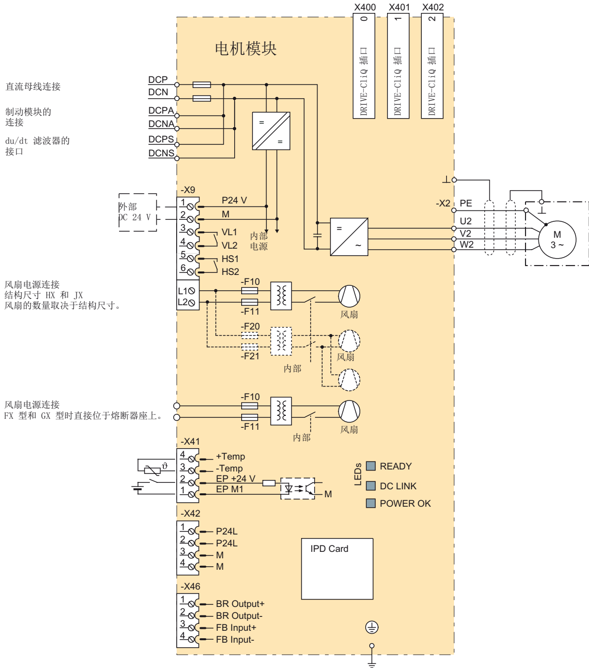
图 4-5 电机模块接线示例
