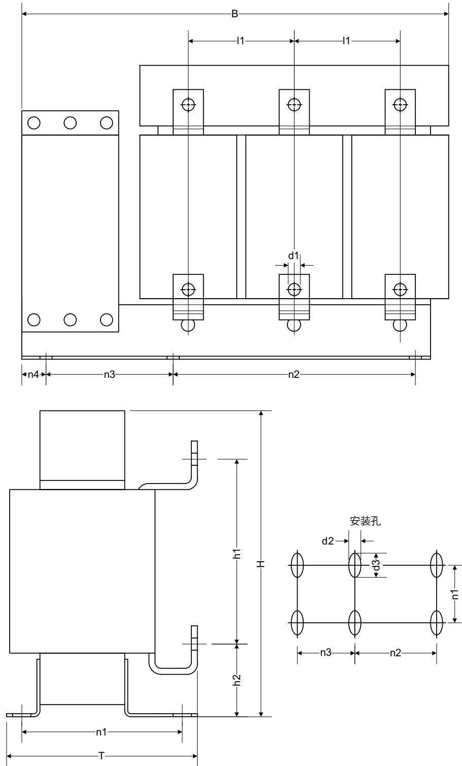
图 6-2 正弦滤波器的外形尺寸图
