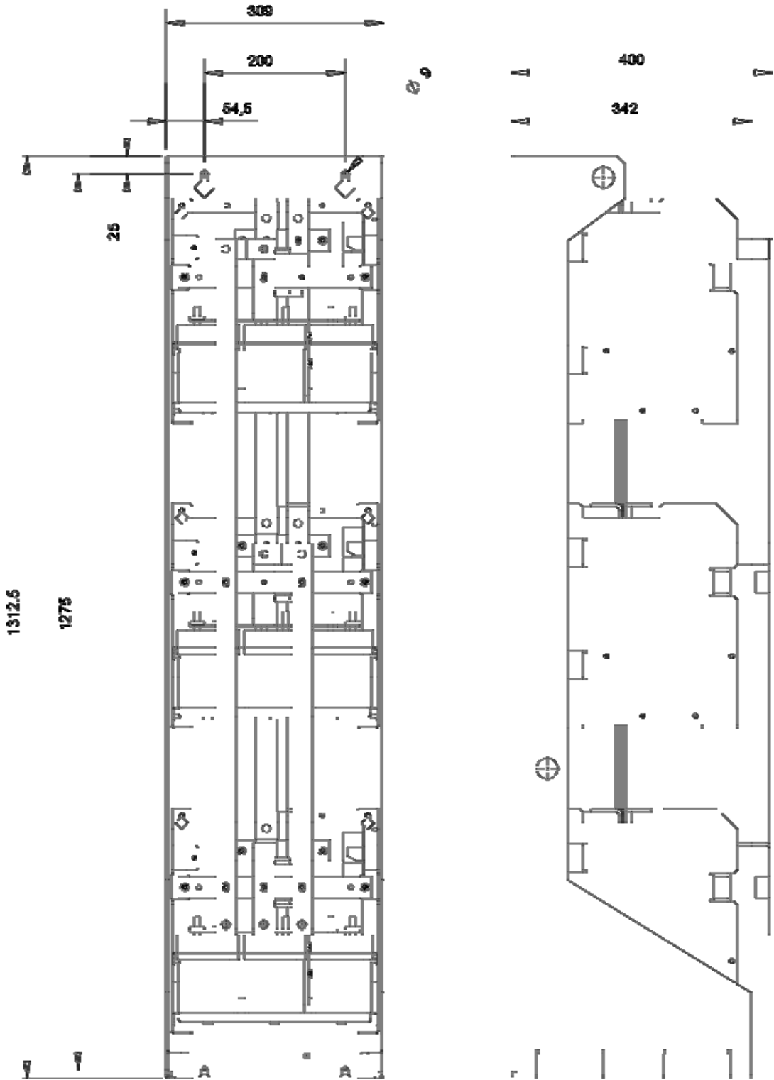
图 6-12 3 类电压峰值限制器的外形尺寸图
