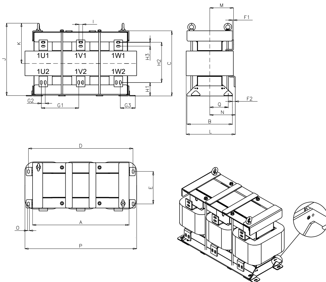
图 2-9 电源电抗器 6SL3000-0EH41-4AA0 的外形尺寸图
