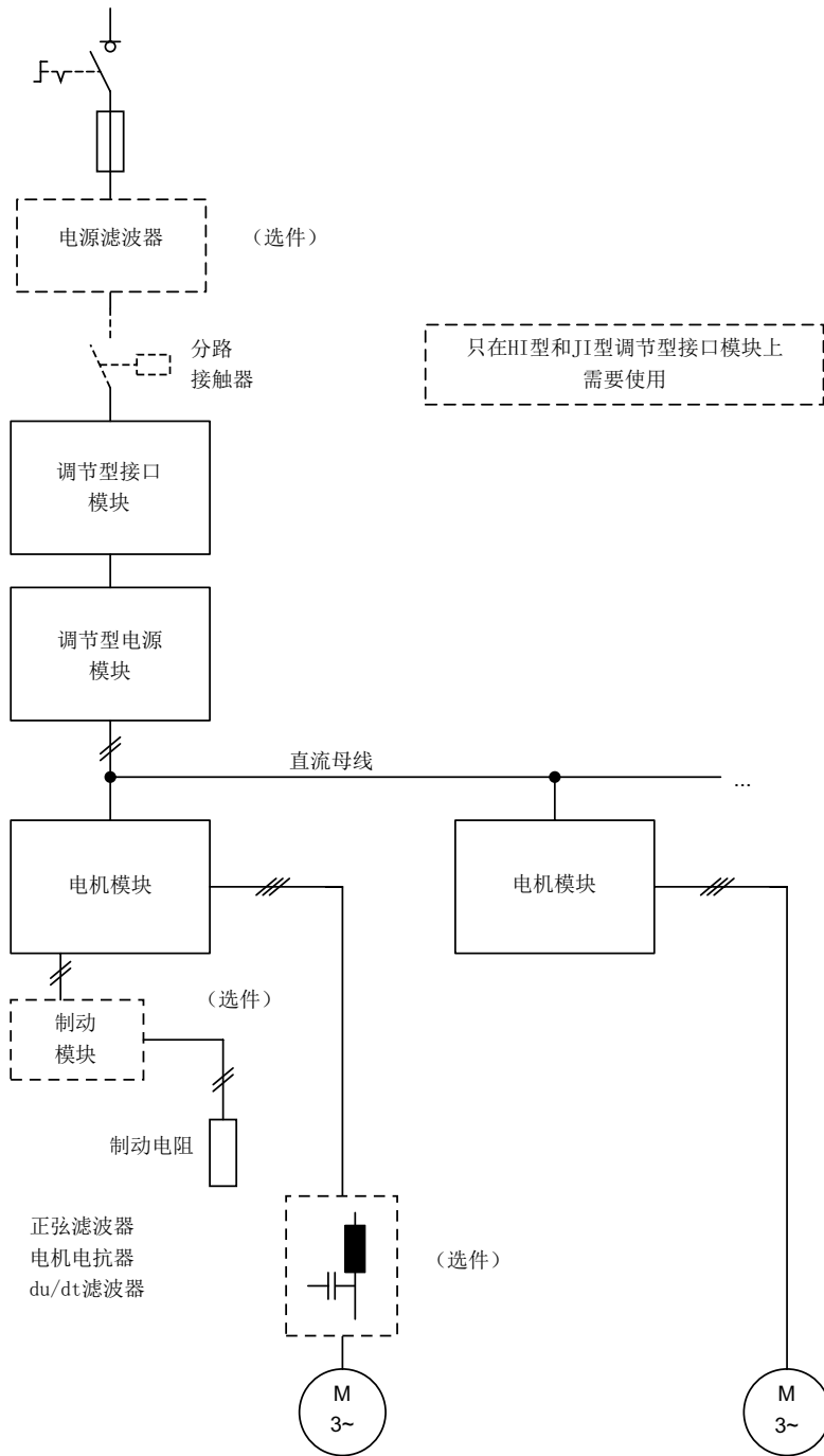
图 1-4 SINAMICS S120 和受控型电源模块组成的驱动系统的基本结构
