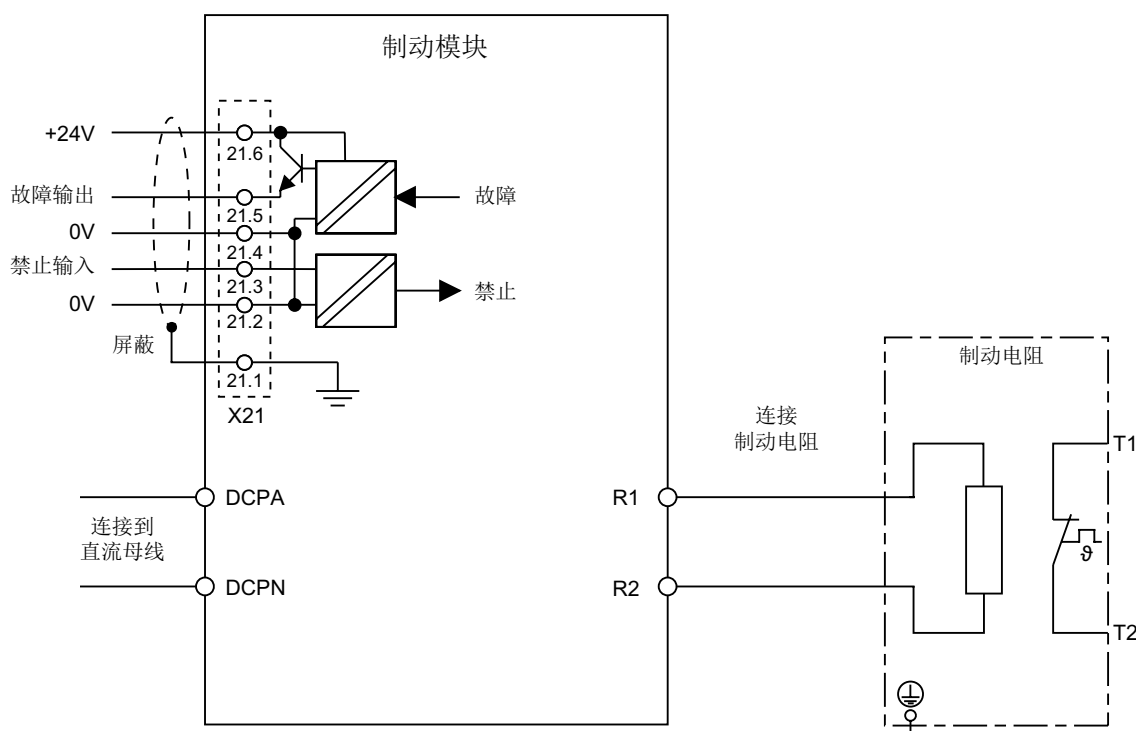
图 5-5 制动模块连接示例
