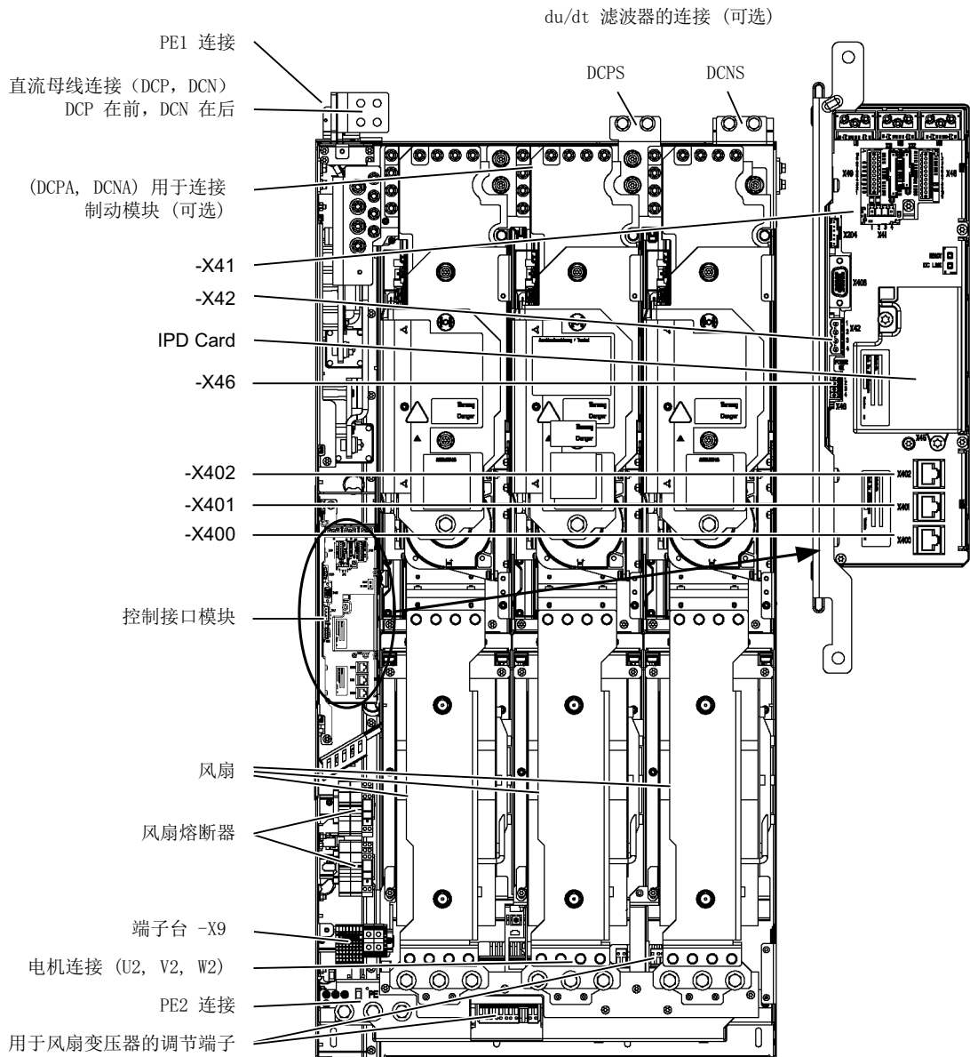
图 4-4 电机模块, JX 型
