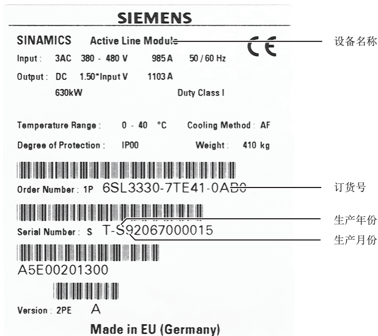
图 8-29 比如调节型电源模块的铭牌
