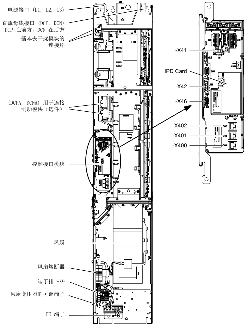
图 3-2 GB、GD 型基本型电源模块
