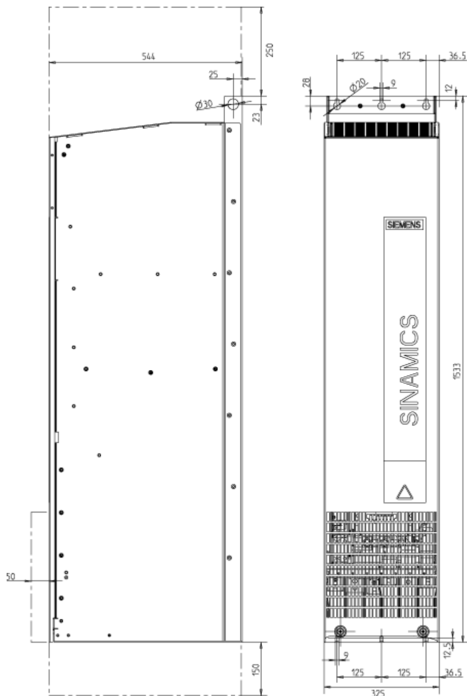
图 2-18 GI 型调节型接口模块的外形尺寸图。侧视图和正视图
