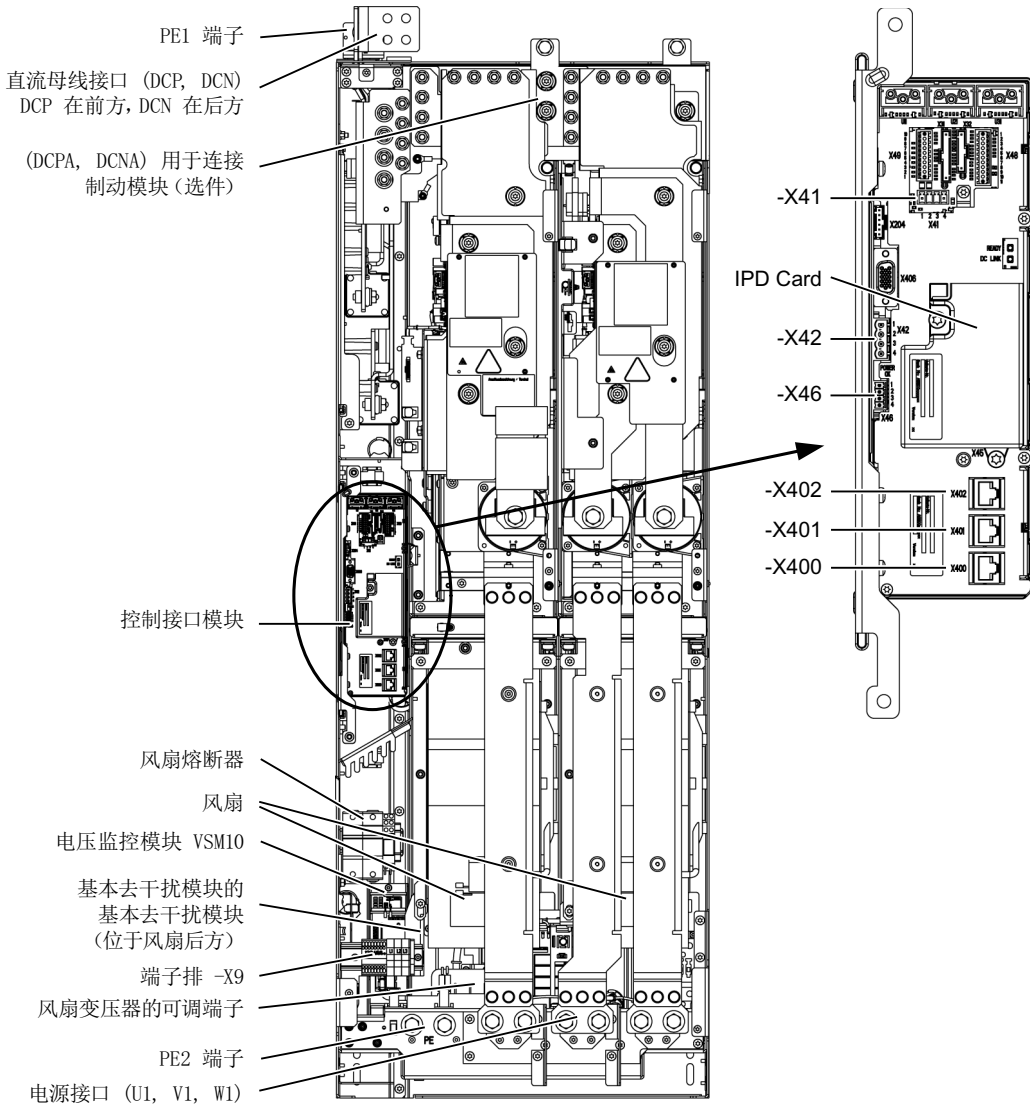
图 3-15 HX 型非调节型电源模块
