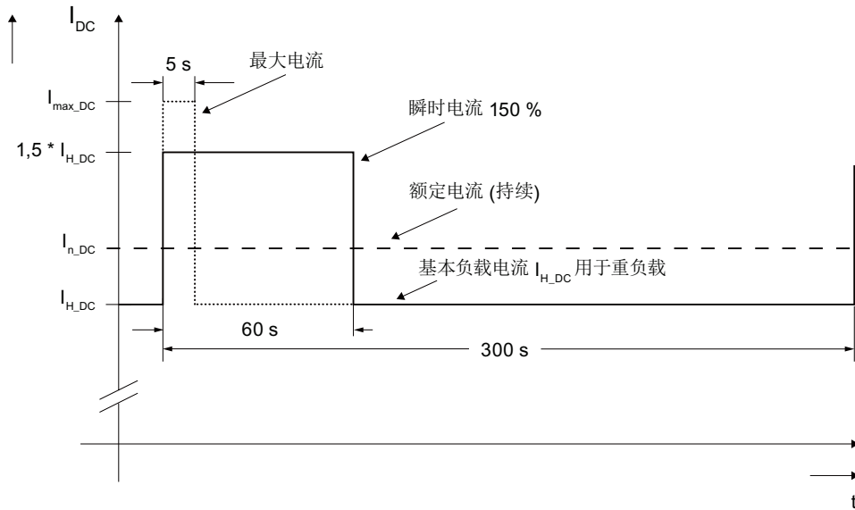
图 3-26 重过载
