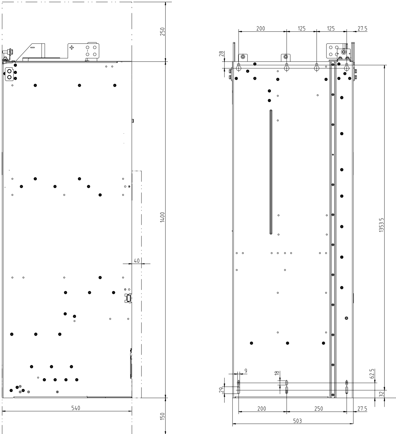
图 3-36 HX 型调节型电源模块的外形尺寸图 侧视图和背视图
