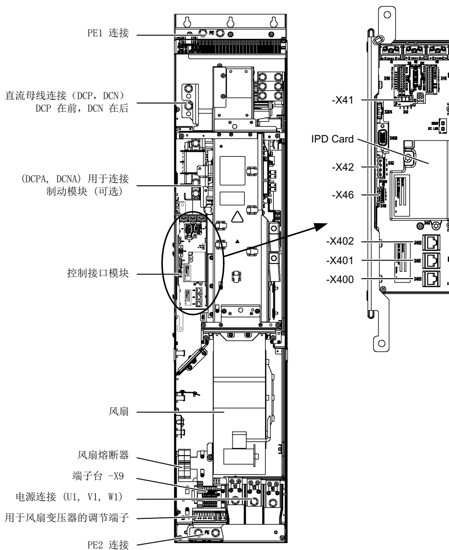
图 3-30 GX 型调节型电源模块
