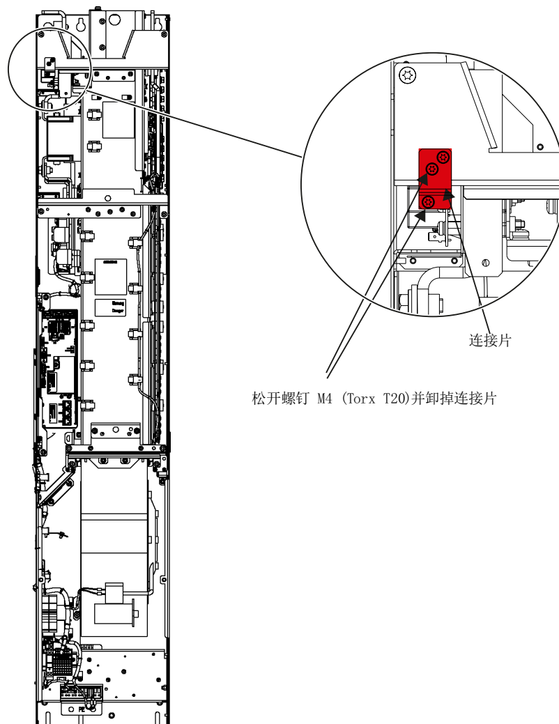
图 3-9 取出 GB、GD 型调节型接口模块中的基本去干扰模块的连接片
