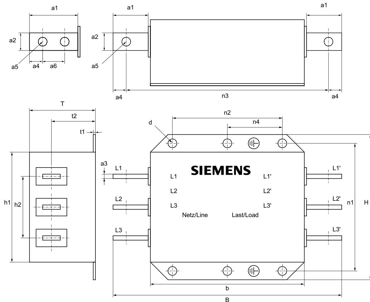
图 2-2 和调节型电源模块 ALM 和非调节电源模块 SLM 配套的电源滤波器的外形尺寸图
