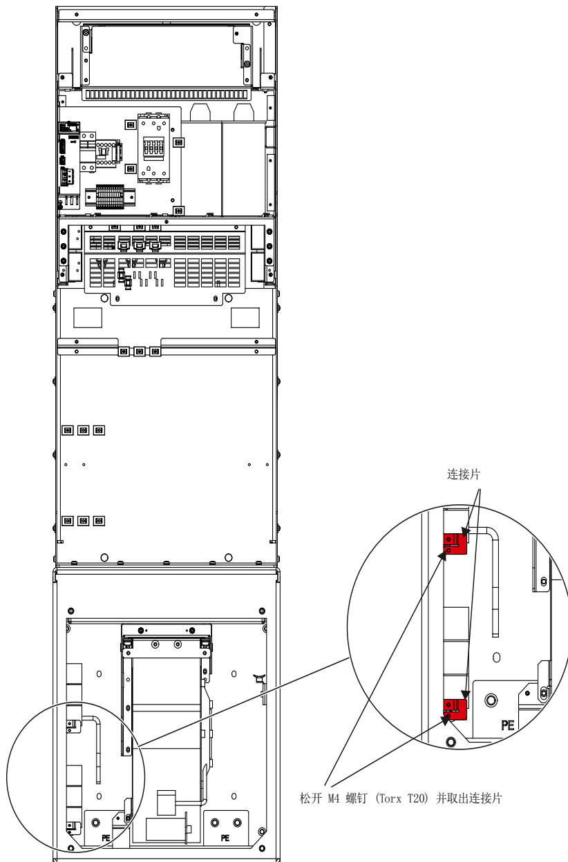
图 2-25 取出 J1 型调节型接口模块中的基本去干扰模块的连接片
