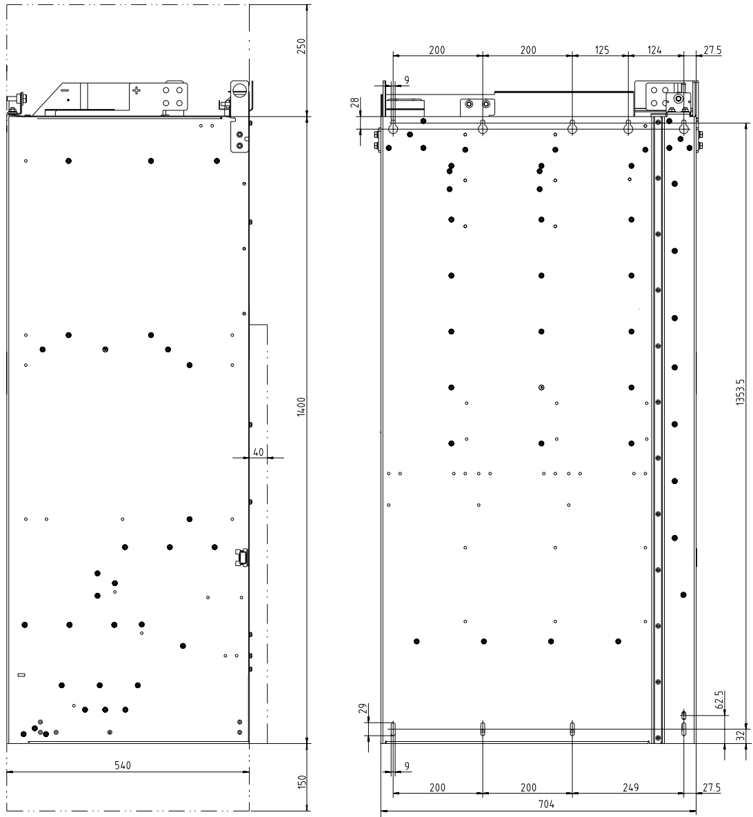
图 4-9 JX 型电机模块的外形尺寸图 侧视图和背视图
