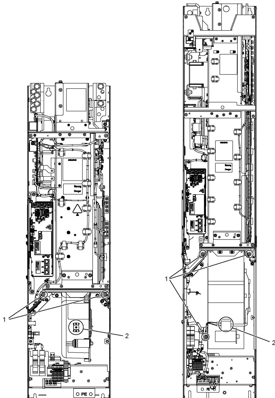
图 8-26 更换 FB、GB、GD 型 BLM 的风扇
