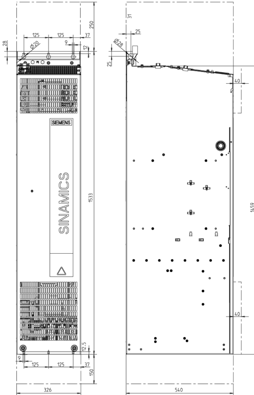
图 4-7 GX 型电机模块的外形尺寸图 正视图和侧视图
