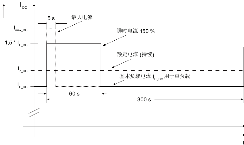
图 3-39 重过载
