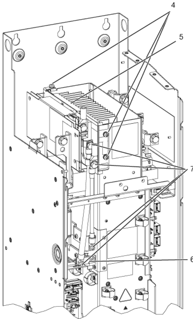
图 5-7 将制动模块安装到 FX 型调节型电源模块/电机模块中 - 步骤 4 - 7
