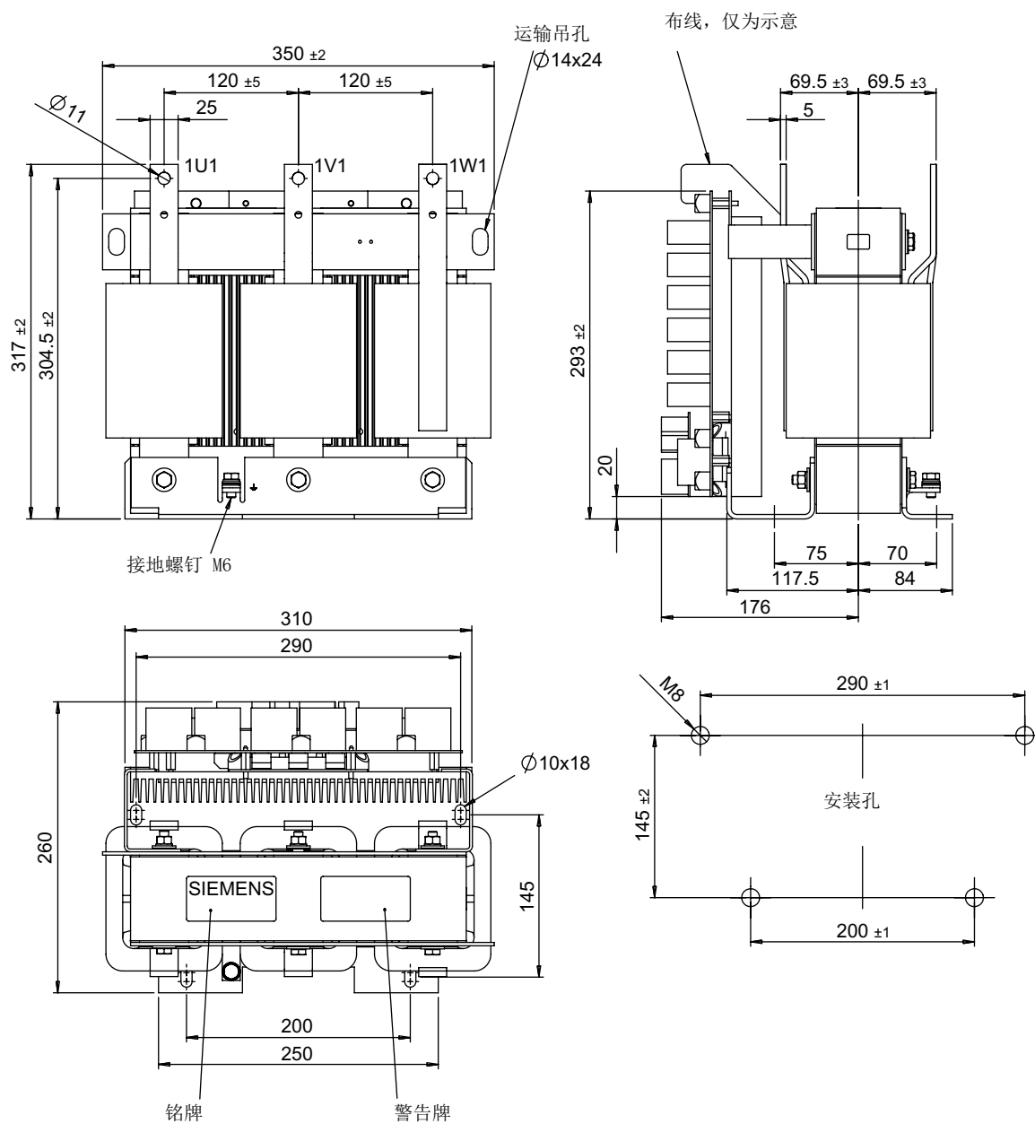
图 6-21 带电压峰值限制器的紧凑型 du/dt 滤波器的尺寸图，类型 2
