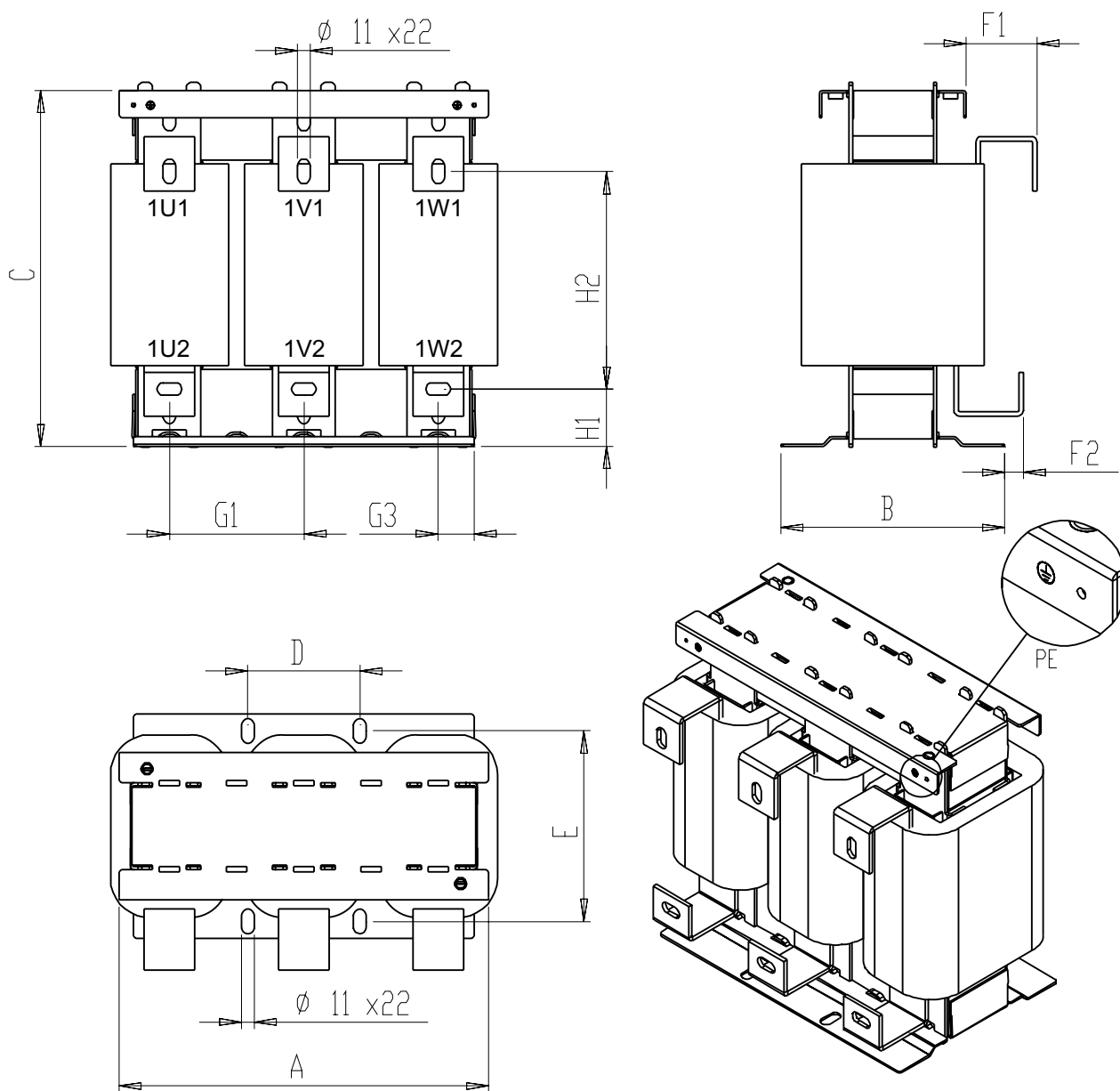
图 2-7 电源电抗器 6SL3000-0EH34-7AA0 的外形尺寸图
