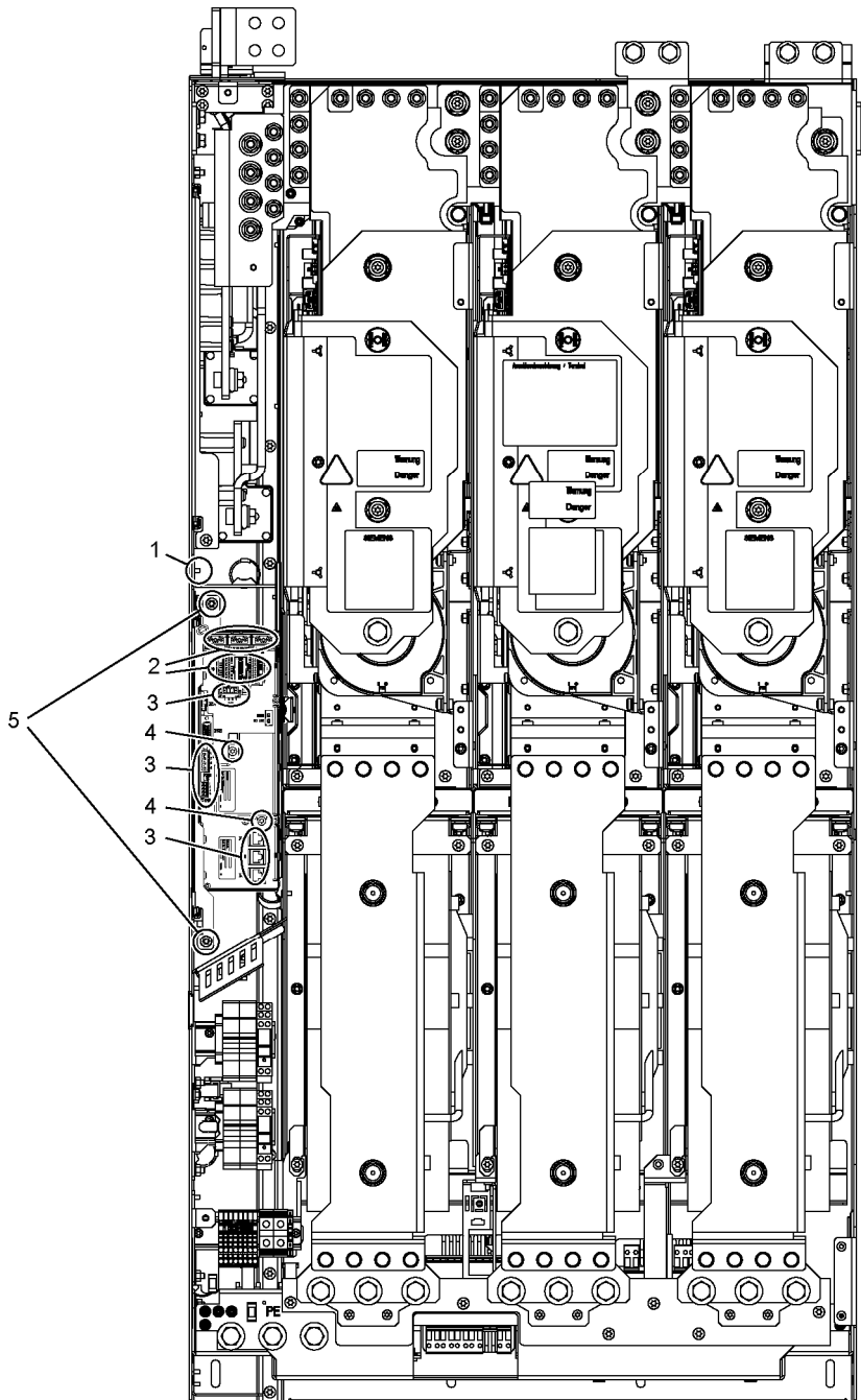
图 8-15 更换 JX 型非调节型/调节型电源模块和电机模块的控制接口模块
