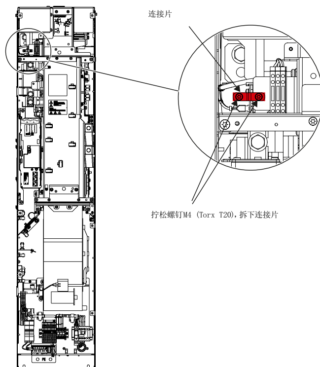
图 3-22 取出 GX 型非调节型电源模块中的基本去干扰模块的连接片
