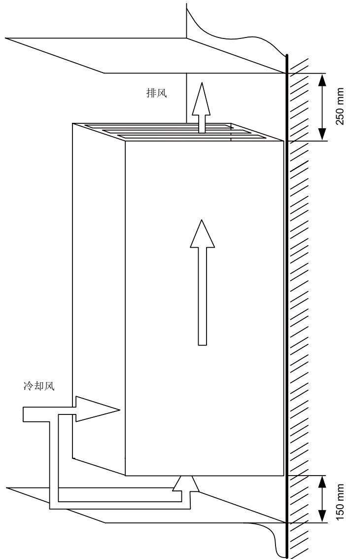
图 7-4 HX, JX 型非调节型/调节型电源模块和电机模块的通风
