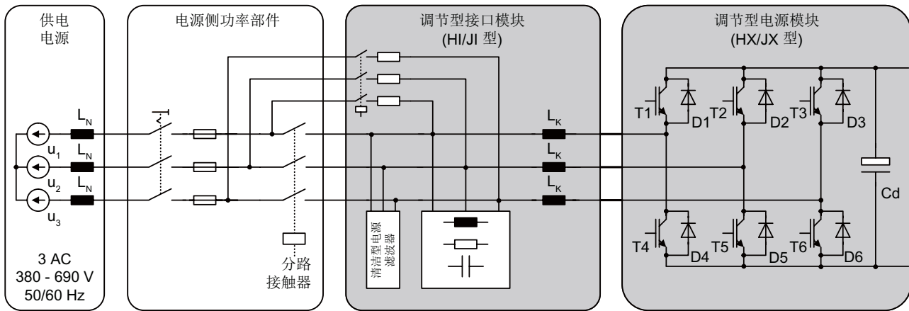
图 3-28 调节型电源 HI/HX 和 JI/JX 型的概览
