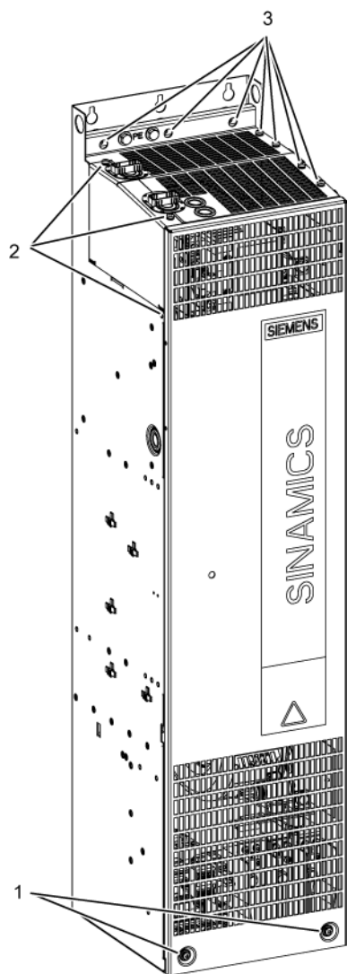
图 5-6 将制动模块安装到 FX 型调节型电源模块/电机模块中 - 步骤 1-3
