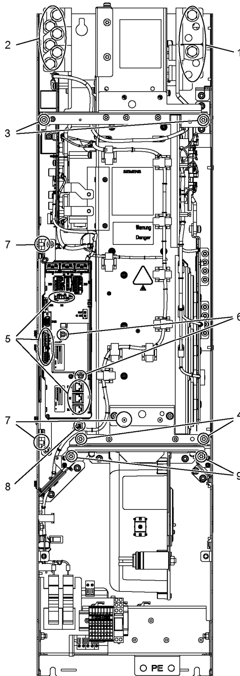
图 8-10 更换 FB 型基本型电源模块的功率单元
