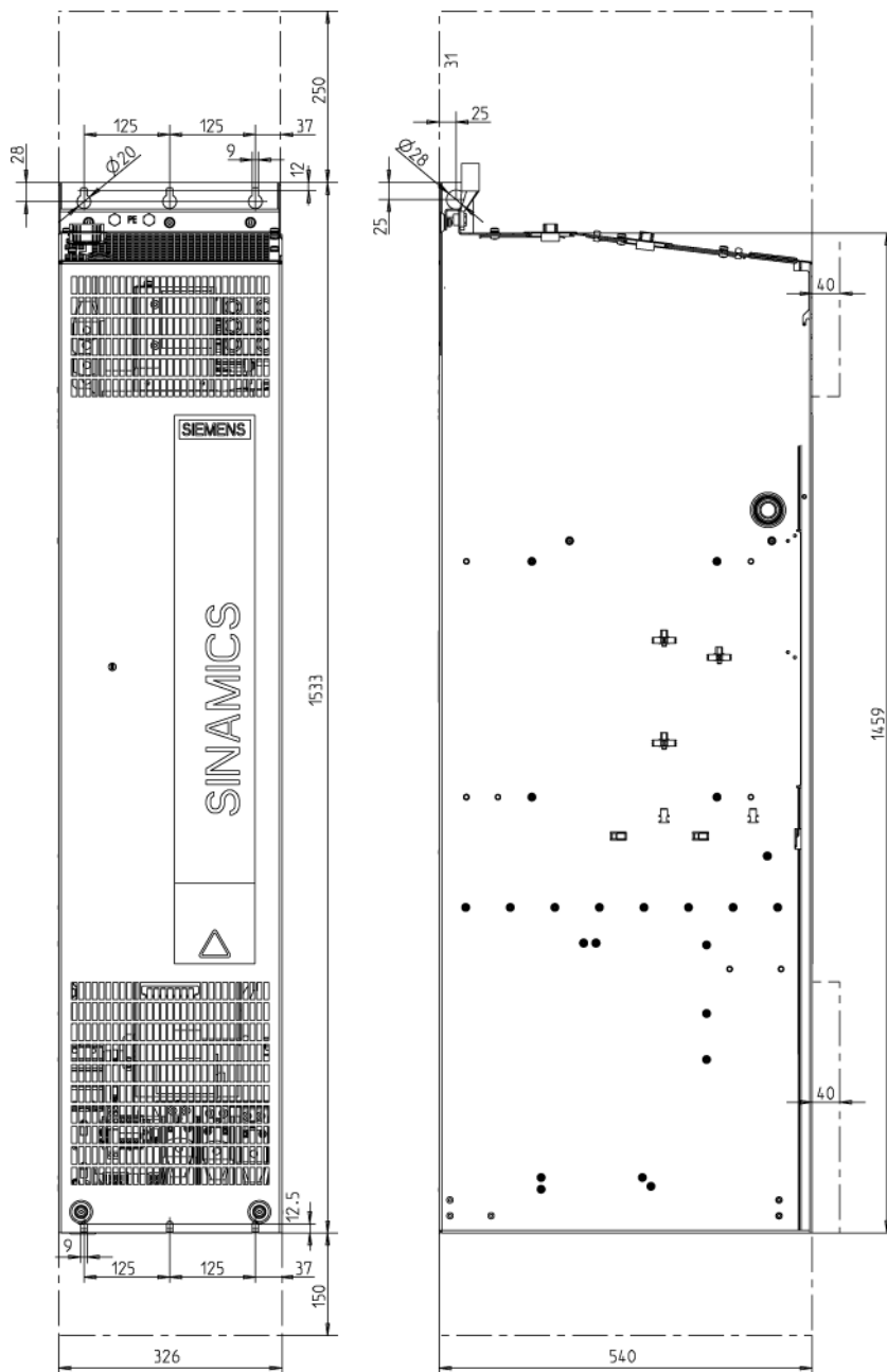
图 3-35 GX 型调节型电源模块的外形尺寸图 正视图和侧视图
