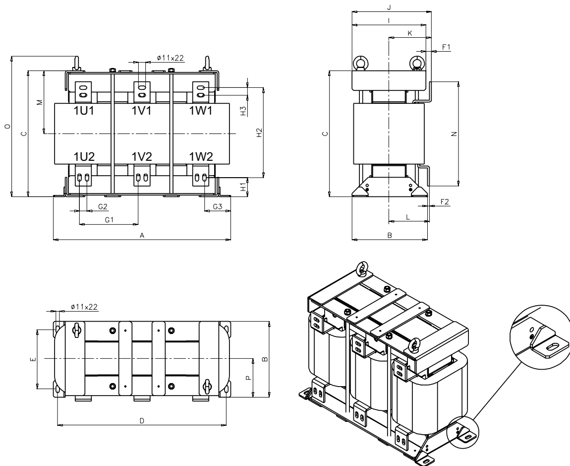
图 2-6 电源电抗器 6SL3000-0EE41-4AA0 的外形尺寸图
