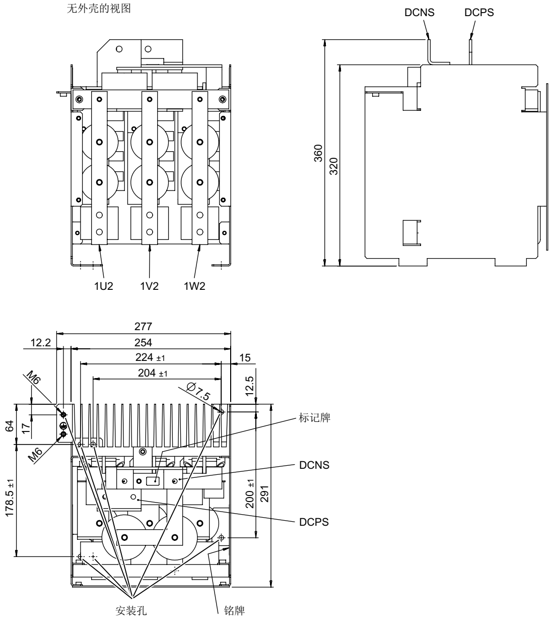
图 6-24 带电压峰值限制器的紧凑型 du/dt 滤波器的尺寸图，类型 4：电压峰值限制器
