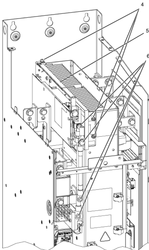
图 5-9 将制动模块安装到 GX 型非调节型/调节型电源模块/电机模块中 - 步骤 4-6
