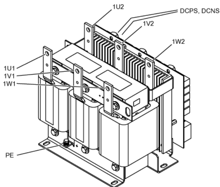
图 6-13 带有电压峰值限制器的紧凑型 du/dt 滤波器的接口一览，类型 1
