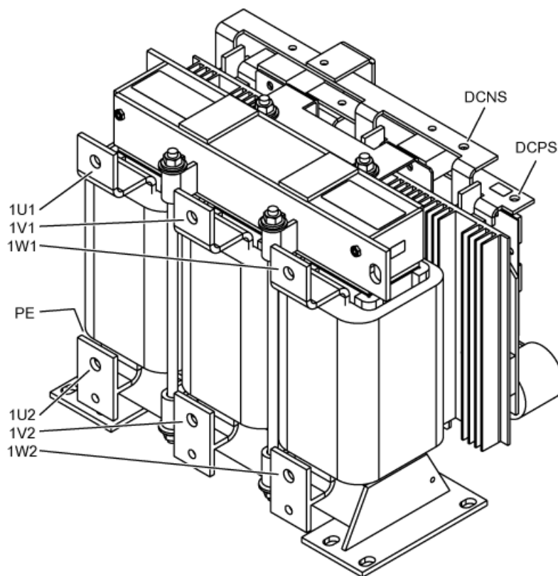
图 6-15 带有电压峰值限制器的紧凑型 du/dt 滤波器的接口一览，类型 3
