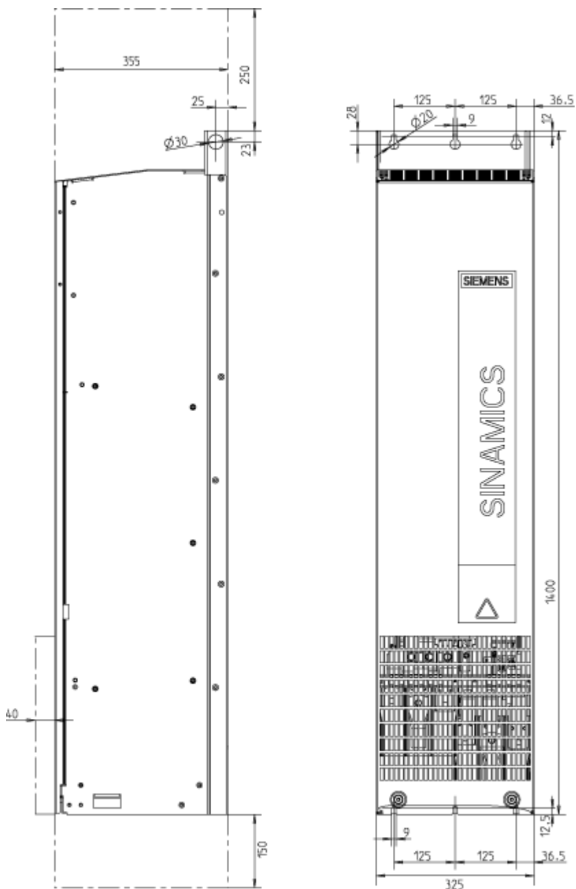
图 2-17 FI 型调节型接口模块的外形尺寸图。侧视图和正视图
