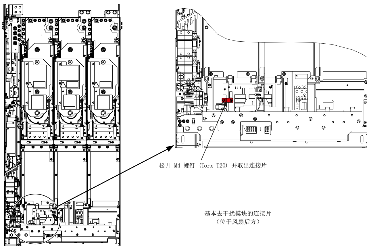
图 3-24 取出 JX 型非调节型电源模块中的基本去干扰模块的连接片
