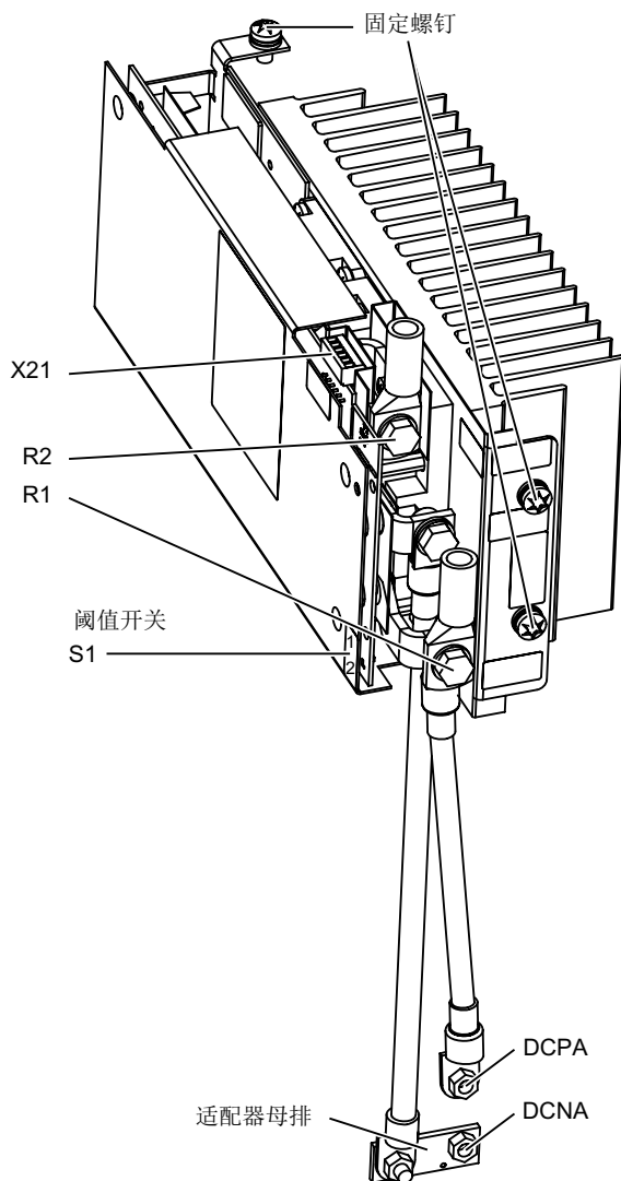
图 5-2 制动模块，用于 FX 型调节型电源模块/电机模块和 FB 型基本型电源模块
