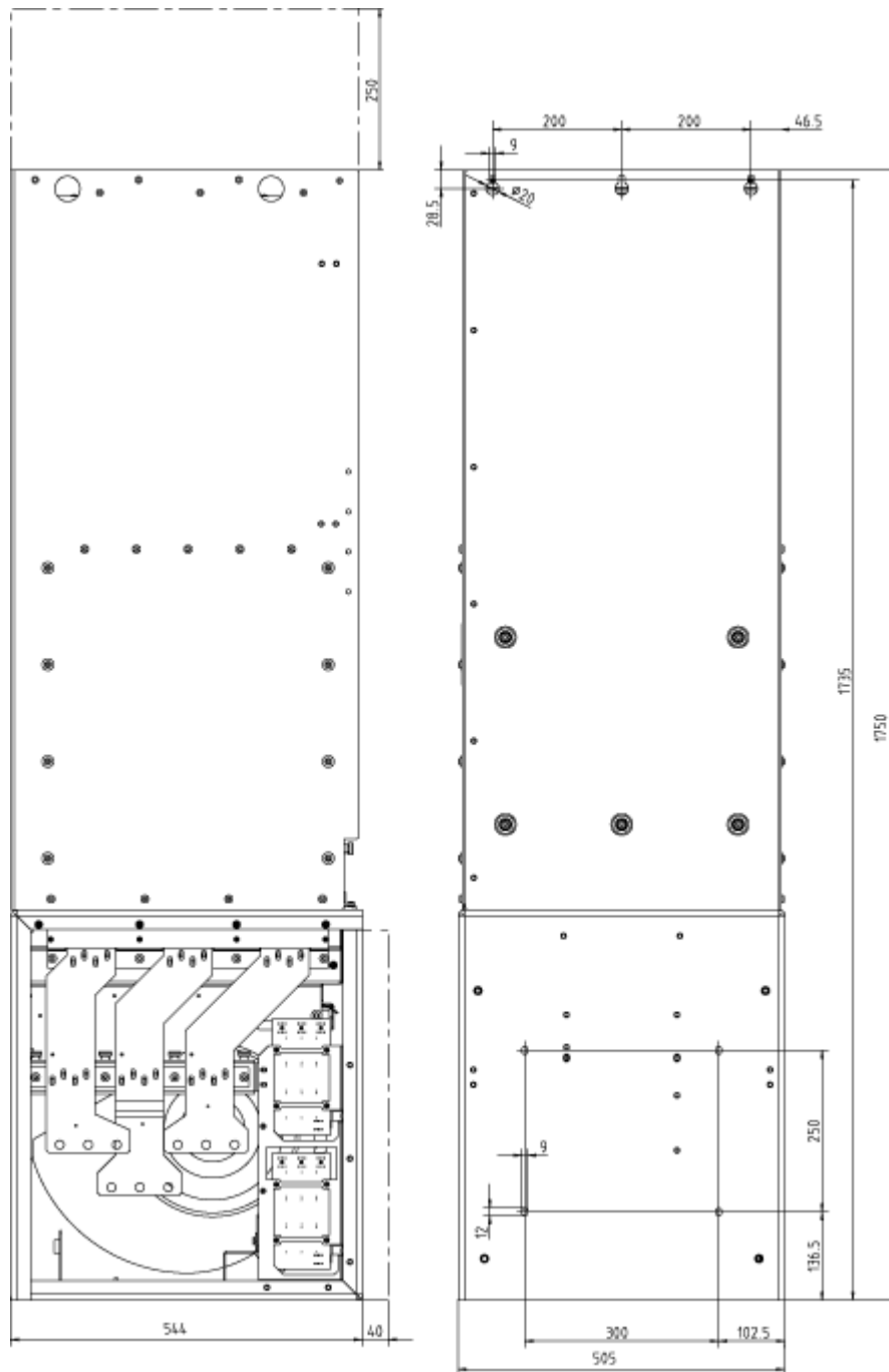
图 2-20 J1 型调节型接口模块的外形尺寸图。侧视图和背视图
