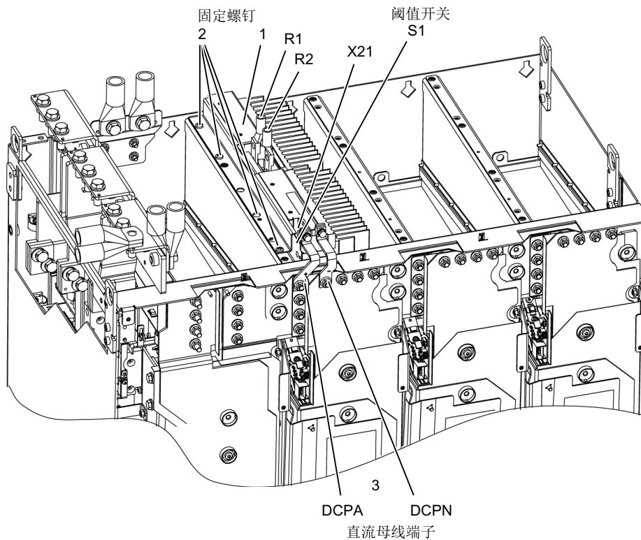
图 5-11 将制动模块安装到 JX 型非调节型/调节型电源模块/电机模块中
