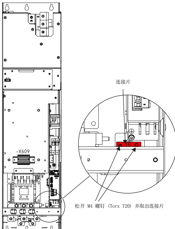
图 2-22 取出 FI 型调节型接口模块中的基本去干扰模块的连接片
