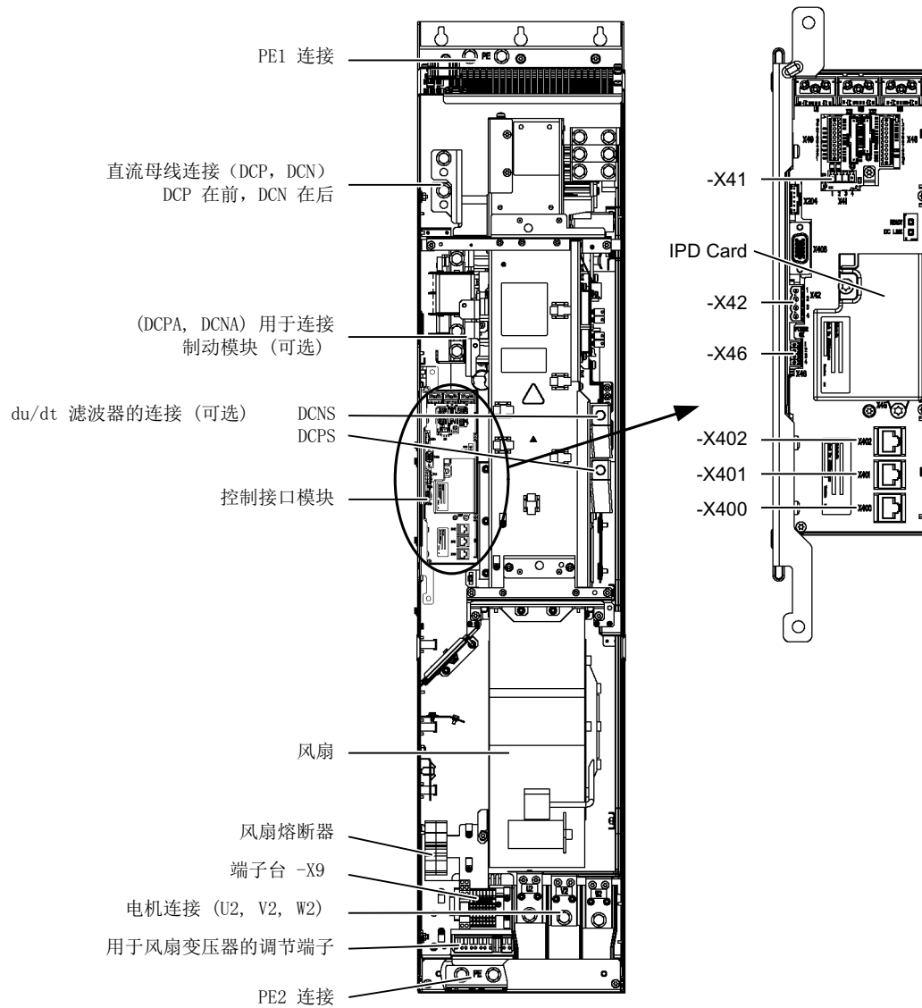
图 4-2 电机模块, GX 型
