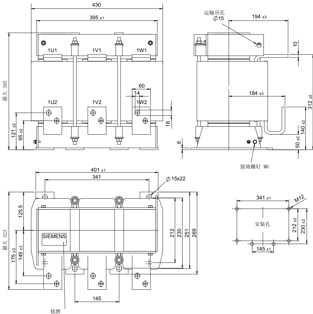
图 6-23 带电压峰值限制器的紧凑型 du/dt 滤波器的尺寸图，类型 4： du/dt 电抗器
