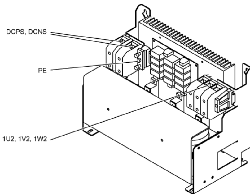
图 6-5 2 类电压峰值限制器的接口概览
