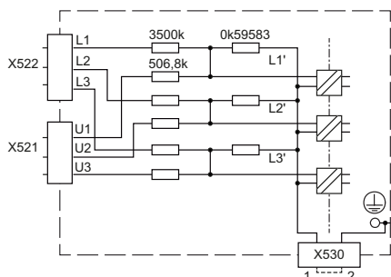
图 2-16 内电路电压监控模块 VSM10
