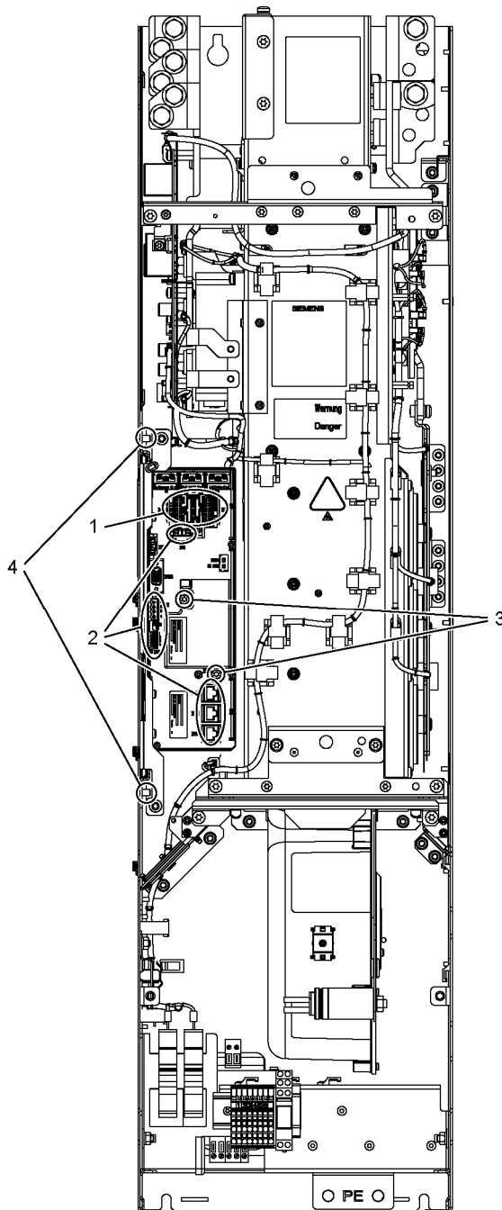
图 8-16 更换 FB 型基本型电源模块的控制接口模块
