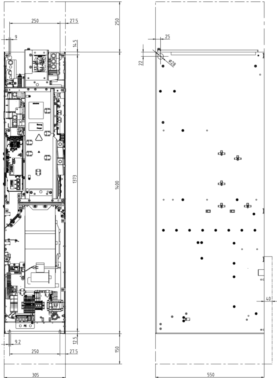
图 3-18 GX 型非调节型电源模块的外形尺寸图 正视图和侧视图
