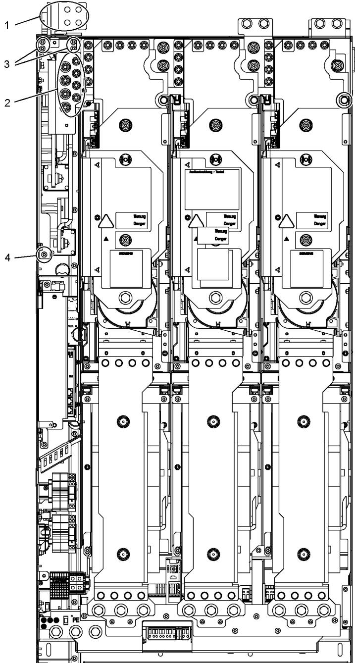
图 8-28 更换 JX 型非调节型/调节型电源模块和电机模块的直流熔断器
