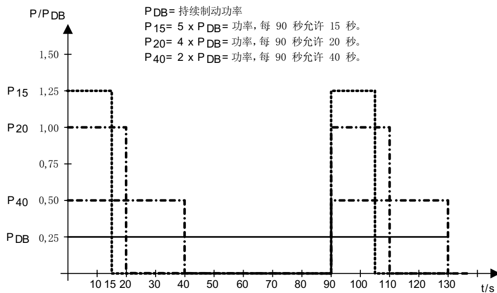
图 5-16 用于制动电阻的负载循环
