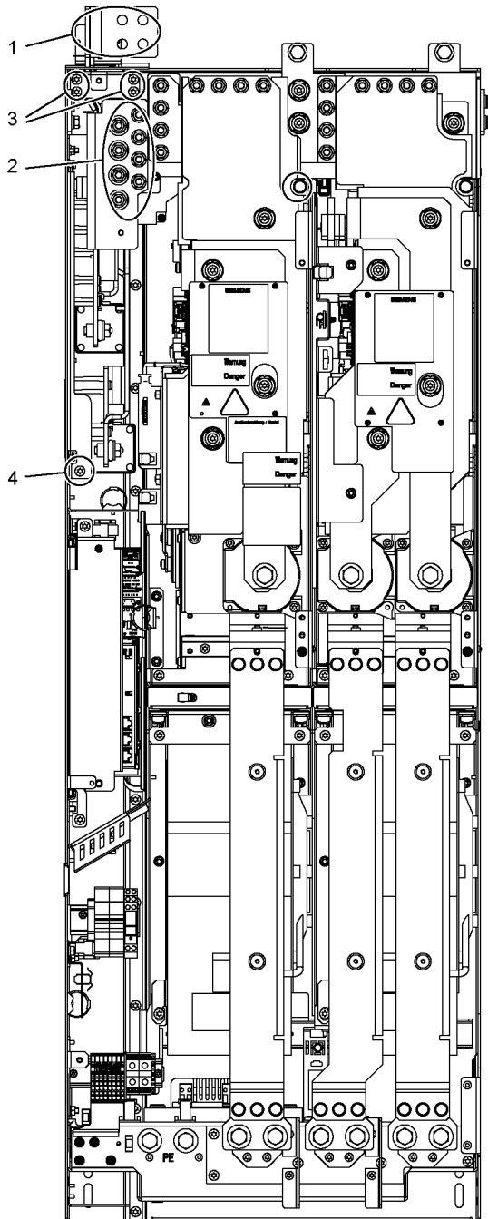
图 8-27 更换 HX 型非调节型/调节型电源模块和电机模块的直流熔断器
