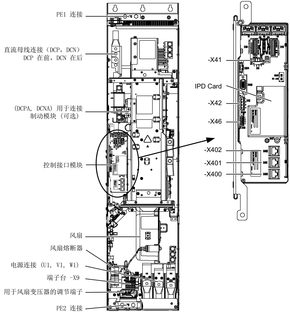
图 3-29 FX 型调节型电源模块
