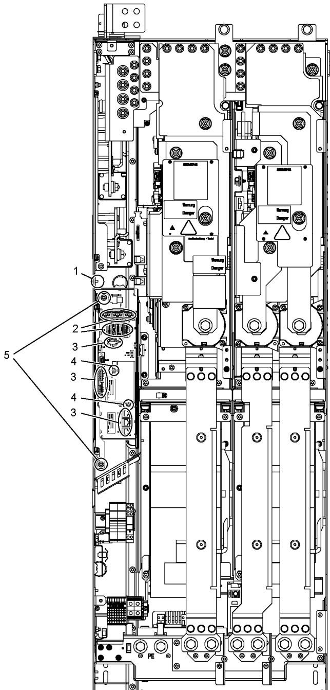
图 8-14 更换 HX 型非调节型/调节型电源模块和电机模块的控制接口模块
