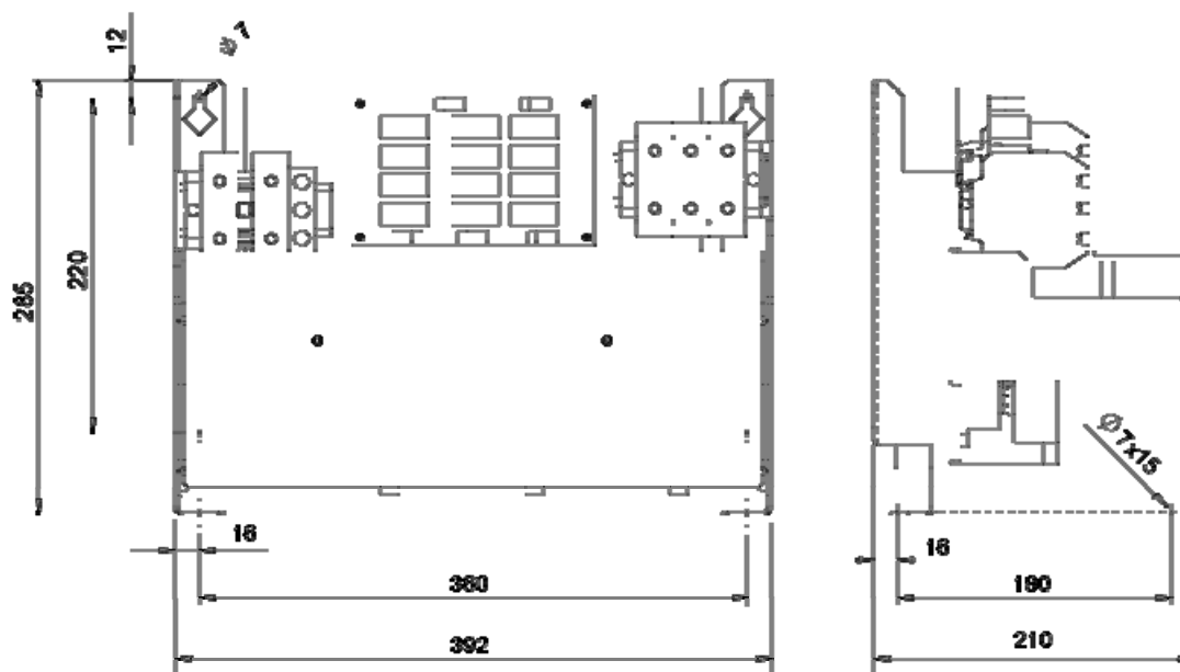
图 6-11 2 类电压峰值限制器的外形尺寸图
