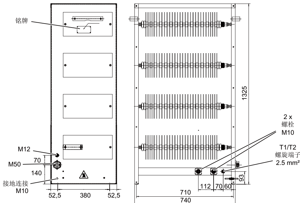
图 5-15 制动电阻 50 kW / 250 kW 的外形尺寸图
