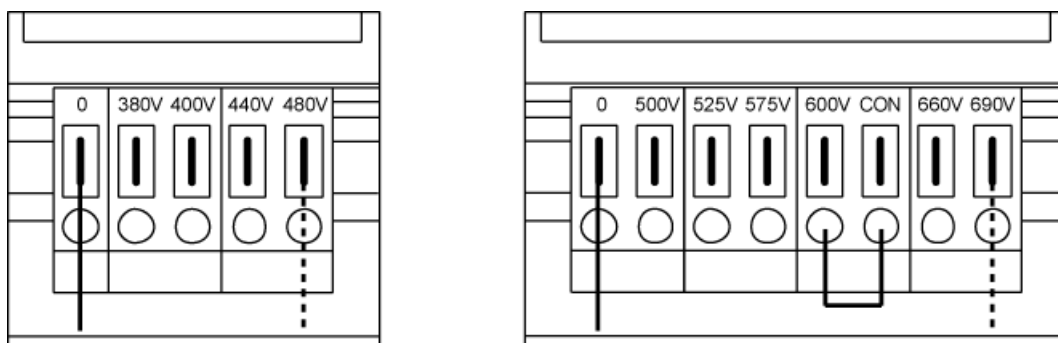
图 3-10 风扇变压器的可调端子(3 AC 380 到 480 V / 3 AC 500 到 690 V)
