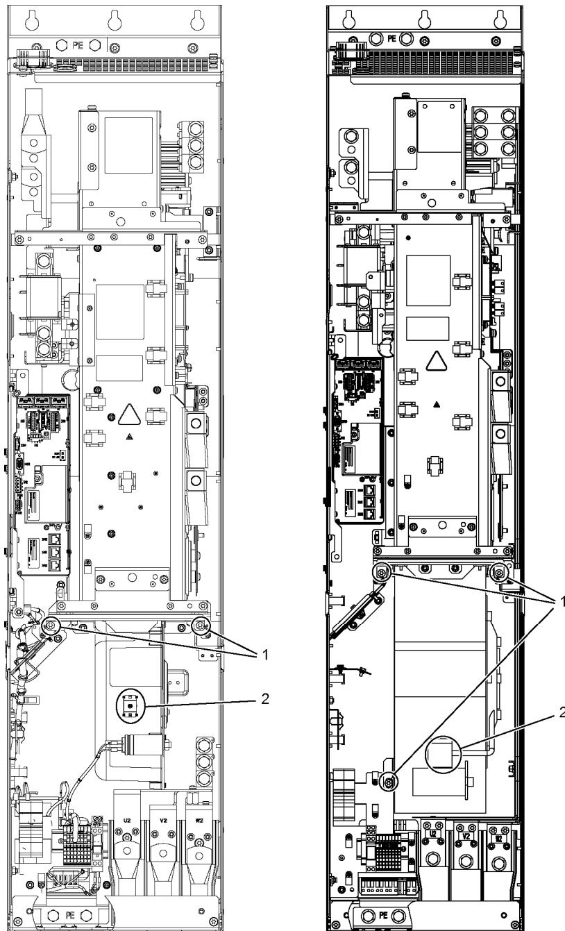
图 8-18 更换 FX, GX 型非调节型/调节型电源模块和电机模块的风扇
