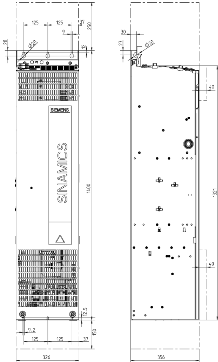
图 4-6 FX 型电机模块的外形尺寸图 正视图和侧视图
