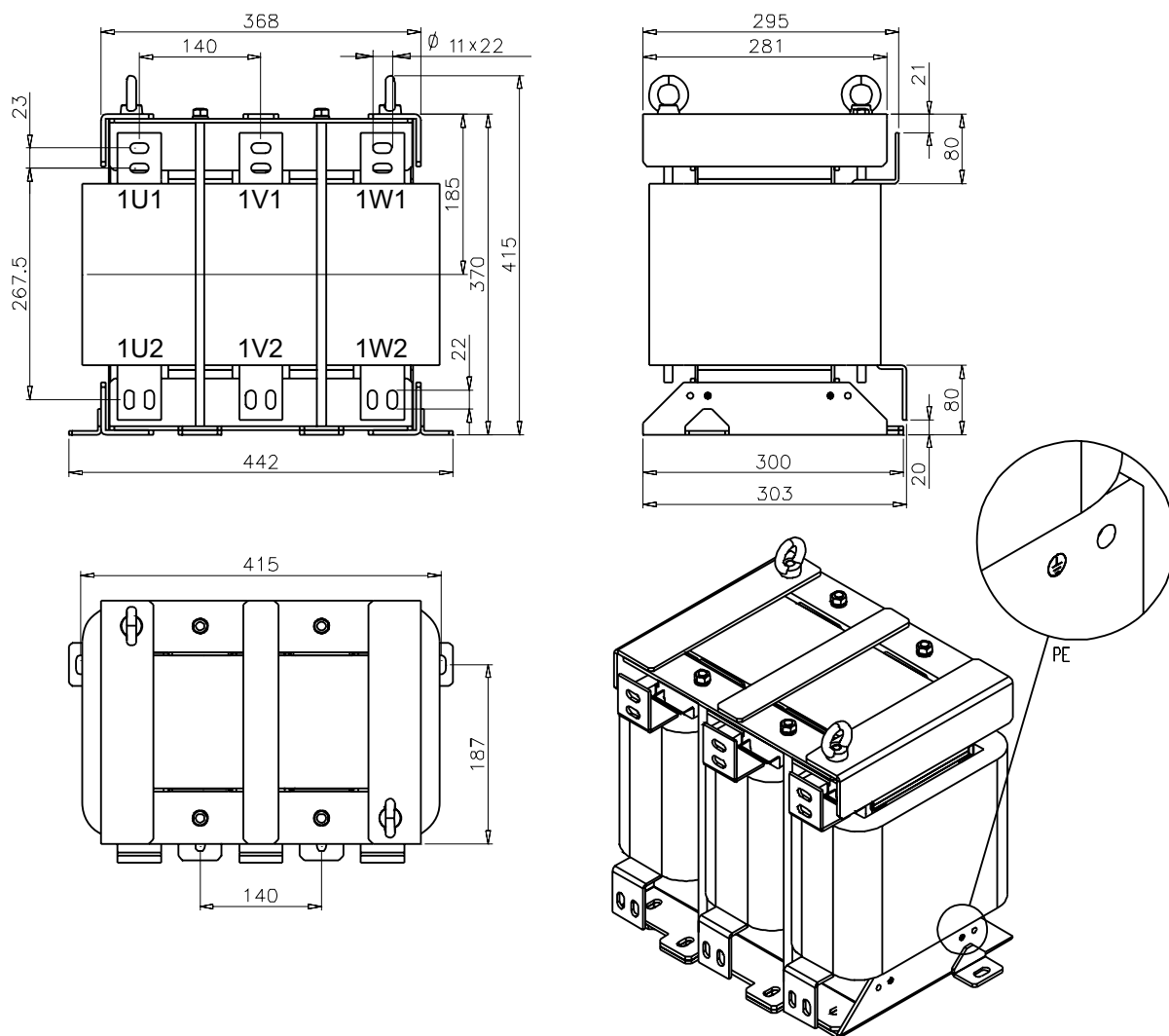
图 2-8 电源电抗器 6SL3000-0EH37-6AA0 的外形尺寸图，所有尺寸以 mm 为单位
