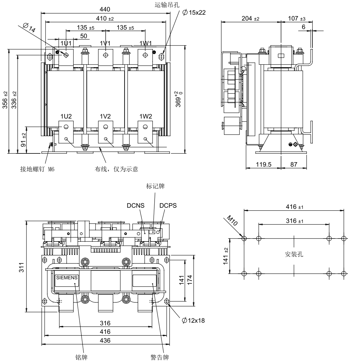
图 6-22 带电压峰值限制器的紧凑型 du/dt 滤波器的尺寸图，类型 3
