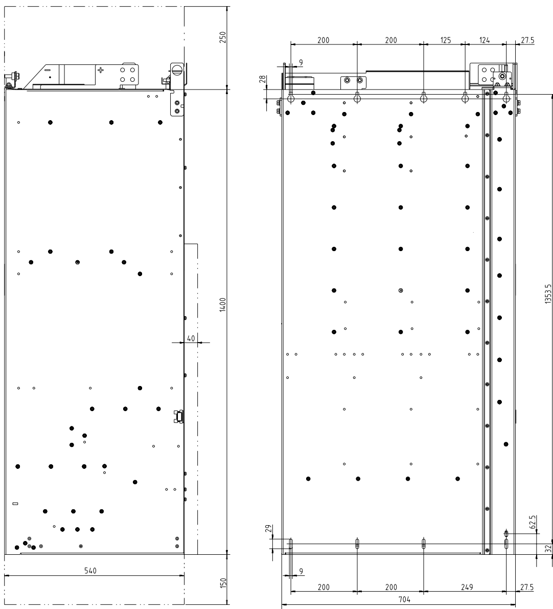
图 3-37 JX 型调节型电源模块的外形尺寸图 侧视图和背视图
