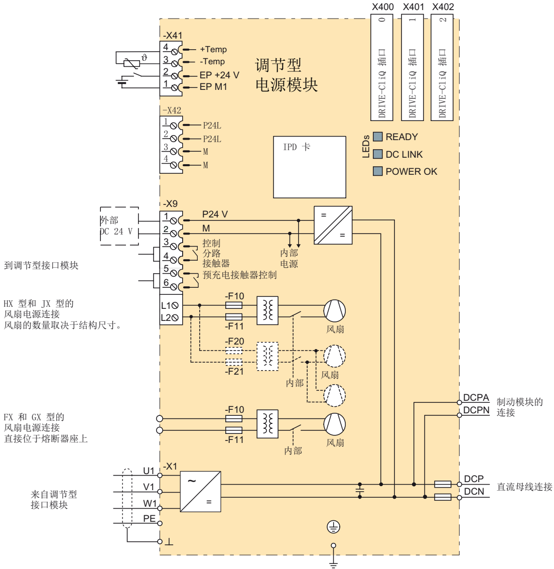
图 3-33 调节型电源模块的连接图
