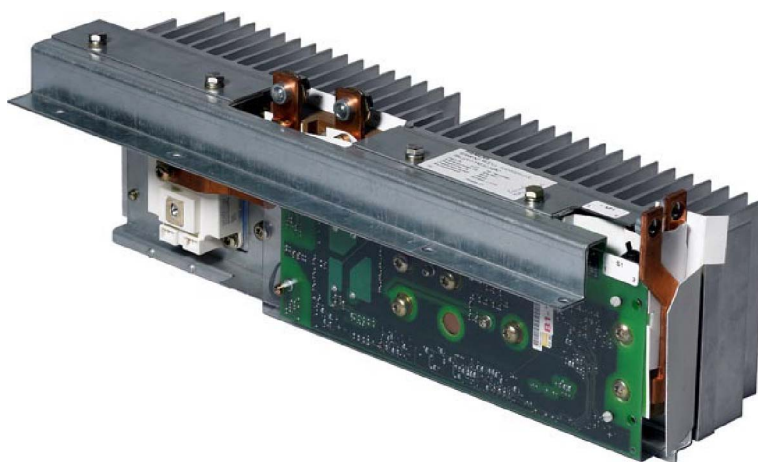
图 5-1 制动模块
