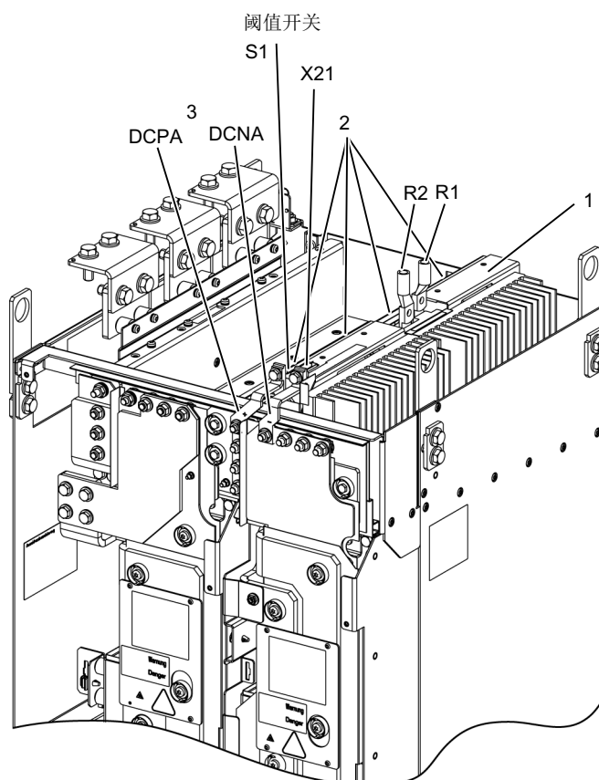
图 5-10 将制动模块安装到 HX 型非调节型/调节型电源模块/电机模块中
