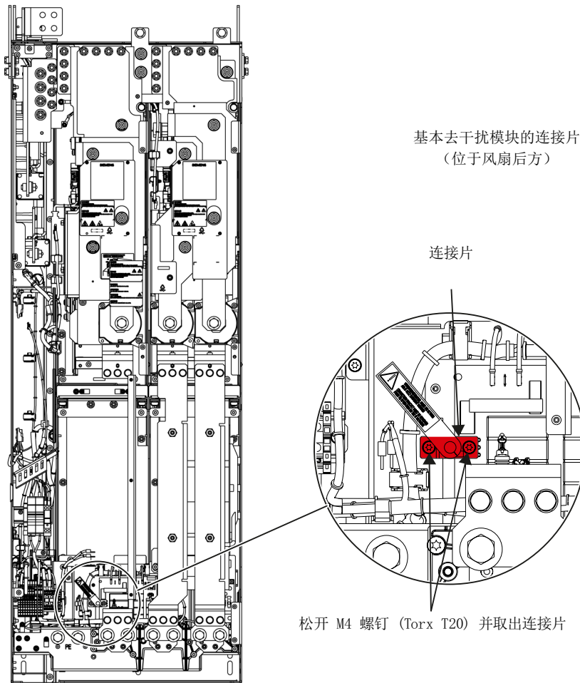
图 3-23 取出 HX 型非调节型电源模块中的基本去干扰模块的连接片
