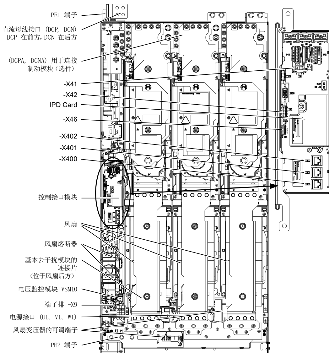
图 3-16 JX 型非调节型电源模块
