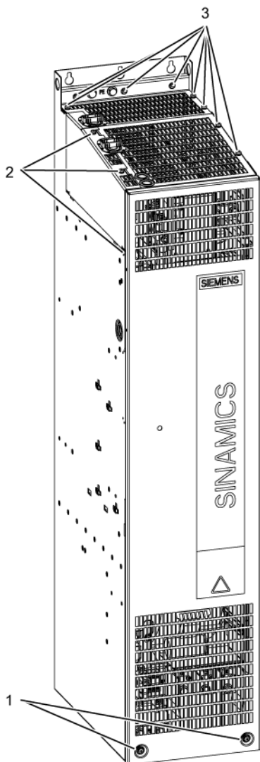
图 5-8 将制动模块安装到 GX 型非调节型/调节型电源模块/电机模块中 - 步骤 1-3
