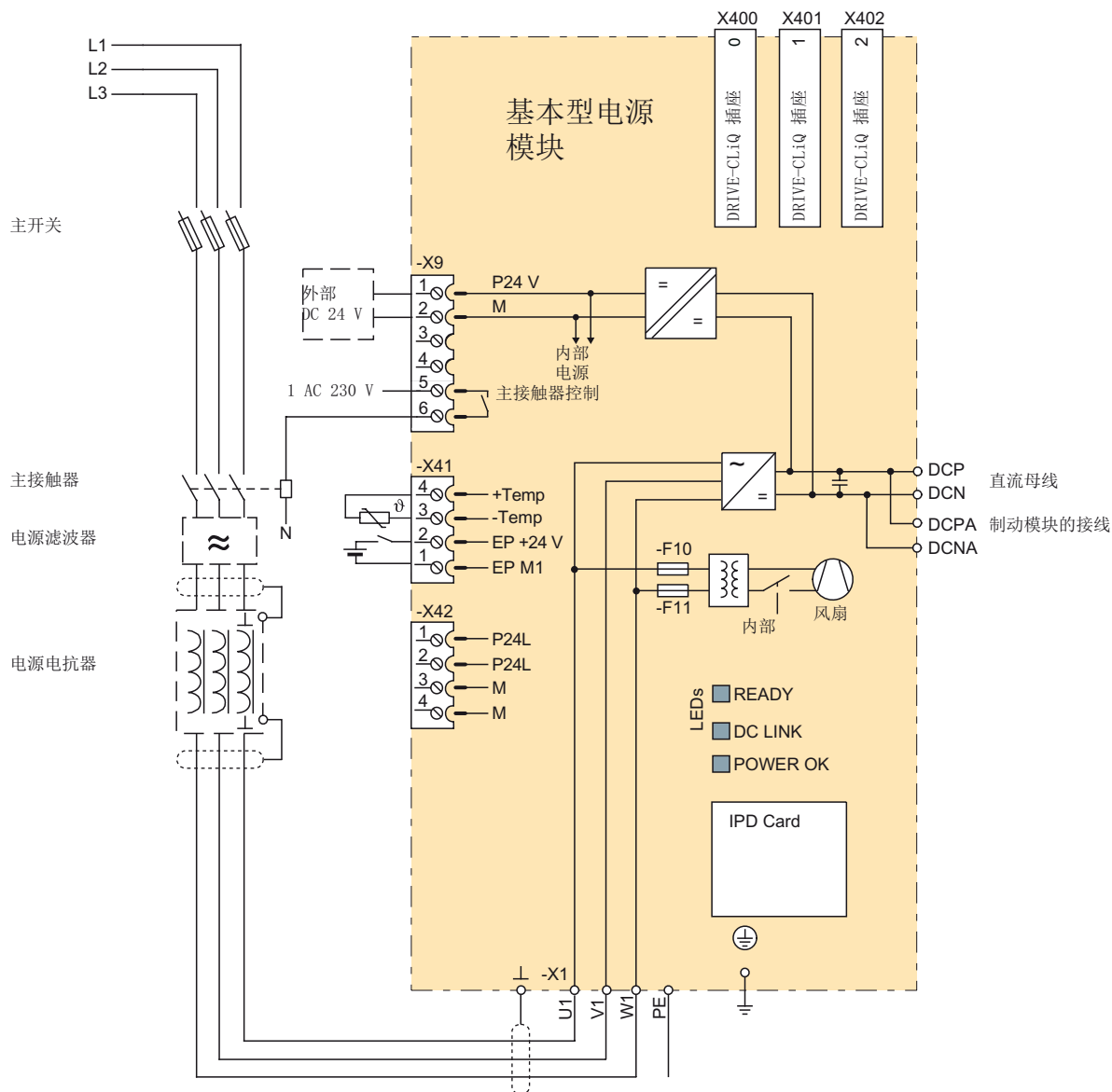
图 3-3 FB、GB 型基本型电源模块的接线示例
