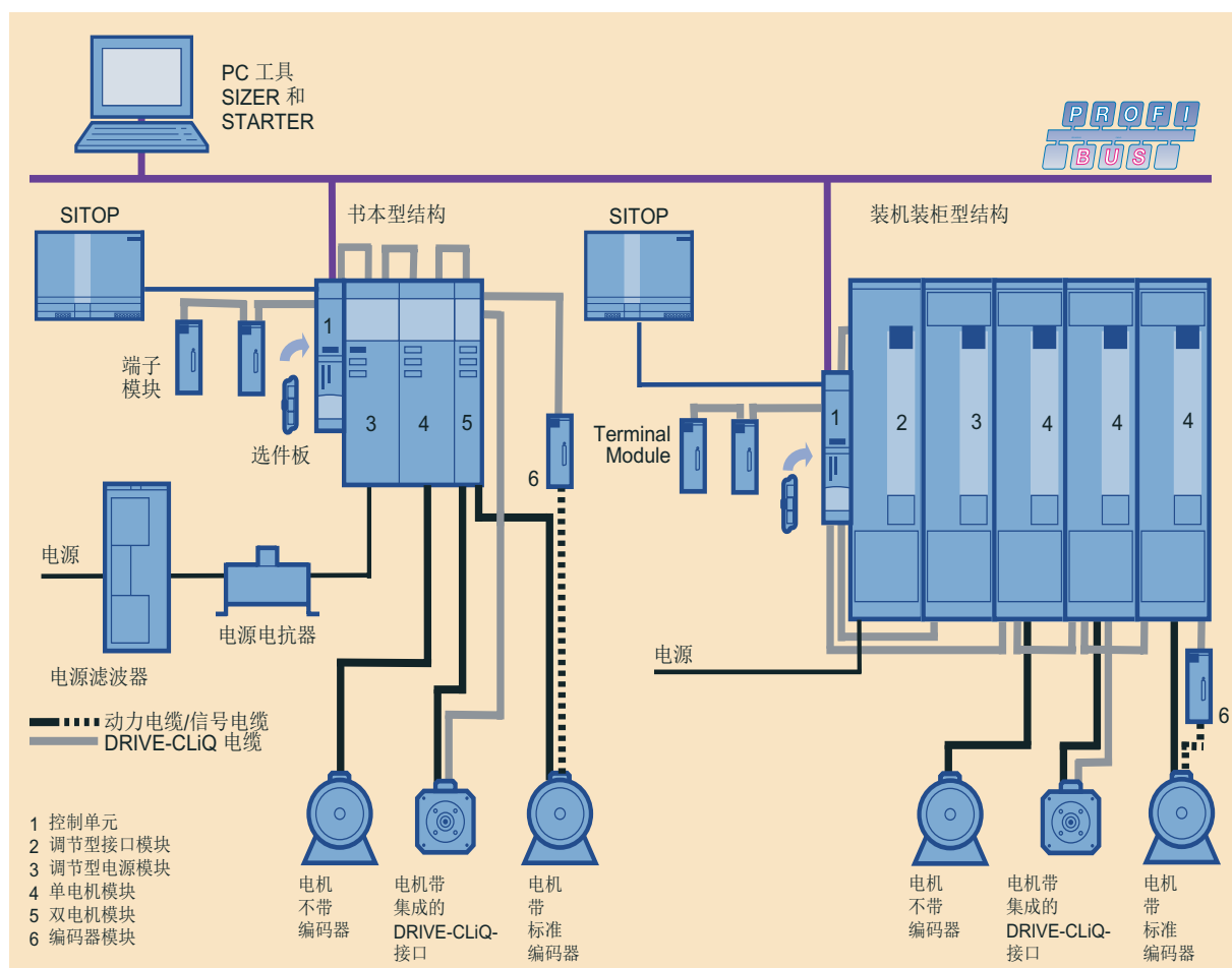
图 1-3 SINAMICS S120 系统概览
