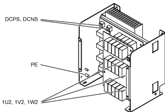
图 6-4 1 类电压峰值限制器的接口概览
