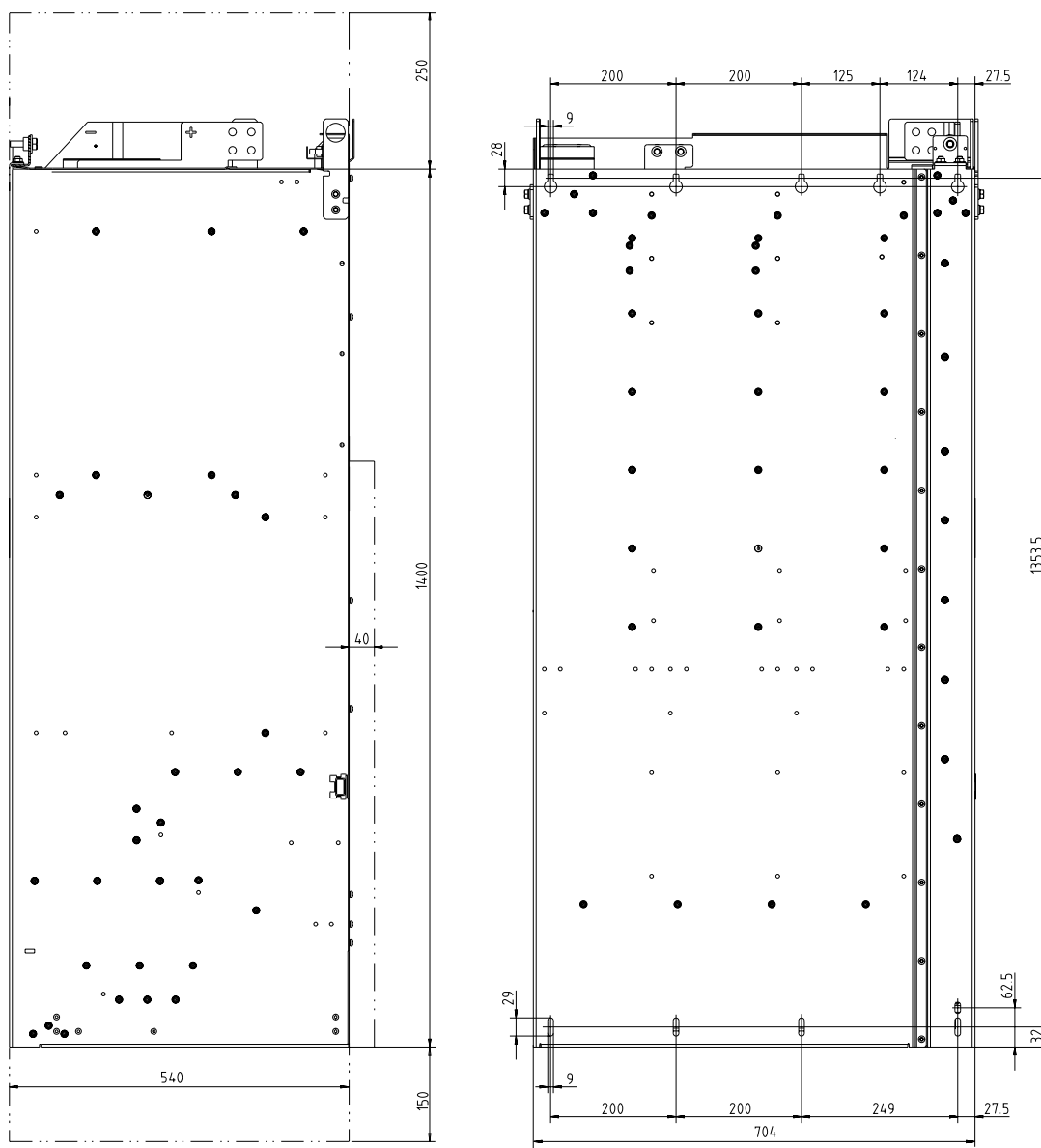
图 3-20 JX 型非调节型电源模块的外形尺寸图 侧视图和背视图
