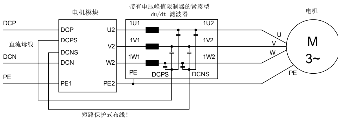
图 6-18 连接带有电压峰值限制器的紧凑型 du/dt 滤波器 - 整套设备
