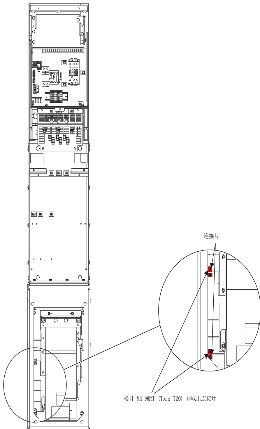
图 2-24 取出 HI 型调节型接口模块中的基本去干扰模块的连接片
