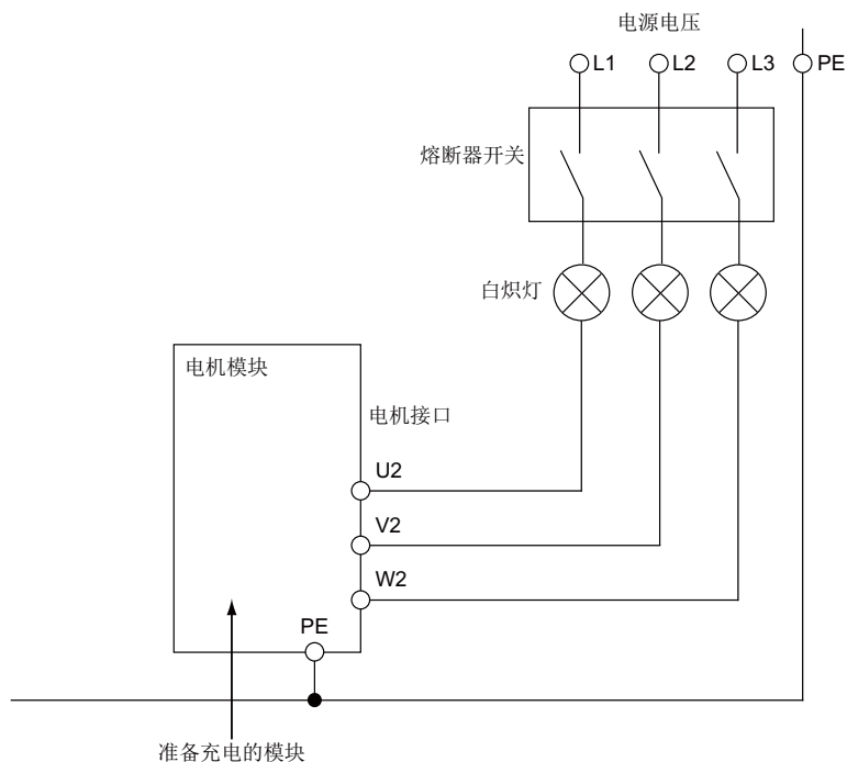
图 8-31 电机模块的充电回路
