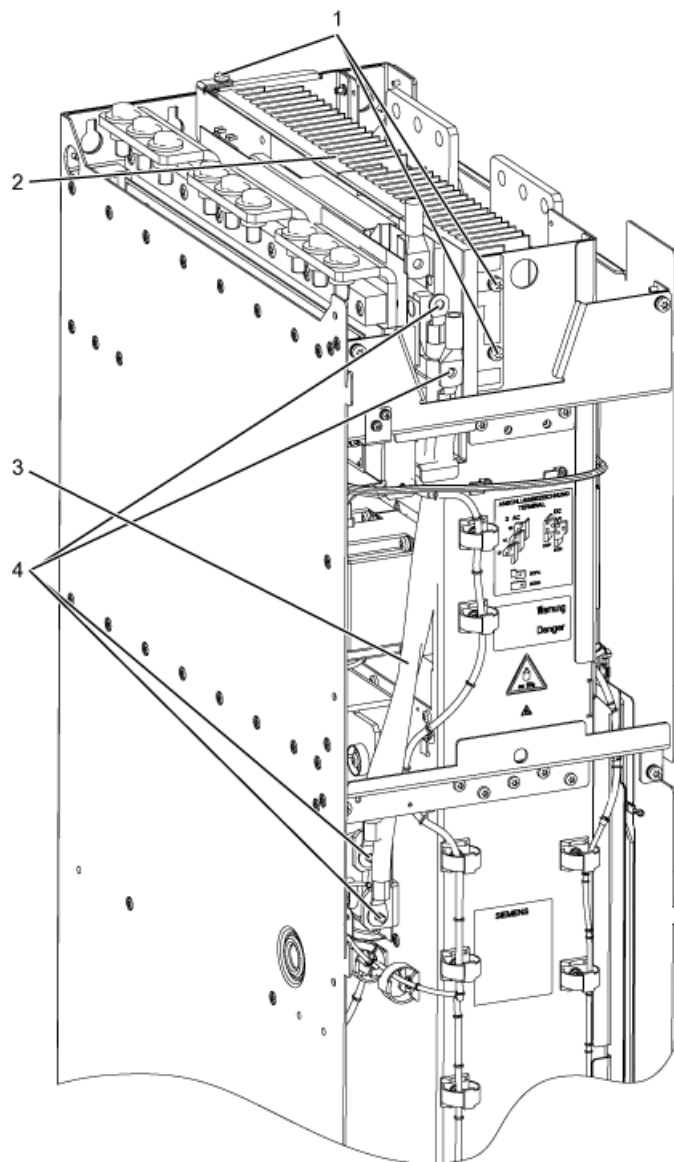
图 5-13 将制动模块安装到 GB、GD 型基本型电源模块中
