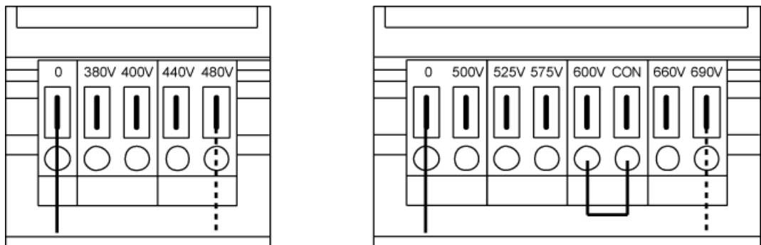
图 3-38 风扇变压器的可调端子(3 AC 380 到 480 V / 3 AC 500 到 690 V)
