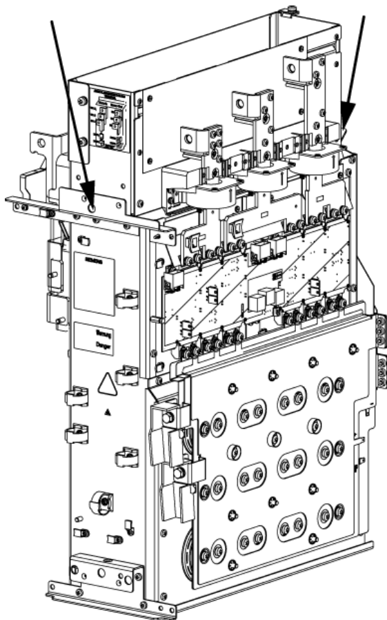
图 8-2 功率单元（FX、GX、FB 型）上的吊孔
