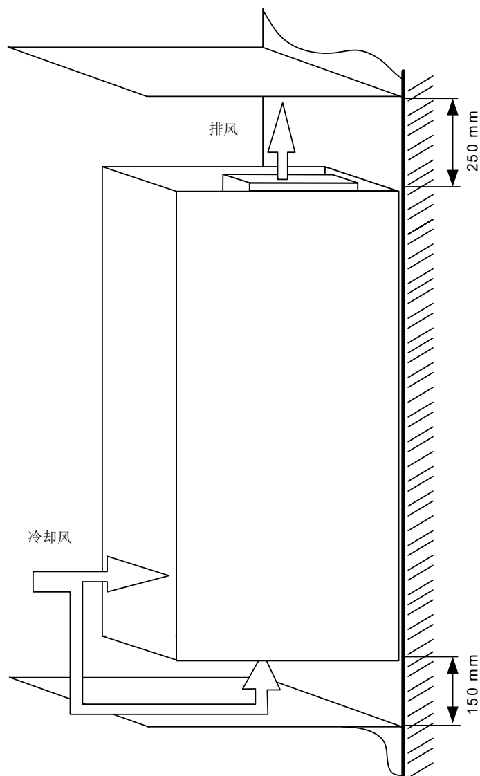
图 7-5 FB、GB、GD 型基本型电源模块的通风
