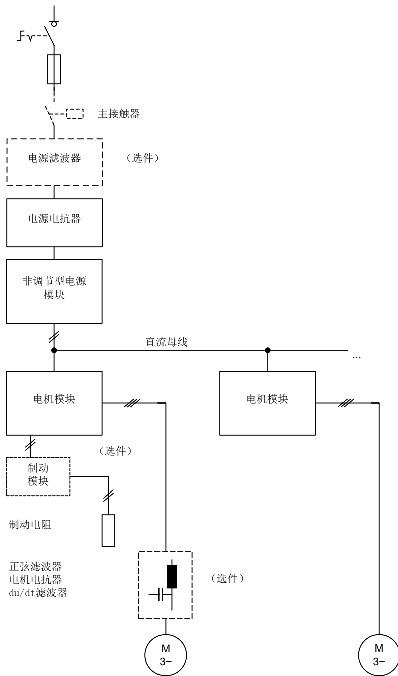
图 1-5 SINAMICS S120 和非受控型电源/再生馈电模块组成的驱动系统的基本结构
