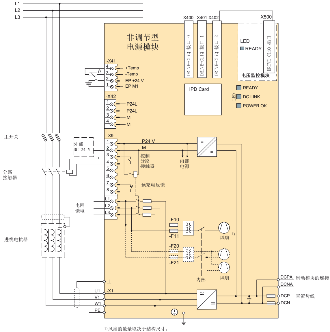
图 3-17 非调节型电源模块的连接图
