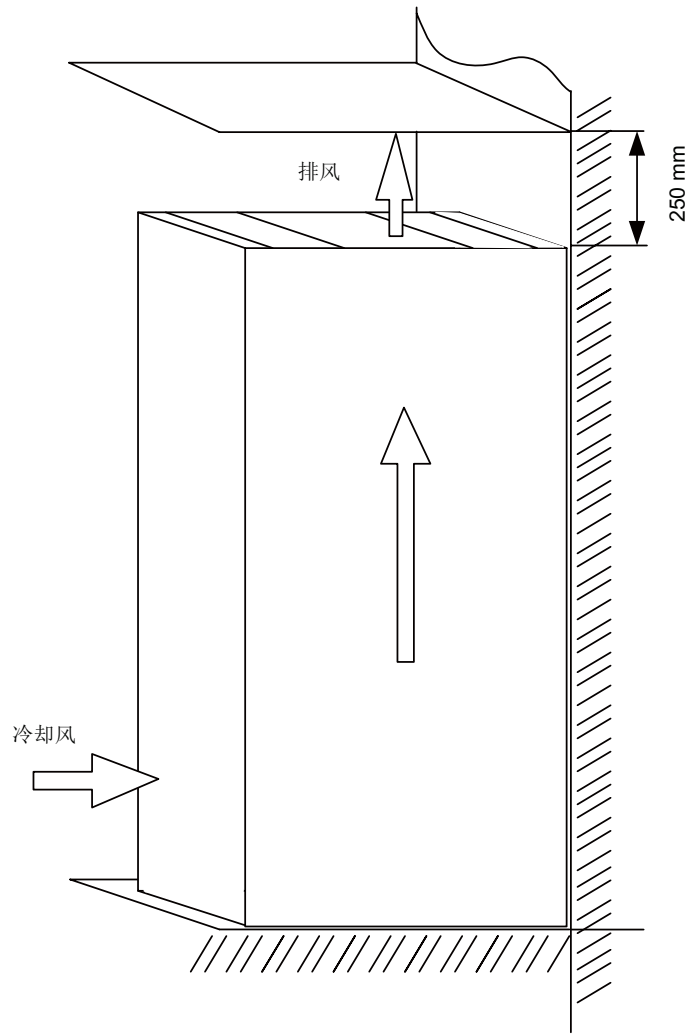
图 7-2 HI, JI 型调节型接口模块的通风
