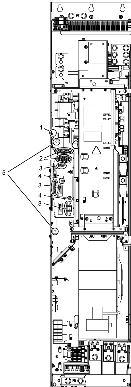
图 8-13 更换 GX 型非调节型/调节型电源模块和电机模块的控制接口模块
