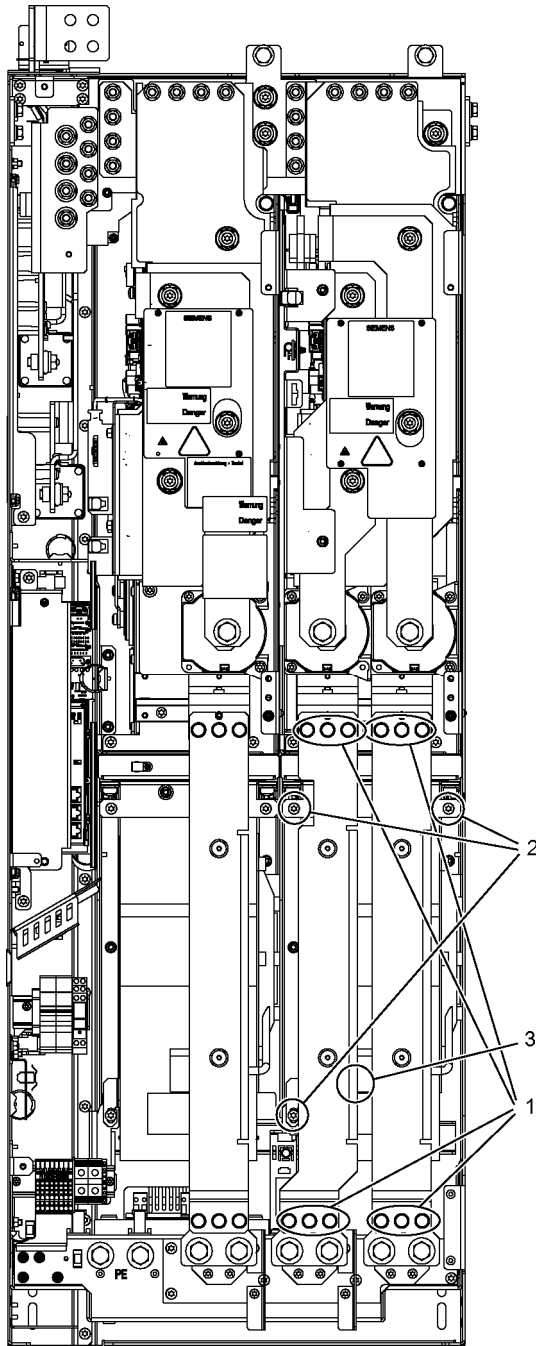
图 8-20 更换 HX 型非调节型/调节型电源模块、电机模块、右侧功率单元的风扇
