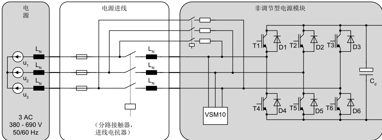
图 3-13 非调节型电源概览
