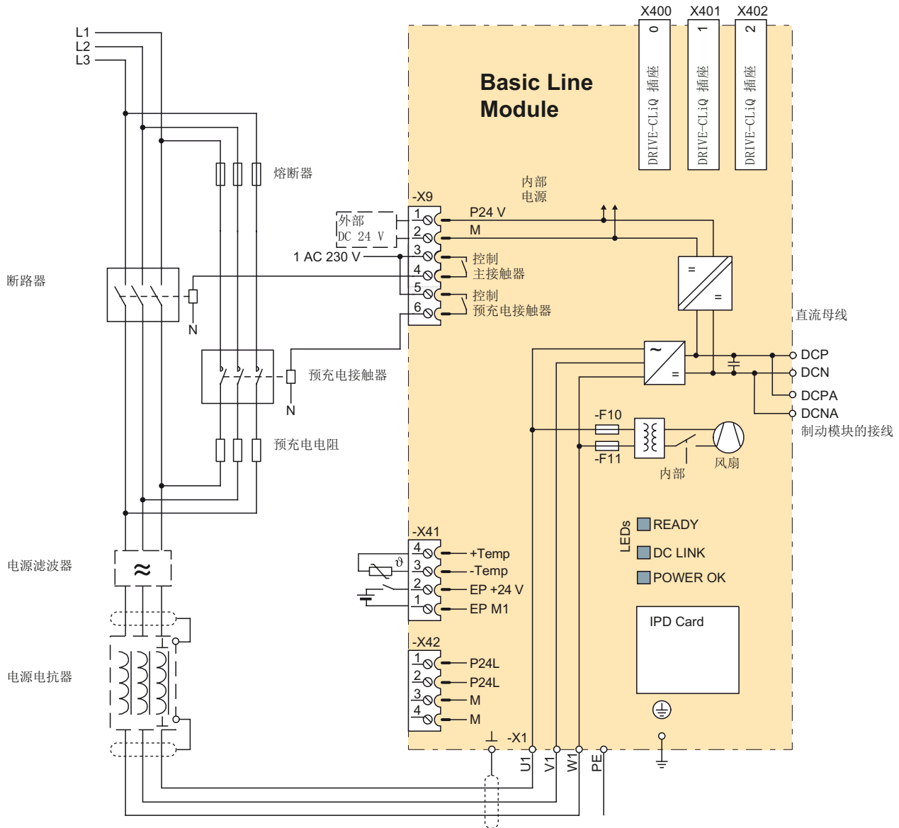
图 3-11 GD 型基本型电源模块的接线示例
