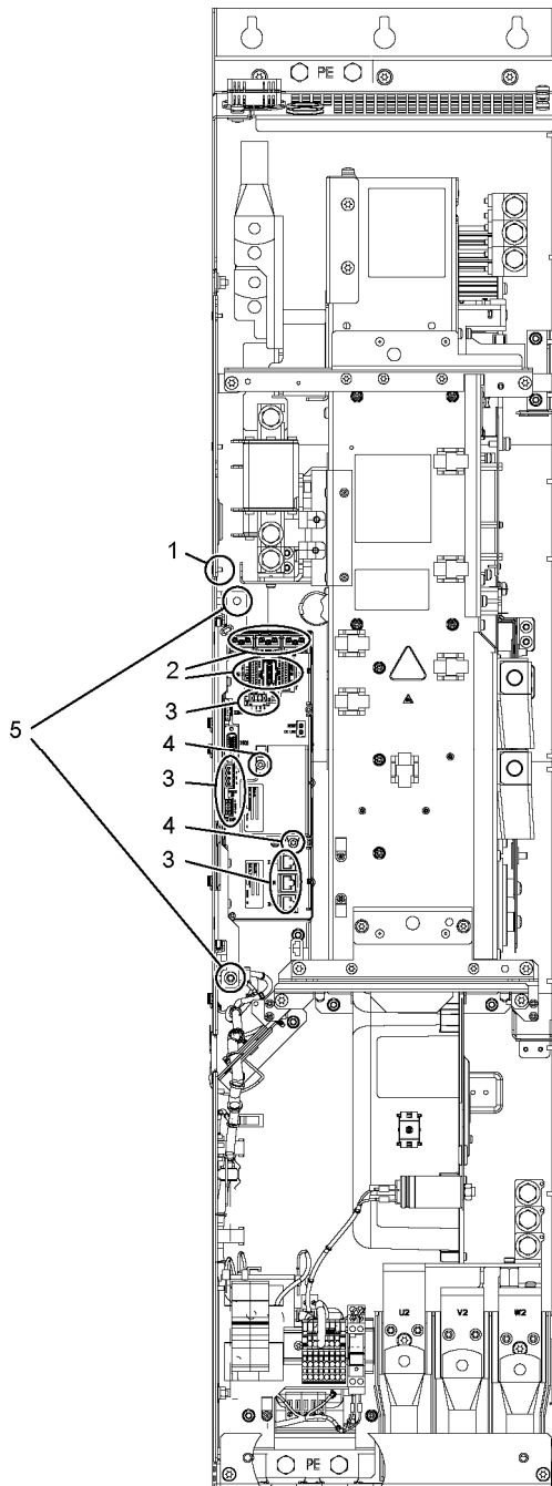
图 8-12 更换 FX 型调节型电源模块和电机模块的控制接口模块
