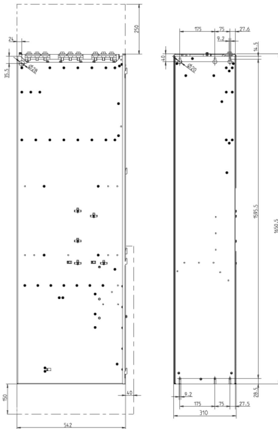
图 3-6 GB、GD 型基本型电源模块的外形尺寸图 侧视图和背视图
