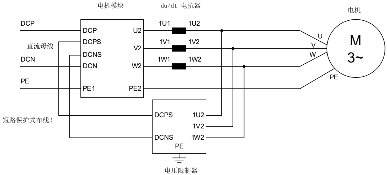
图 6-7 连接带有电压峰值限制器、一个 du/dt 电抗器的 du/dt 滤波器
