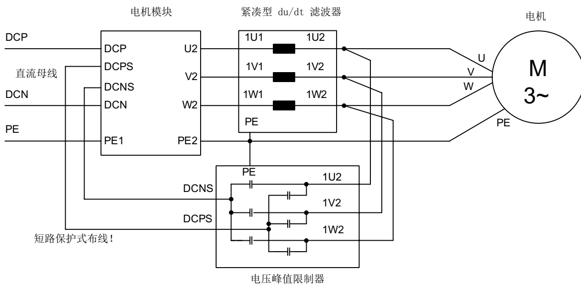
图 6-19 连接带有电压峰值限制器的紧凑型 du/dt 滤波器 - 单个组件
