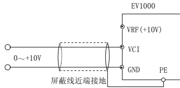
图 3-9 VCI 端子配线图
