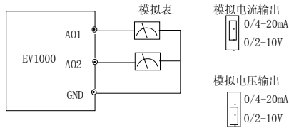
图 3-11 模拟输出端子配线
