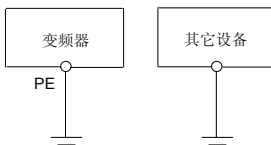
图 3-26 接地示意图 1
