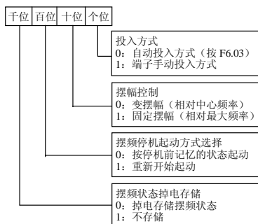
图 5-37 摆频运行方式参数含义
