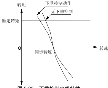
图 5-65 下垂控制电机特性
