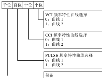
图 5-9 频率给定曲线选择
