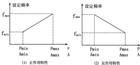
(1) 正作用特性
