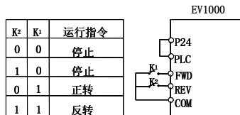
图 5-42 两线式运转模式 2
