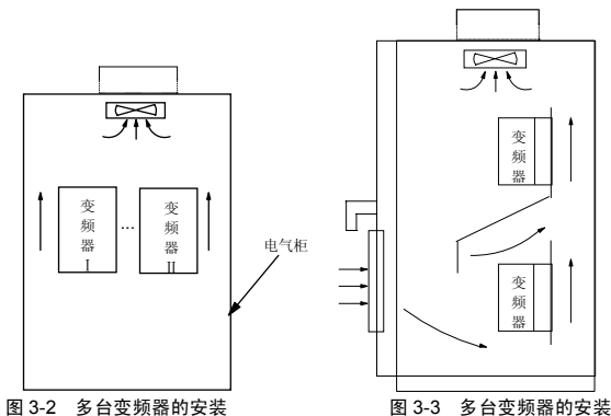
图 3-2 多台变频器的安装
