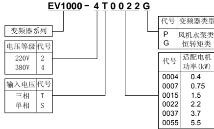
图 2-1a EV1000 变频器型号
