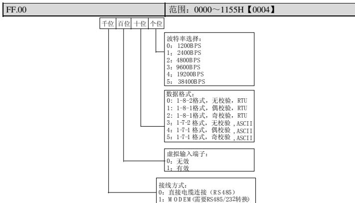
图 5-68 通讯配置设定
