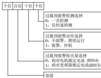
图 5-72 过载检出设置设定
