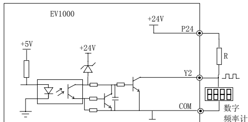
图 3-21 输出端子 Y2 连接方式 1
