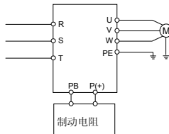
图 2-4 变频器与制动电阻连线图
