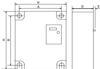
图 2-2 EV1000 变频器外形图
