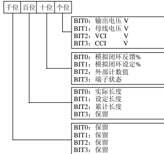
图 5-52 LED 运行显示参数选择 2 设定
