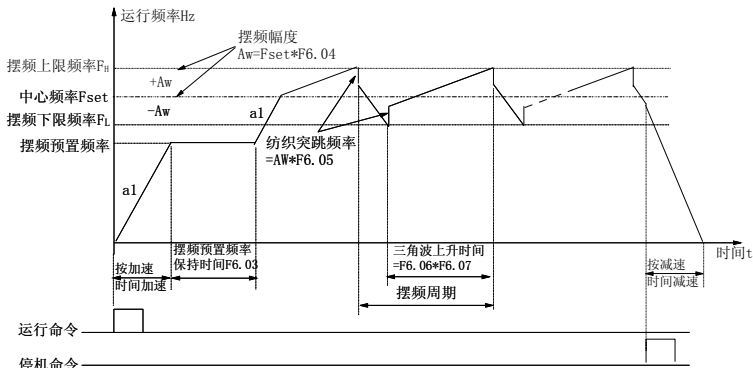
图 5-36 摆频示意图
