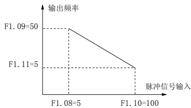
图 5-10 脉冲信号输入实例参数设置
