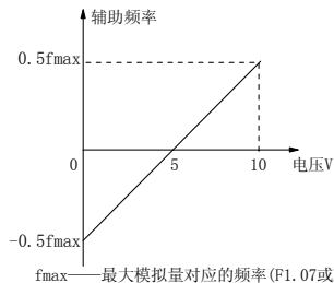
图 5-60 VCI-5 或 CCI-5 作为辅助频率给定通道
