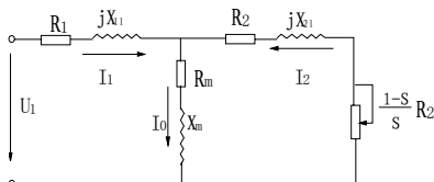
图 5-69 异步电机稳态等效电路图
