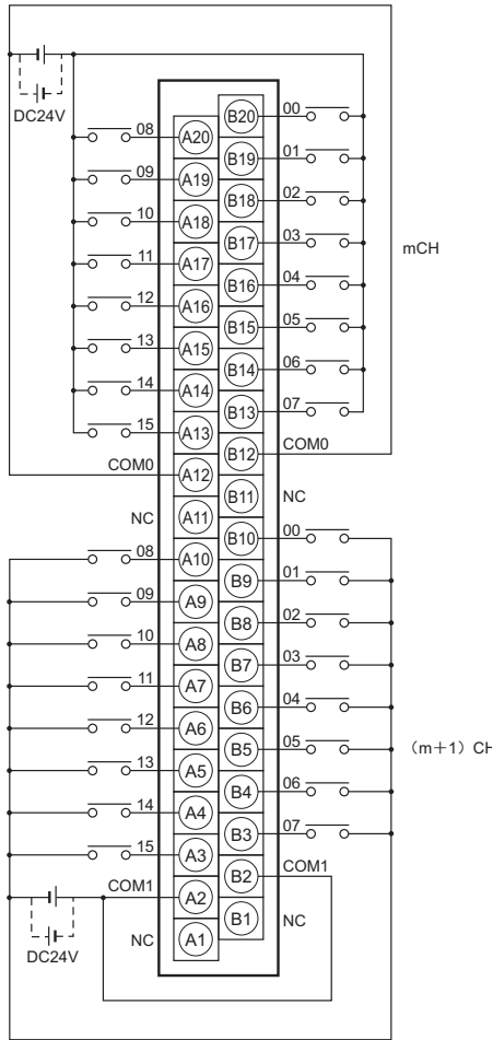
连接图
