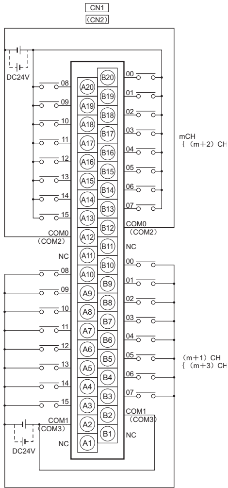
连接图
