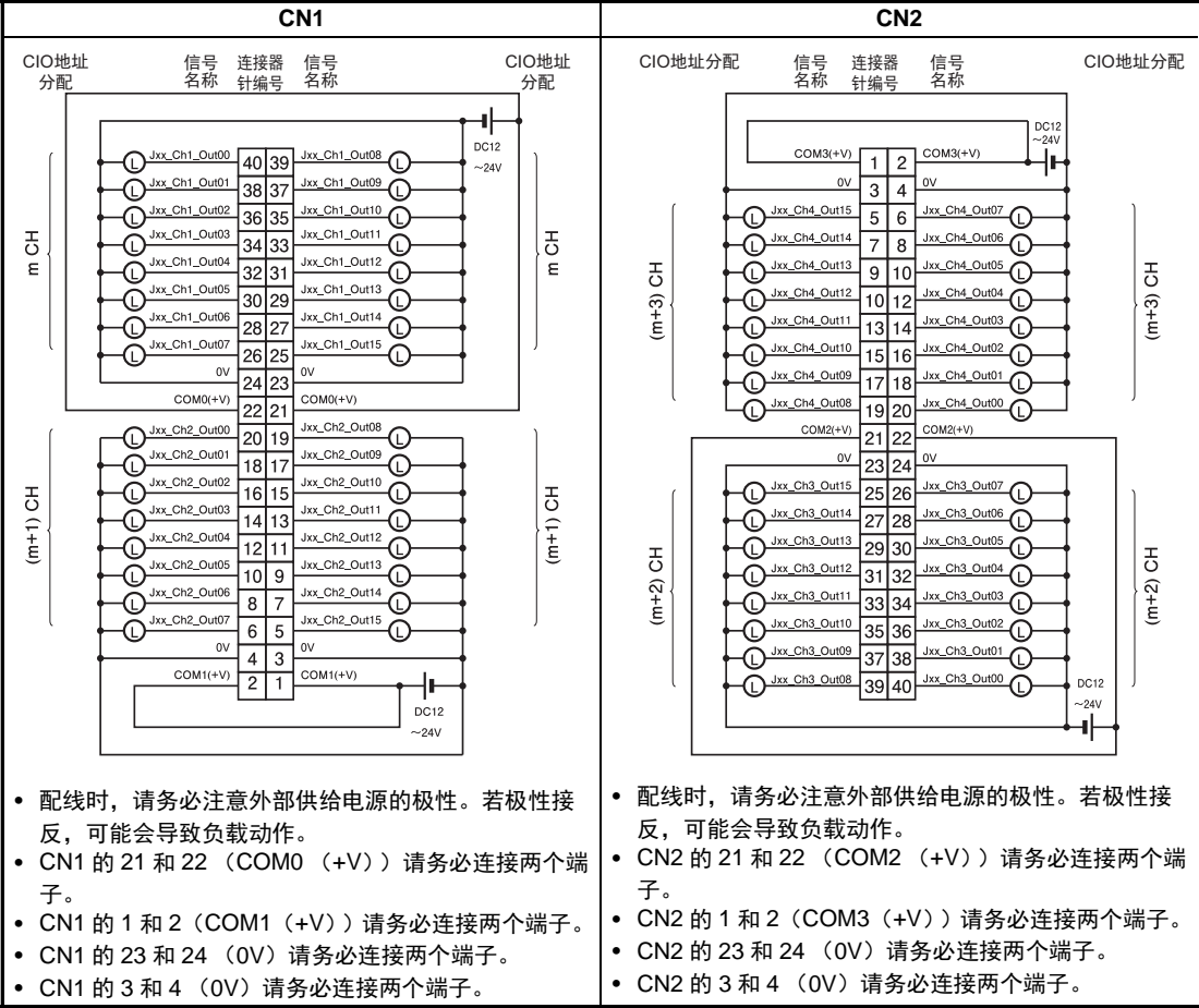
外部连接图 端子和设备变量的对应图
