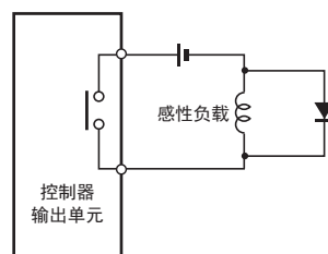
DC回路时安装二极管
