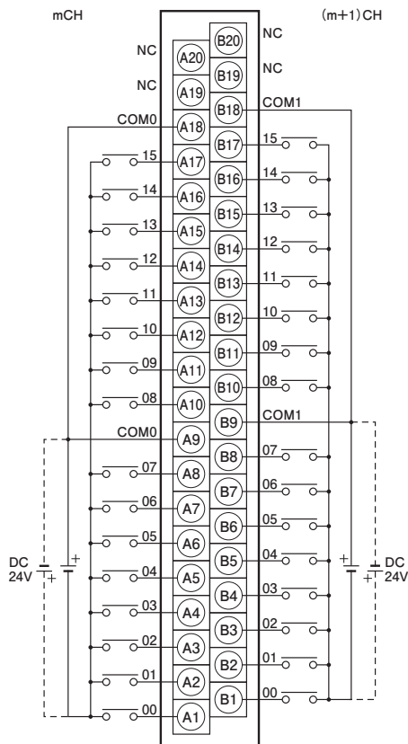
连接图
