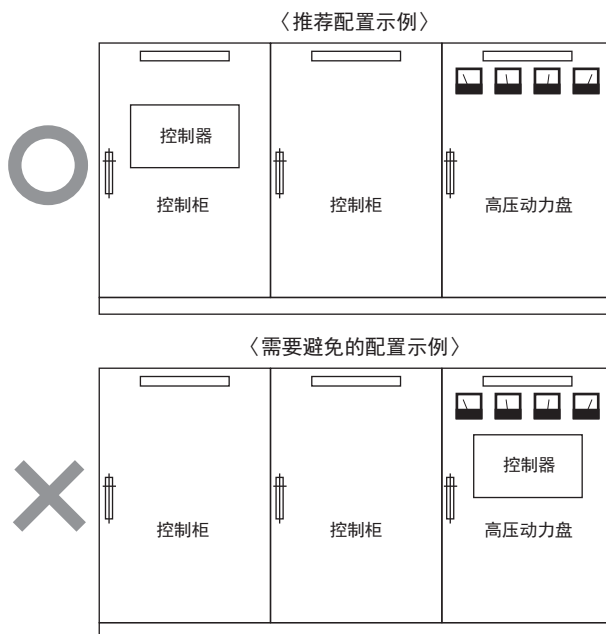
安装到有高压设备的控制柜内的示例
