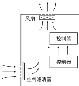
强制通风式
