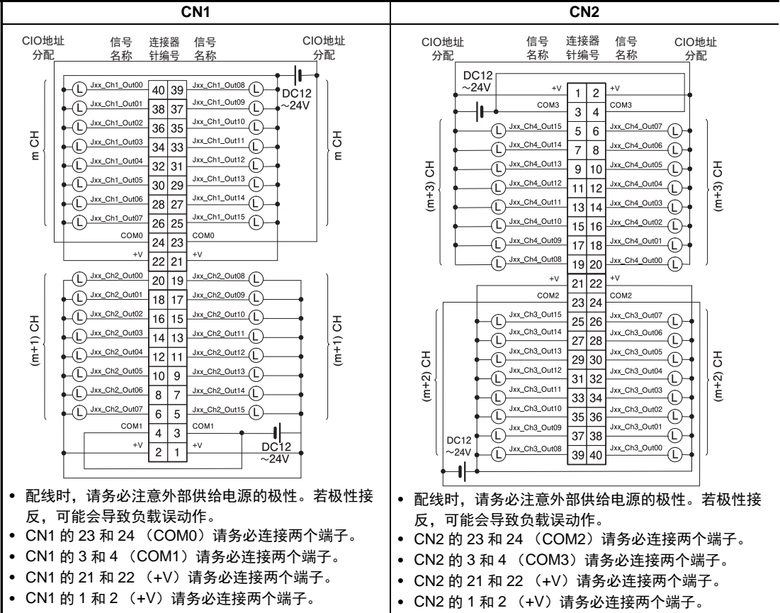
外部连接图 端子和设备变量的对应图
