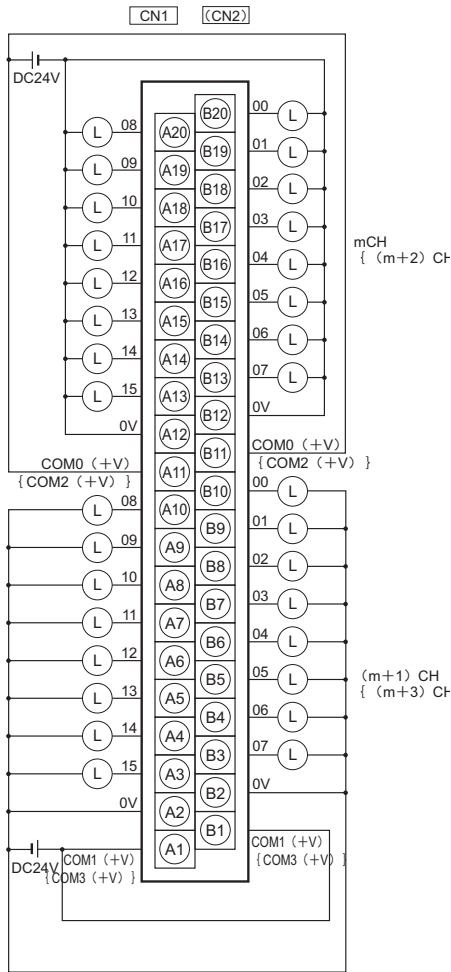
连接图
