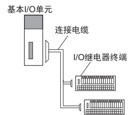
与 I/O 继电器终端连接的示例
