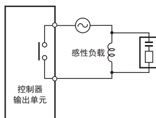
AC回路时安装浪涌抑制器
