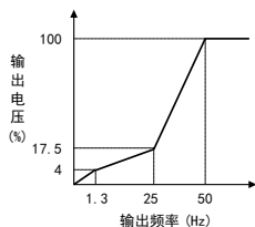
■ 3点固定模式4
