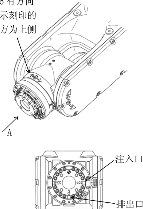
视图 A RS06L, RS10N
