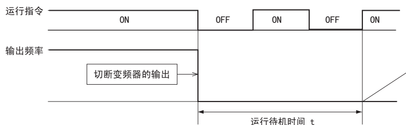
图 48 带定时的自由运行停止
