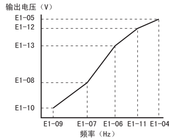
图 55 V/f 曲线图
