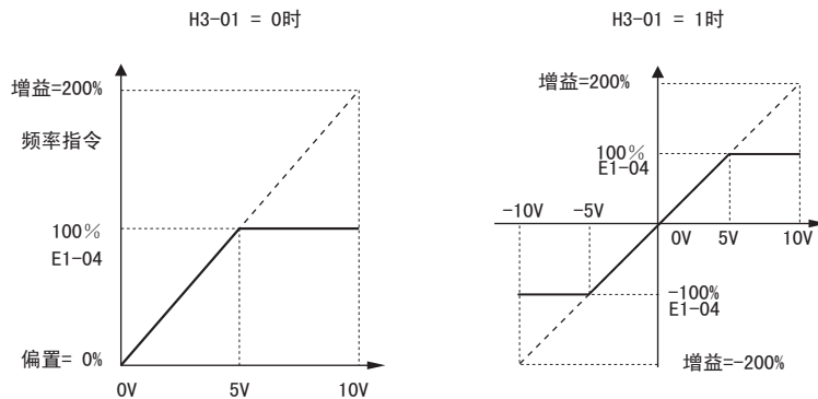
图 60 调整了模拟量输入的增益设定时的频率指令
