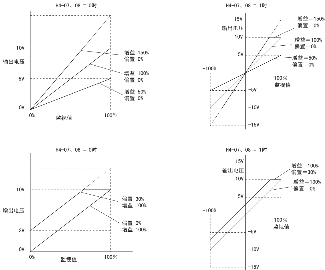
图 62 模拟量输出的增益 / 偏置设定
