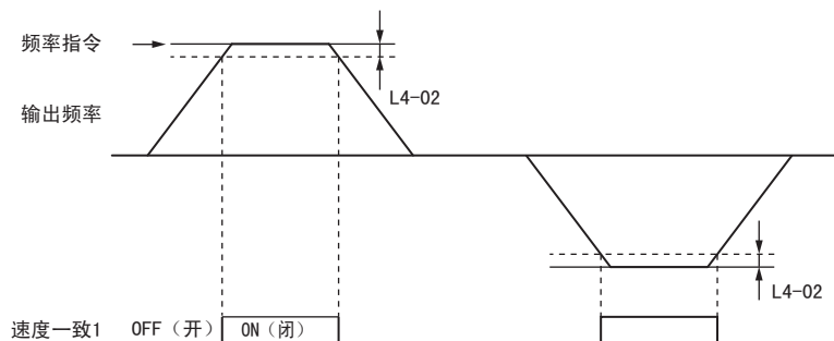
图 58 速度一致 1 的时序图
