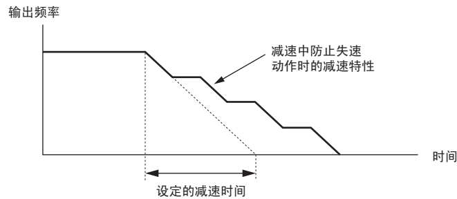
图 66 减速中防止失速的动作示例
