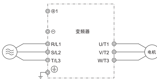
图 11 主回路端子的连接
