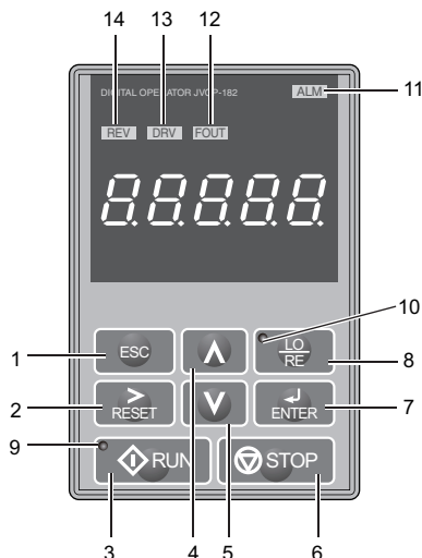
图 38 操作器各部分的名称与功能
