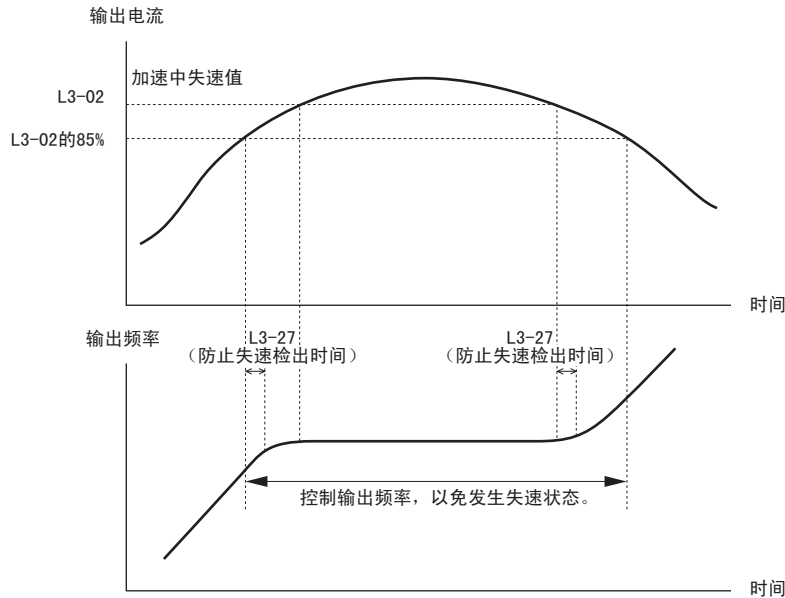
图 63 使用 IM 电机时的加速中防止失速功能
