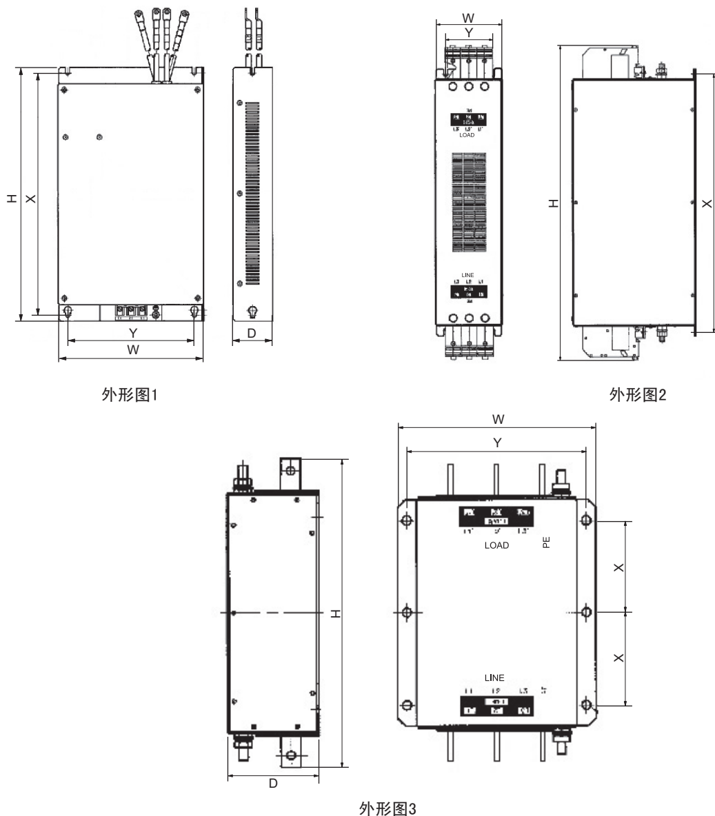
图 79 EMC 噪音滤波器的外形尺寸
