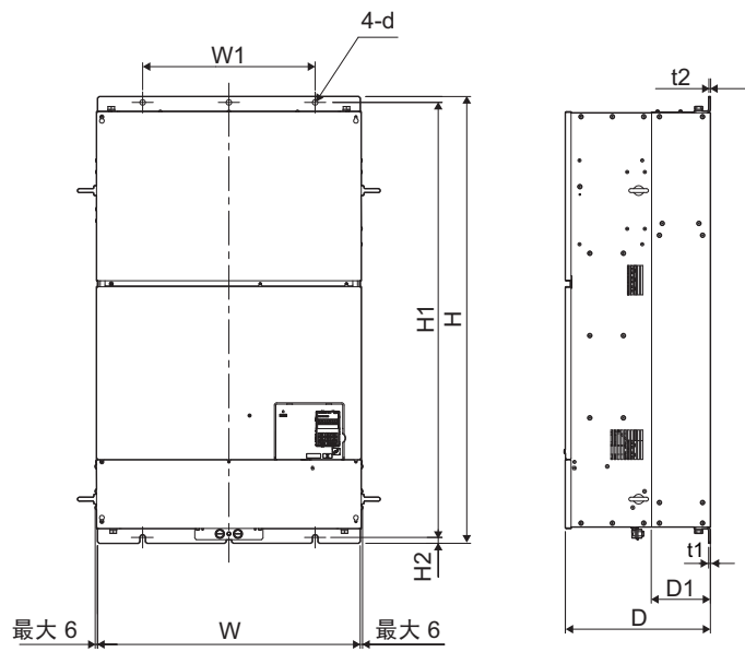
外形图 5
