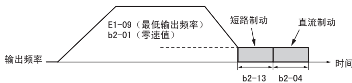
图 51 停止时短路制动（无 PG：PM 电机）
