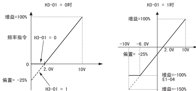
图 61 设定了负值偏置时的频率指令
