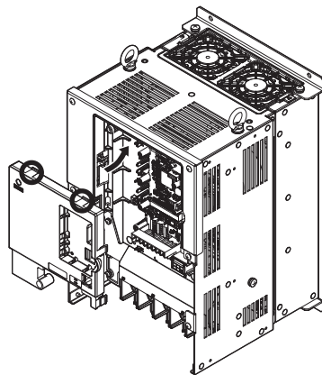
图 24 前外罩的安装 (2A0110 ~ 2A0415, 4A0058 ~ 4A0675)
