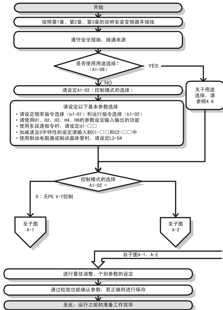
图 40 运行前的基本步骤
