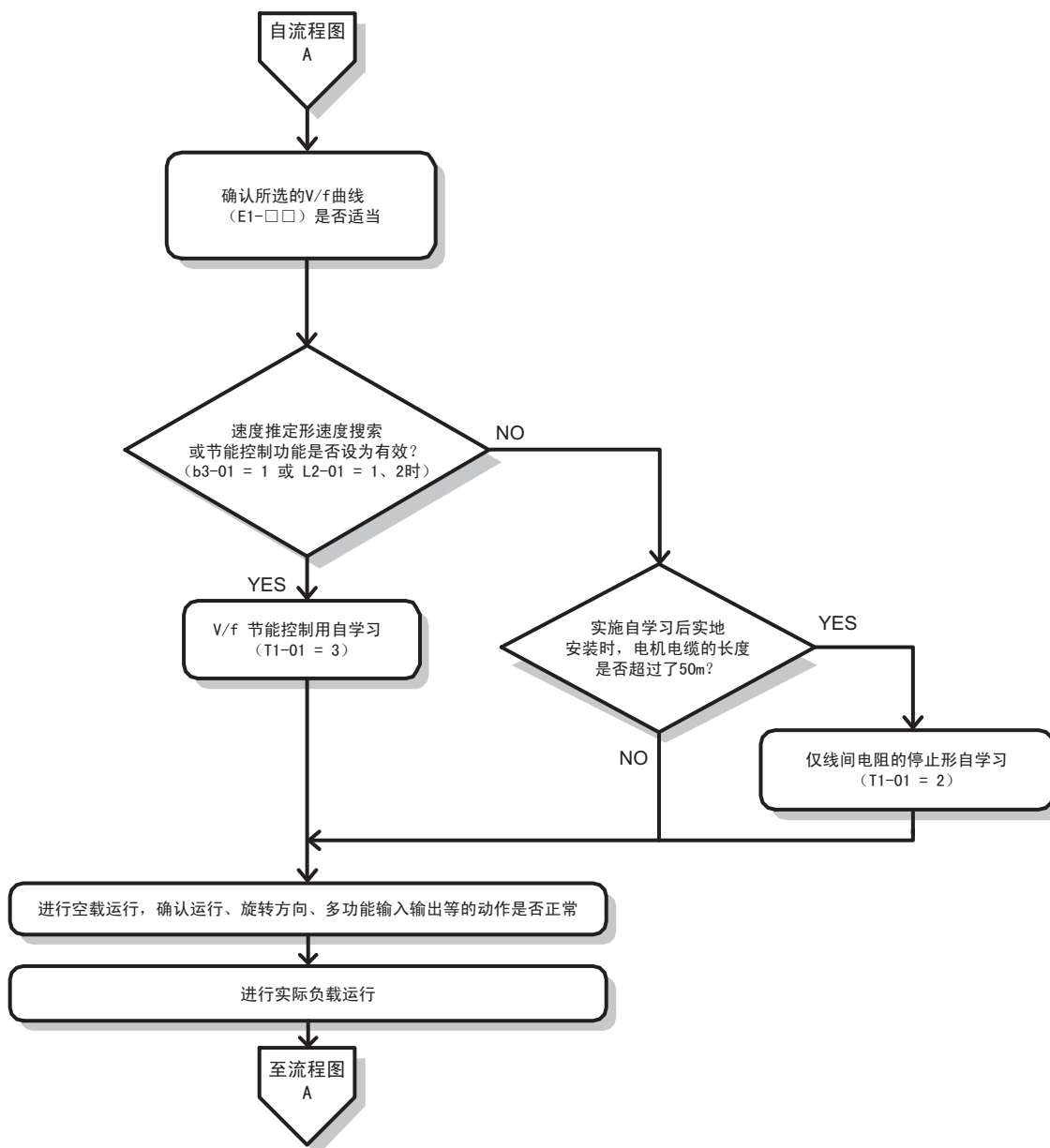
图 41 V/f 控制下的节能运行或速度搜索等简单的运行
