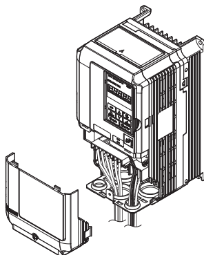
图 69 变频器的更换（端子外罩的拆卸）
