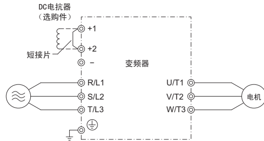
图 10 主回路端子的连接
