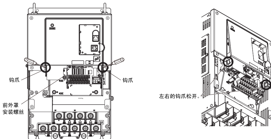
图 22 前外罩的拆卸 (2A0110 ~ 2A0415, 4A0058 ~ 4A0675)
