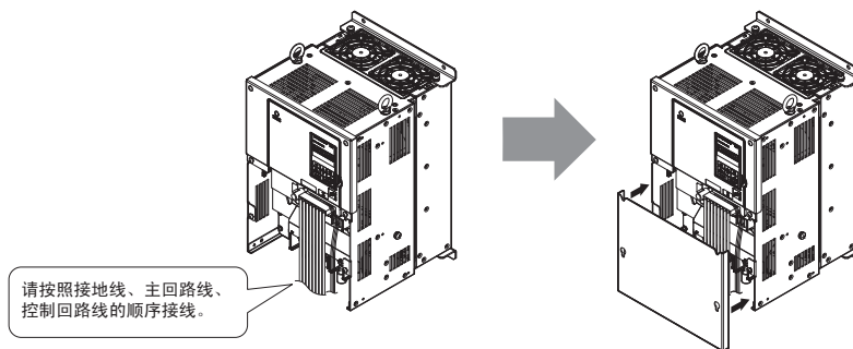
图 18 端子外罩的安装方法（柜内安装型）
