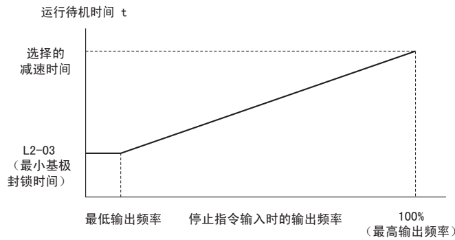
图 49 运行等待时间与输出频率的关系
