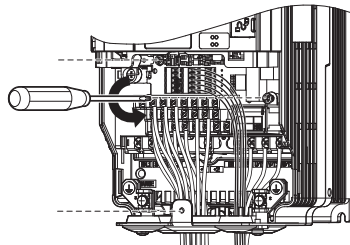
图 70 变频器的更换（拧松固定螺丝）
