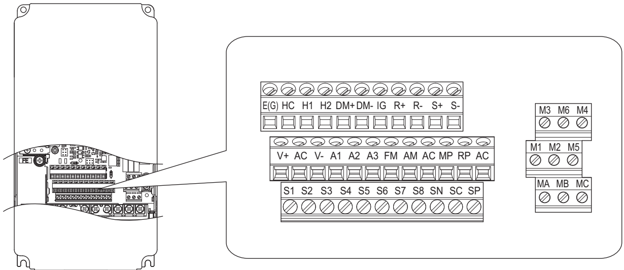
图 31 端子排的排列
