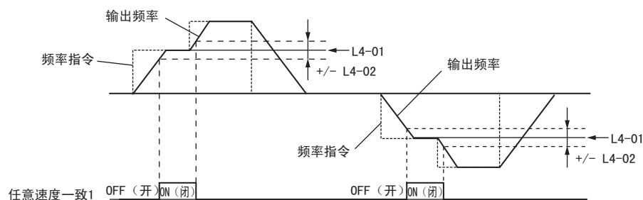
图 59 任意速度一致 1 的时序图
