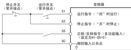
图 56 3 线制顺控的接线示例
