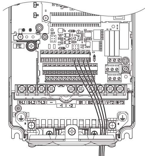
图 34 端子排的接线
