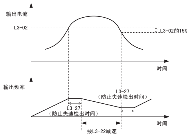
图 64 PM 用无 PG 矢量控制时的加速中防止失速功能
