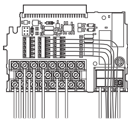
图 72 变频器的更换 (已拆下的拆装式端子排)
