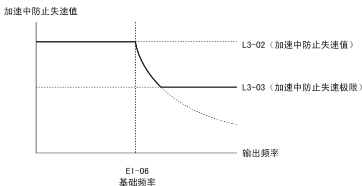
图 65 加速中防止失速值 / 极限
