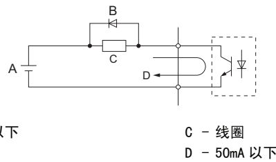
图 30 旁路二极管的连接
