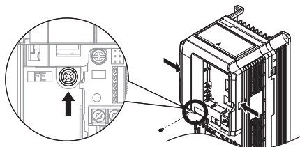
图 21 前外罩的拆卸 (2A0004 ~ 2A0081, 4A0002 ~ 4A0044)
