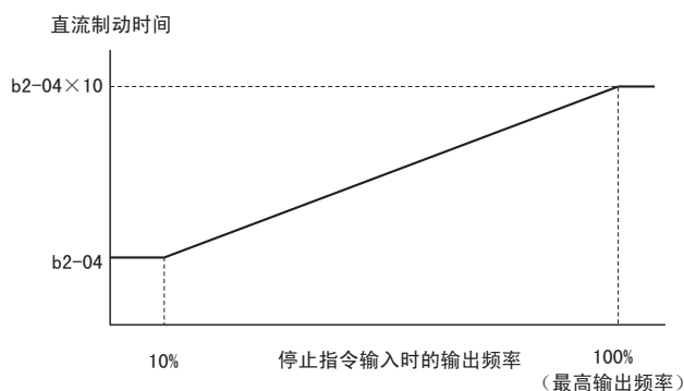
图 47 直流制动时间与输出频率的关系
