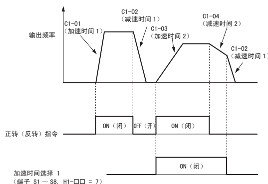
图 52 加减速时间的时序图
