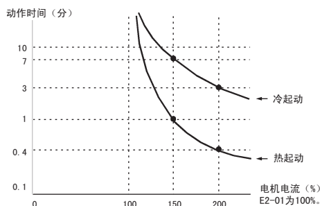
图 81 由输出频率和负载决定的电机过载保护时间
