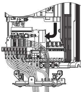
图 71 变频器的更换（端子排的拆卸）
