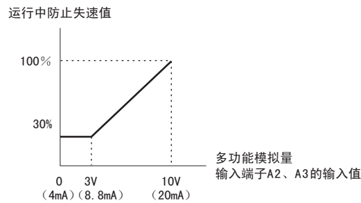
图 67 通过模拟量输入设定运行时防止失速值
