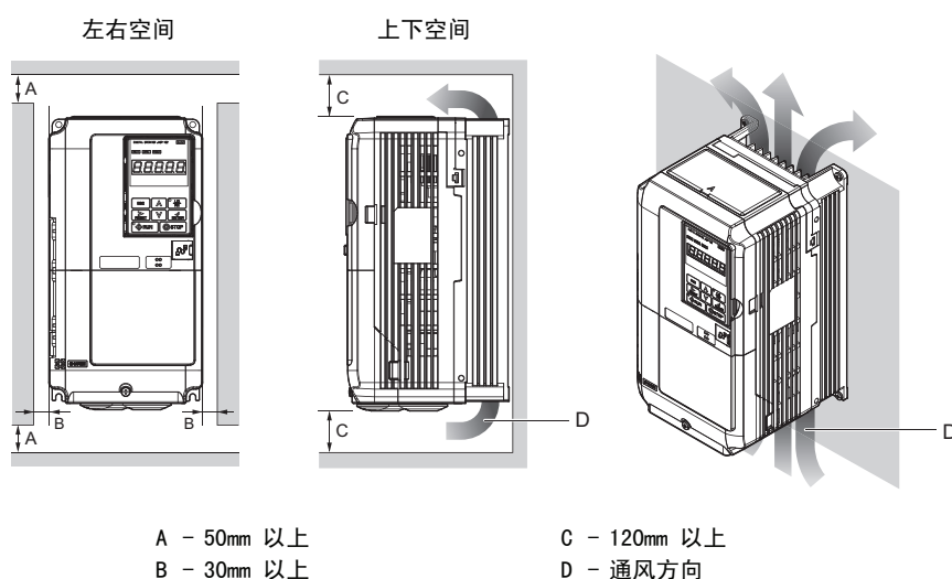
图 5 变频器的安装空间（单机）
