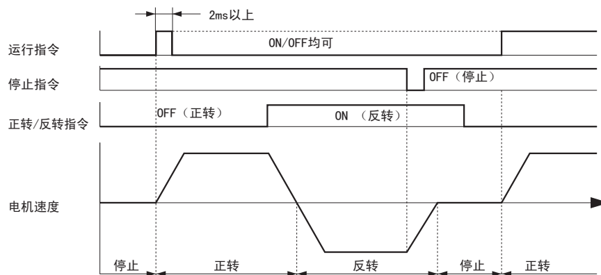
图 57 3 线制顺控的时序图
