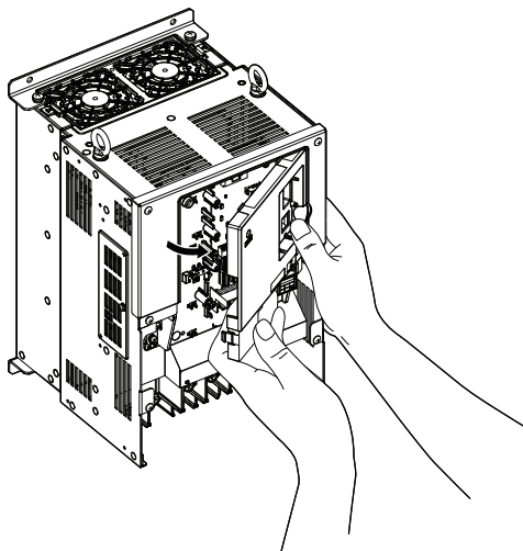
图 23 前外罩的拆卸 (2A0110 ~ 2A0415, 4A0058 ~ 4A0675)
