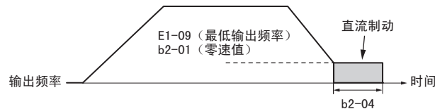
图 50 无 PG V/f 控制、无 PG 矢量控制时的停止时直流制动动作
