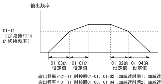
图 53 加减速时间的切换频率
