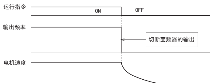
图 45 自由运行停止
