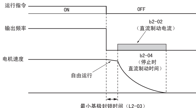
图 46 全域直流制动（DB）停止
