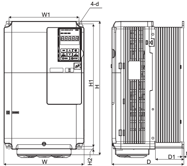
外形图 2
