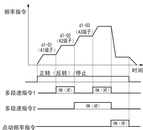
图 54 多段速指令 / 点动频率选择的时序图
