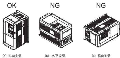
图 4 安装方向
