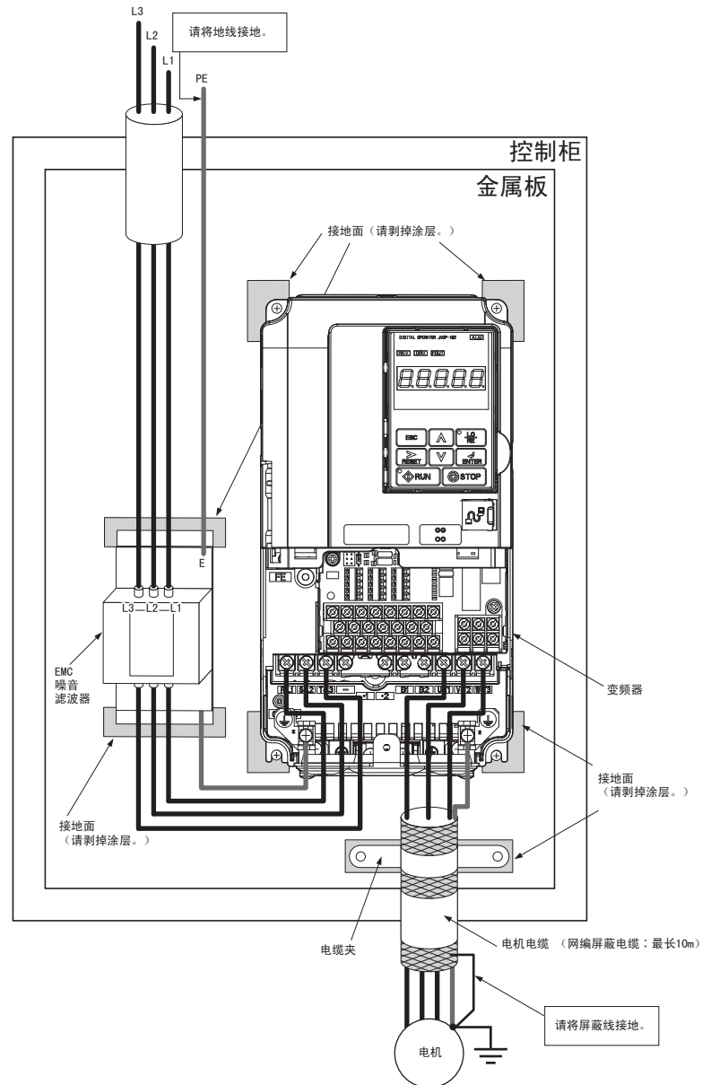
图 78 EMC 噪音滤波器和变频器的安装方法 (三相 200V/400V 级)
