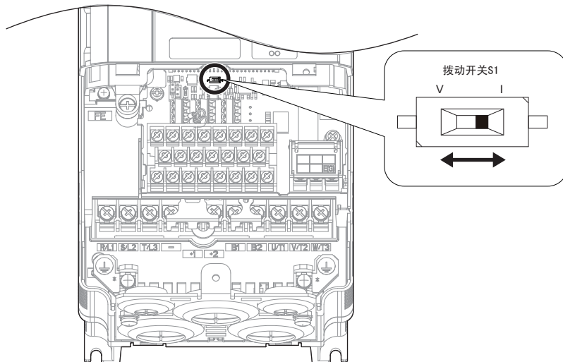
图 36 拨动开关 S1
