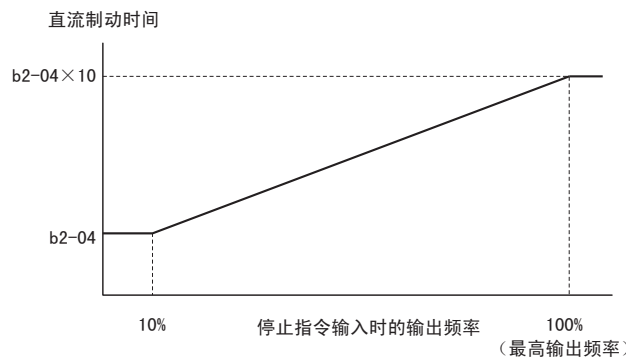
图 50 直流制动时间与输出频率的关系
