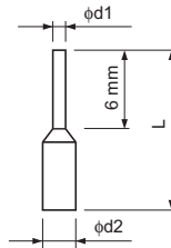
图 27 棒端子的外形尺寸图
