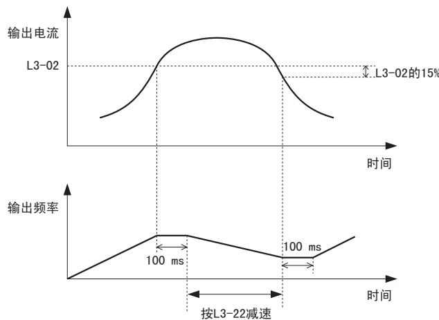
图 68 PM 用无 PG 矢量控制时的加速中防止失速功能
