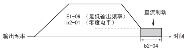
图 53 无 PG V/f 控制、带 PG V/f 控制、无 PG 矢量控制时的停止时直流制动动作
