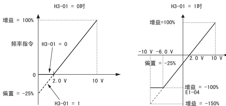
图 65 设定了负值偏置时的频率指令
