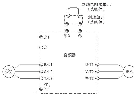
图 10 主回路端子的连接
