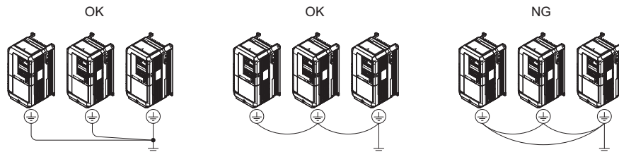
图 22 多台变频器的接线
