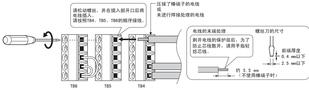
图 28 控制回路的接线步骤
