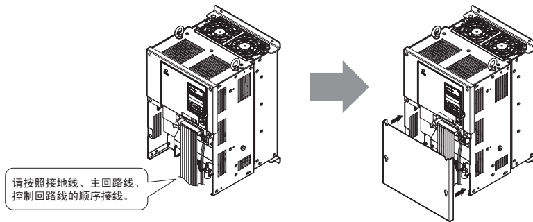
图 16 端子外罩的安装方法（柜内安装型）
