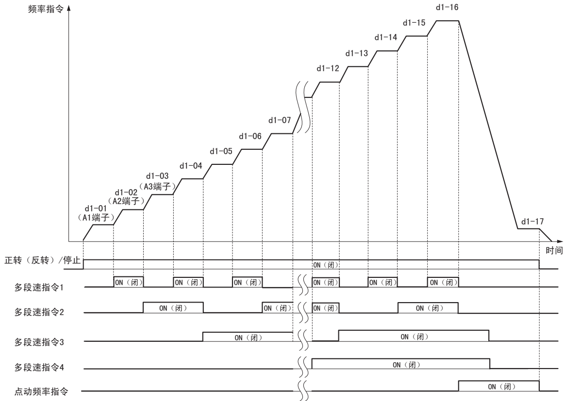
图 58 多段速指令 / 点动频率选择的时序图
