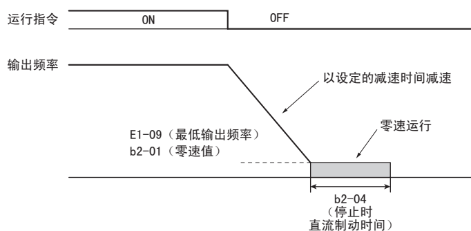
图 47 减速停止（带 PG 矢量控制、PM 用带 PG 矢量控制模式时）
