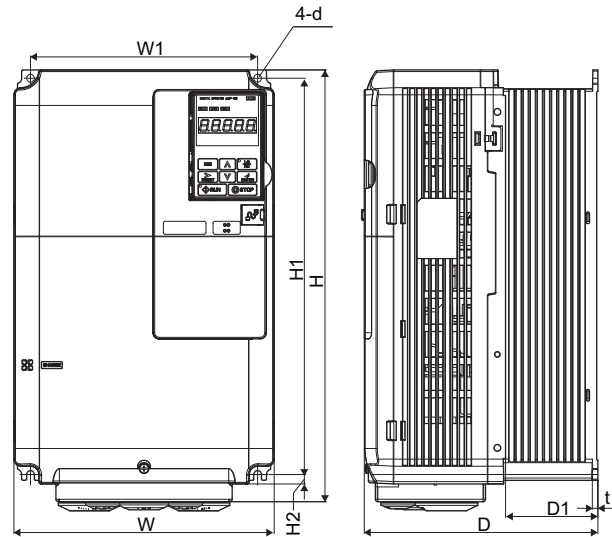
外形图 2
