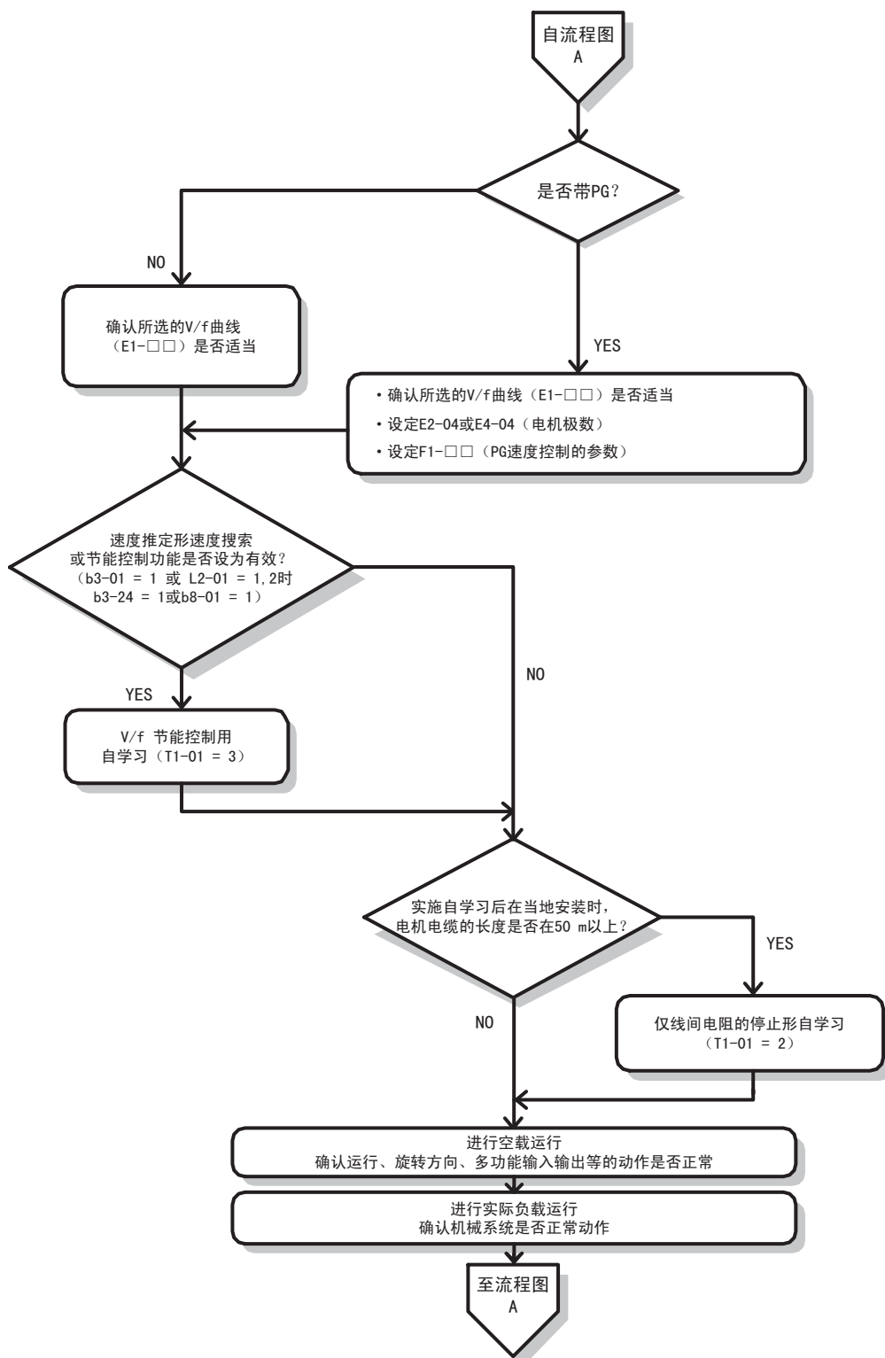
图 40 V/f 控制下的节能运行或速度搜索等简单的运行
