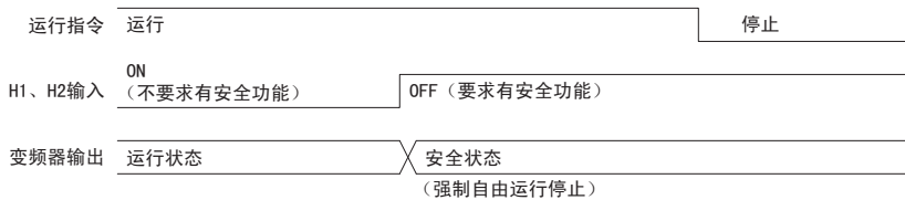
图 89 如果在运行中将安全输入置为 OFF，电机将自由运行停止
