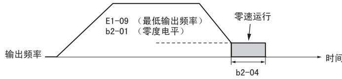
图 55 停止时零速运行
