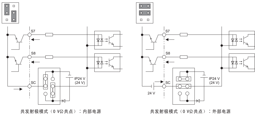
图 32 共发射极模式（0 V 公共点）
