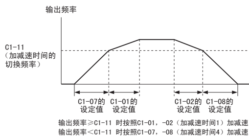
图 57 加减速时间的切换频率
