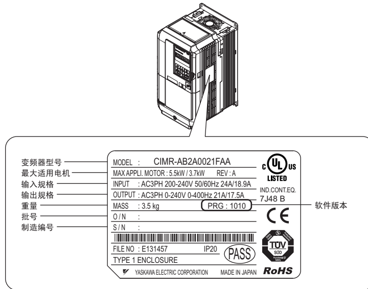
图 1 变频器的铭牌
