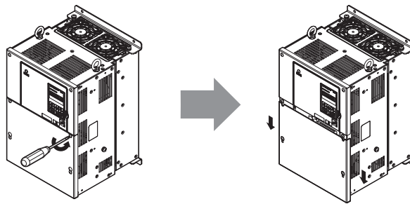
图 14 端子外罩的拆卸方法（柜内安装型）
