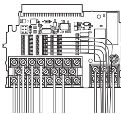
图 77 变频器的更换 (已拆下的拆装式端子排)
