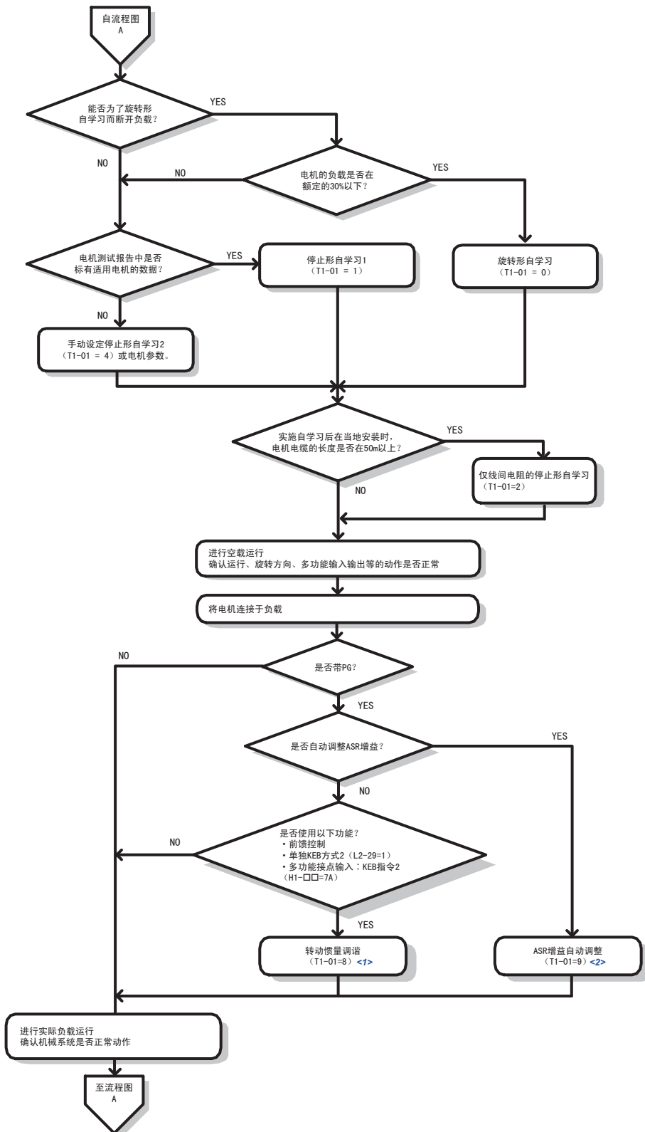
图 41 无 PG/带 PG 矢量控制下的高精度运行
