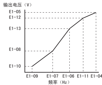
图 59 V/f 曲线图
