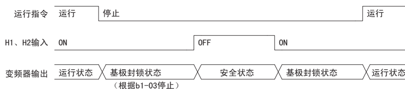
图 90 从安全状态 (ST0 状态) 返回
