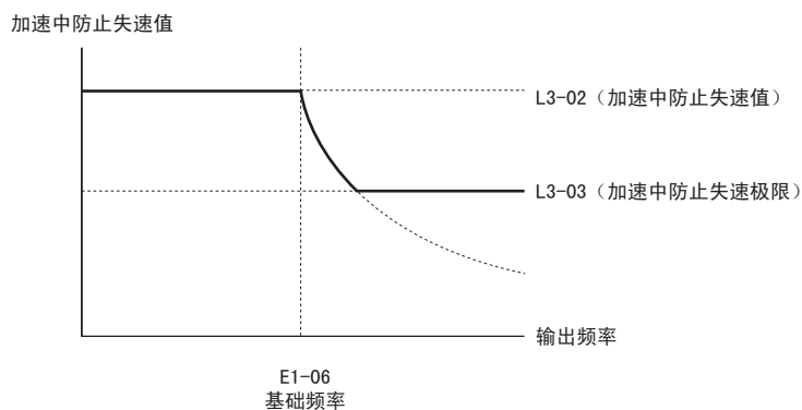
图 69 加速中防止失速值 / 极限
