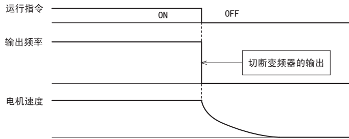
图 48 自由运行停止
