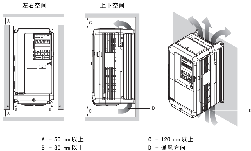
图 3 变频器的安装空间（单机）
