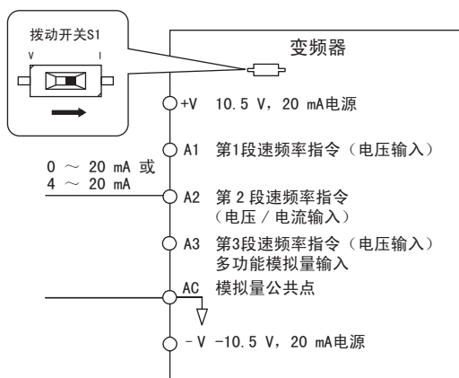
图 44 端子 A2 的电流输入设定
