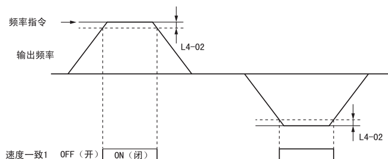
图 62 速度一致 1 的时序图
