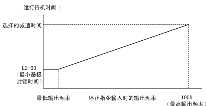
图 52 运行等待时间与输出频率的关系
