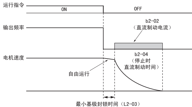
图 49 全域直流制动（DB）停止
