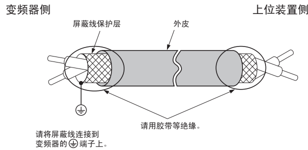
图 30 屏蔽线的线头处理
