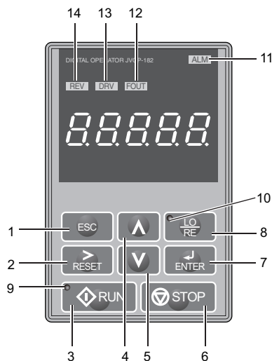
图 37 操作器各部分的名称与功能
