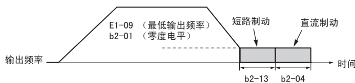
图 54 停止时短路制动（无 PG：PM 电机）
