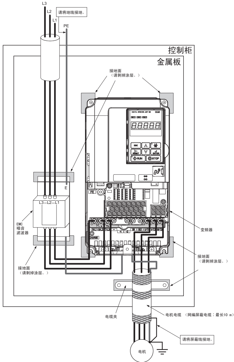
图 83 EMC 噪音滤波器和变频器的安装方法 (三相 200 V/400 V 级)
