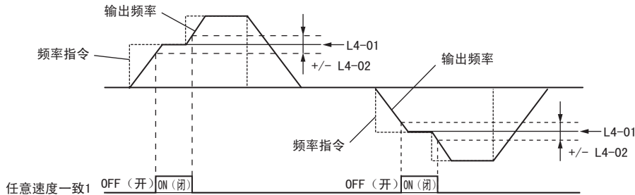
图 63 任意速度一致 1 的时序图
