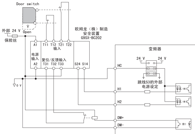
图 94 安全功能的连接示例
