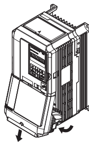
图 12 端子外罩的拆卸方法 (封闭壁挂型)
