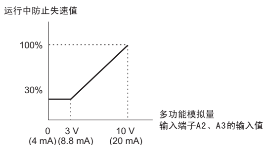
图 71 通过模拟量输入设定运行时防止失速值
