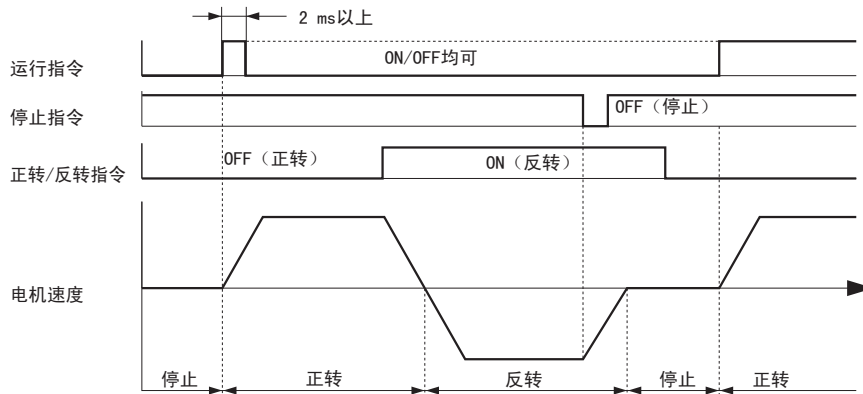
图 61 3 线制顺控的时序图
