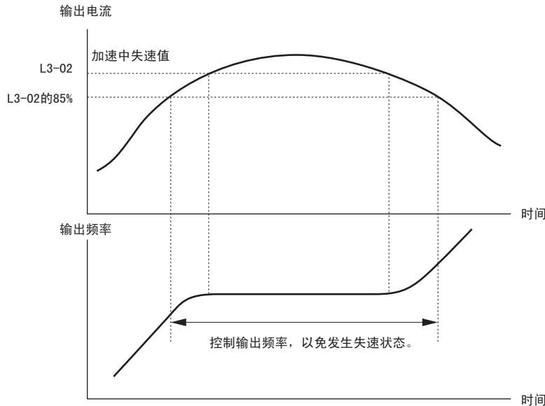
图 67 使用 IM 电机时的加速中防止失速功能
