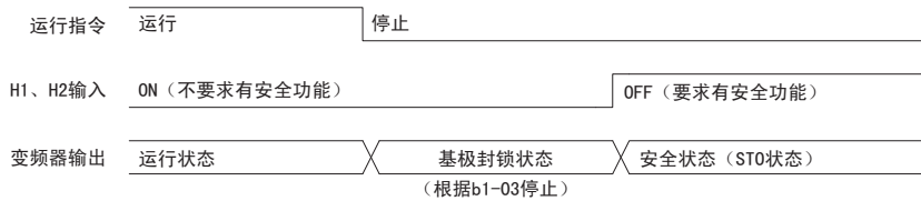
图 88 安全功能动作时的变频器状态
