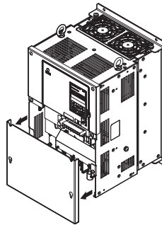
图 15 端子外罩的拆卸方法（柜内安装型）
