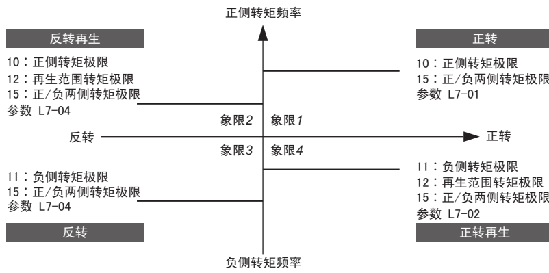
图 72 模拟量输入的转矩极限
