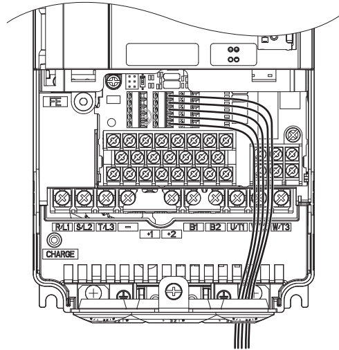
图 29 控制回路的接线 (TB4、TB5、TB6)
