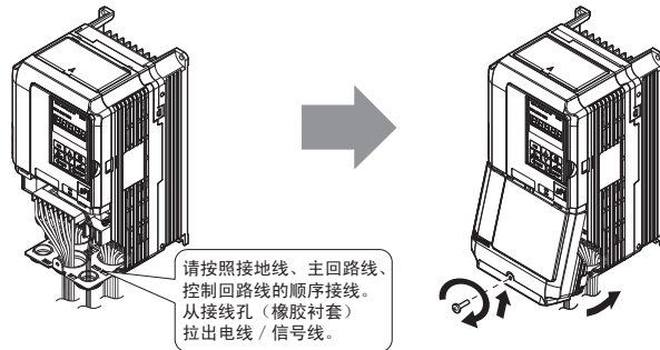
图 13 端子外罩的安装方法（封闭壁挂型）
