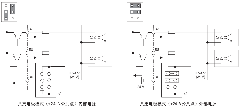
图 33 共集电极模式（+24 V 公共点）
