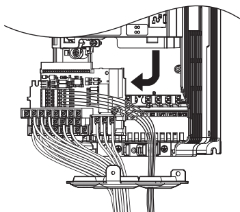
图 76 变频器的更换 (端子排的拆卸)
