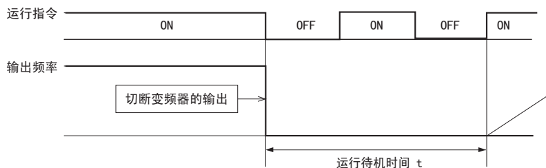
图 51 带定时的自由运行停止
