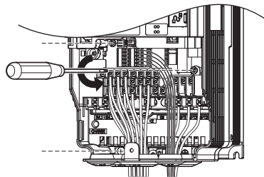
图 75 变频器的更换 (拧松固定螺丝)
