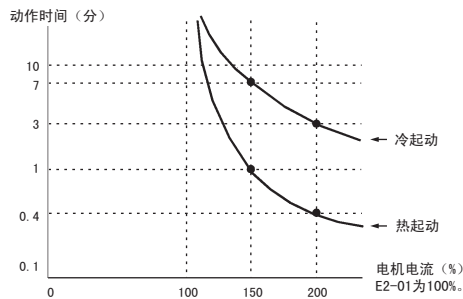
图 86 由输出频率和负载决定的电机过载保护时间
