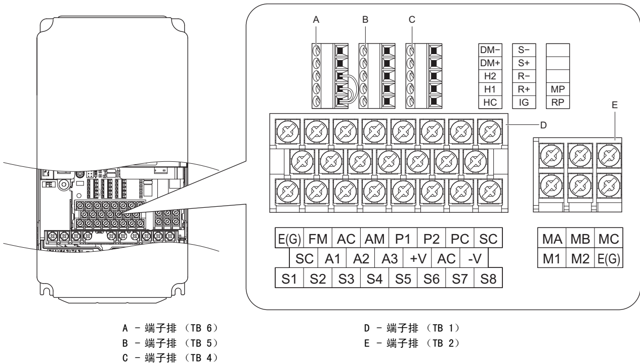
图 25 带参数备份功能的拆装式端子排的排列 (CIMR-AB□□□□□□□□)
