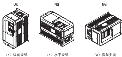
图 2 安装方向
