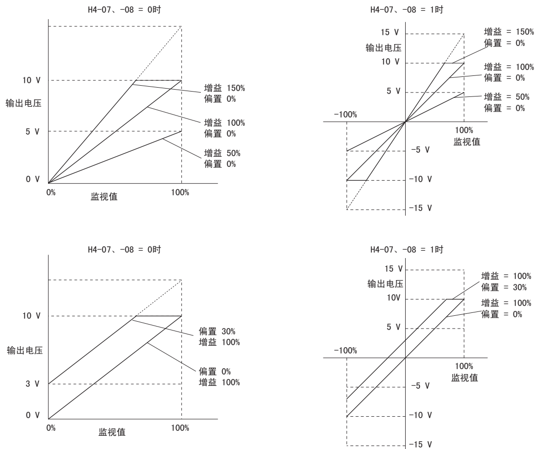
图 66 模拟量输出的增益 / 偏置设定
