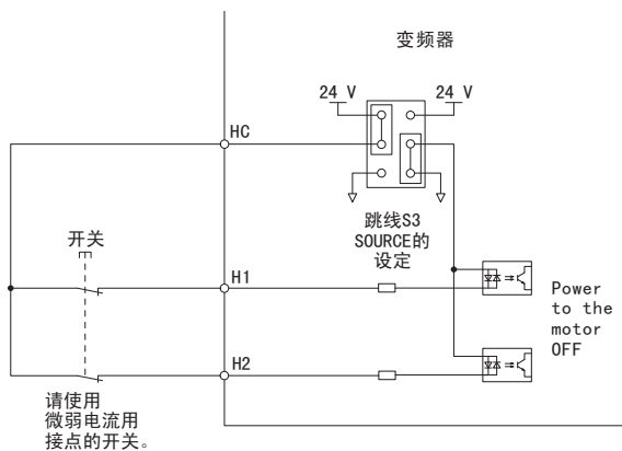
图 92 安全输入的连接示例 (双工化)
