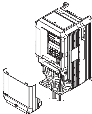
图 74 变频器的更换 (端子外罩的拆卸)
