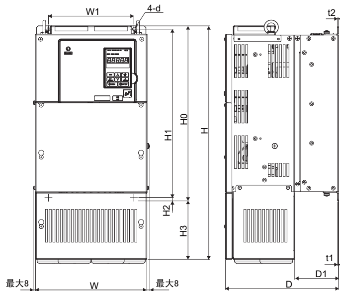
外形图 3
