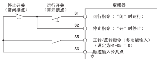
图 7 3 线制顺控的接线示例
