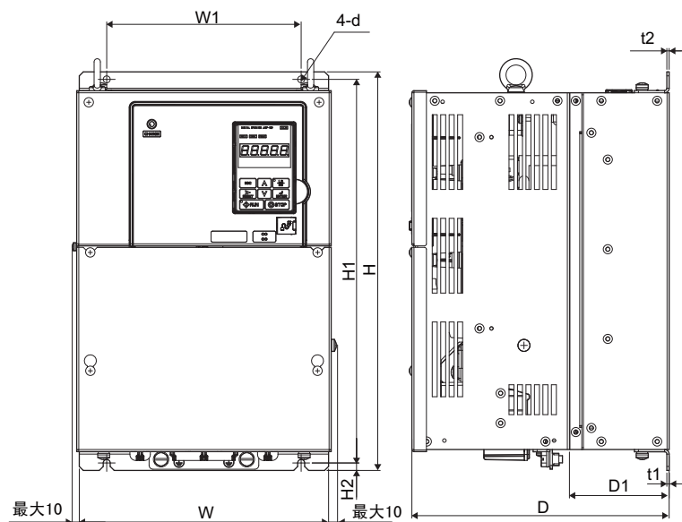
外形图 3
