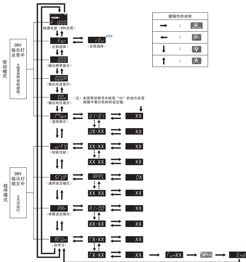
图 38 操作器显示功能的层次结构
