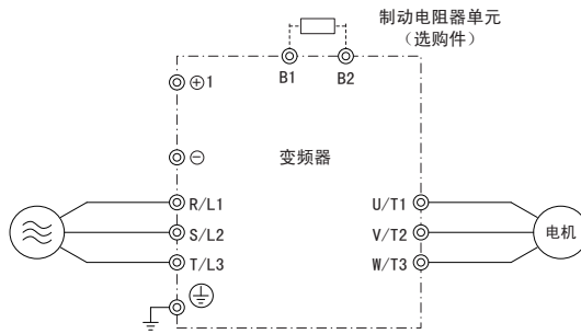
图 9 主回路端子的连接
