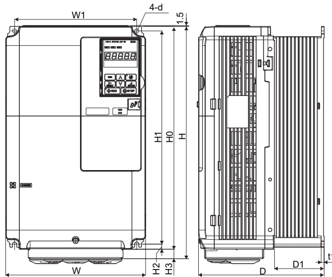
外形图 2
