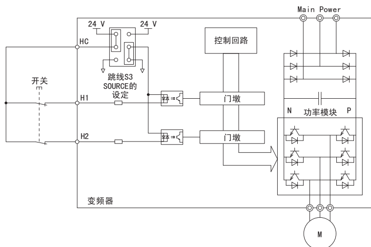
图 87 安全输入的接线示例（SOURCE 模式）
