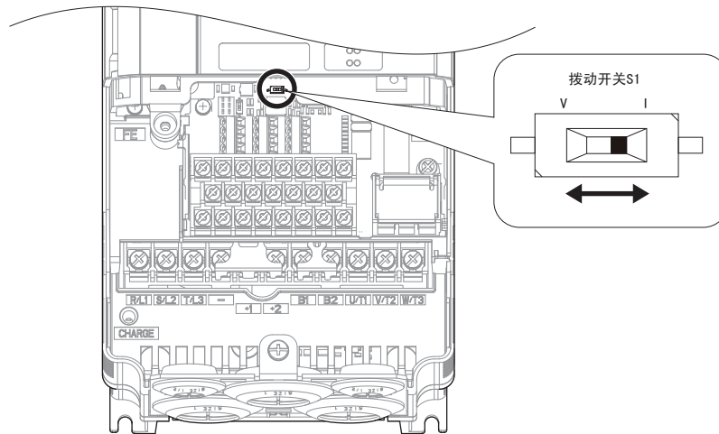
图 35 拨动开关 S1
