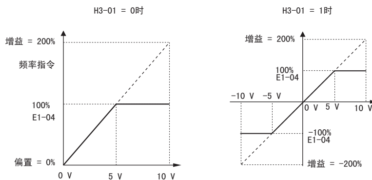
图 64 调整了模拟量输入的增益设定时的频率指令
