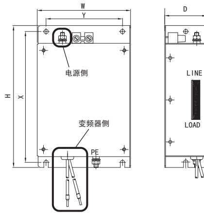
图 84 EMC 噪音滤波器的外形尺寸
