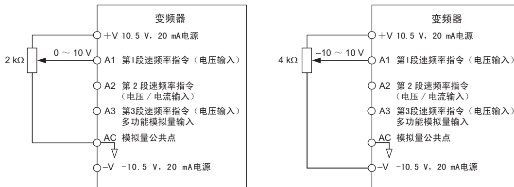
图 43 端子 A1 的电压输入设定示例
