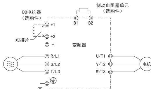
图 8 主回路端子的连接
