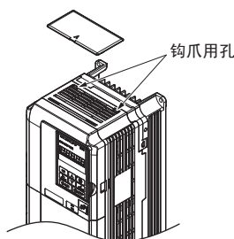
图 21 上部保护罩的安装
