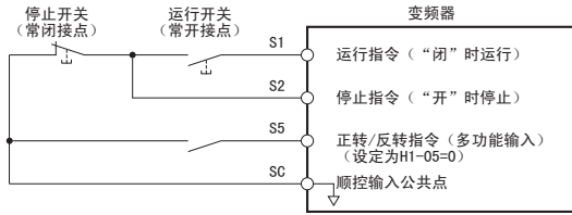
图 60 3 线制顺控的接线示例
