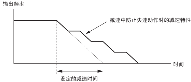
图 70 减速中防止失速的动作示例
