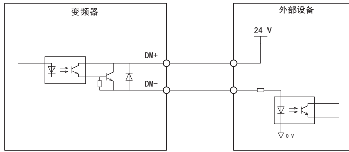
图 93 安全监视输出的连接示例
