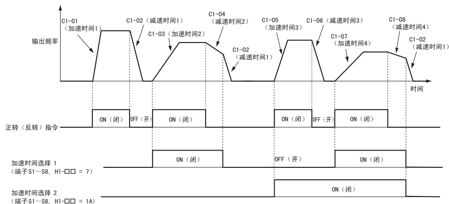
图 56 加减速时间的时序图
