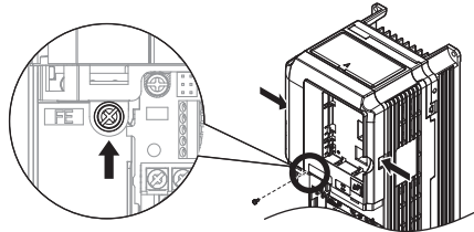
图 19 前外罩的拆卸
