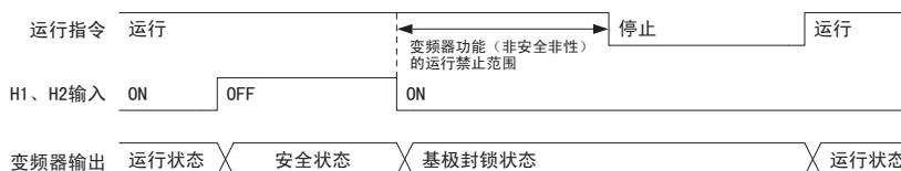
图 91 从安全状态 (ST0 状态) 返回 (在运行过程中 H1、H2 输入变为 OFF 而进入安全状态时)
