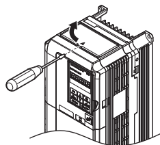
图 20 上部保护罩的拆卸
