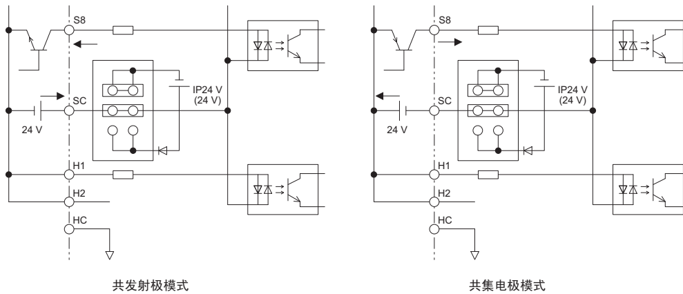
图 34 不使用安全输入时的接线示例
