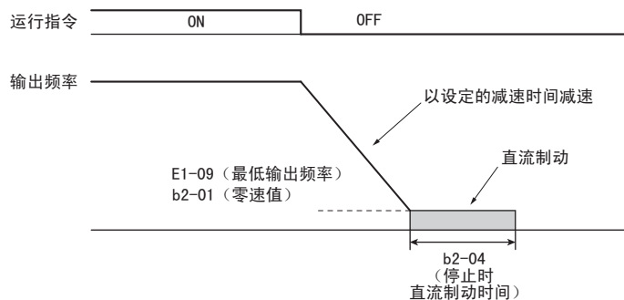
图 45 减速停止（无 PG V/f 控制、带 PG V/f 控制、无 PG 矢量控制模式时）
