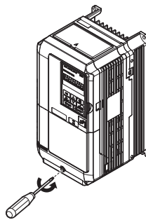
图 11 端子外罩的拆卸方法 (封闭壁挂型)
