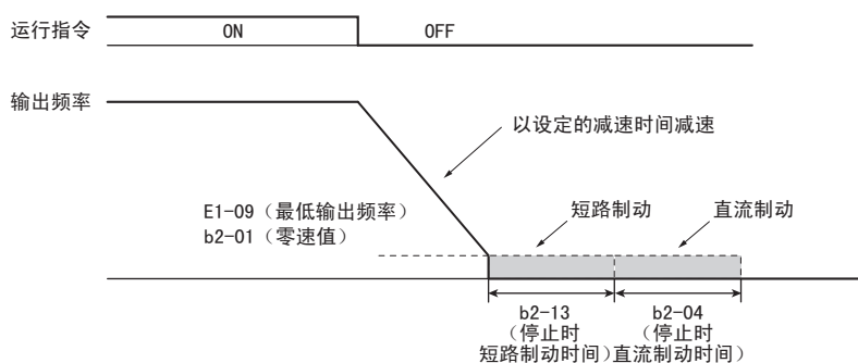
图 46 减速停止（PM 用无 PG 矢量控制、PM 用无 PG 高级矢量控制模式时）
