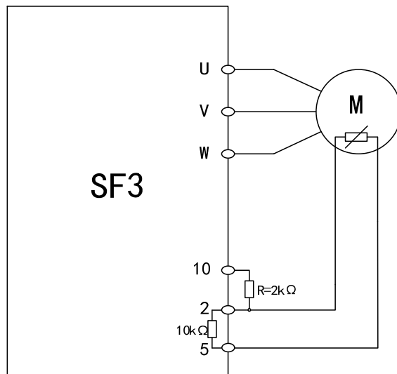
PTC電阻輸入接線圖
