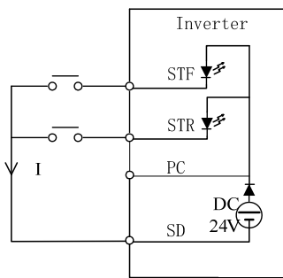
Sink Input: 多功能控制端子直接與SD相連接
