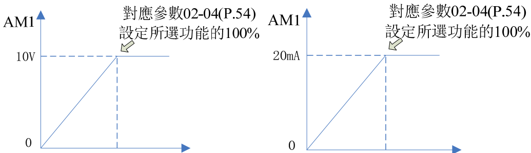
圖 1. AM1-5 輸出 0~10V 電壓 圖 2. AM1-5 輸出 0~20mA 電流
