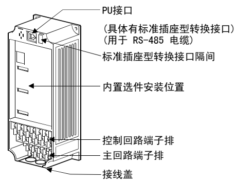
(2) 无前盖板
