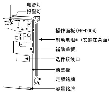
(1) 前视图
