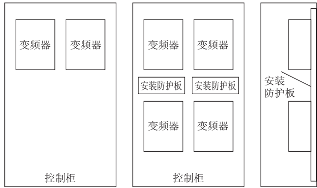
(a) 横向摆放时 (b) 纵向摆放时 安装多台变频器时
