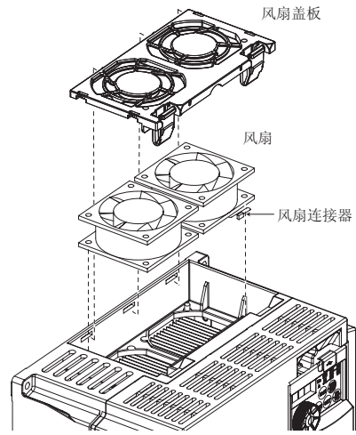
FR-E740-5.5K-CHT的示例
