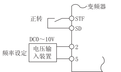
使用端子2（DC0~10V）接线的示例
