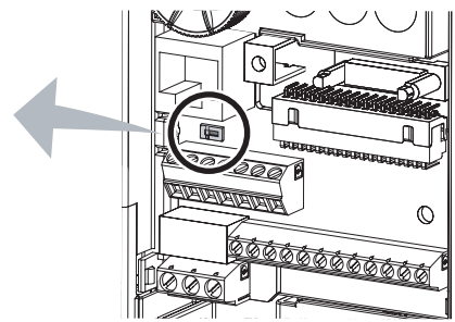
控制电路端子排
