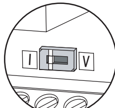
电流输入时（初始设定）
