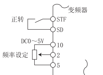
使用端子2（DC0~5V）接线的示例
