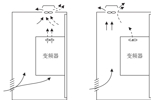
<好的例子> <坏的例子> 换气风扇和变频器的配置
