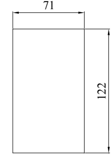
b) 键盘托架开孔尺寸图
