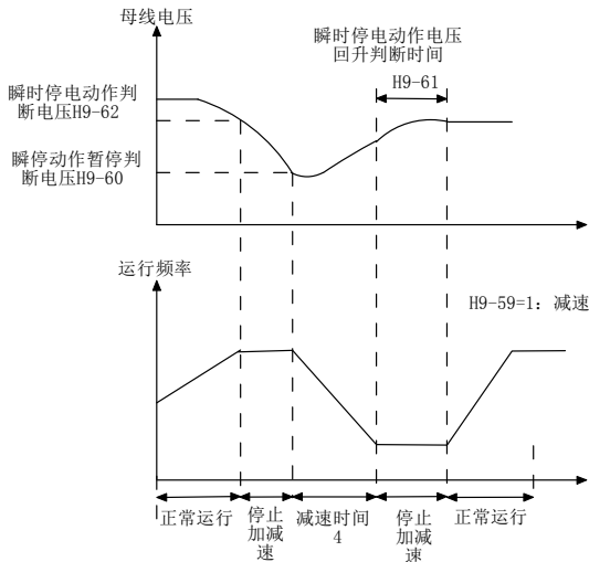
图 6-19 瞬停电动作示意
