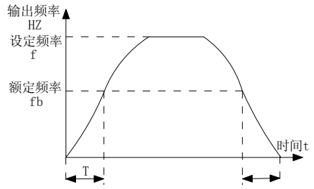
图 6-11 S 曲线加减速 B 示意图
