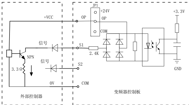
图 3-10 多台变频器 S 端子并接漏型接线方式
