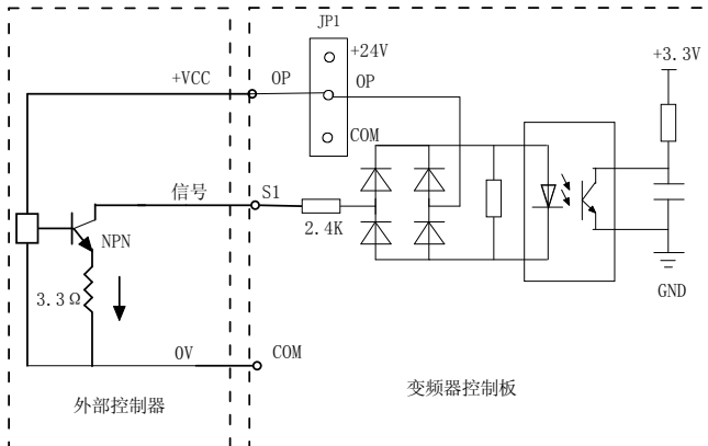
图 3-9 漏型接线方式
