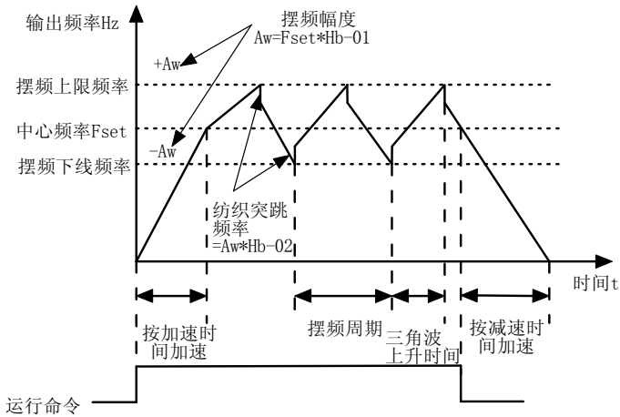
图 6-26 摆频工作示意
