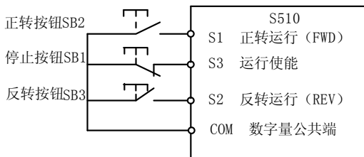
图 6-7 三线式控制模式 1
