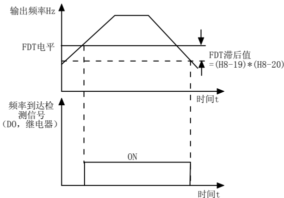
图 6-15 FDT 电平示意图
