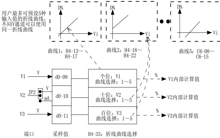
图4-29 V信号对应实际给定
