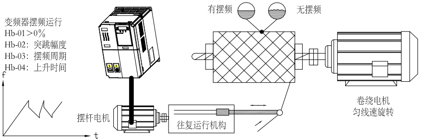
图4-22 摆频工作模式
