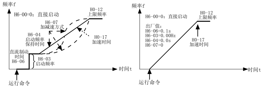
图4-7 直接启动方式
