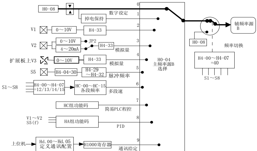
图4-16 辅助频率给定来源选择
