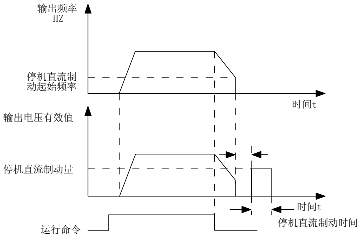
图 6-12 停机直流制动示意图
