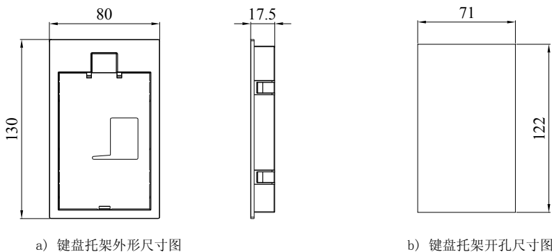
图 2-7 键盘托架外形尺寸及开孔尺寸图
