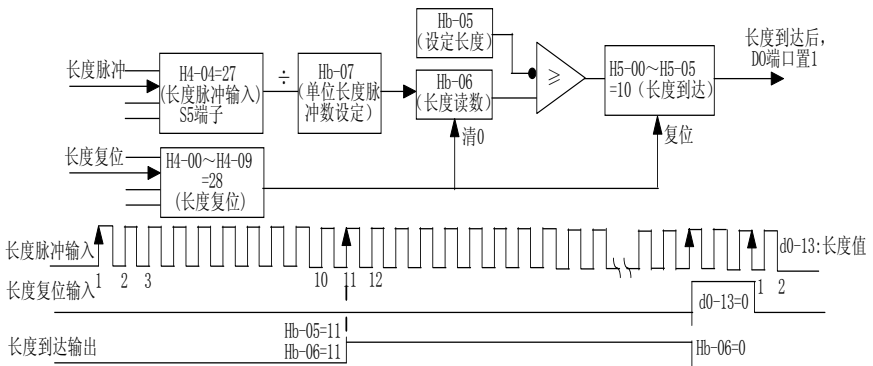
图4-25定长控制模式功能码设置
