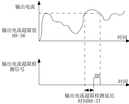
图 6-21 输出电流超限检测示意
