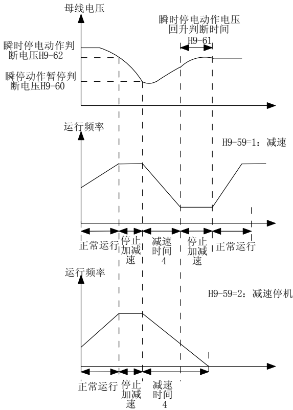
图 6-24 瞬时停电动作示意图
