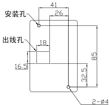
图 2-6 键盘背面固定开孔尺寸图
