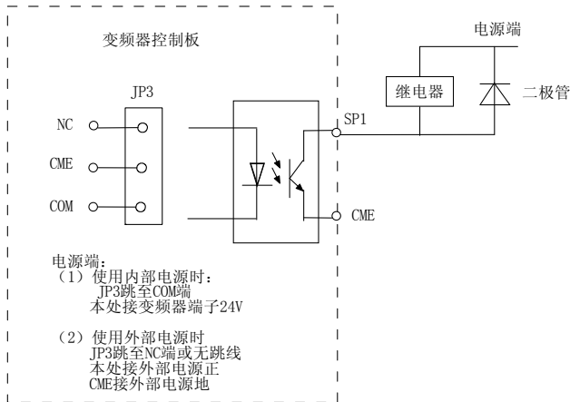
图 3-12 数字输出端子接线示意图
