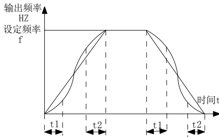
图 6-10 S 曲线加减速 A 示意图
