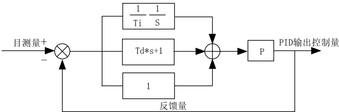
图 6-25 过程 PID 原理框图
