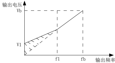
图 6-3 手动转矩提升示意图
