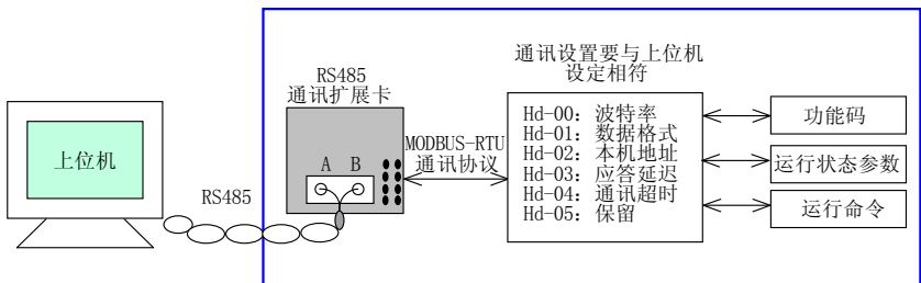
图 4-30 变频器串行通讯的使用
