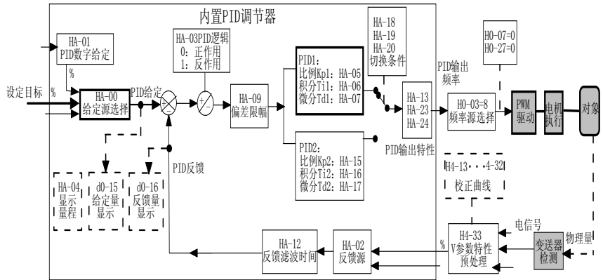
图4-21 过程控制的频率闭环控制
