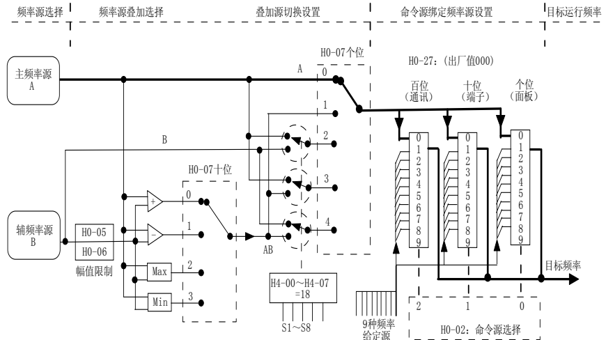
图 4-17 主辅助频率混合给定来源选择
