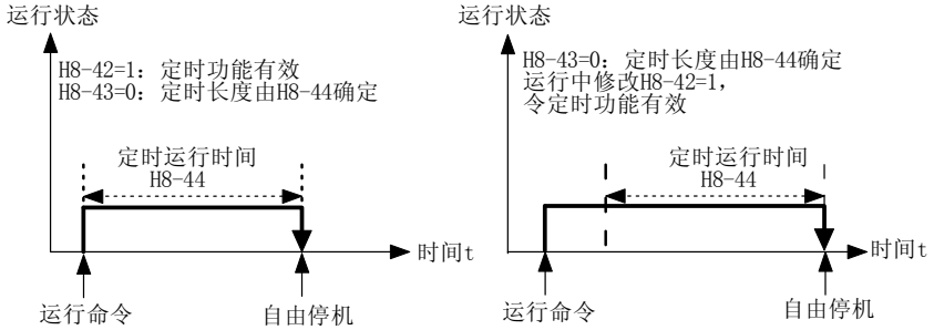
图4-11 定时停机功能
