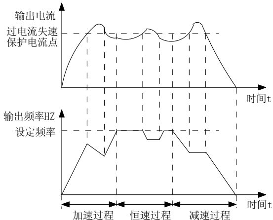
图 6-23 过流失速保护示意图
