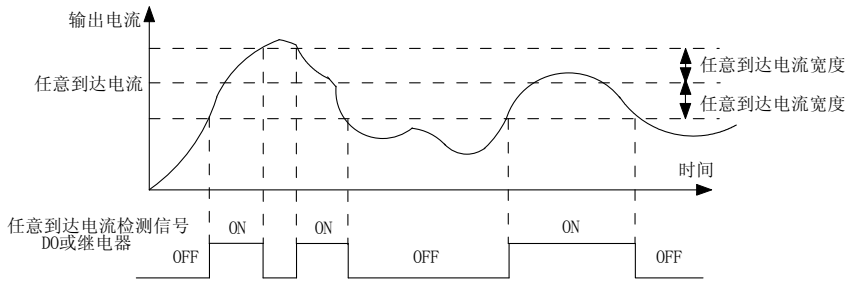
图 6-22 任意到达电流检测示意图
