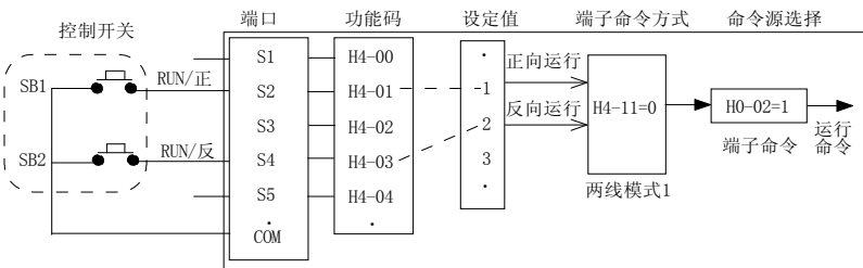
图 4-4 端子启停控制方式举例
