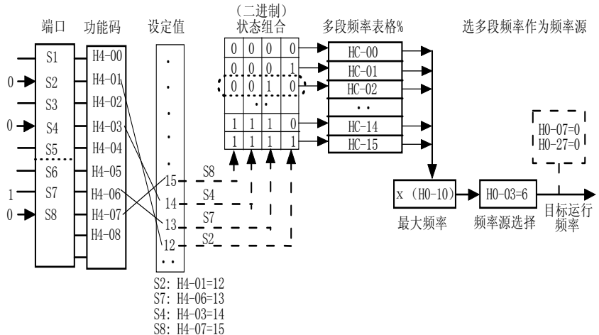
图4-23 多段速模式的设置
