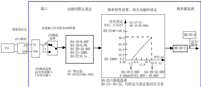
图4-19 V2电流型输入给定频率功能码设置
