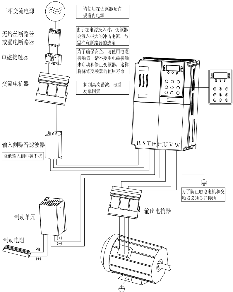
图 2-10 变频器系统构成图
