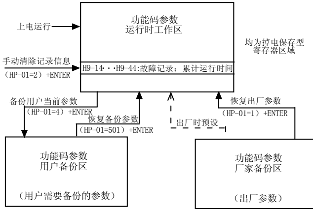
图 4-31 参数备份与恢复设置
