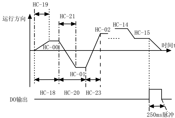
图 6-28 简易 PLC 示意图
