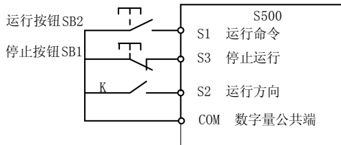
图 6-8 三线式控制模式 2
