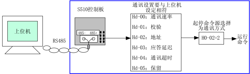
图4-6 通讯启停控制方式举例
