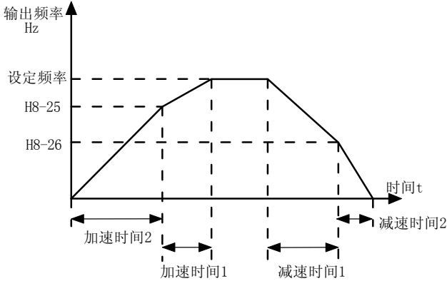
图 6-18 加减速时间切换示意图
