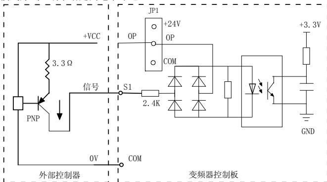
图 3-11 源型接线方式
