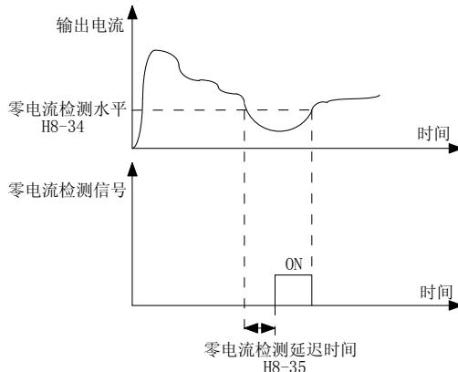
图 6-20 零电流检测示意图
