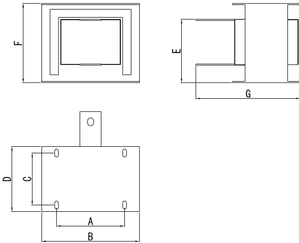
图 2-11 外置电抗器尺寸示意图
