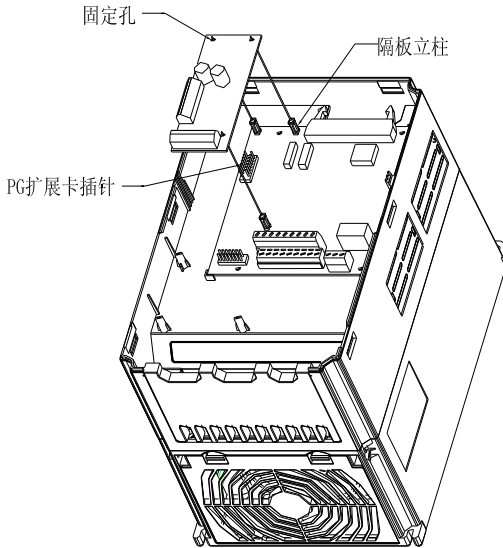
附录 D: 图 1 PG 卡 1 JP-PG2-0C 安装方式
