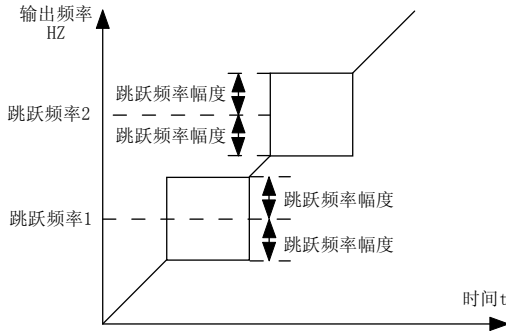
图 6-13 跳跃频率示意图
