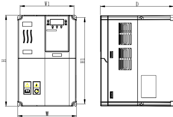
图 2-3 S510 系列 0.4~15KW 壁挂式塑料结构外形及尺寸示意图
