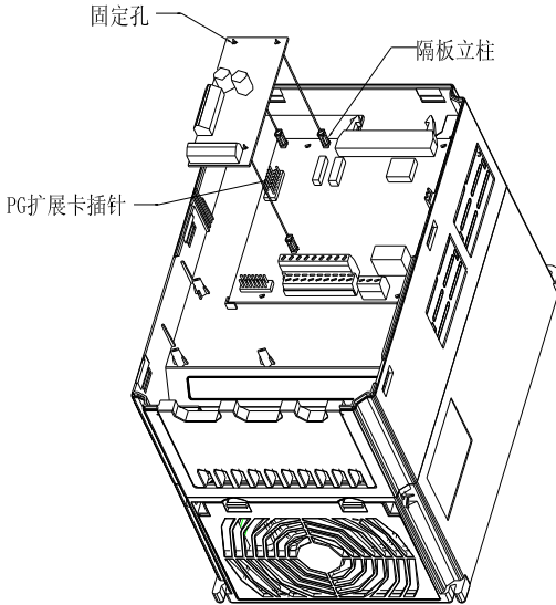
附录 C：图 1 PG 卡 1 JP-PG1-DIFF 安装方式
