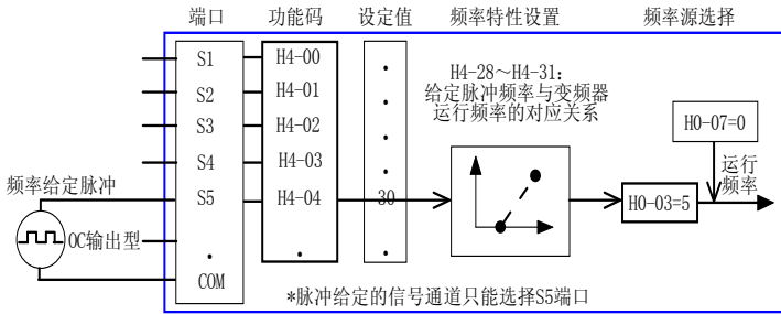
图4-20 脉冲给定频率功能码设置
