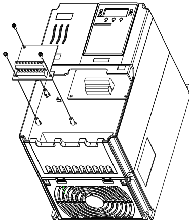
附录 B：图 1 扩展卡 JP-EXT2-IO 安装方式
