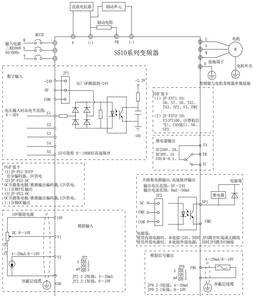
图 3-5 变频器接线示意图
