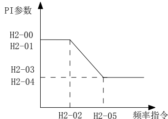
图 6-2 PI 参数示意图
