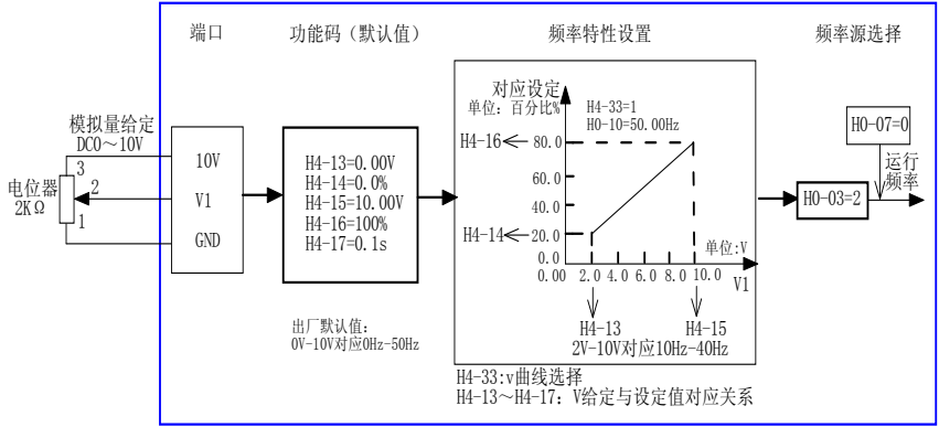
图 4-18 V1 电压型输入给定频率功能码设置
