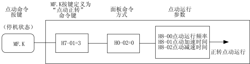
图4-13 操作面板点动运行
