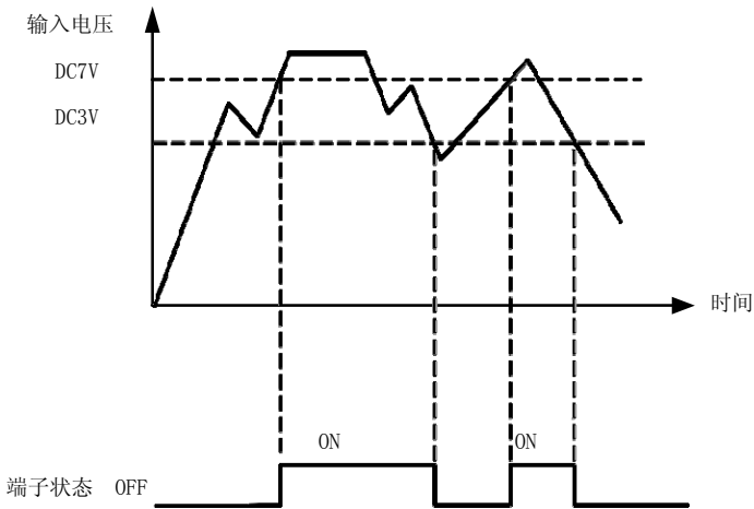
图 6-29 模拟输入作为数字量端子有效状态判断
