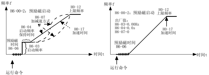
图4-9 启动过程频率曲线
