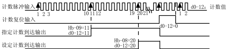
图 6-27 设定计数值给定和指定计数值给定示意图
