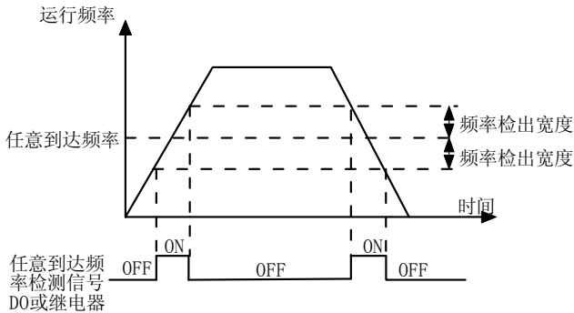
图 6-19 任意到达频率检测示意图
