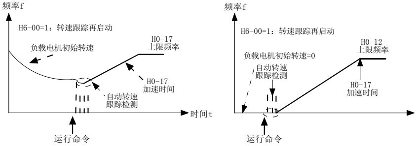
图4-8 速度跟踪再启动方式
