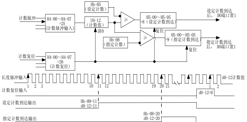
图4-27 计数模式功能码设置
