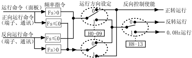
图4-24 电机运转方向设置
