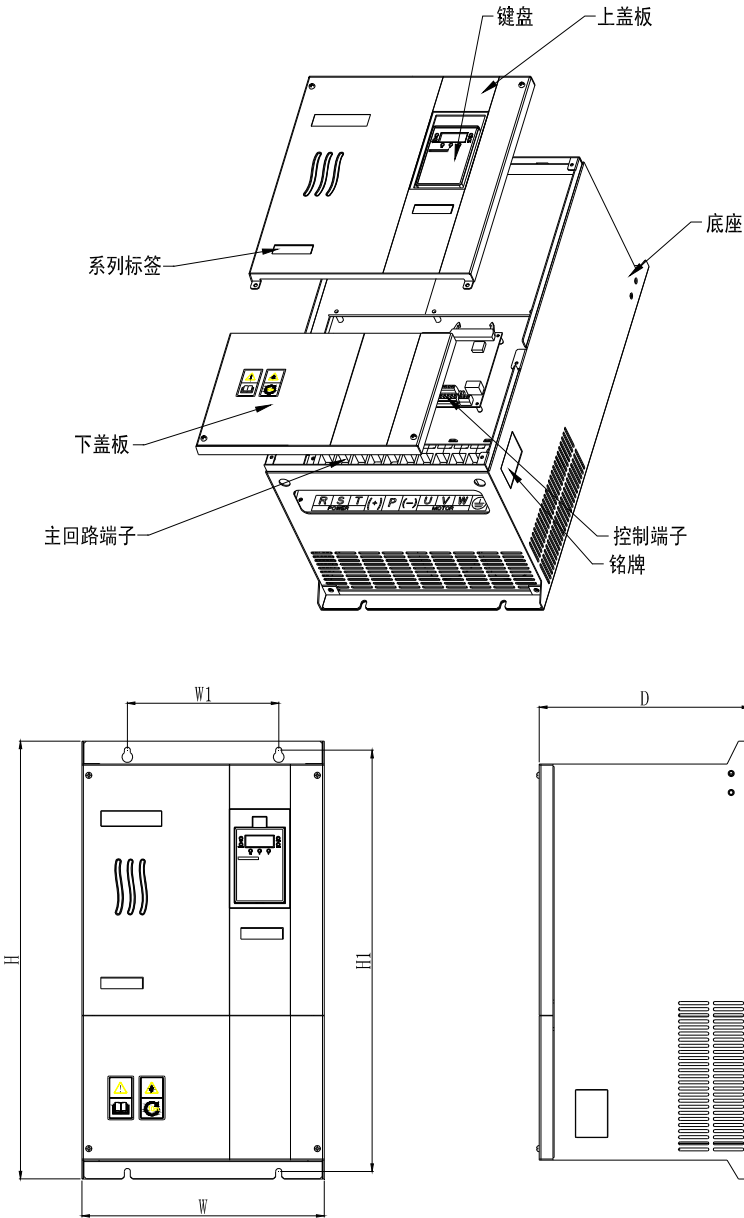
图 2-4 S510 系列 18.5~400KW 钣金结构外形及尺寸示意图
