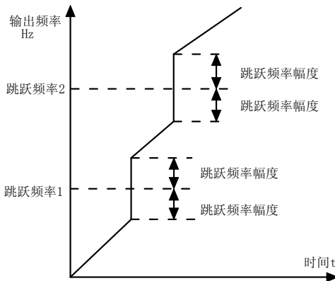
图 6-17 加减速过程中跳跃频率有效示意图
