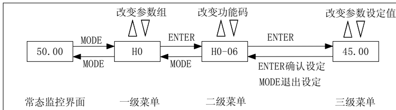
图 4-3 三级菜单操作流程图
