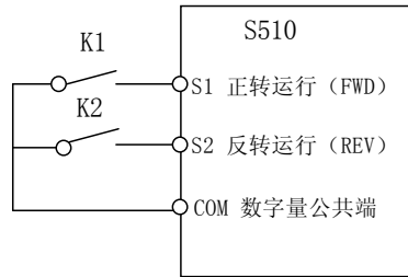
图 6-5 两线式模式 1
