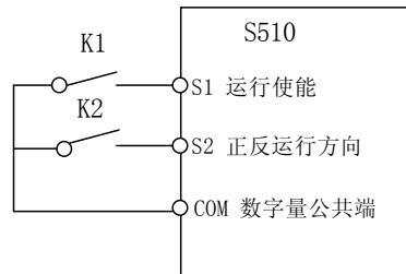
图 6-6 两线式模式 2
