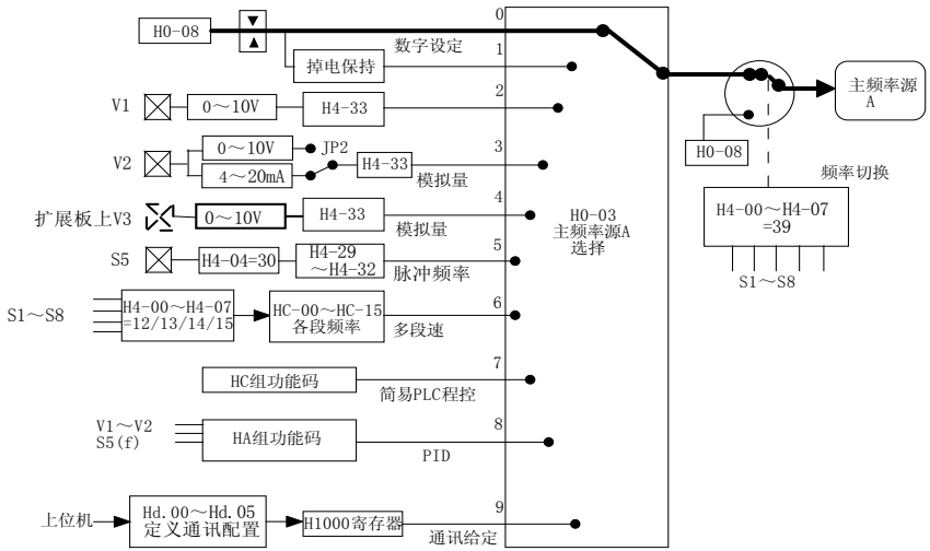
图4-15 主频率给定来源选择
