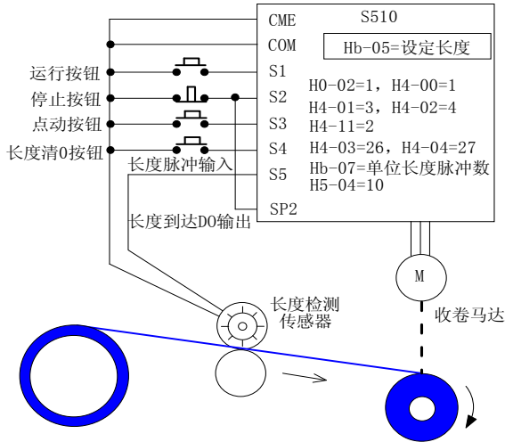
图4-26 定长控制功能常见应用举例
