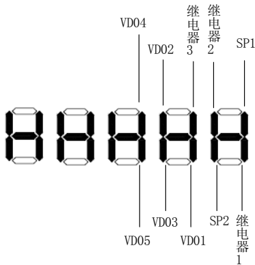
图 6-31 输出端子有效输出示意图
