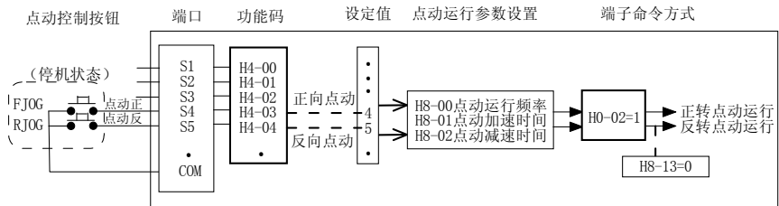
图4-14 S输入端子点动运行
