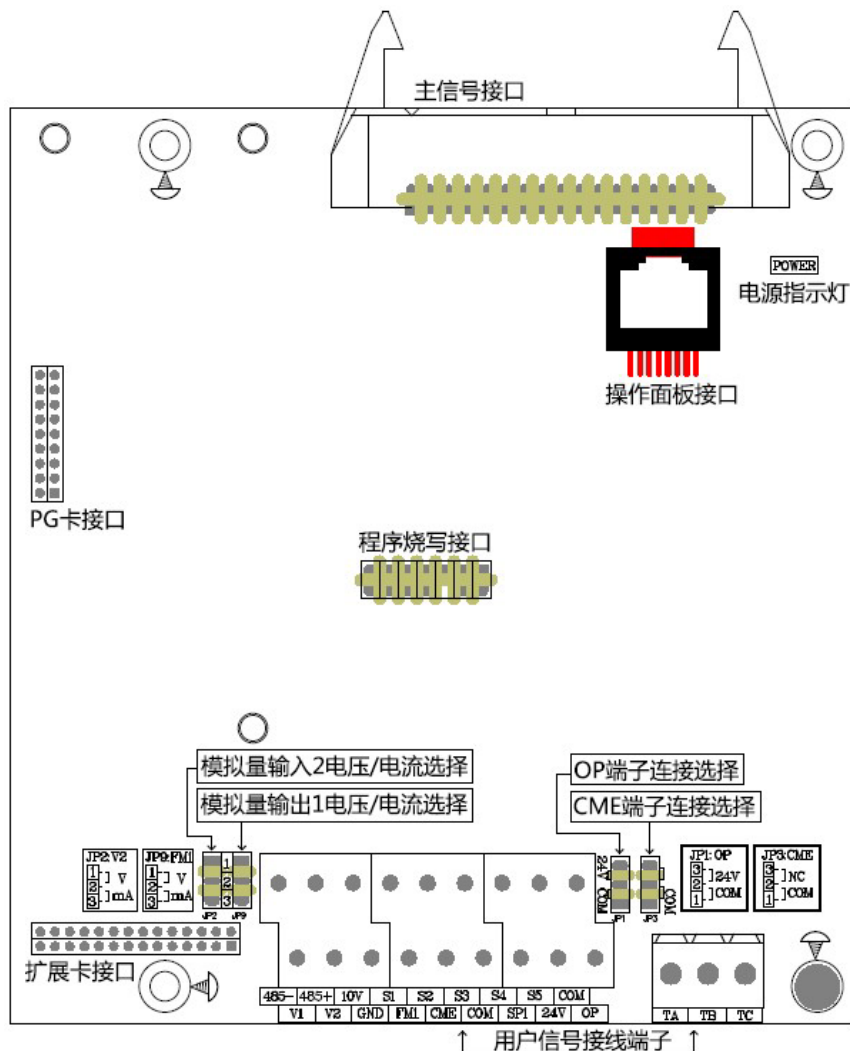
图 3-4 控制板布局图
