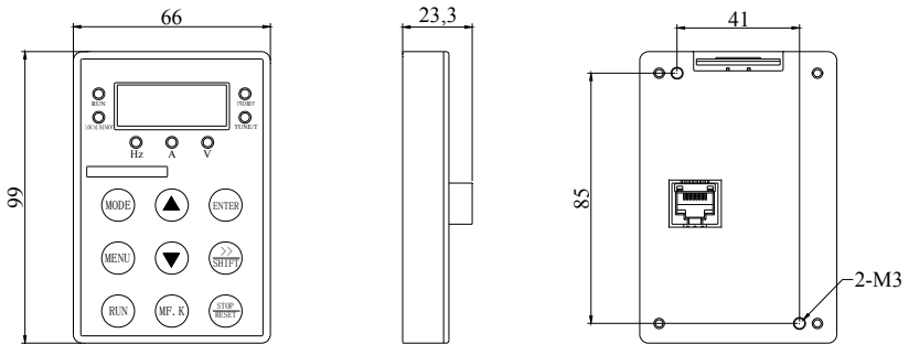
图 2-5 外引键盘外形尺寸
