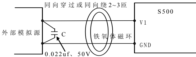
图 3-7 模拟量输入端子接线示意图
