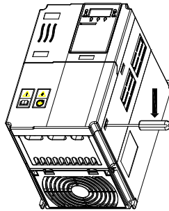
图 3-2 塑胶外壳下面板拆卸图
