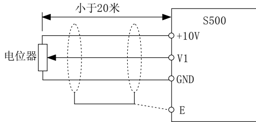
图 3-7 模拟量输入端子接线示意图
