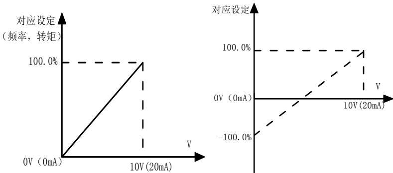
图 6-9 模拟给定与设定量的对应关系
