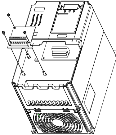
附录 A：图 1 扩展卡 JP-EXT1-I/O 安装方式
