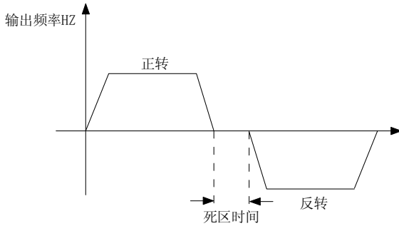
图 6-14 正反转死区时间示意图
