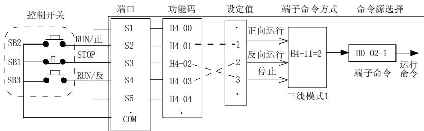
图 4-5 端子启停控制方式举例
