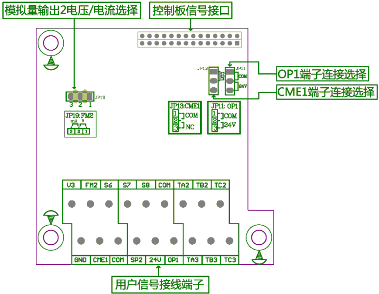
附录 A：图 2 扩展卡 JP-EXT1-IO 布局图
