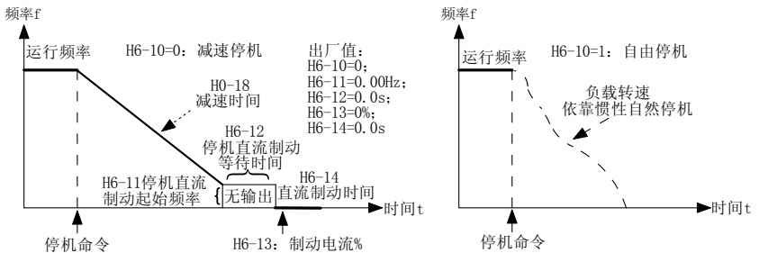
图 4-10 停机模式
