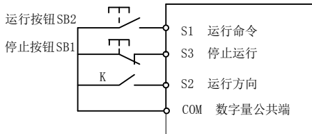
图 6-8 三线式控制模式 2
