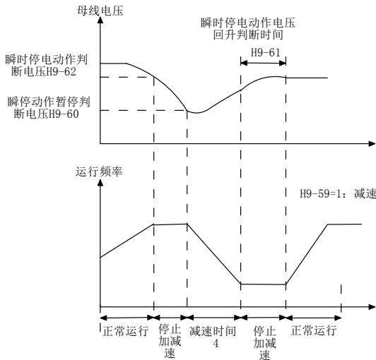
图 6-19 瞬时停电动作示意
