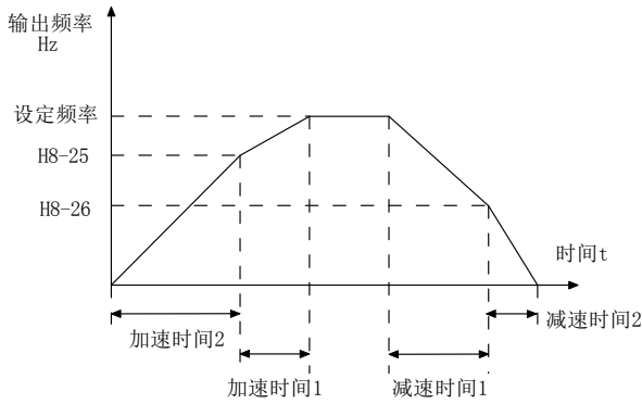
图 6-16 加减速时间切换示意图
