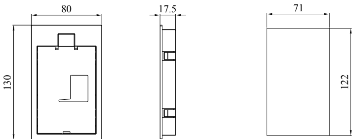
键盘托架外形尺寸图
