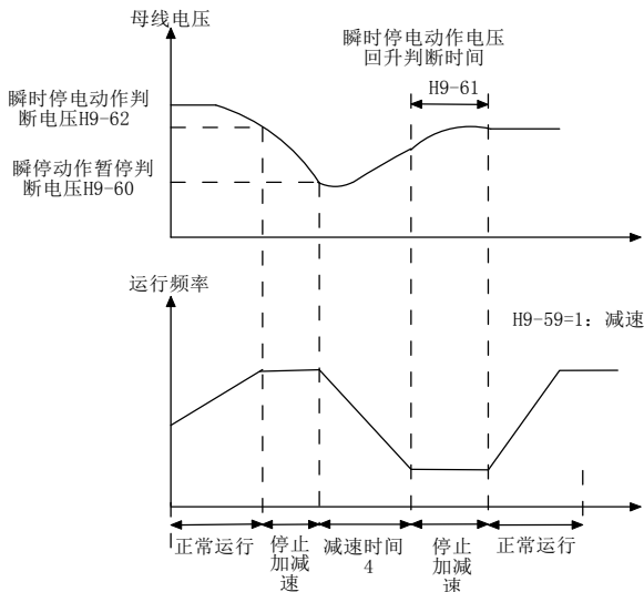
图 6-21 瞬时停电动作示意图
