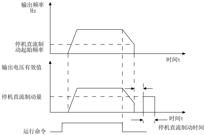
图 6-8 停机直流制动示意图
