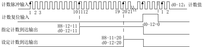
6-12 设定计数值给定和指定计数值给定示意图
