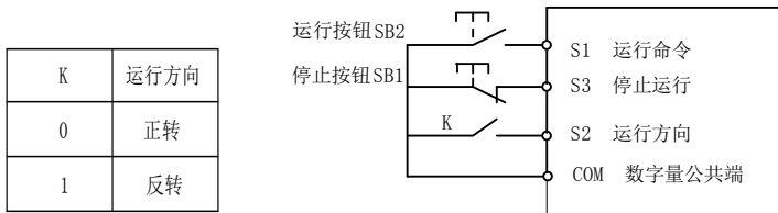
图 6-6 三线式控制模式 2
