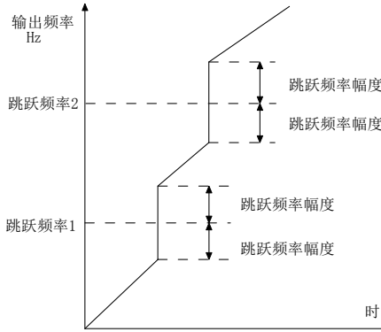
图 6-15 加减速过程中跳跃频率有效示意图
