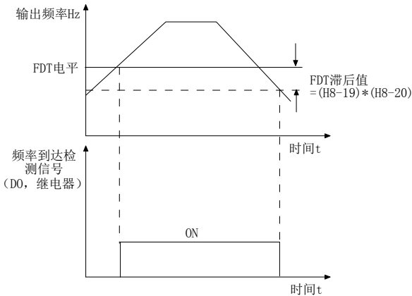
图 6-13 频率 FDT 示意图
