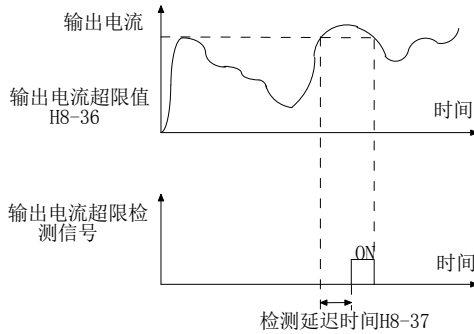
图 6-18 输出电流超限检测示意
