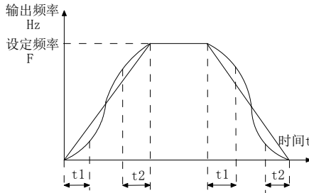
图 6-7 S 曲线加减速示意图
