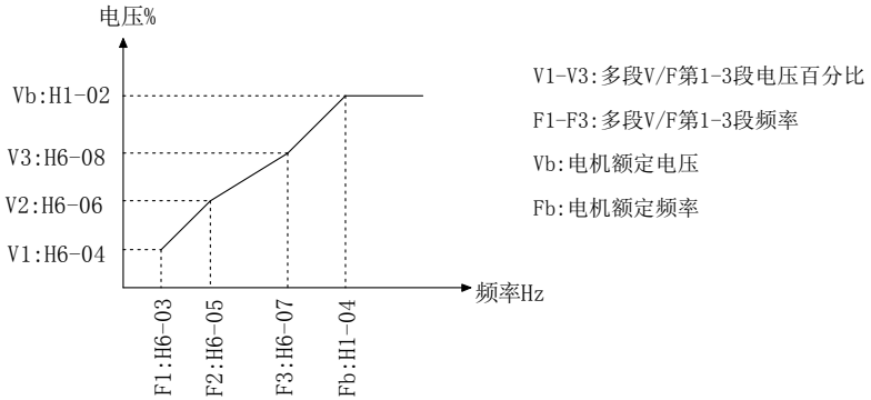
图 6-10 多点 V/F 曲线设定示意图
