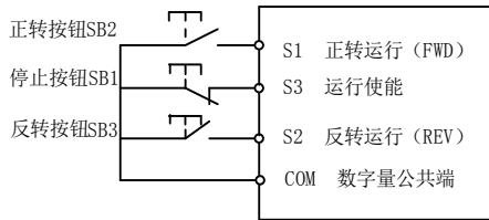
图 6-5 三线式控制模式 1
