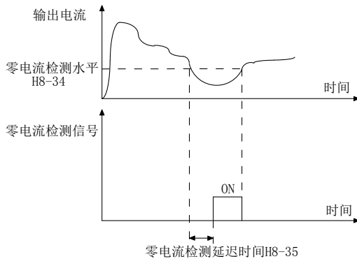
图 6-17 零电流检测示意图
