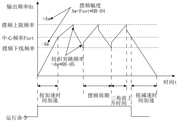
图 6-11 摆频运行示意图
