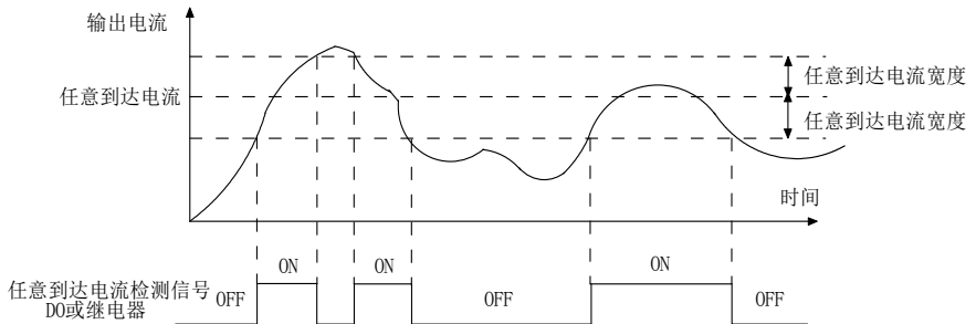
图 6-19 任意到达电流检测示意图
