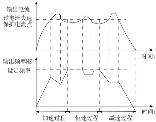
图 6-20 过流失速保护示意图
