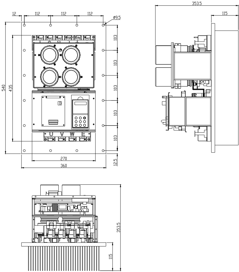
45~75KW 变频器外形图及外形尺寸示意图
