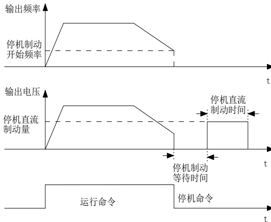
图6-1 减速停机制动示意图
