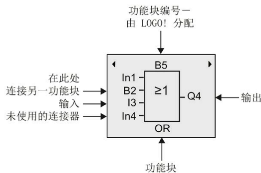
LOGO! 显示屏视图
