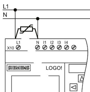
LOGO! ... AC 电源供电
