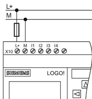
LOGO! ... DC 电源供电
