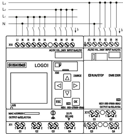
主机模块和扩展模块的三相连接
