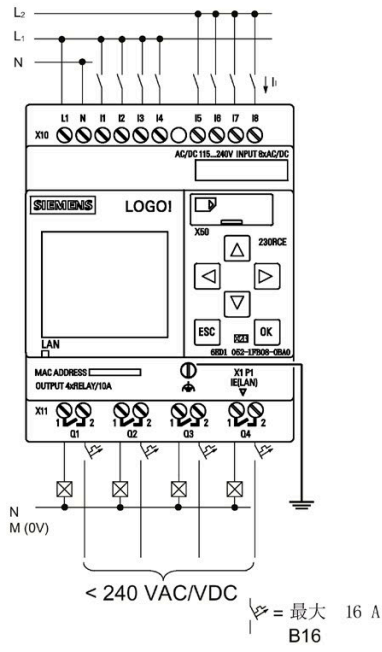
主机模块的两相连接
