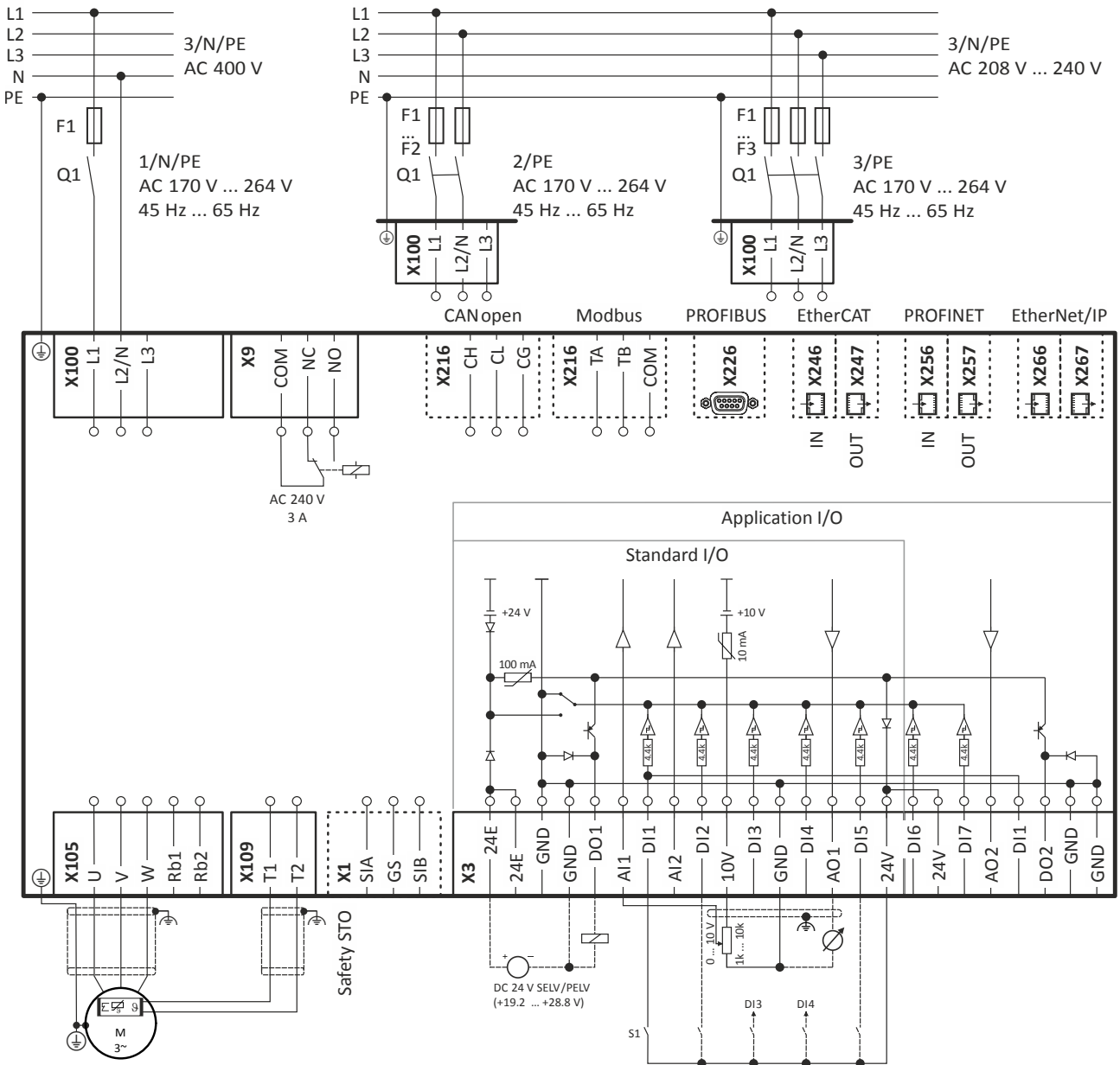
图 4: 接线示例
