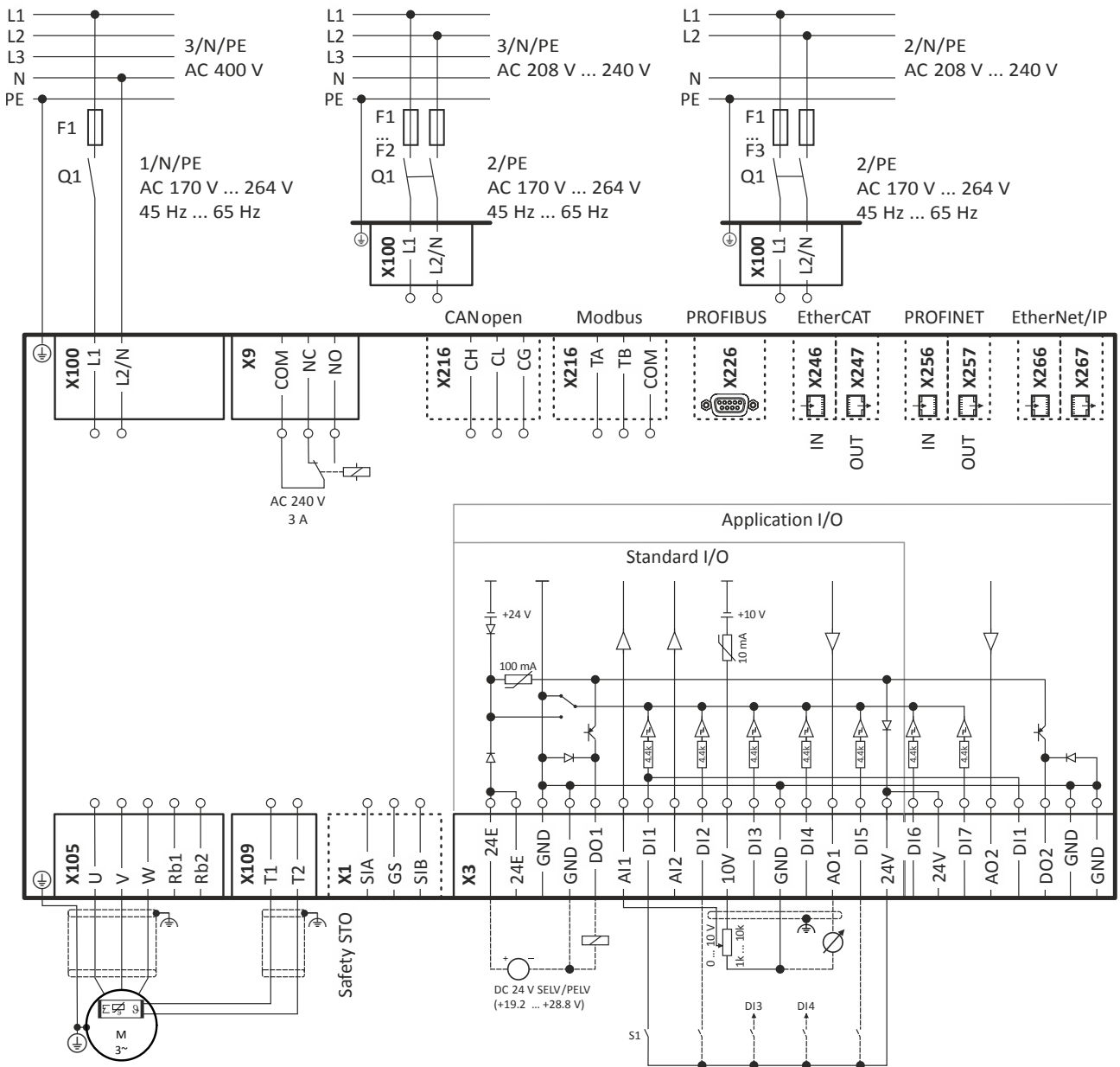
图 3: 接线示例
