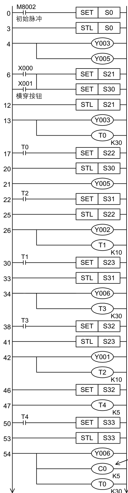
《步进梯形图》
