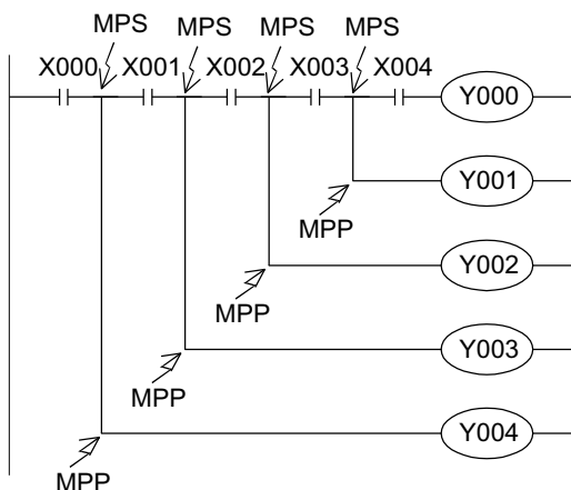
梯形图程序
