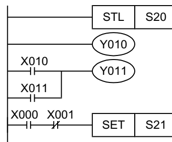
《步进梯形图》
