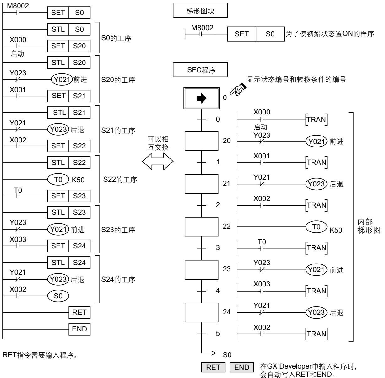
《SFC程序》
