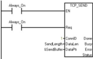
程序段 15：向被动设备发送新消息。设置 Req 为 TRUE 以初始化新的发送操作。
