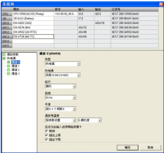
TC 模拟量扩展模块可测量连接到模块输入的电压值。
