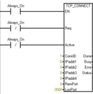
程序段 8： 如果 Done 为 TRUE ，则表示 CPU 已建立该连接，所以继续进入“空闲”状态。 如果 Busy 为 TRUE ，则 CPU 停留在“连接等待”状态。由于该连接为被动连接，所以停留在“忙碌”状态直到主动伙伴连接到该 CPU 。被动连接不会超时。 如果 Error 为 TRUE ，则表示出现问题，返回到上一个操作，并在下次扫描时再次尝试建立连接。
