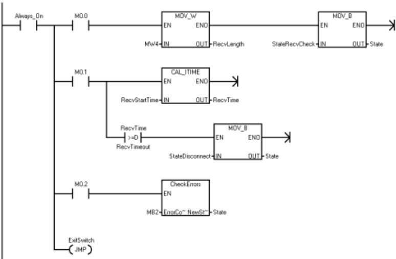
程序段 25：状态“RecvCheck”...
