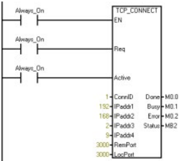
程序段 5: 如果 Done 为 TRUE，则 CPU 建立该连接以进入“空闲”状态。 如果 Busy 为 TRUE，则 CPU 进入“连接等待”状态以等待连接的建立。 如果 Error 为 TRUE，则可能输入参数有误，检查输入参数以决定 CPU 接下来要进入哪个状态。
