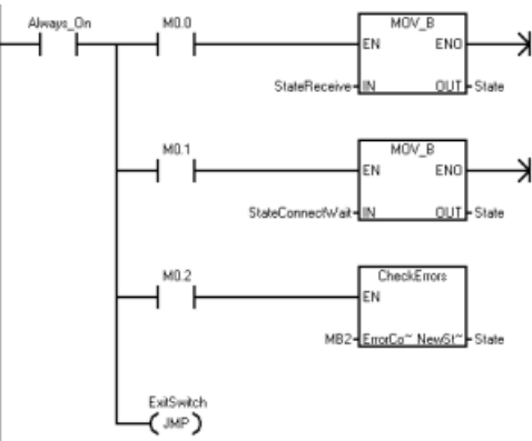
程序段 6： 状态“连接等待”... 在该状态等待直到主动伙伴与该 CPU 创建连接。
