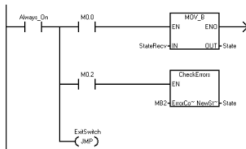
程序段 20: 状态“接收”...
