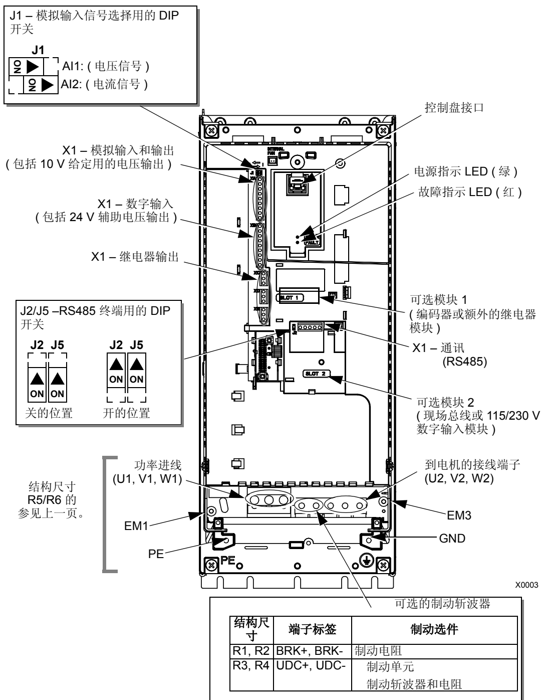
上图 R3 结构尺寸的模块。其它结构尺寸的布置也都是相近的。
