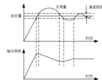
图6-25 偏差极限与输出频率的对应关系
