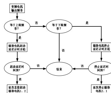
图6-23 简易供水功能逻辑示意图
