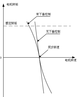
图6-22 下垂控制电机特性示意图
