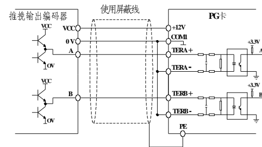
图 7-11 推挽式输出编码器接线图
