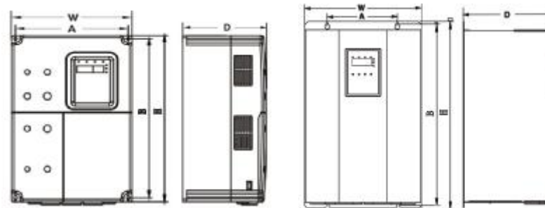
图 1-5 15kW 及以下机型的外形尺寸(380V)
