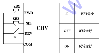
图6-12 三线式控制模式1
