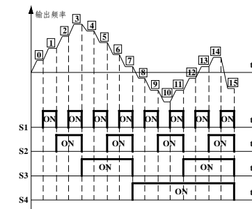
图6-27 多段速度运行逻辑图
