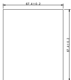
图 3-5 外引键盘(小)的开孔尺寸
