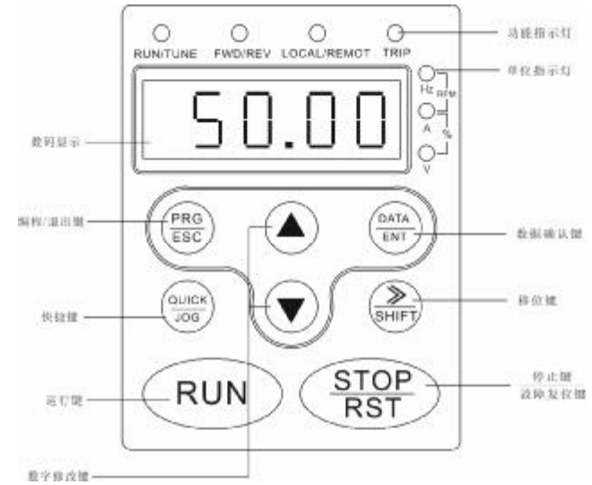
图 5-1 操作面板示意图
