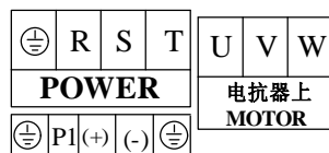
图 4-6 主回路接线端子图(350~630kW)
