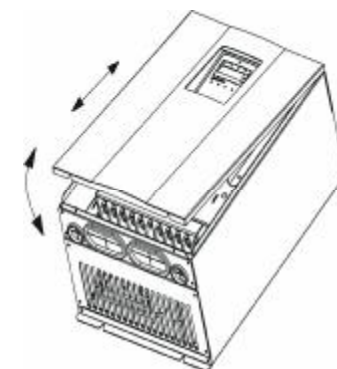
图 3-9 钣金盖板的拆卸和安装示意图
