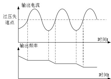
图6-30 过压失速功能
