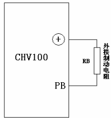
图 1-12 制动电阻的安装
