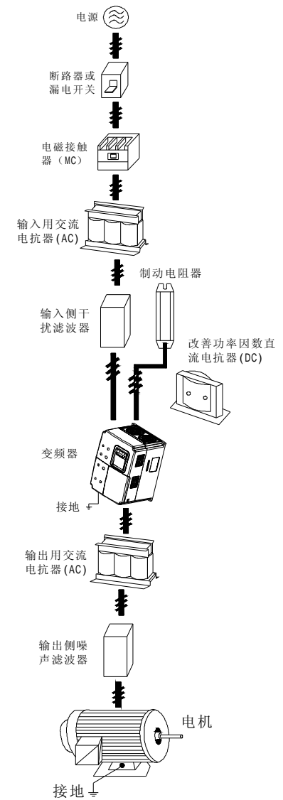
图 4-1 外围设备的连接图
