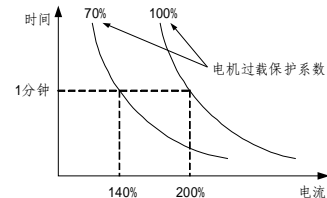
图6-28 电机过载保护系数设定
