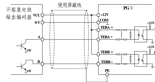
图 10-12 集电极开路输出编码器接线图
