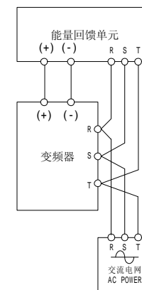
图 4-15 能量回馈单元连接图
