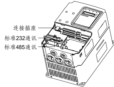
图 10-2 通讯卡安装示意图
