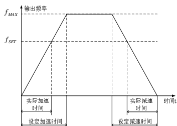
图6-1 加减速时间示意图
