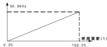
图6-16 给定量与高速脉冲输出对应关系
