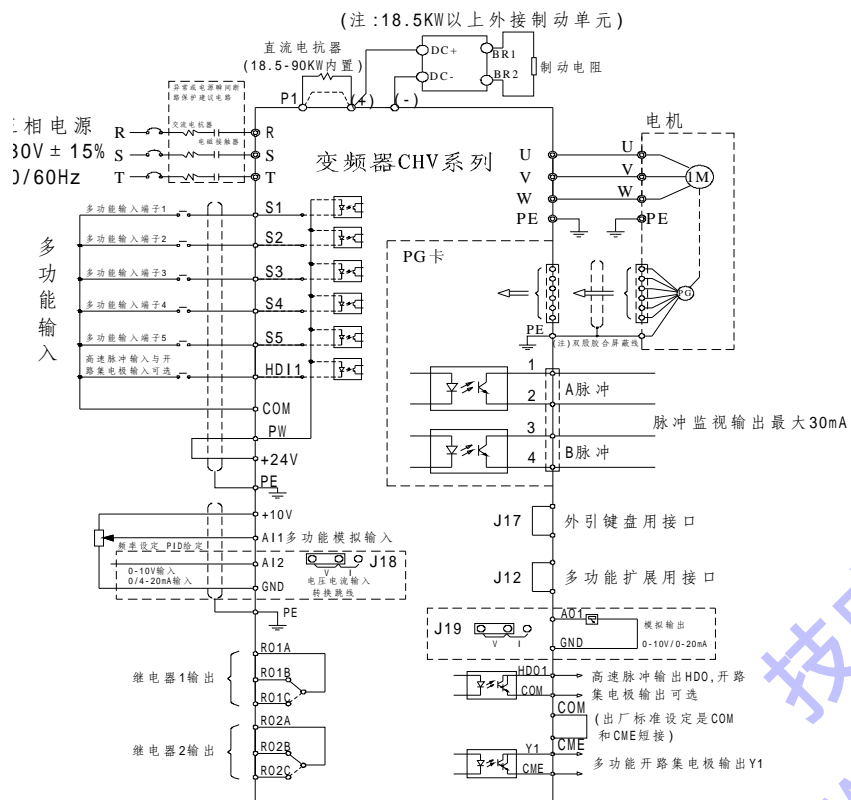
图 4-8 标准接线图
