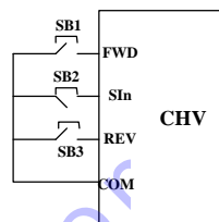
图 6-13 三线式控制模式 2
