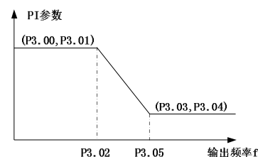
图 6-6 PI 参数示意图
