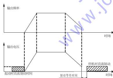
图 6-5 直流制动示意图
