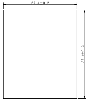
图 3-5 外引键盘(小)的开孔尺寸
