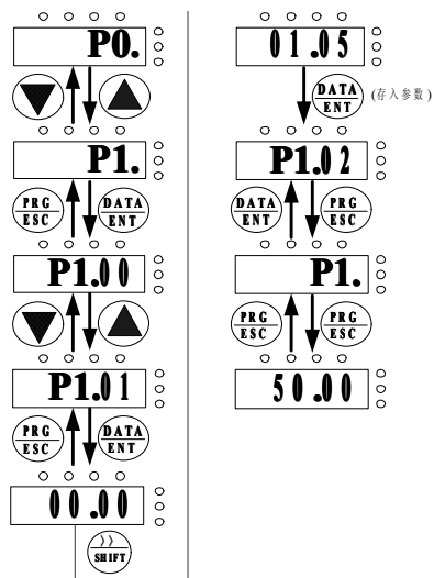
图 5-2 三级菜单操作流程图
