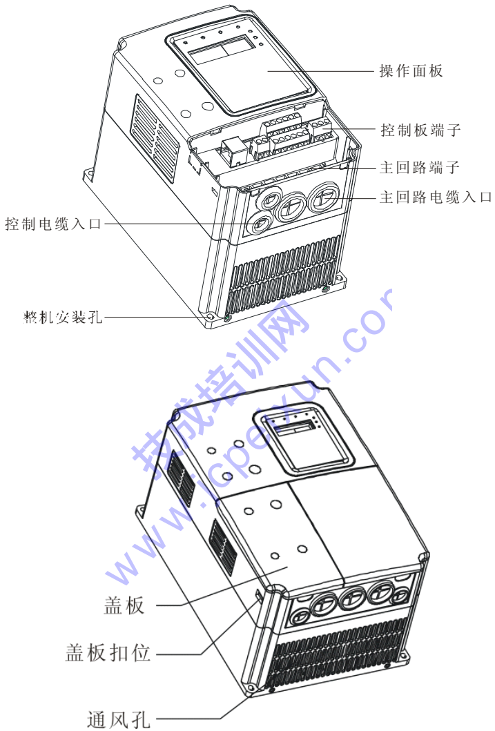
图 1-2 15kW 及以下变频器各部件名称
