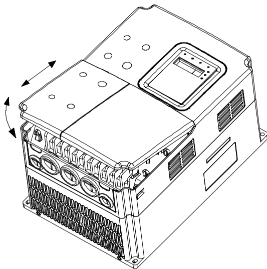
图 3-8 顶部盖板拆卸和安装示意图
