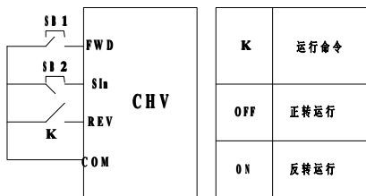
图 6-11 三线式控制模式 1
