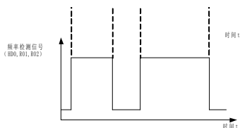
图 6-19 频率到达检出幅值示意图
