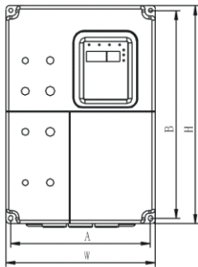
图 1-8 7.5kW 及以下机型的外形尺寸 (220V)
