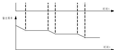
图 6-28 过压失速功能
