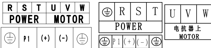
图 4-6 主回路接线端子图(132~315kW) 图 4-7 主回路接线端子图(350~630kW)
