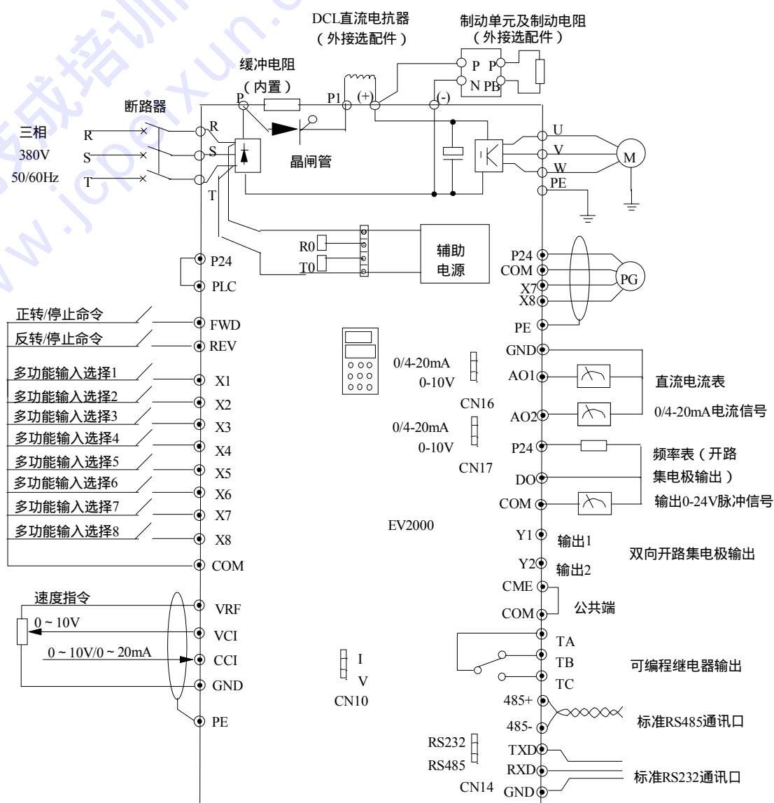
图3 - 11 基本配线图 3
