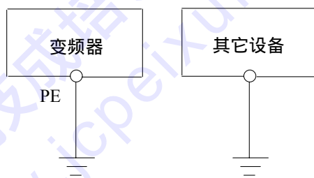
图3 - 37 接地示意图1
