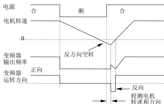
图5-11 转速跟踪再启动示意图
