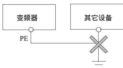
图3 - 39 接地示意图3
