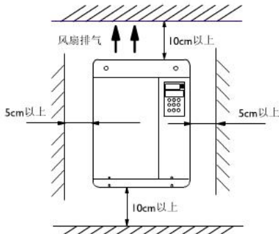
图3-1 安装的间隔距离
