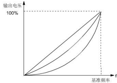
图6-17 节能运行时的V/F曲线
