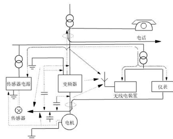
图10-2 噪声传播路径示意图
