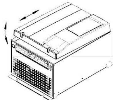
图3-4 塑胶盖板的拆卸和安装示意图
