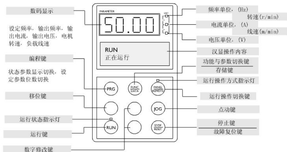
图4-1 操作面板示意图
