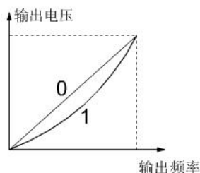
图6-2 V/F曲线
