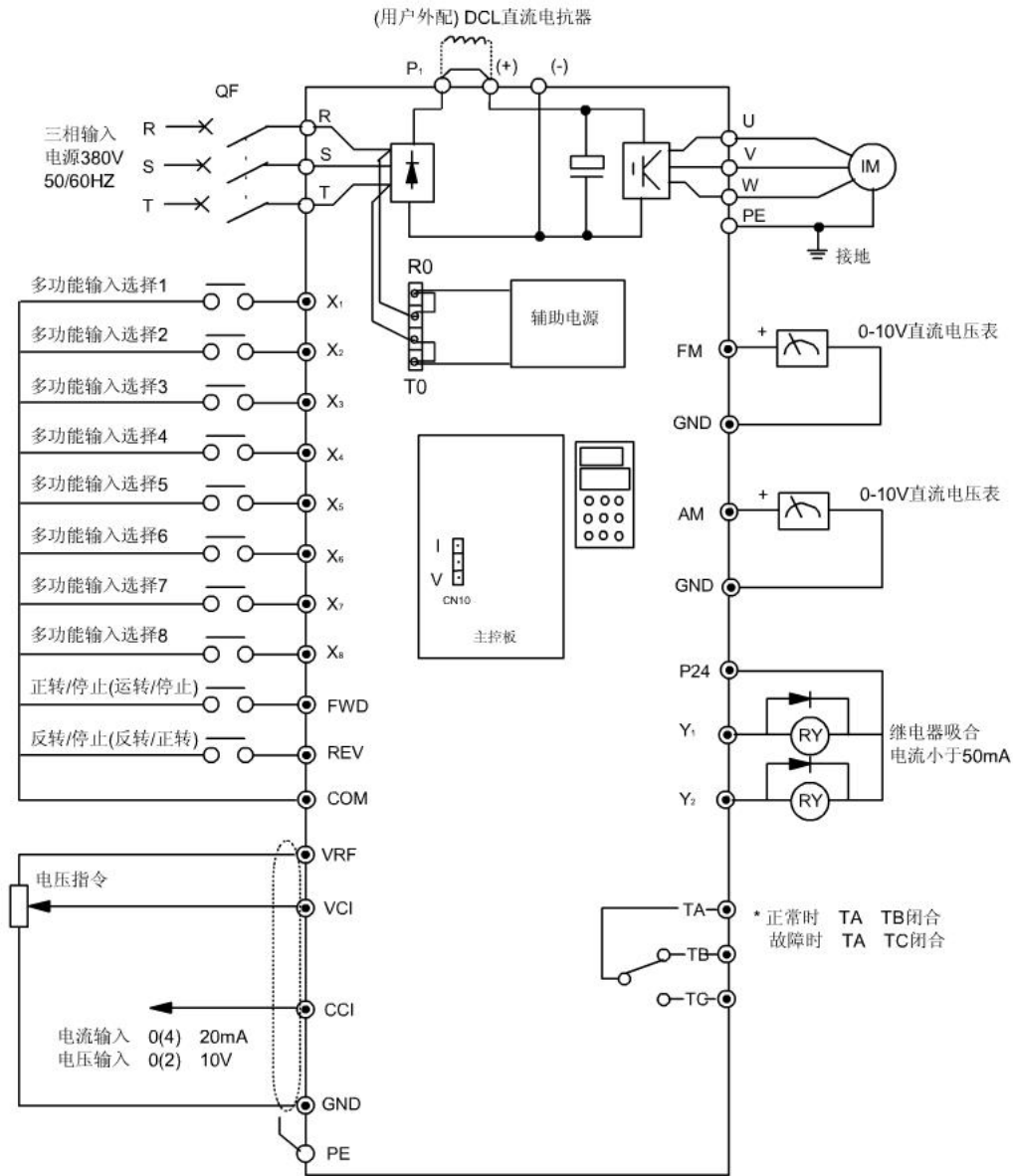
图3-8 基本配线图3
