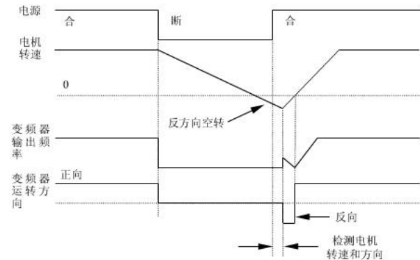
图6-7 停电再启动示意图
