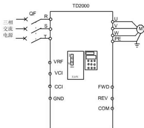
图3-9 基本配线图
