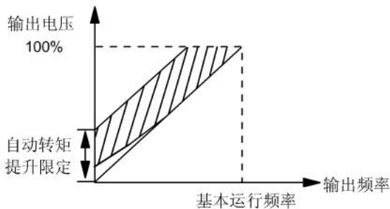
图6-16 自动转矩提升补偿
