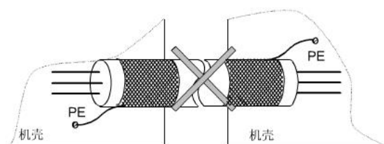
图10-5 错误的屏蔽接地方法
