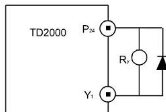
图6-35 开路集电极输出端子接线图
