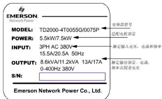
图1-1 变频器铭牌
