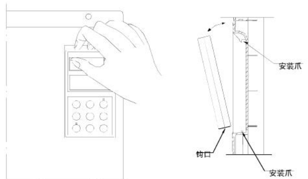
图3-3 操作面板的拆卸和安装
