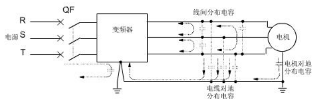
图10-11 漏电流路径
