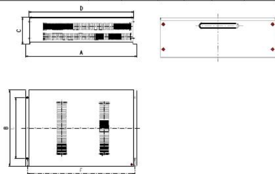
图9-5 制动电阻的安装尺寸示意图
