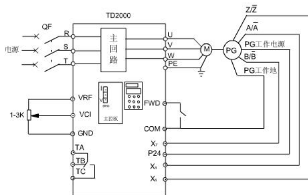
图6-27 PG速度闭环控制系统接线图
