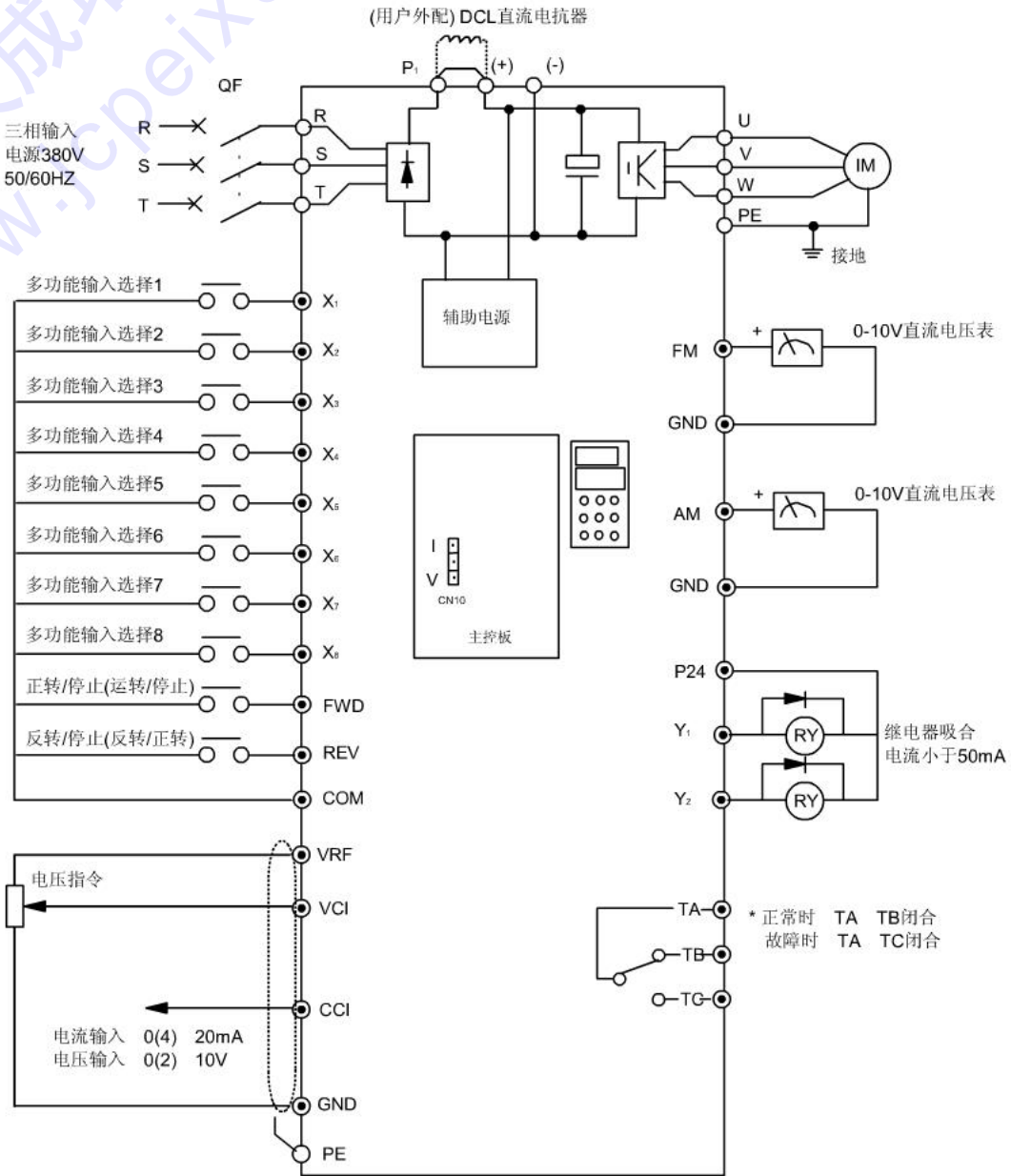
图3-7 基本配线图2
