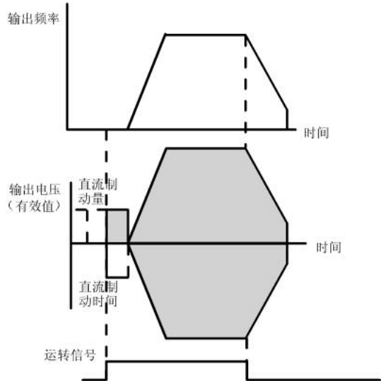
图6-8 启动方式1说明
