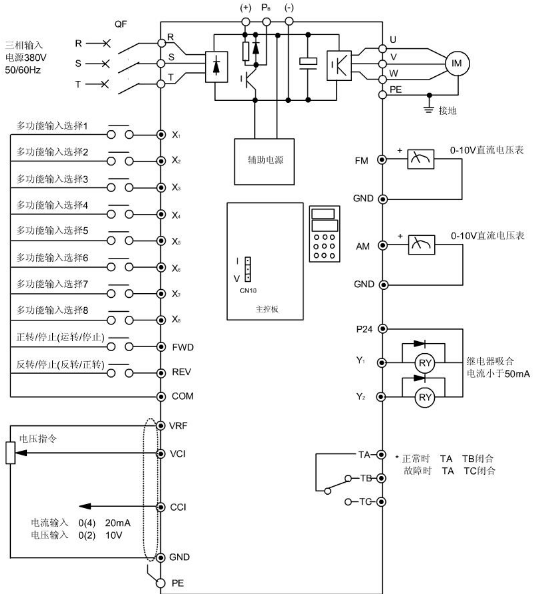
图3-6 基本配线图1
