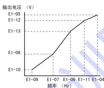
图 4.22 V/f 曲线图
