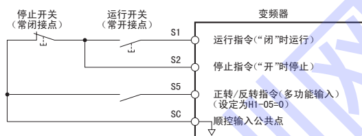
图 5.43 3 线制顺控的接线示例
