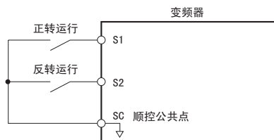
图 5.54 2 线制顺控的接线示例
