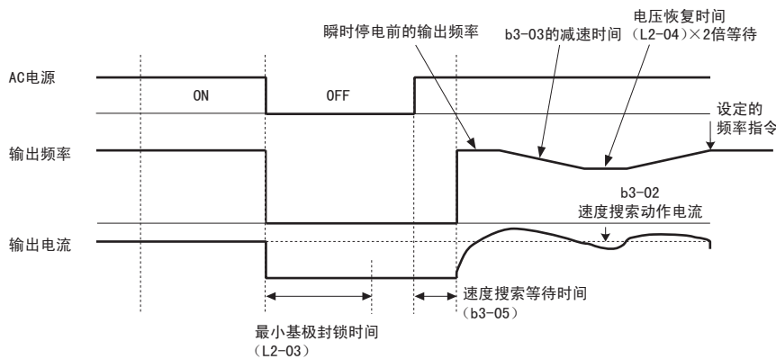
图 5.18 瞬时停电后的速度搜索（电流检出形：瞬时停电时间 > L2-03 时）
