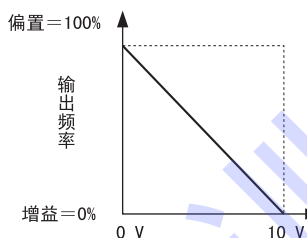
图 5.71 调整逆变性场合的增益和偏置时的输出频率
