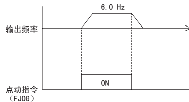
图 4.28 点动运行曲线
