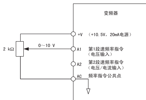
图 5.3 第 1 段速频率指令的电压输入
