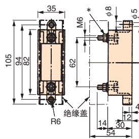
外形图 1
