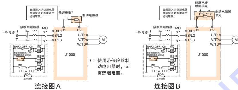
连接图 A
