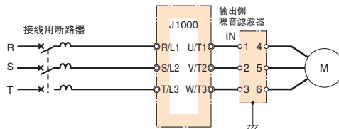
连接图
