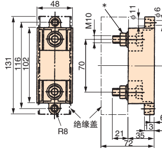
外形图 2
