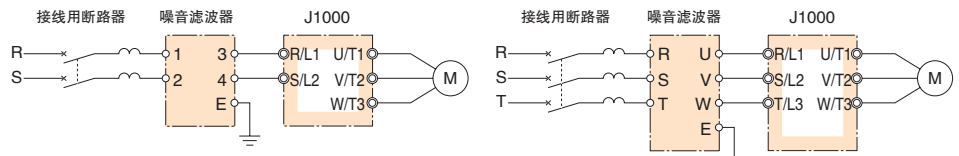
单相输入时(LNFB型)
