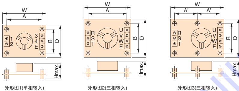
外形图1(单相输入)
