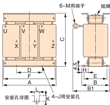
外形图 2
