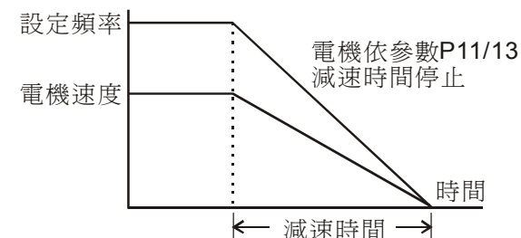
圖一：減速煞車
