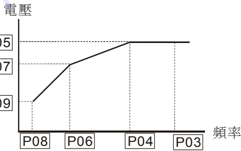
圖二：任意V/F曲線設定
