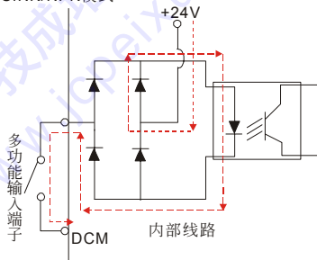
SINK/NPN模式
