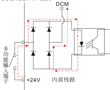
SOURCE/PNP模式
