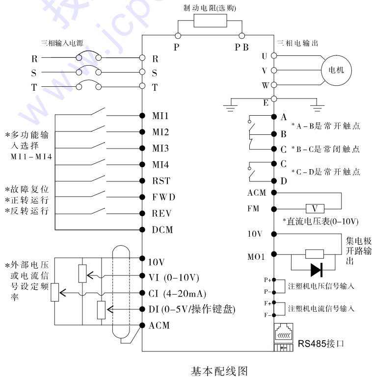
标准配线图
