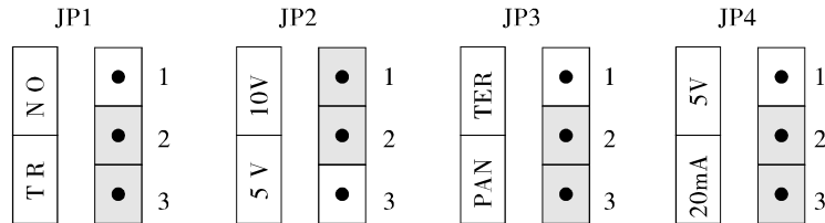
终端电阻选择跳线
