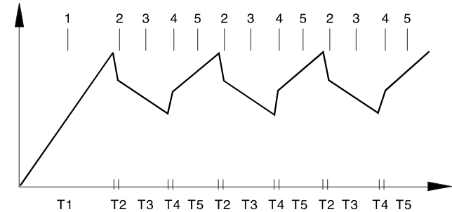
F072=6的应用例图
