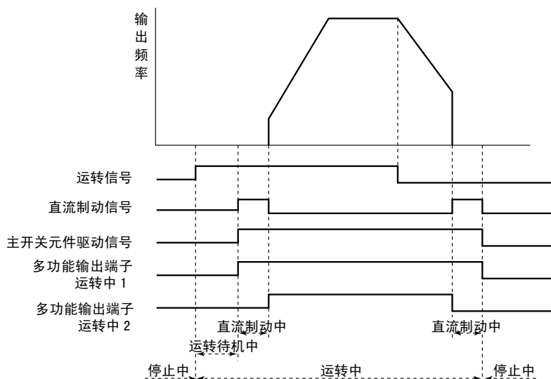
图 6-5 运行动作
