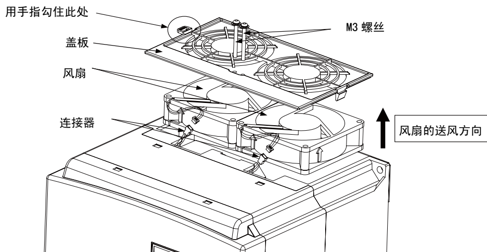
图 10-2 风扇的更换步骤 (SVC06-0110~0150)
