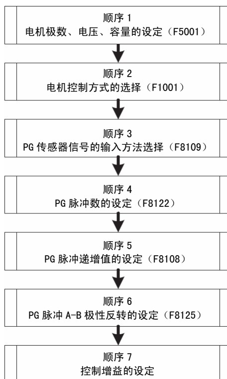
PG 传感器基本功能设定的顺序流程
