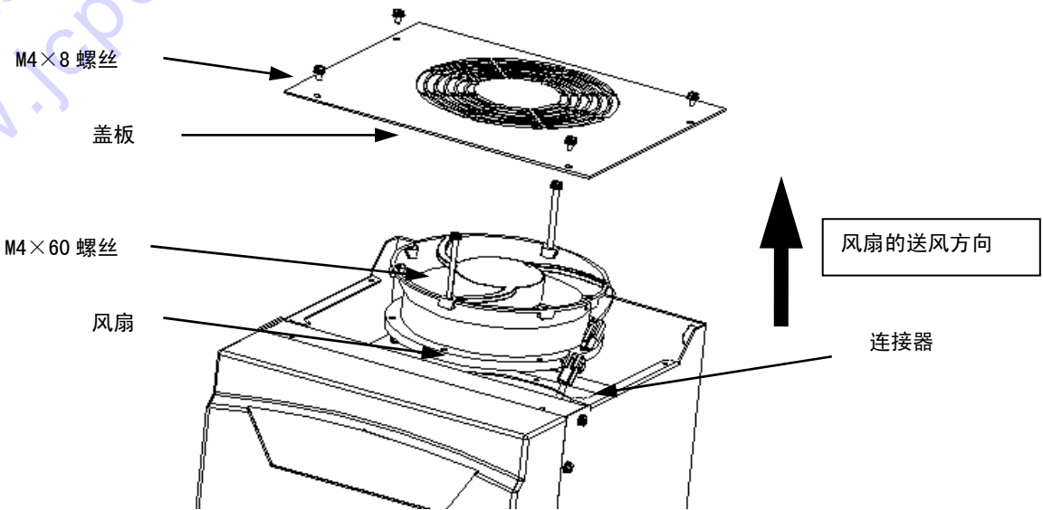
图 10-4 风扇的更换步骤 (SVC06-0370~0450)
