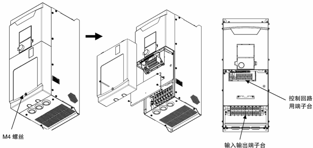
图 3-5 前盖板 (下), 内部封盖铁板拆卸
