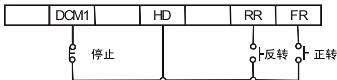
图 6-4 运转信号保持电路
