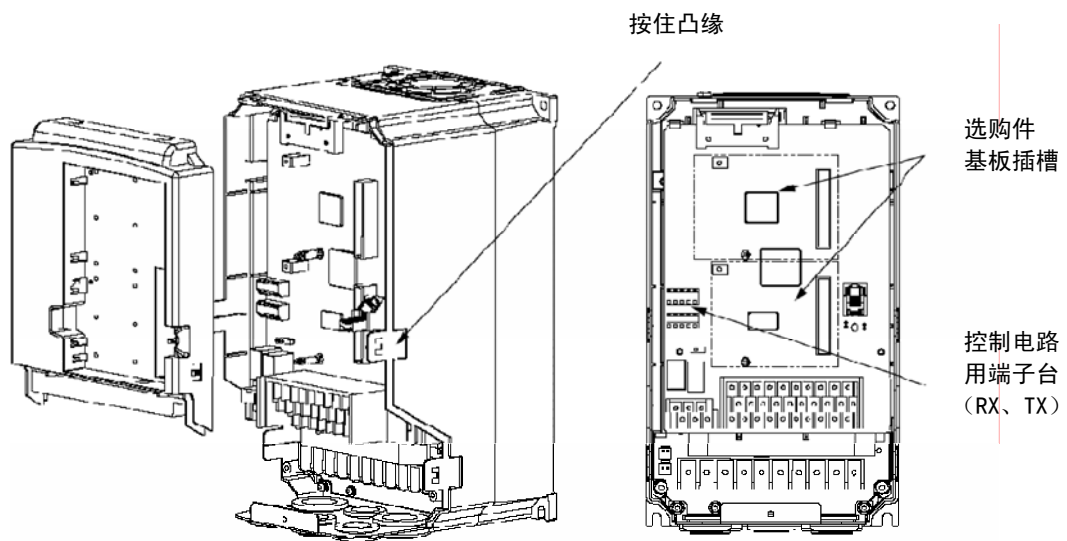
图 3-6 前盖板（上）拆卸
