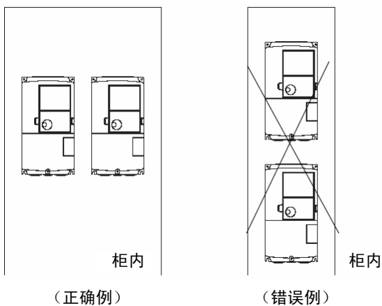
图 3-3 柜内设置方法
