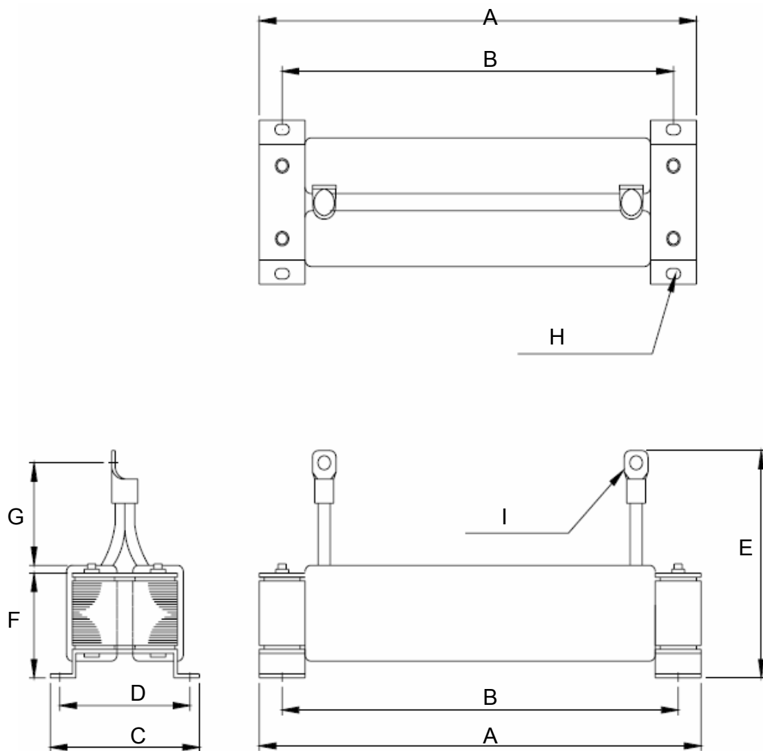
12-3 大容量变频器用 DC 电抗器外形图
