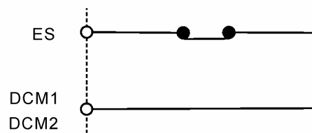
图 4-3 ES 端子的信号模式切换
