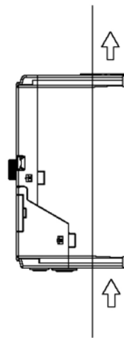
图 3-2 散热部分的柜外设置方法
