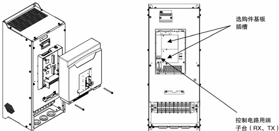
图 3-6 前盖板 (上) 拆卸
