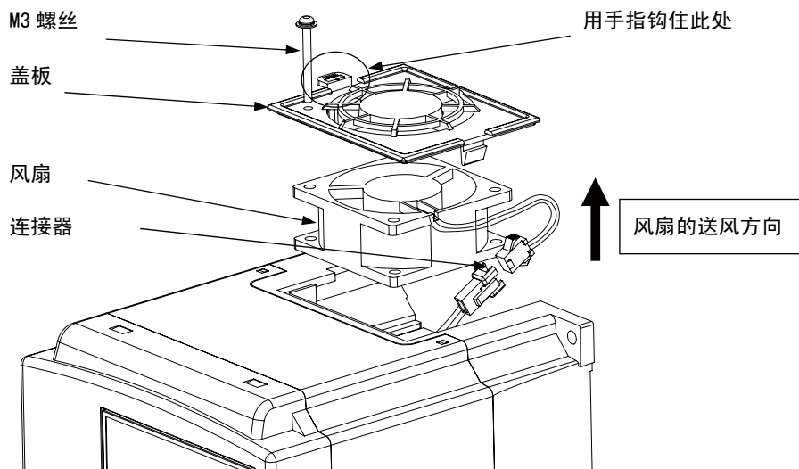
图 10-1 风扇的更换步骤 (SVC06-0015~0075)
