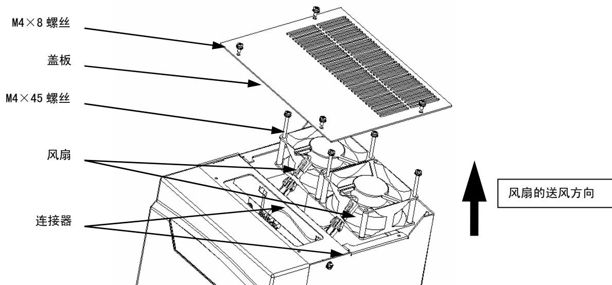
图 10-3 风扇的更换步骤 (SVC06-0185~0300)
