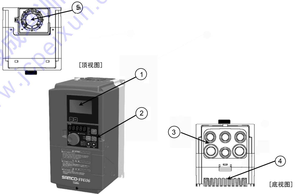
图 2-2 各个部分的名称
