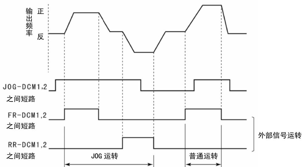
图 6-3 JOG 动作
