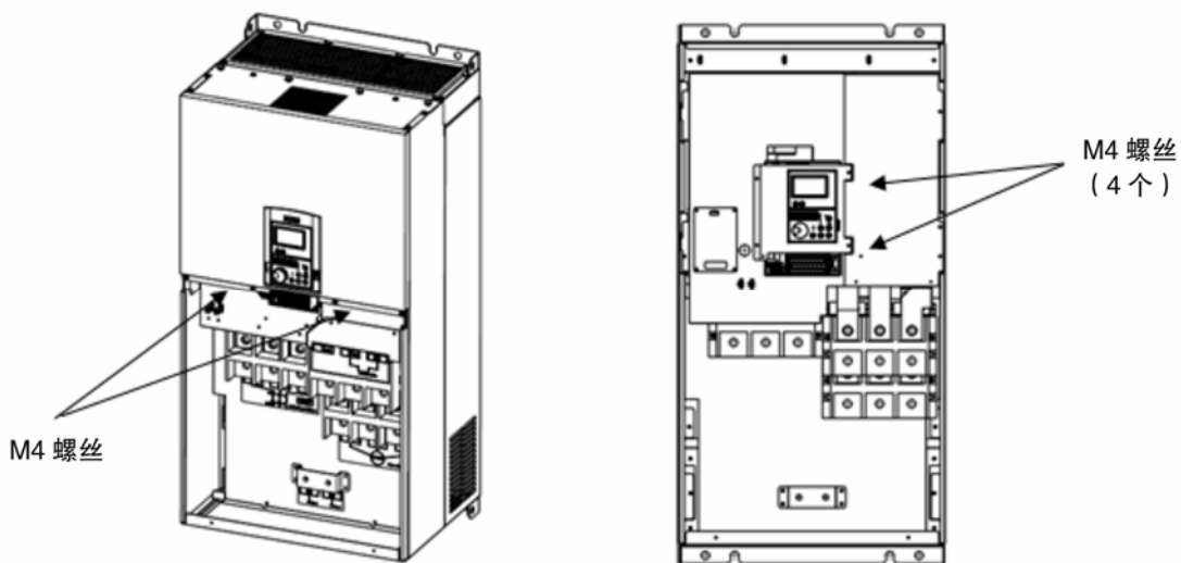
图 3-8 (1) 前盖板（上）拆卸
