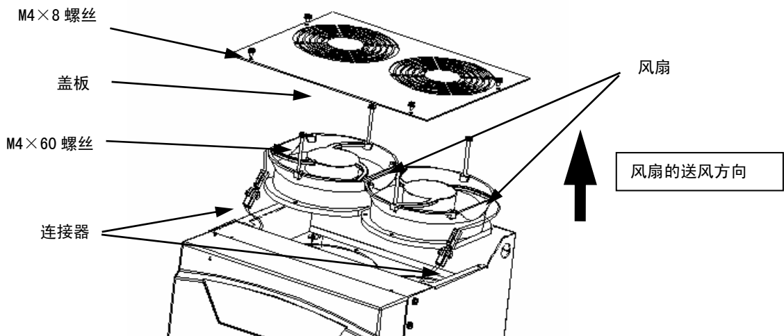
图 10-5 风扇的更换步骤 (SVC06-0550~0570)
