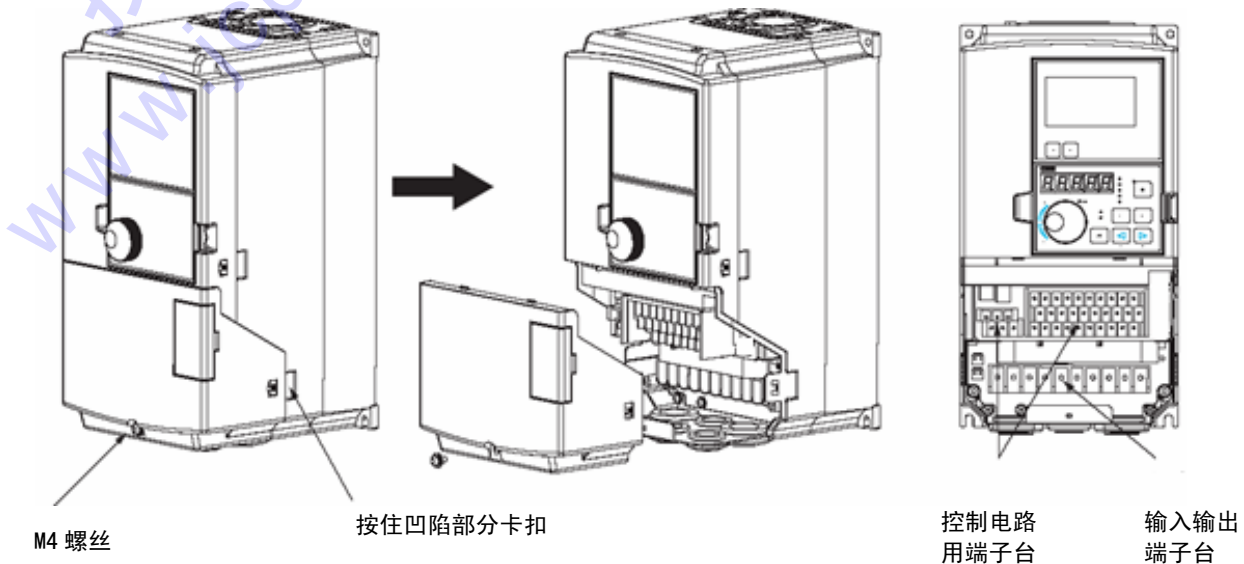
图 3-5 前盖板（下）拆卸
