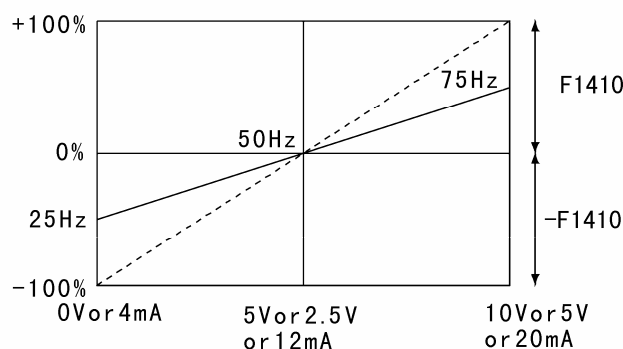
VII F1 或者 VIF2 或者 VIF3 输入
