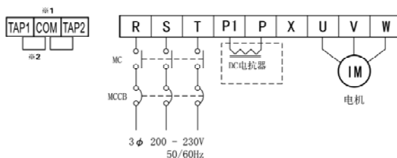
图4-3-4 VM05-37K~75K的情形
