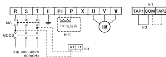
图4-3-5 VM05-90K~220K的情形
