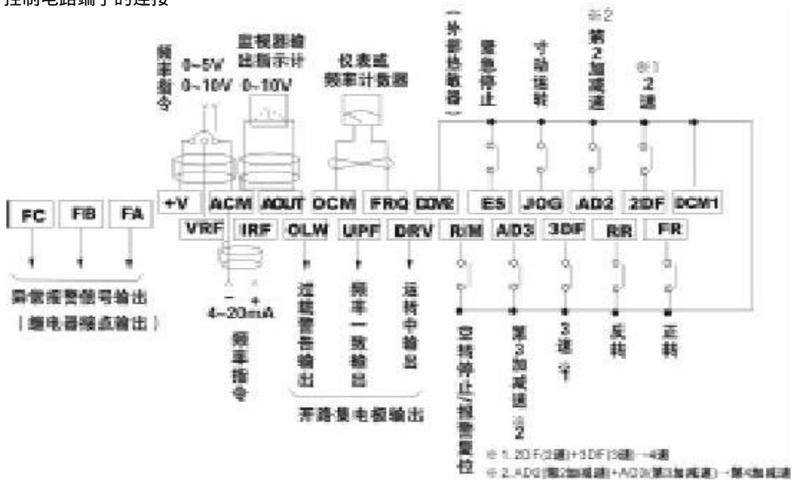
图5 控制电路端子的连接图
