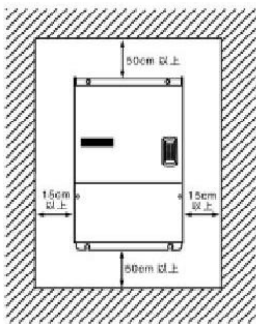
图2 变频器四周的空间
