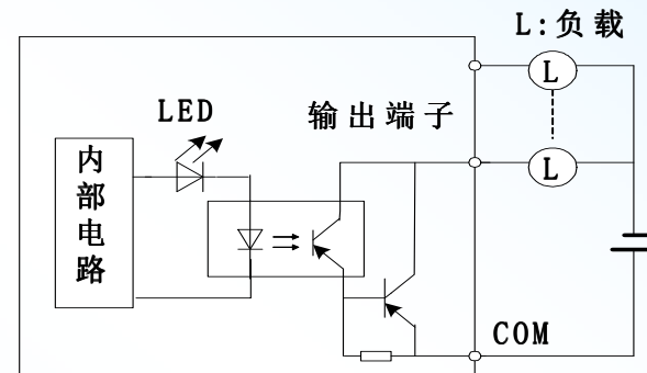
(d) 晶体管输出型 (PNP集电极开路)
