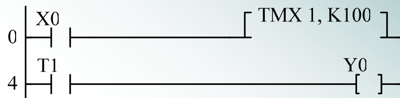
指令表
