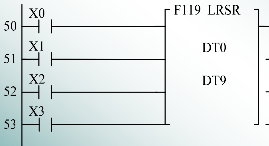
梯形图
