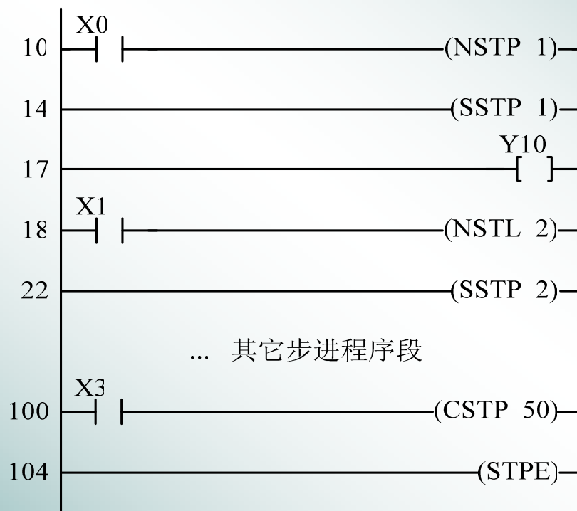
梯形图
