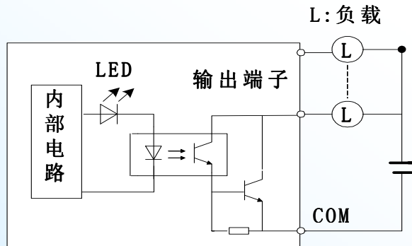
(c) 晶体管输出型 (NPN集电极开路)
