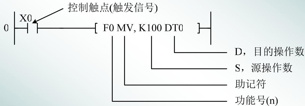
梯形图
