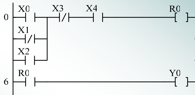
梯形图
