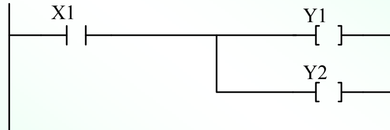
PLC梯形图
