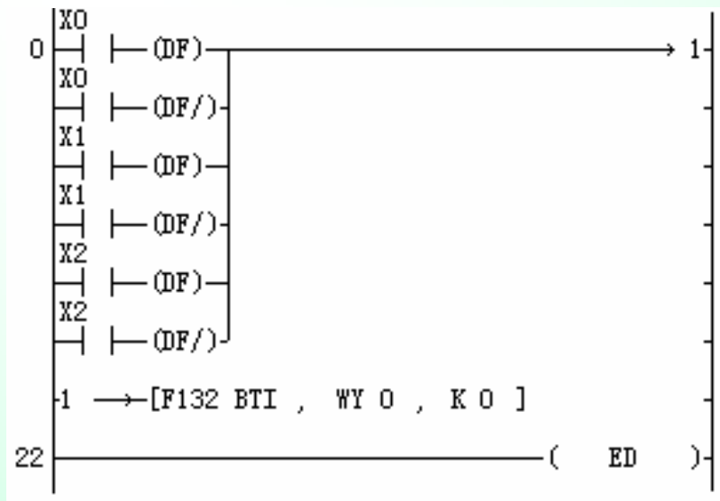
三地控制一盏灯程序 (3)
