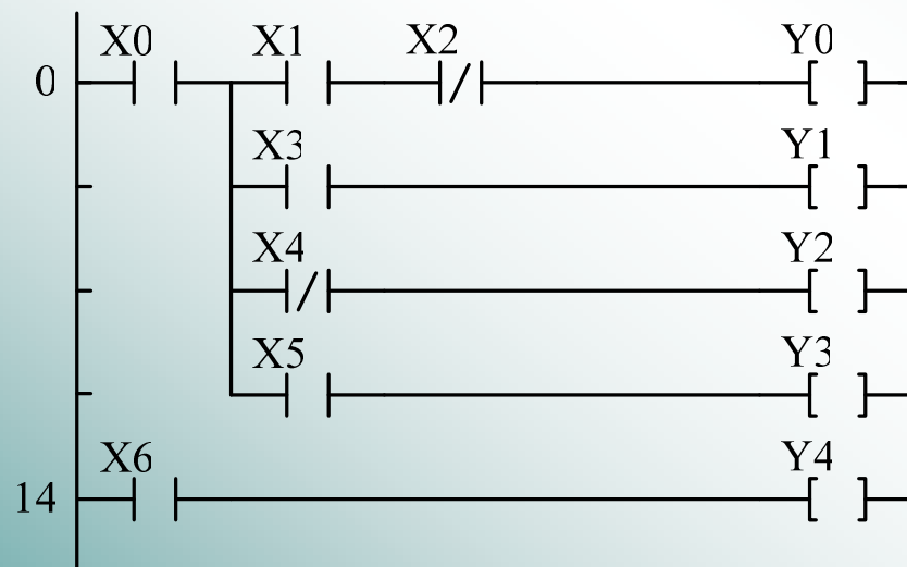
梯形图
