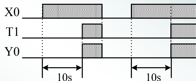
时序图
