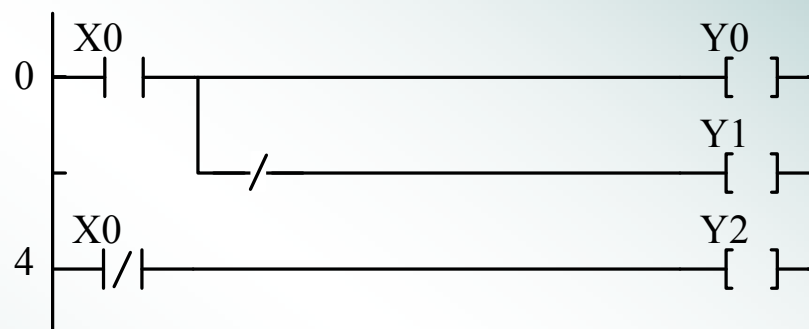
梯形图
