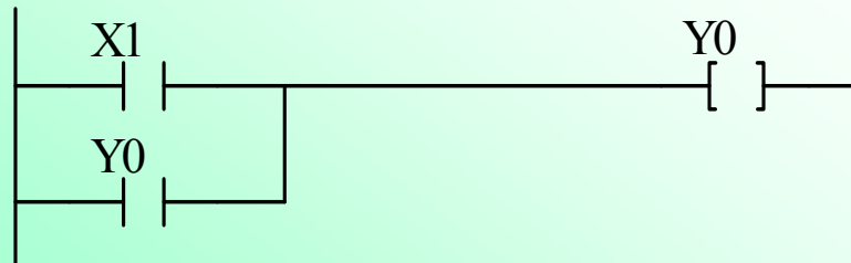
电机初步正转控制电路
