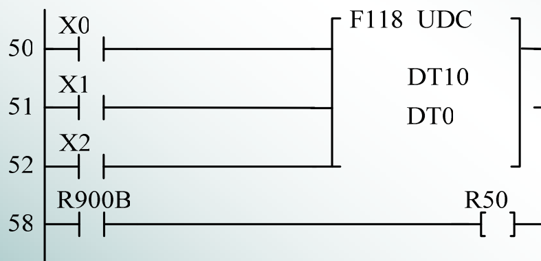
梯形图
