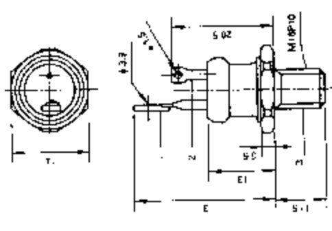
1. 阴极 2. 控制极 3. 阳极
