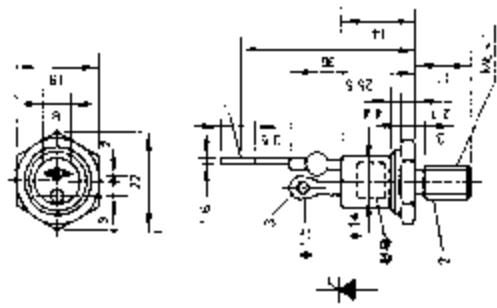
1. 阴极 2. 阳极 3. 控制极
