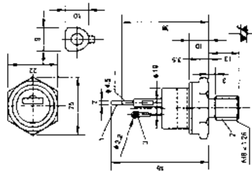
1. T1 2. T2 3. 门极
