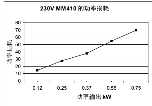
图 2-2 功率损耗, 230 V
