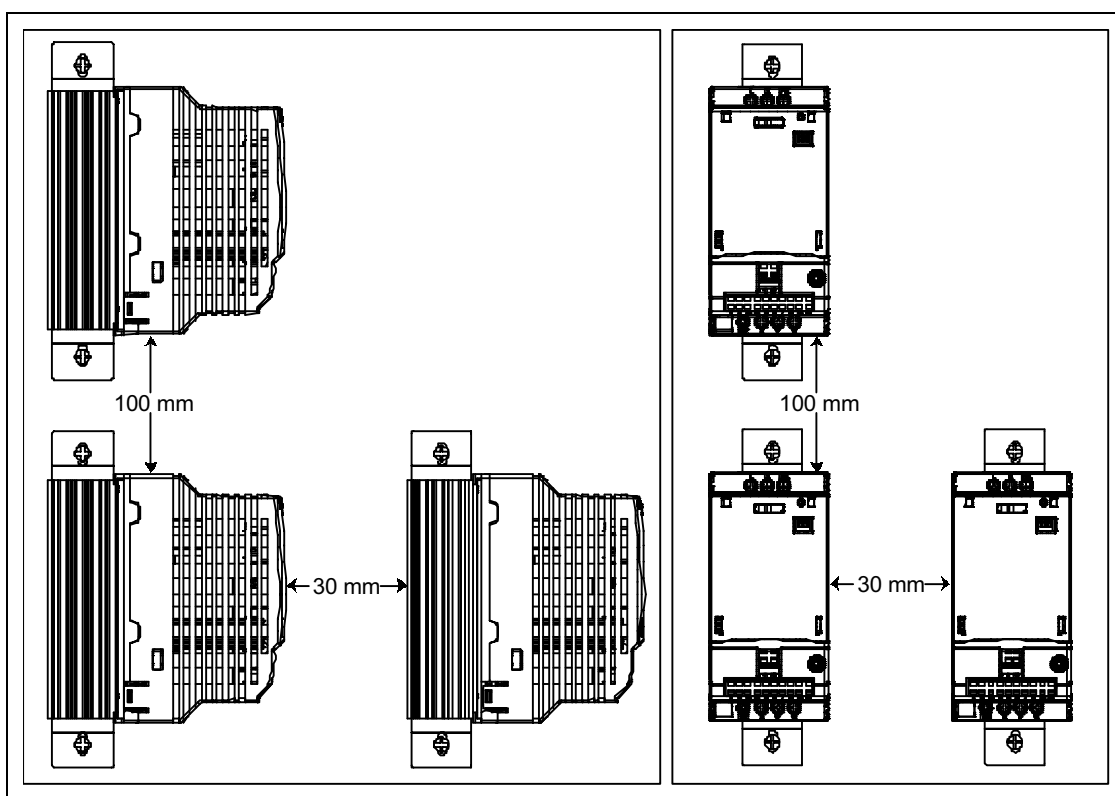
图 2-5 MICROMASTER 410 变频器间的安装间隙
