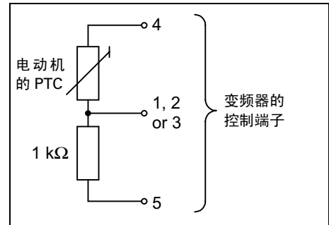
图 3-8 电动机过载保护的 PTC 接线
