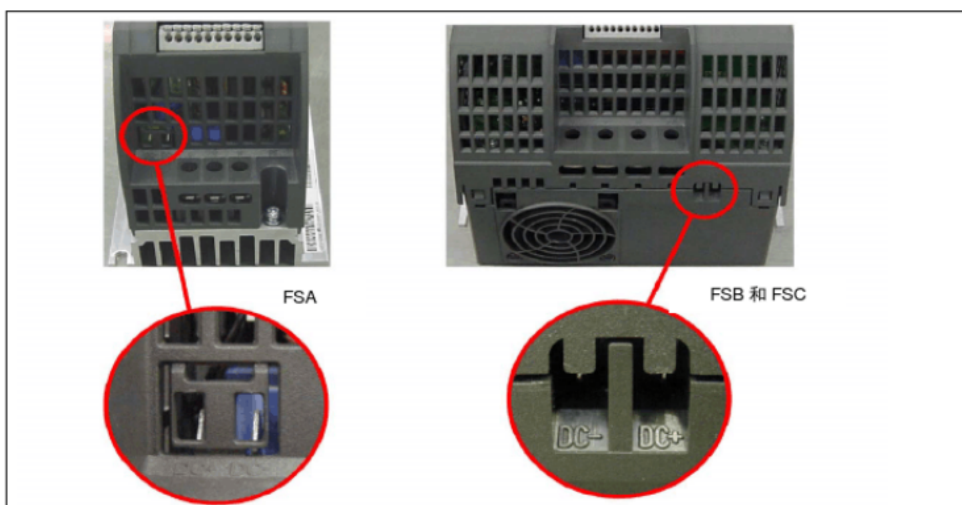
图 2-6 SINAMICS G110 变频器
