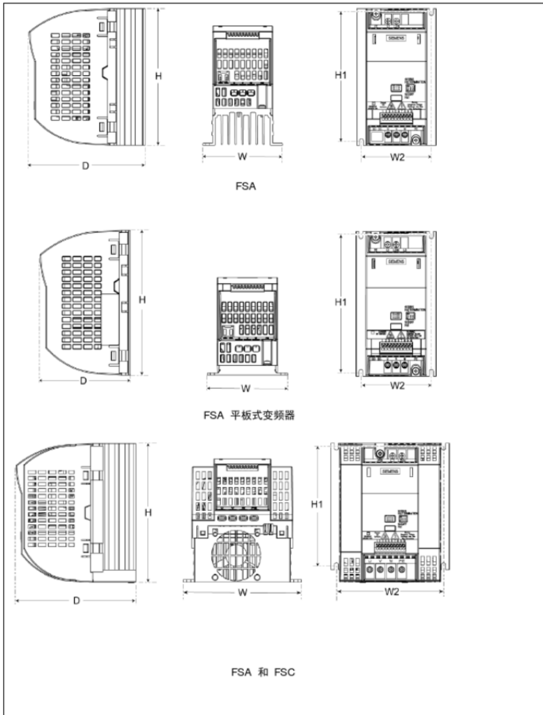
图2-3 SINAMICS G110 变频器的外形尺寸
