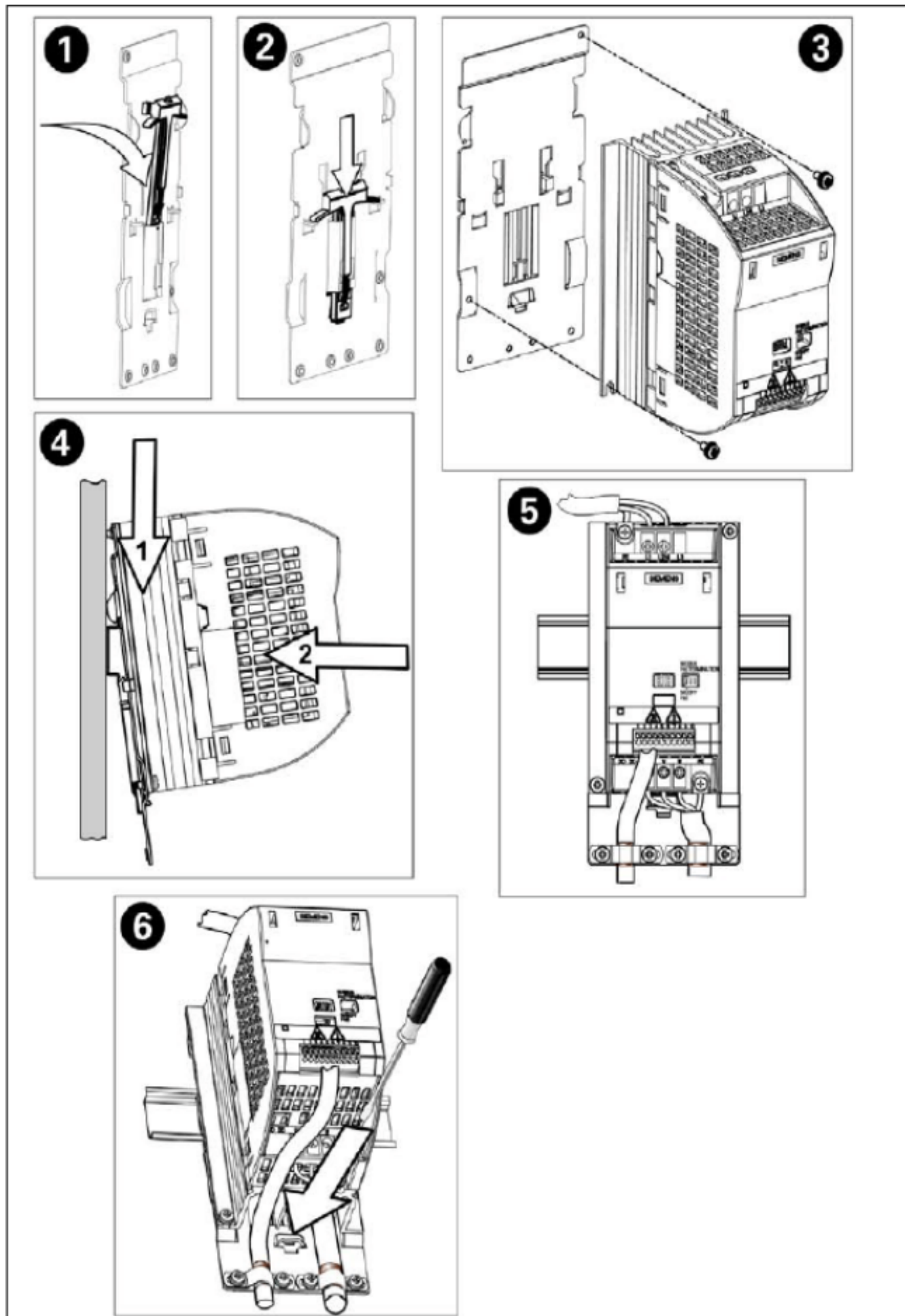
图 B-1 DIN 导轨安装组合件的安装
