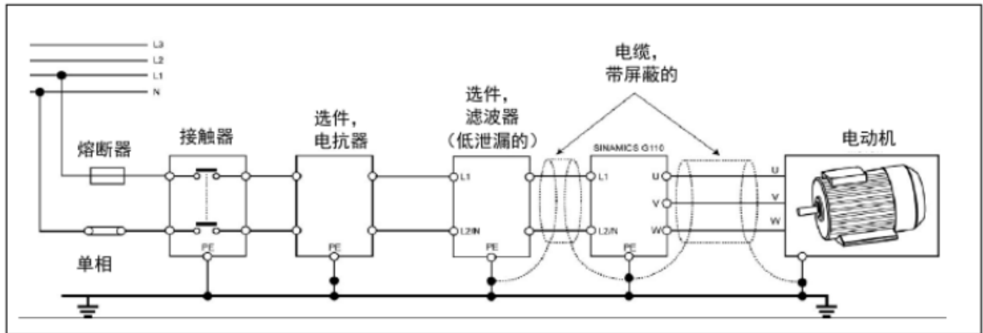
图2-7 电动机和电源端子的接线方法
