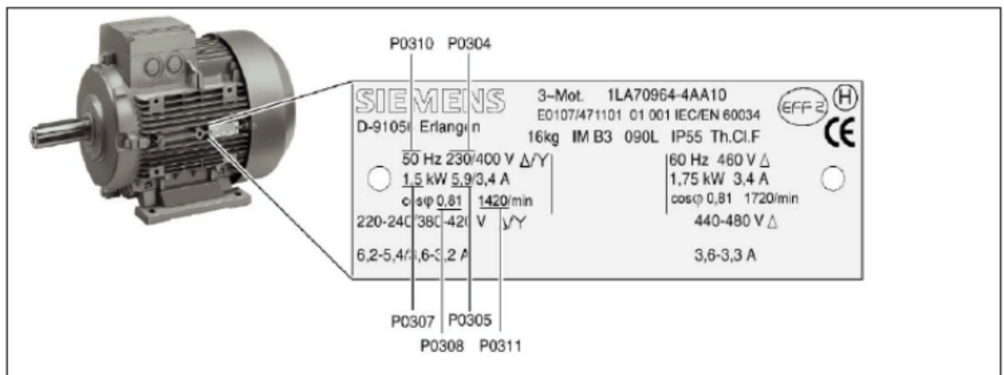
图 3-6 典型的电动机铭牌举例
