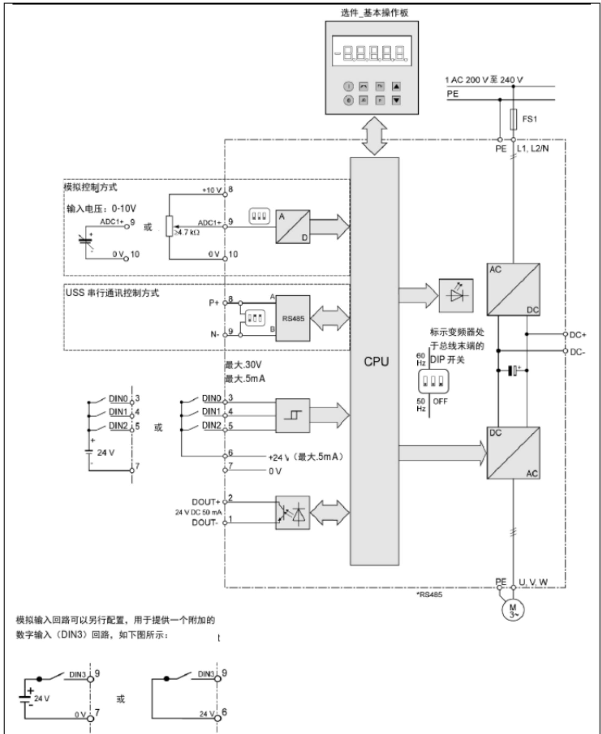
图 3-1 变频器的方框图
