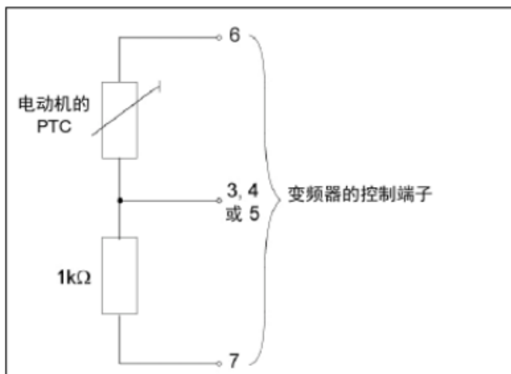
图 3-7 电动机的 PTC 过热保护
