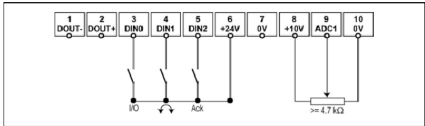
图 3-1 由模拟信号控制时的接线
