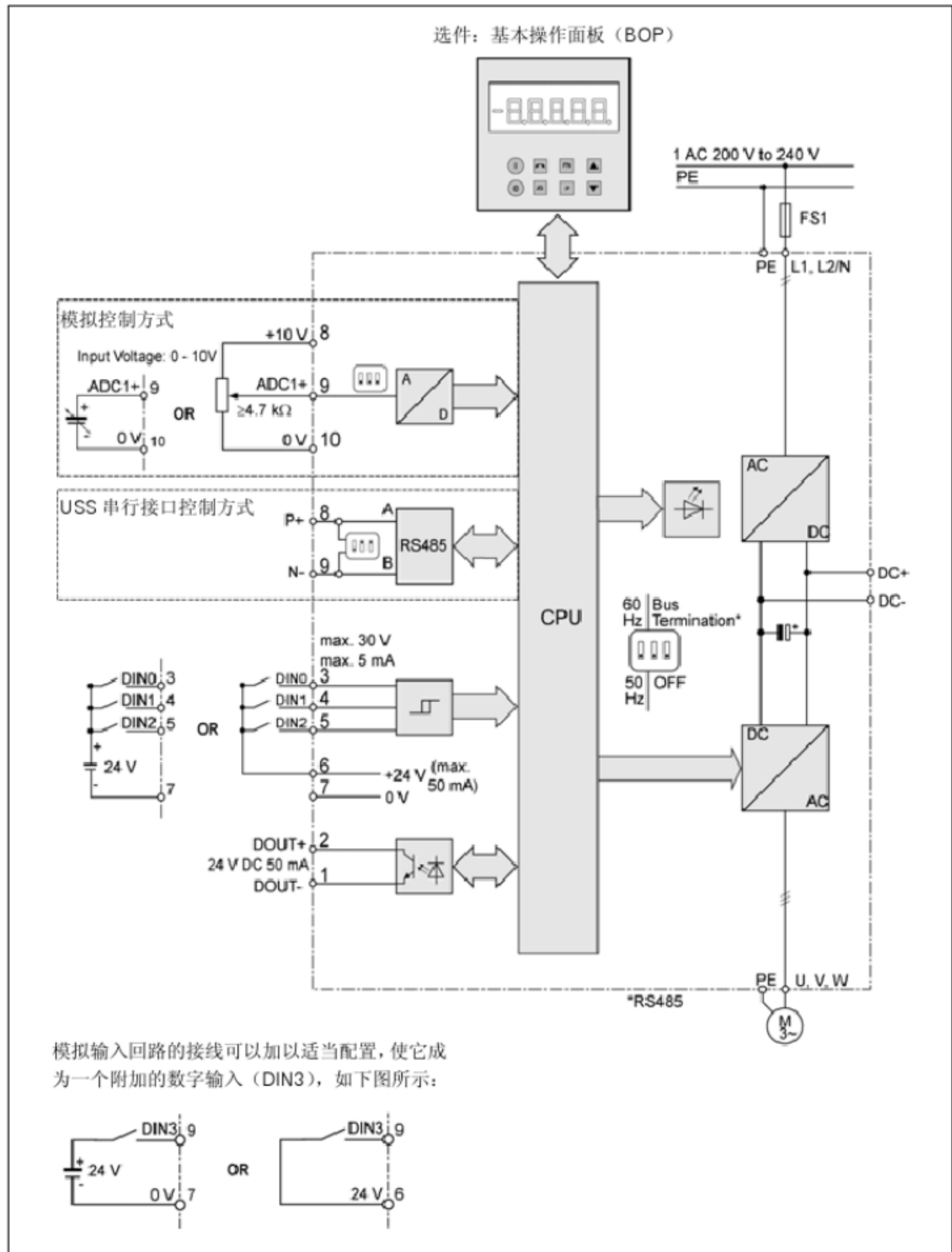
图 2-2 变频器的方框图
