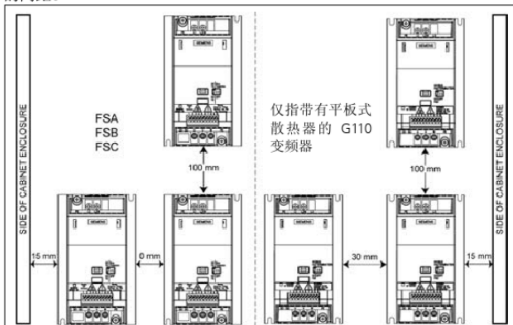
图 1-1 变频器之间的安装间距
