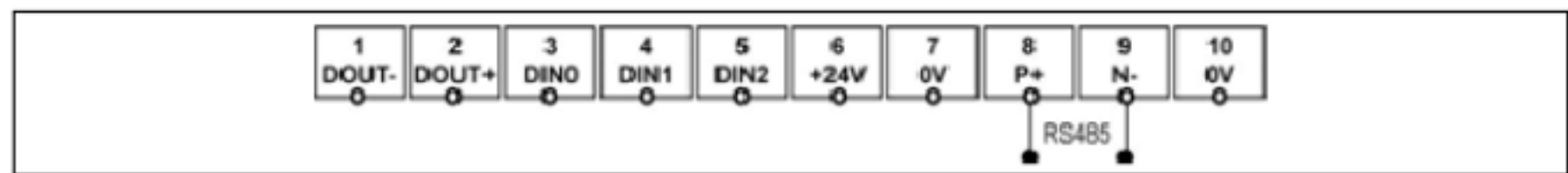
图 3-2 由 USS 串行接口控制时的接线
