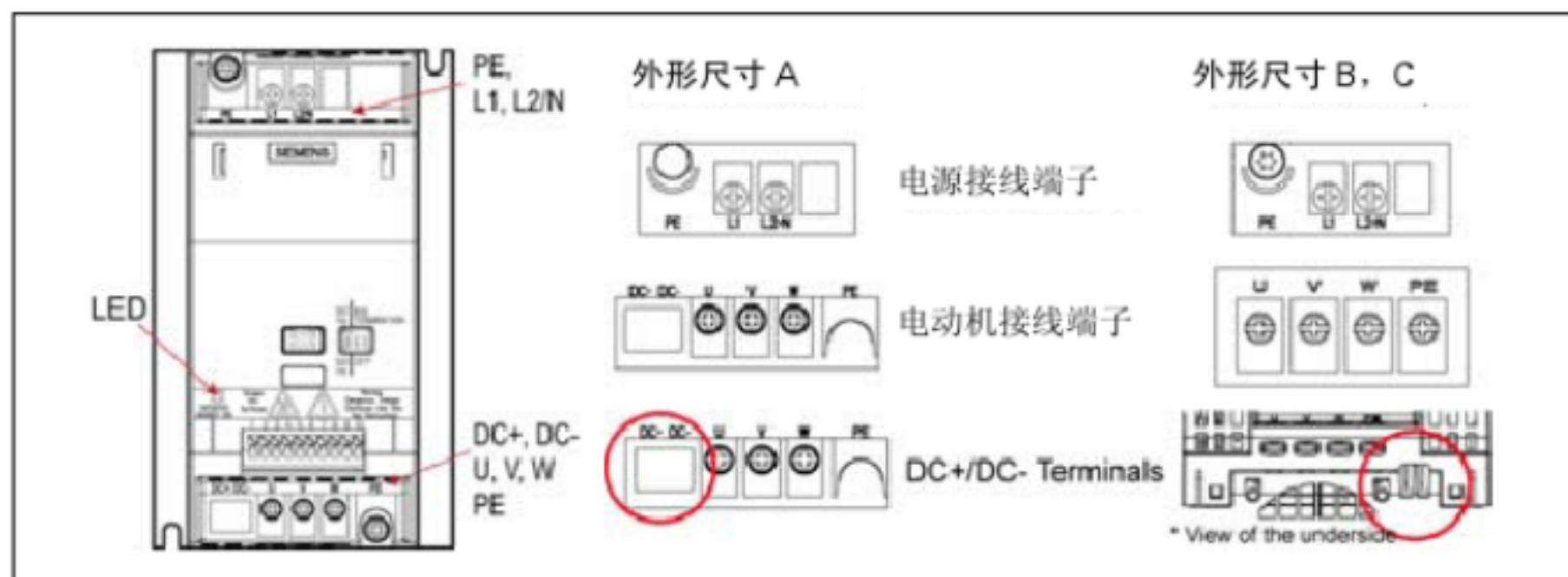
图 2-1 电源和电动机接线端子
