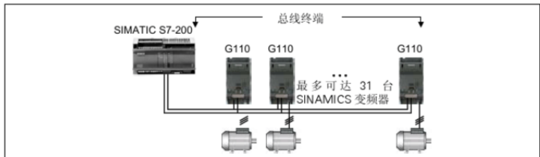
图 3-3 举例，USS 总线
