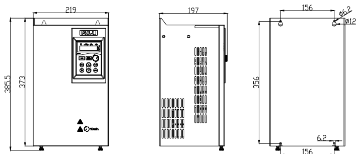
图 1-5 18.5kW-22kW 安装尺寸
