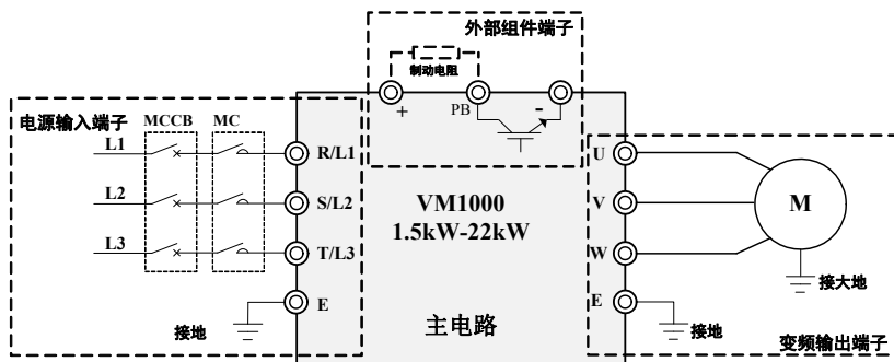
图 2-11 1.5~22kW 主回路接线图
