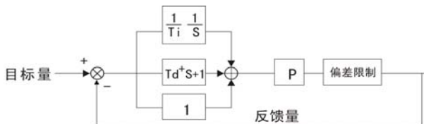
图 6-21 过程 PID 原理框图
