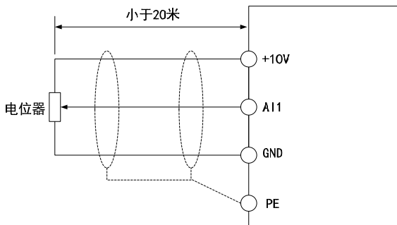
图 2-19 模拟量输入端子接线示意图
