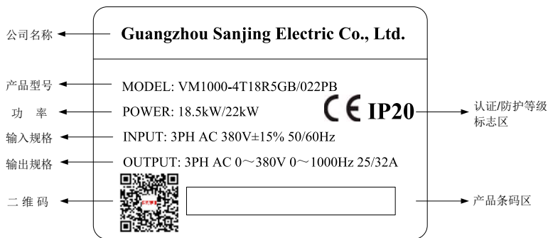
图 1-1 产品铭牌
