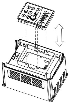
图 2-5 键盘拆装示意图 (1.5kW-7.5kW, , 含 11kW P 型机)
