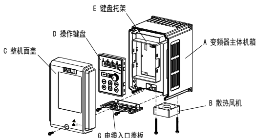
图 2-1 变频器组成 (1.5kW-7.5kW, 含 11kW P 型机)
