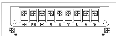
图 2-13 1.5~7.5kW 主回路端子图
