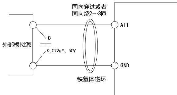
图 2-20 模拟量输入端子处理接线图
