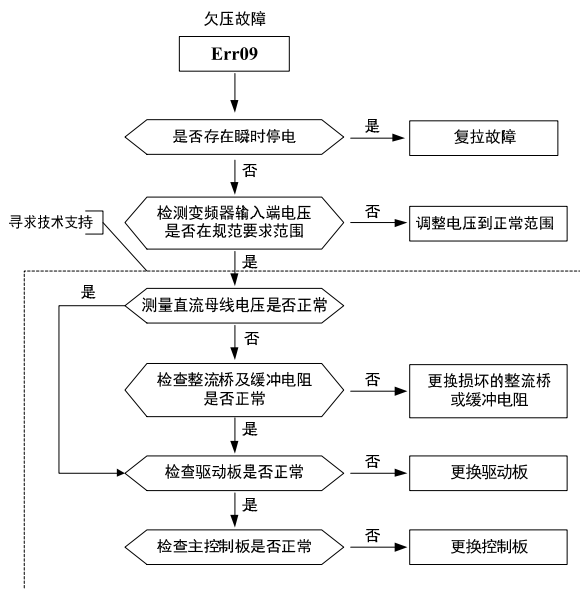
图 8-8 欠电压故障 (Err09)
