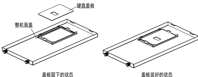
图 1-12 11kW 及以上键盘盖板安装示意图
