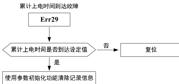
图 8-22 累计上电时间到达故障 (Err29)
