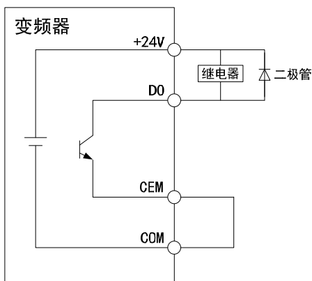
图 2-23 数字输出端子接线示意图
