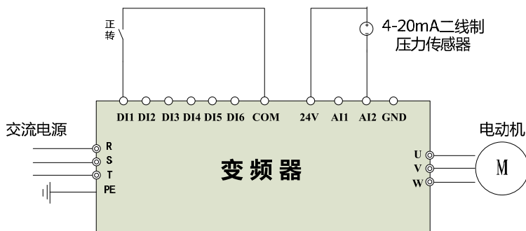
图 4-4 变频器数字给定 PID 控制
