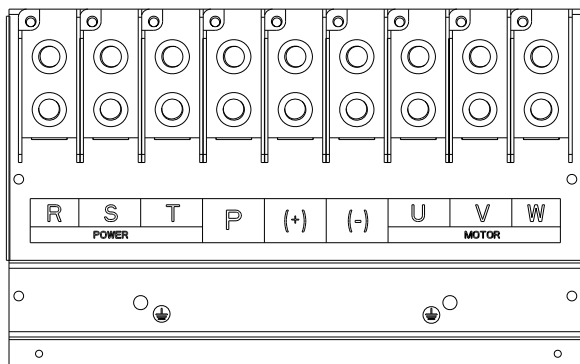
图 2-16 75 ~160kW 主回路端子图
