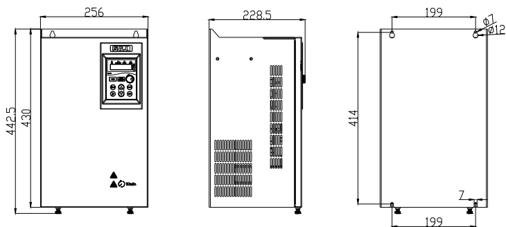
图 1-6 30kW-37kW 安装尺寸
