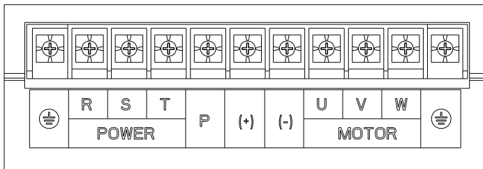
图 2-15 30~37kW 主回路端子图
