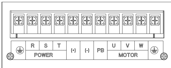
图 2-14 11~22kW 主回路端子图
