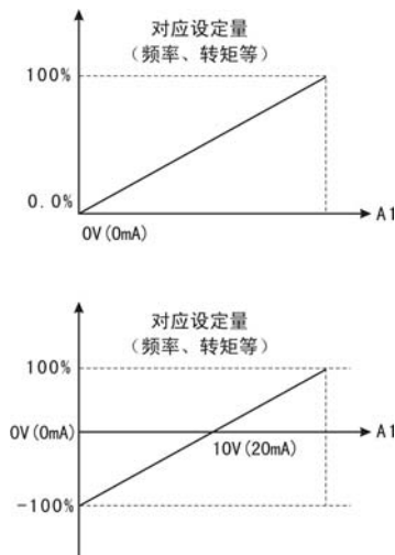
图 6-9 模拟给定与设定量的对应关系
