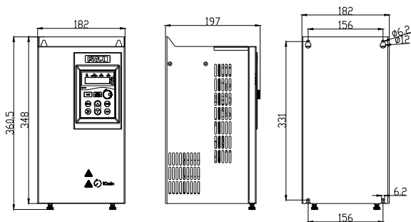
图 1-4 11kW-15kW 安装尺寸
