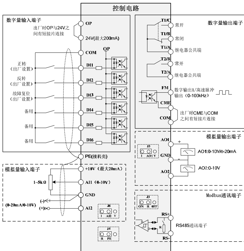
图 2-17 控制回路接线图 (模拟量输入输出改为 0~20mA)
