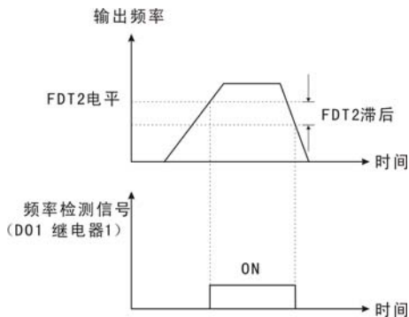
图 6-16 FDT2 电平示意图
