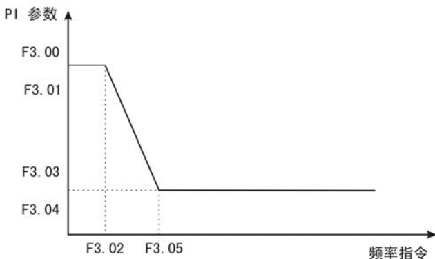
图 6-5 PI 参数示意图
