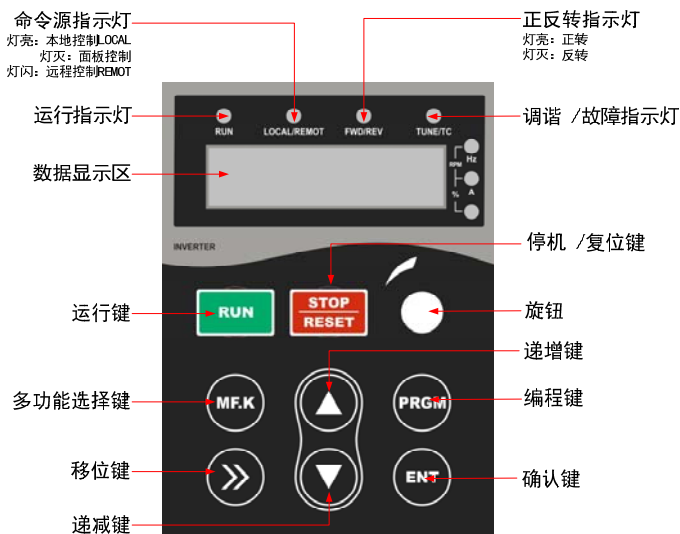
图 3-1 操作面板示意图
