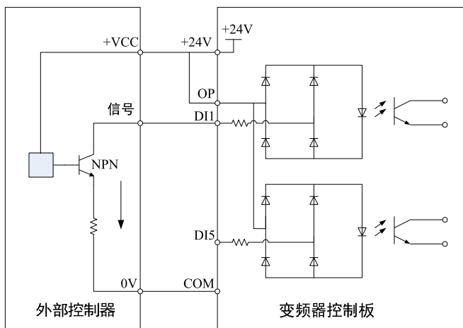
图 2-21 漏型接线方式
