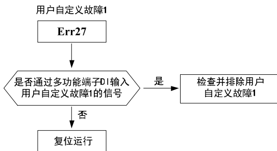
图 8-20 用户自定义故障 1 (Err27)
