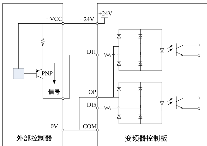
图 2-22 源型接线
