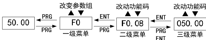
图 3-2 三级菜单操作流程图
