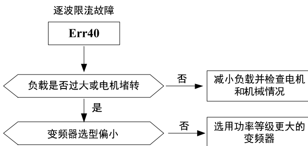
图 8-24 逐波限流故障 (Err40)
