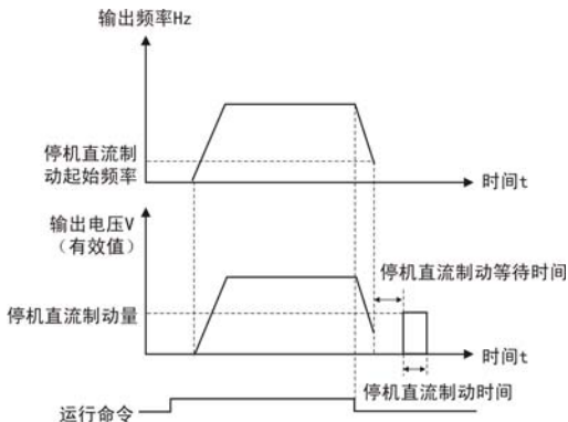
图 6-4 停机直流制动示意图
