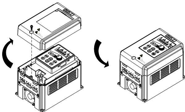
图 2-3 面盖拆装示意图 (1.5kW-7.5kW, 含 11kW P 型机)
