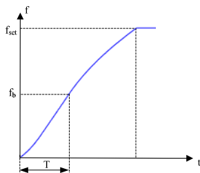
图 6-3 S 曲线加减速 B 示意图
