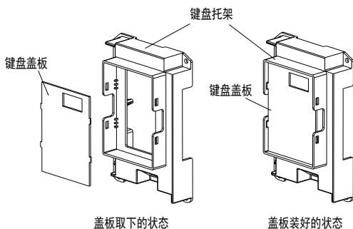
图 1-11 1.5-7.5kW 键盘盖板安装示意图
