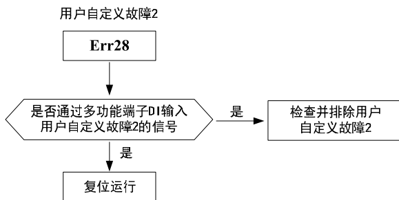
图 8-21 用户自定义故障 2 (Err28)
