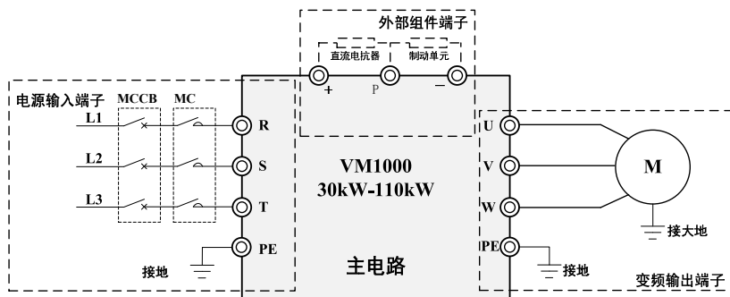
图 2-12 30~400kW 主回路接线图
