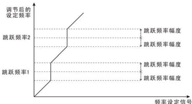
图 6-14 加减速过程中跳跃频率有效示意图
