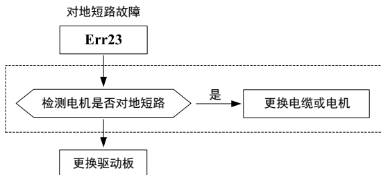
图 8-18 对地短路故障 (Err23)
