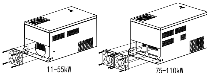
图 2-7 风扇拆装示意图
