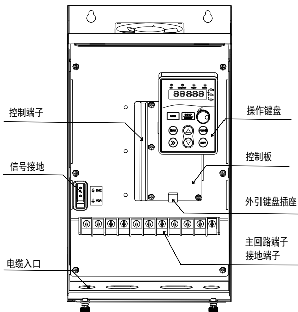
图 2-10 电气组成部分图
