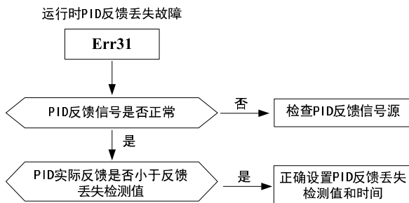
图 8-23 运行时 PID 反馈丢失 (Err31)
