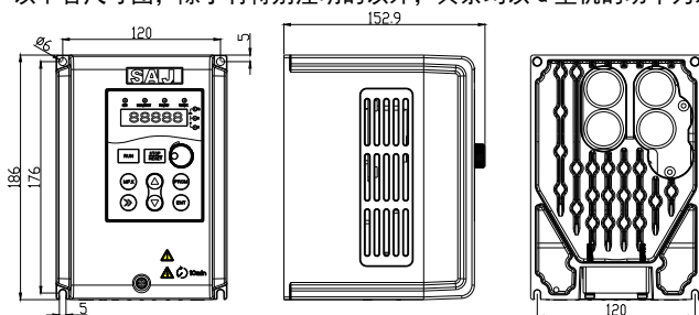
图 1-2 1.5kW-3.7kW 安装尺寸
