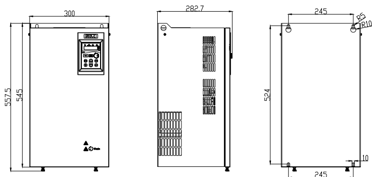
图 1-7 45kW-55kW 安装尺寸
