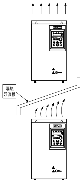
图 2-9 上下安装隔热导流板示意图
