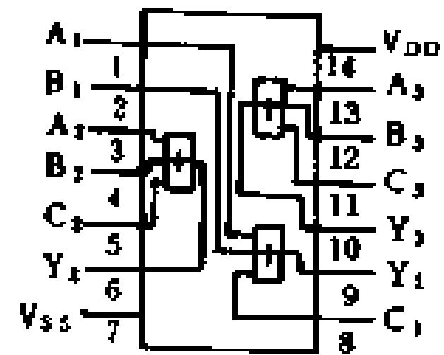
CC4075 三 3 输入或门 Y = A + B + C
