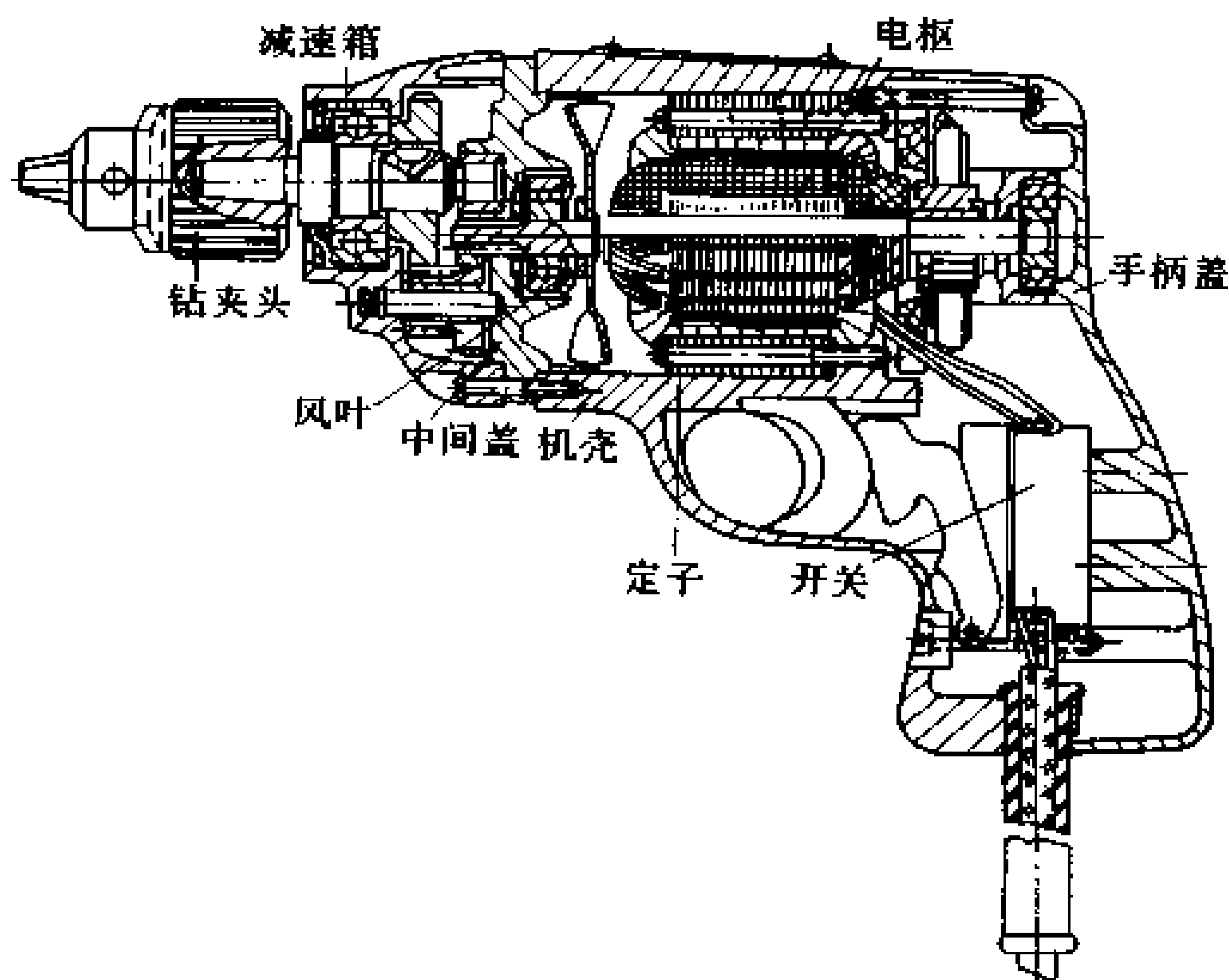
图 12-4 手电钻的结构
