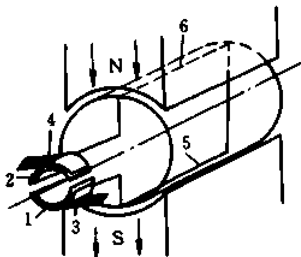
图 6-1 直流发电机原理图
