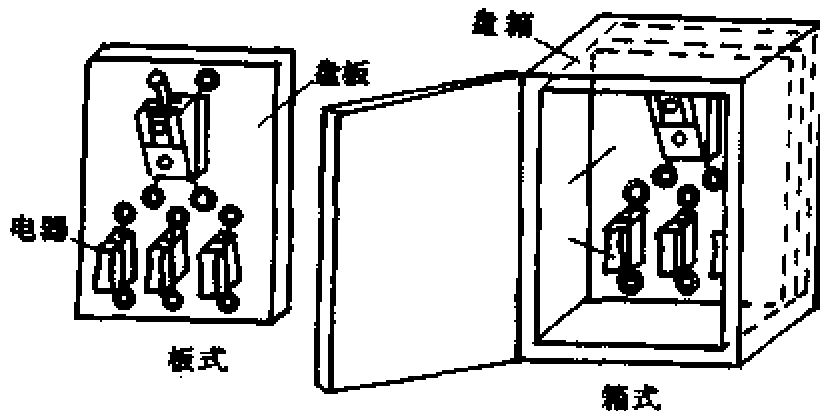
图 10-12 板式和箱式配电盘外形图
