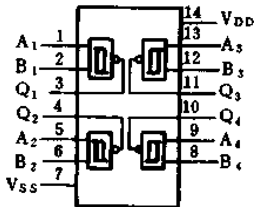
图 3-23 CMOS 电路外引线功能端排列图
