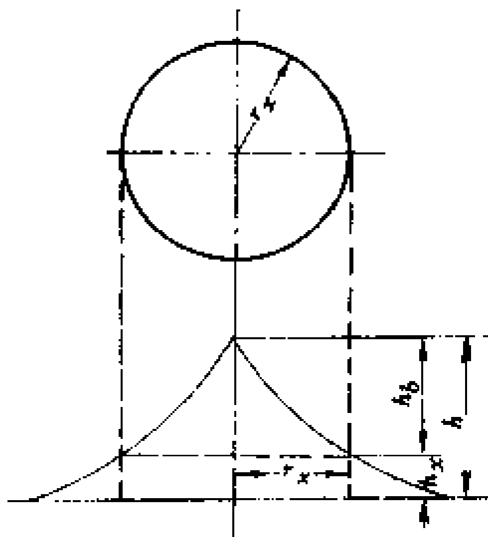
图 1-9 单支避雷针保护范围
