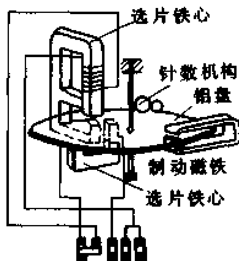
图 2-7 电度表的原理结构图
