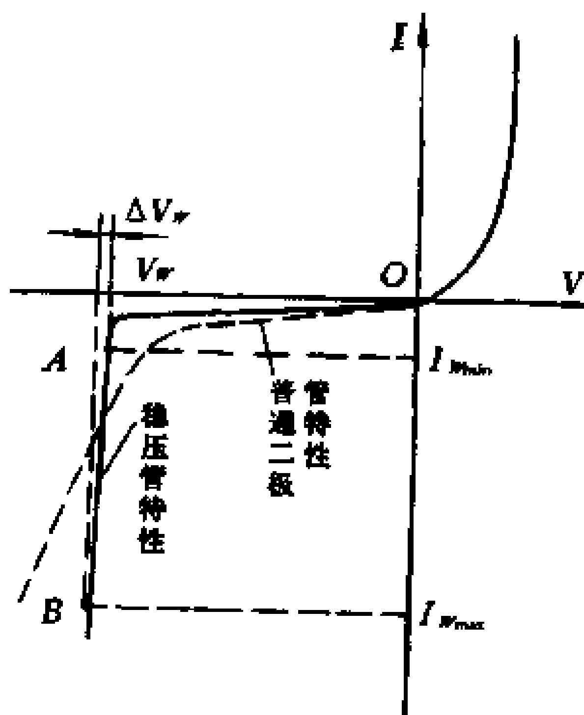
图 3-4 硅稳压二极管伏安特性曲线
