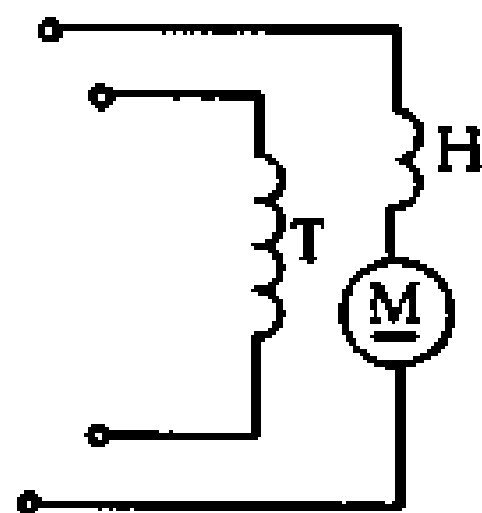
图 6-3 直流电机他励方式原理图
