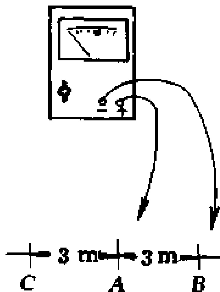
图 1-7 用万用表测量接地电阻简单方法
