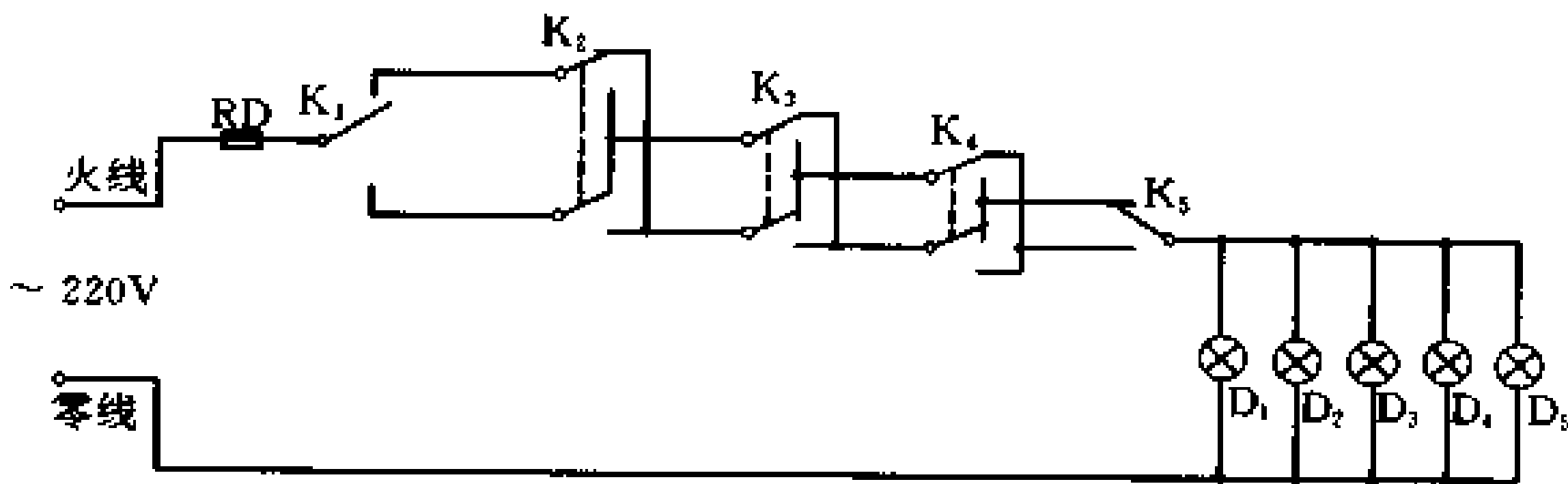
图 10-17 高层楼房走廊照明灯开关控制线路
