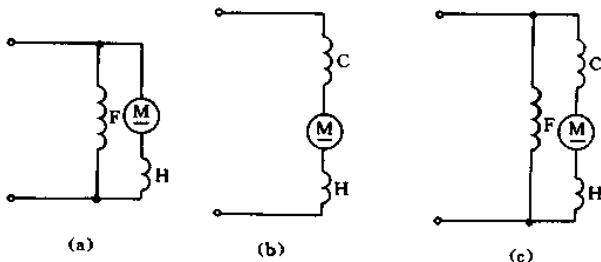
图 6-2 直流电机自励方式原理图
