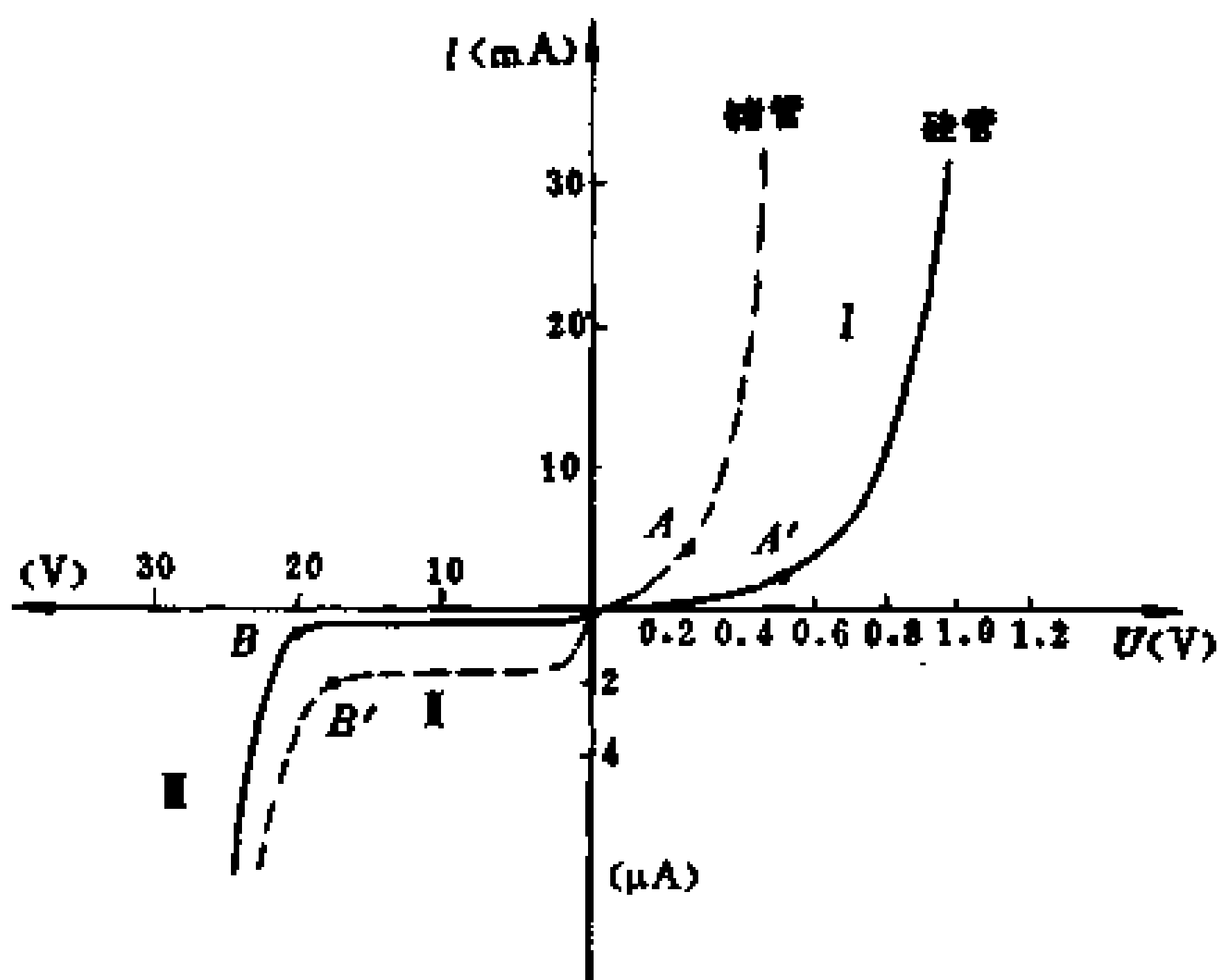
图 3-2 晶体二极管伏安特性曲线
