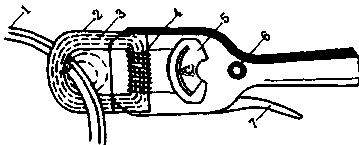
图 2-10 钳形表的结构图
