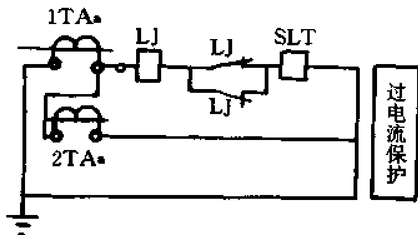
图 1-5 二次电流回路展开图
