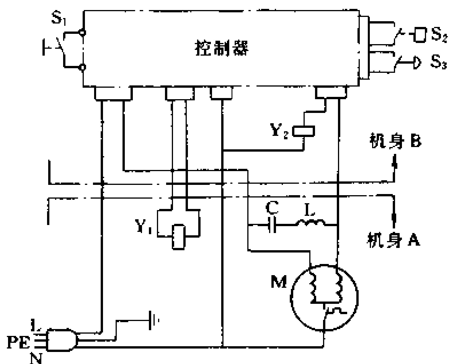
(b) 电脑程序控制器的控制电路
