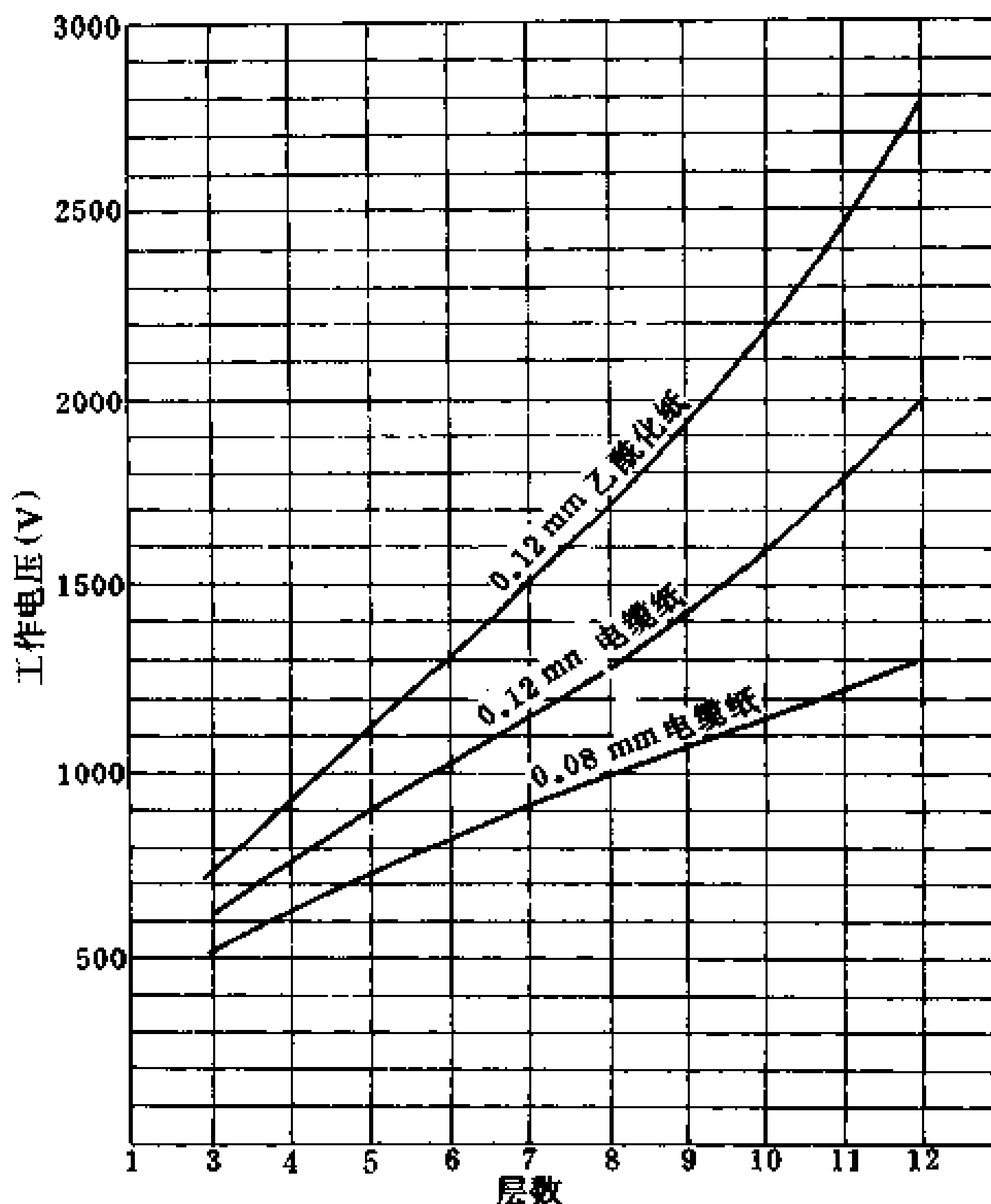
图 8-7 工作电压与线圈层数关系曲线
