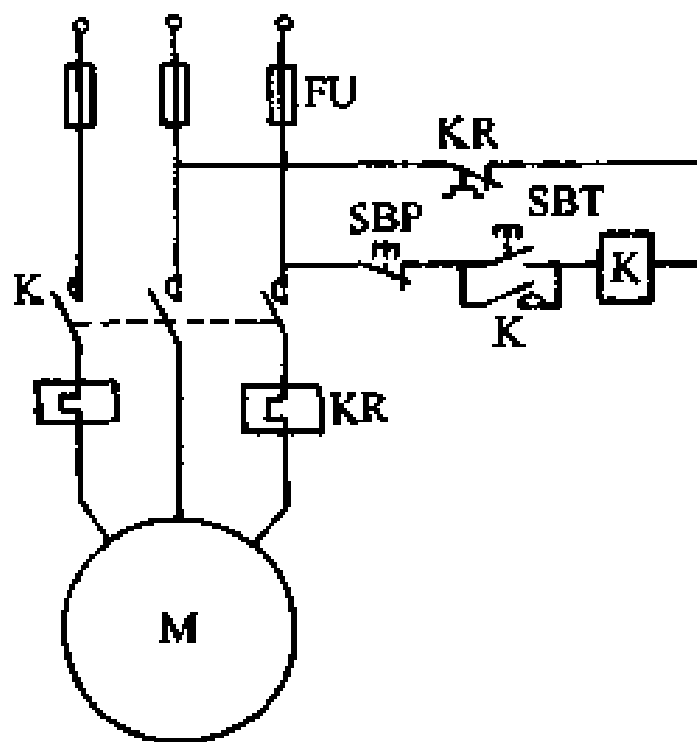
图 5-17 带有热继电器 KR 的保护线路
