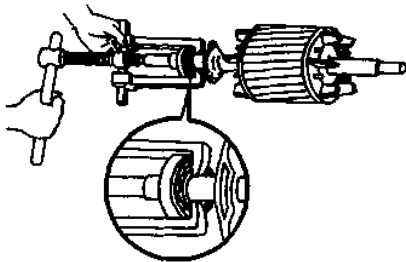
图 5-22 电动机拆装步骤
