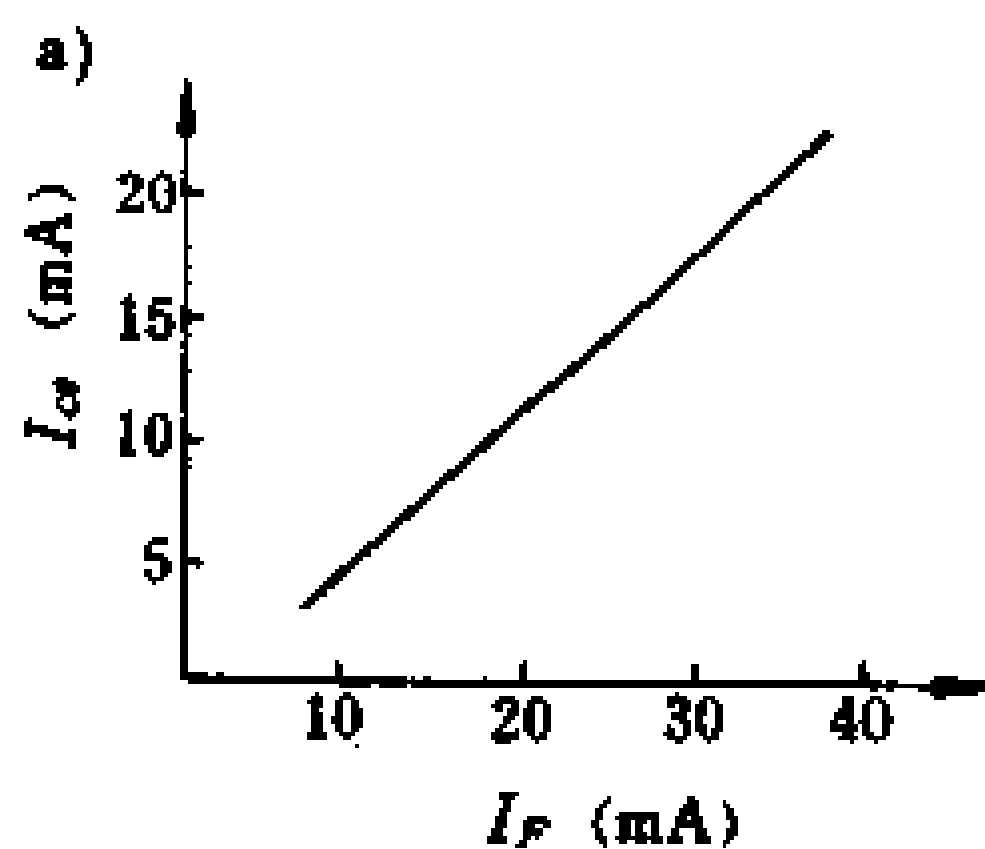
图 3-20 传输特性
