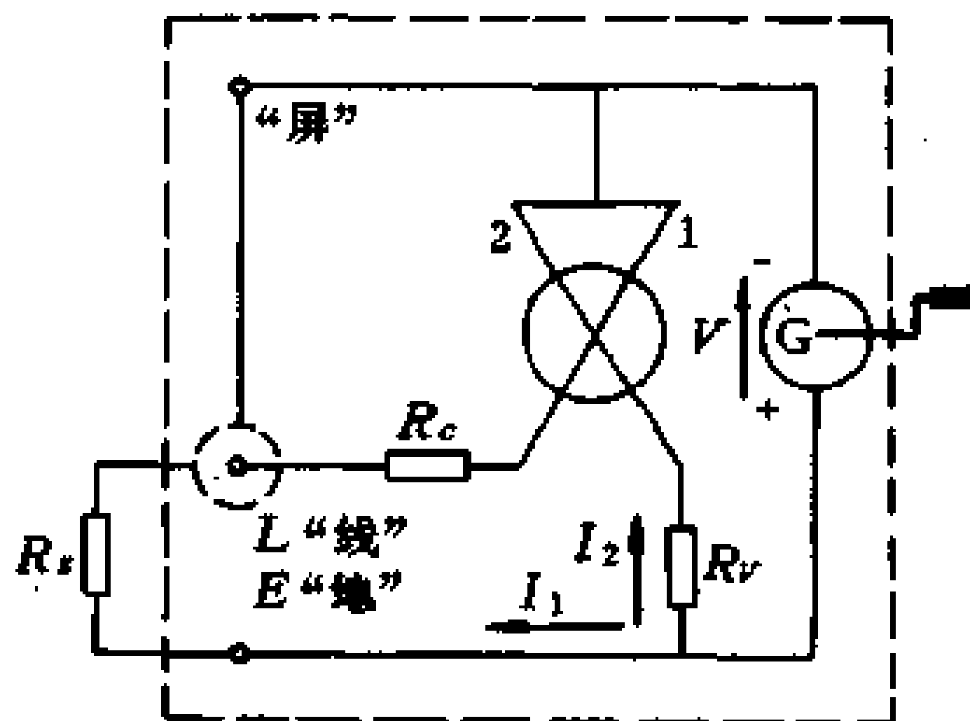
图 2-9 兆欧表工作原理图
