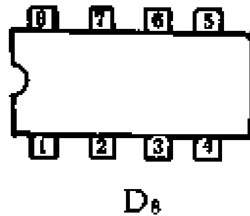
(a) 8 引线金属封装和双列直插封装
