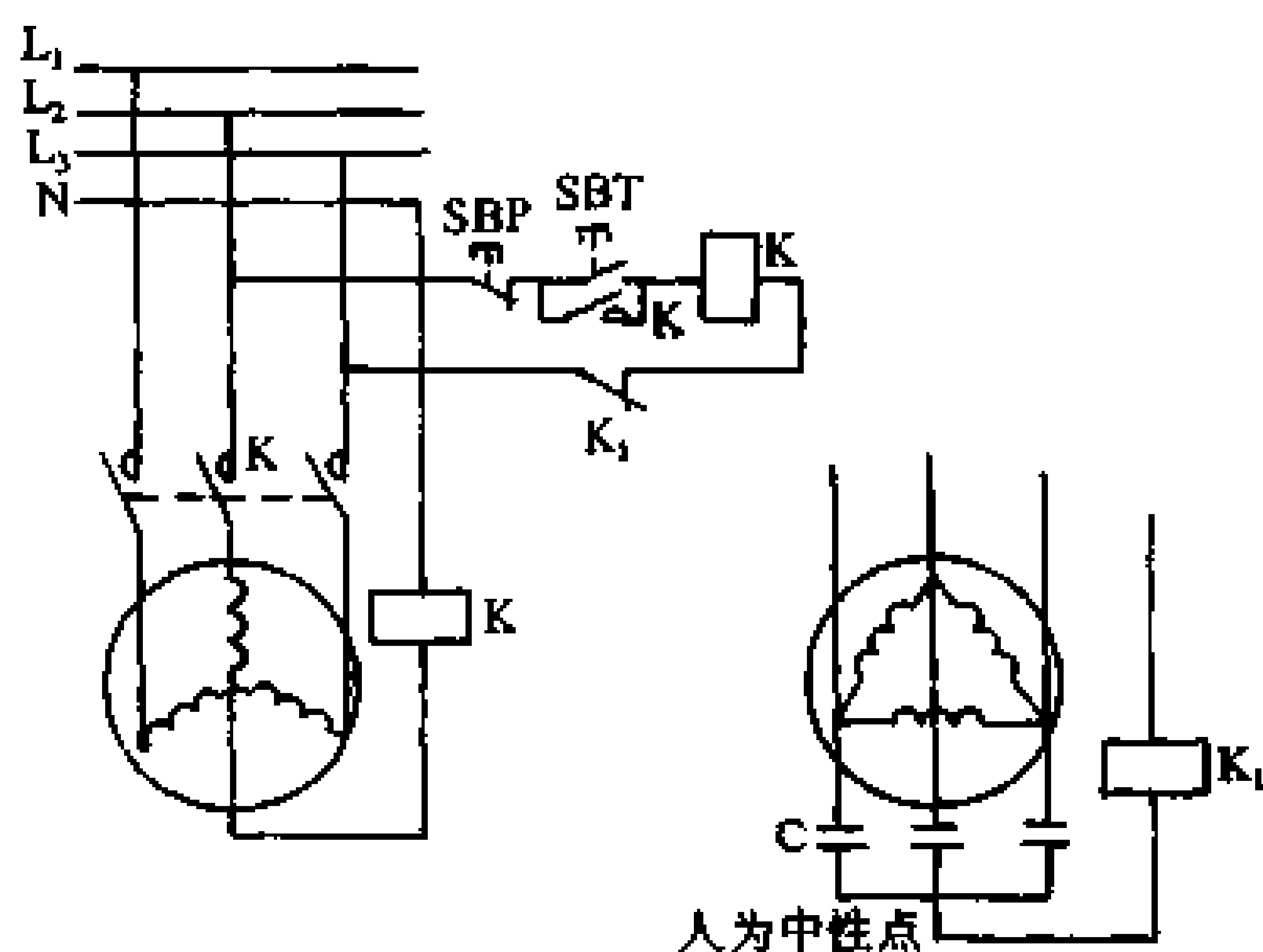
图 5-20 零序电压继电器保护线路
