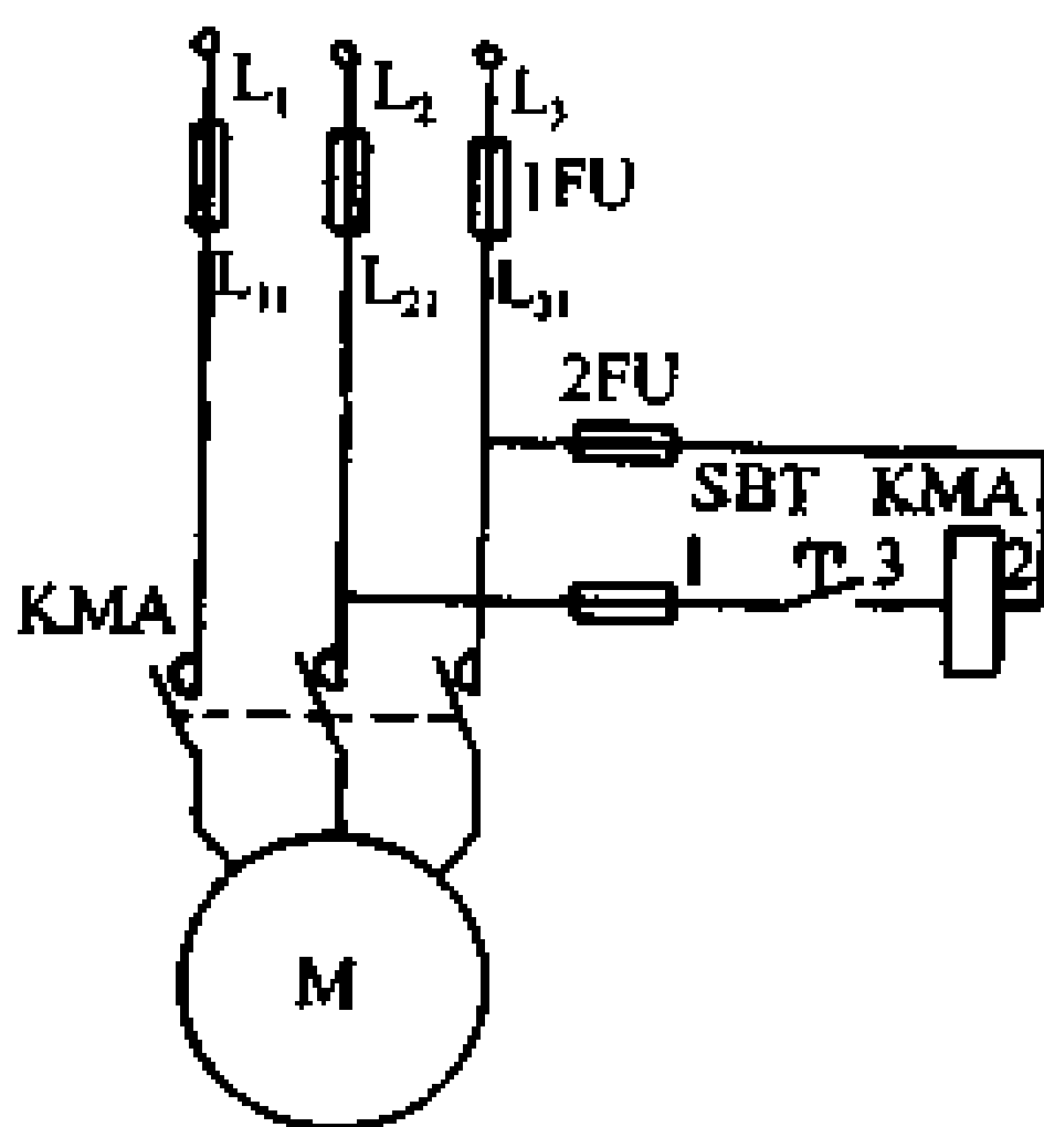
图 5-2 按钮单向点动控制电路
