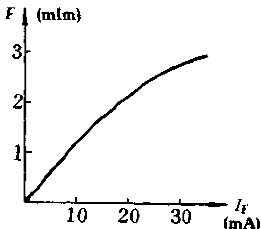
图 3-5 发光二极管电流—亮度特性曲线
