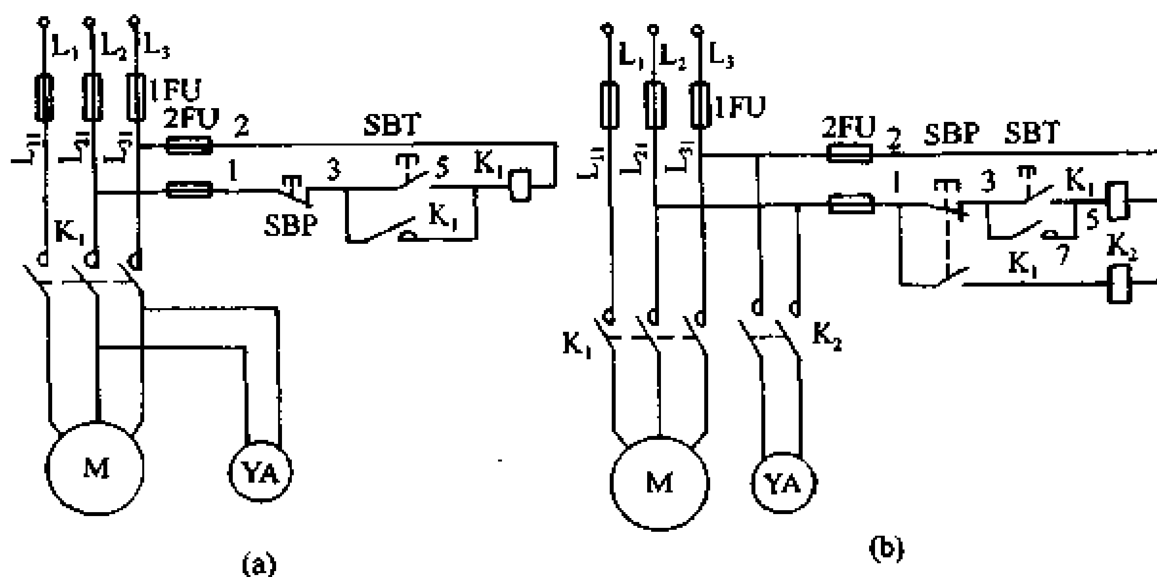
图 5-12 机械制动控制线路
