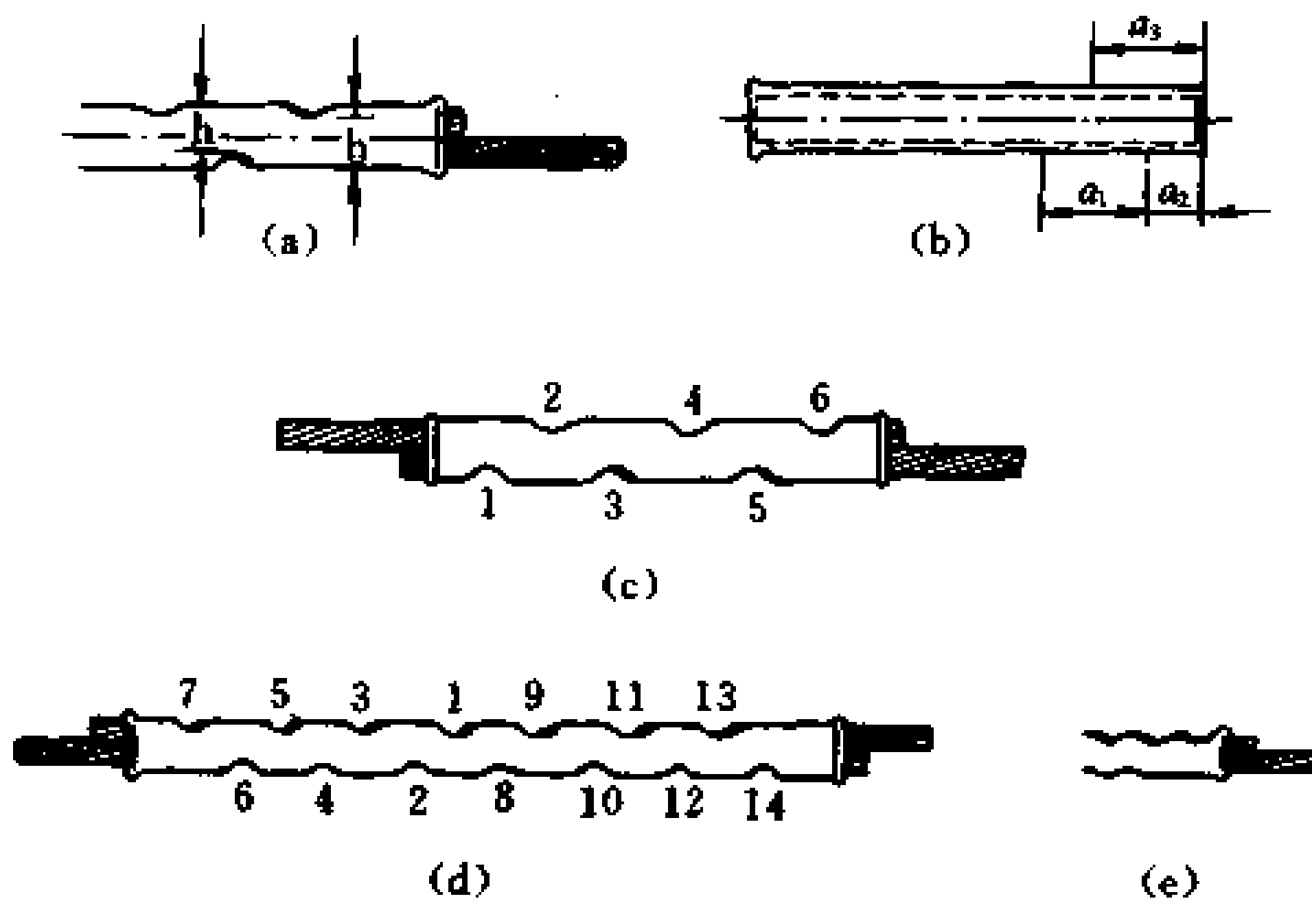
图 10-5 钳接管压坑技术要求
