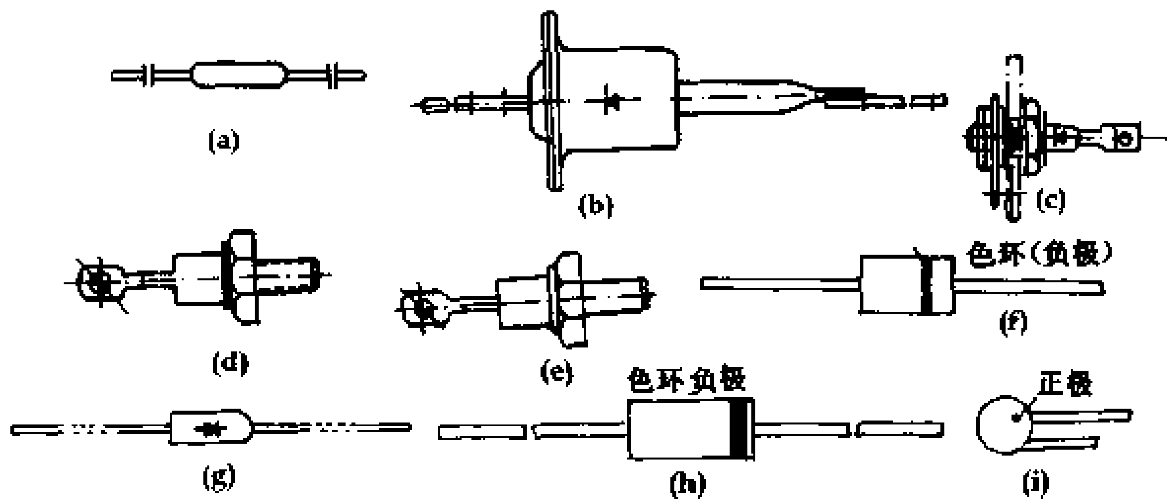
图 3-3 晶体二极管外形图
