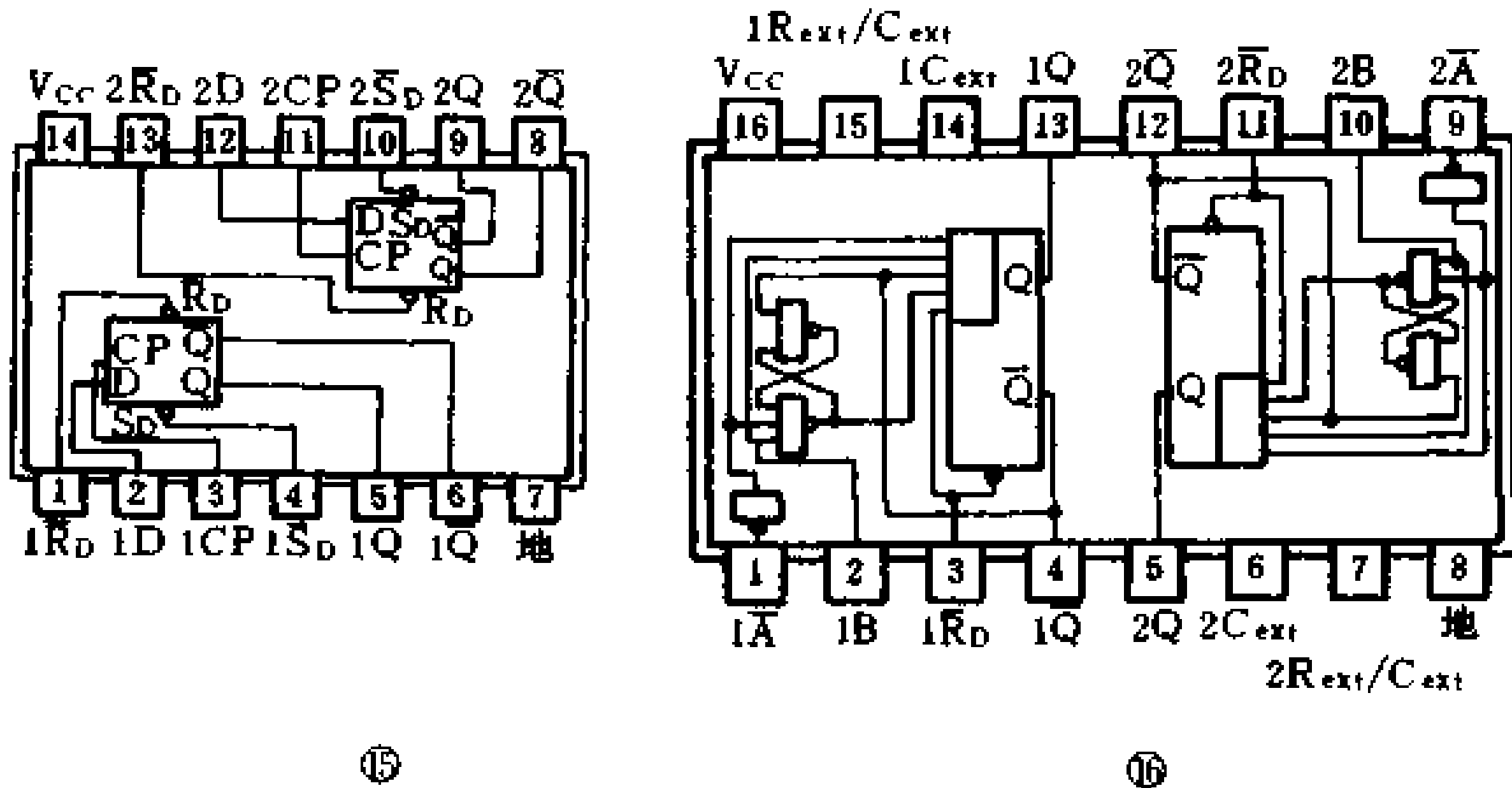
图 3-22 TTL 电路外引线功能端排列图
