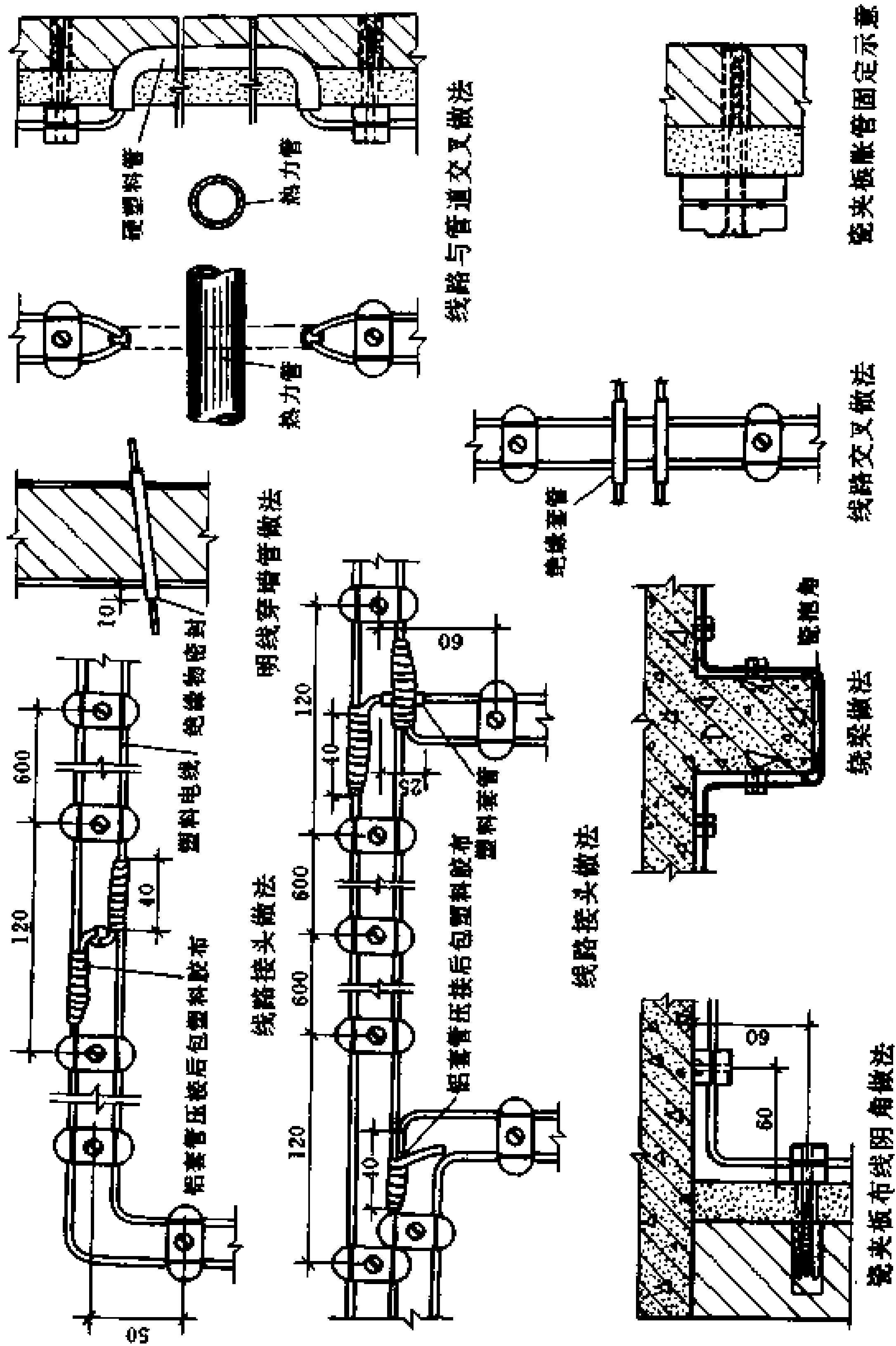
图 10-9 瓷夹板布线
