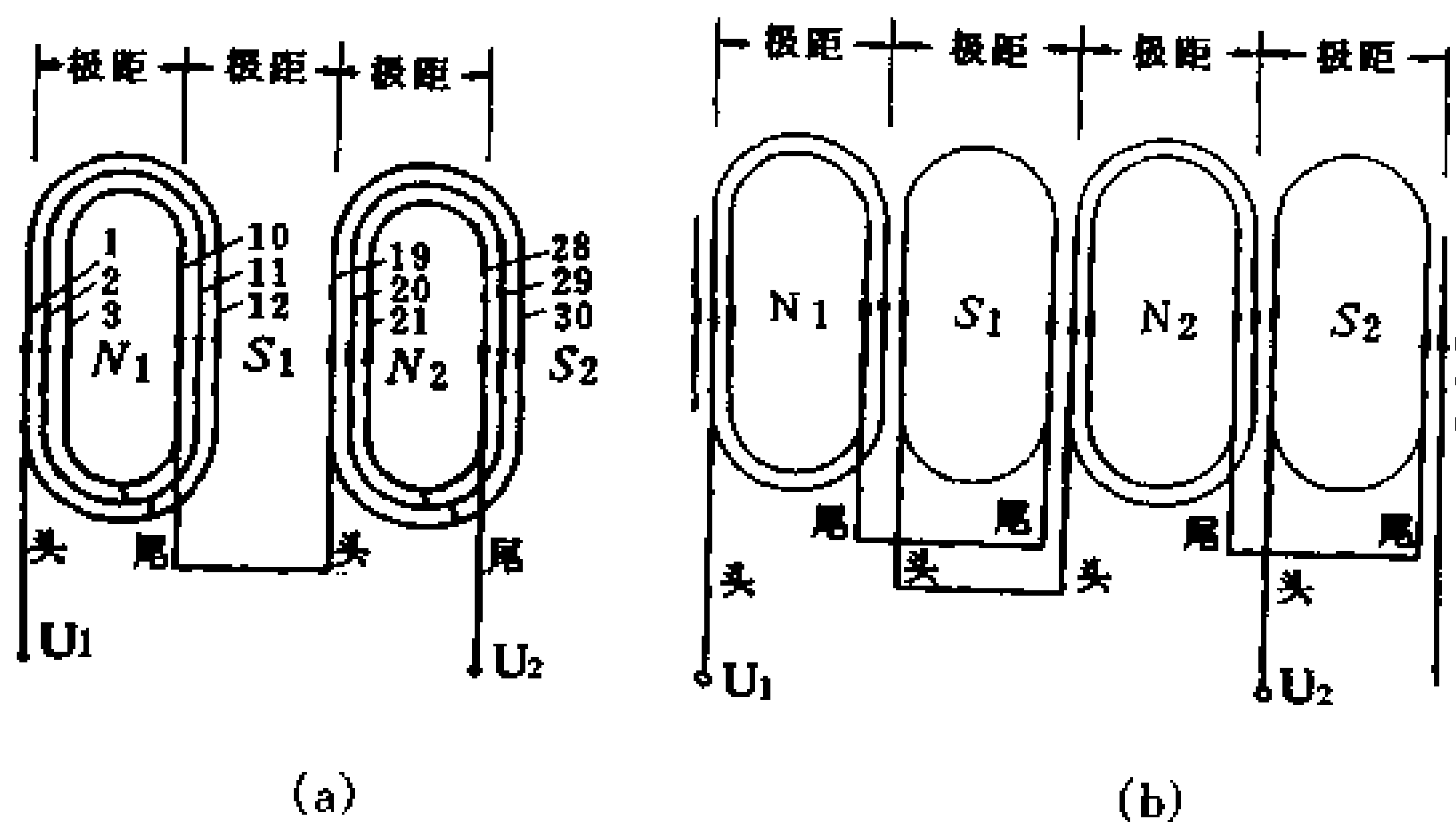
图 5-29 单层绕组的两种形式
