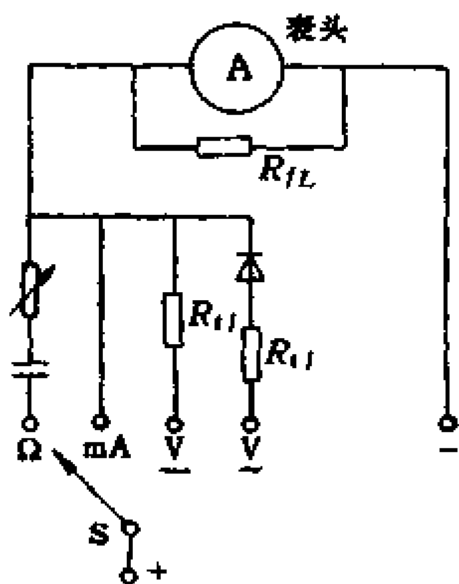
图 2-1 万用表的工作原理简图
