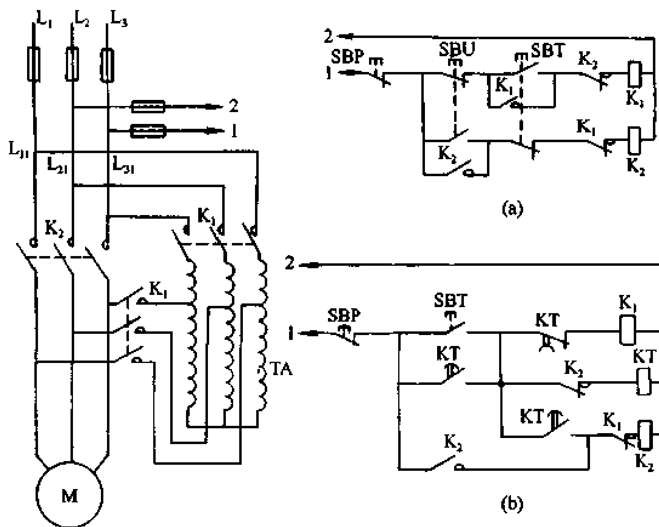
图 5-9 自耦变压器降压起动电路
