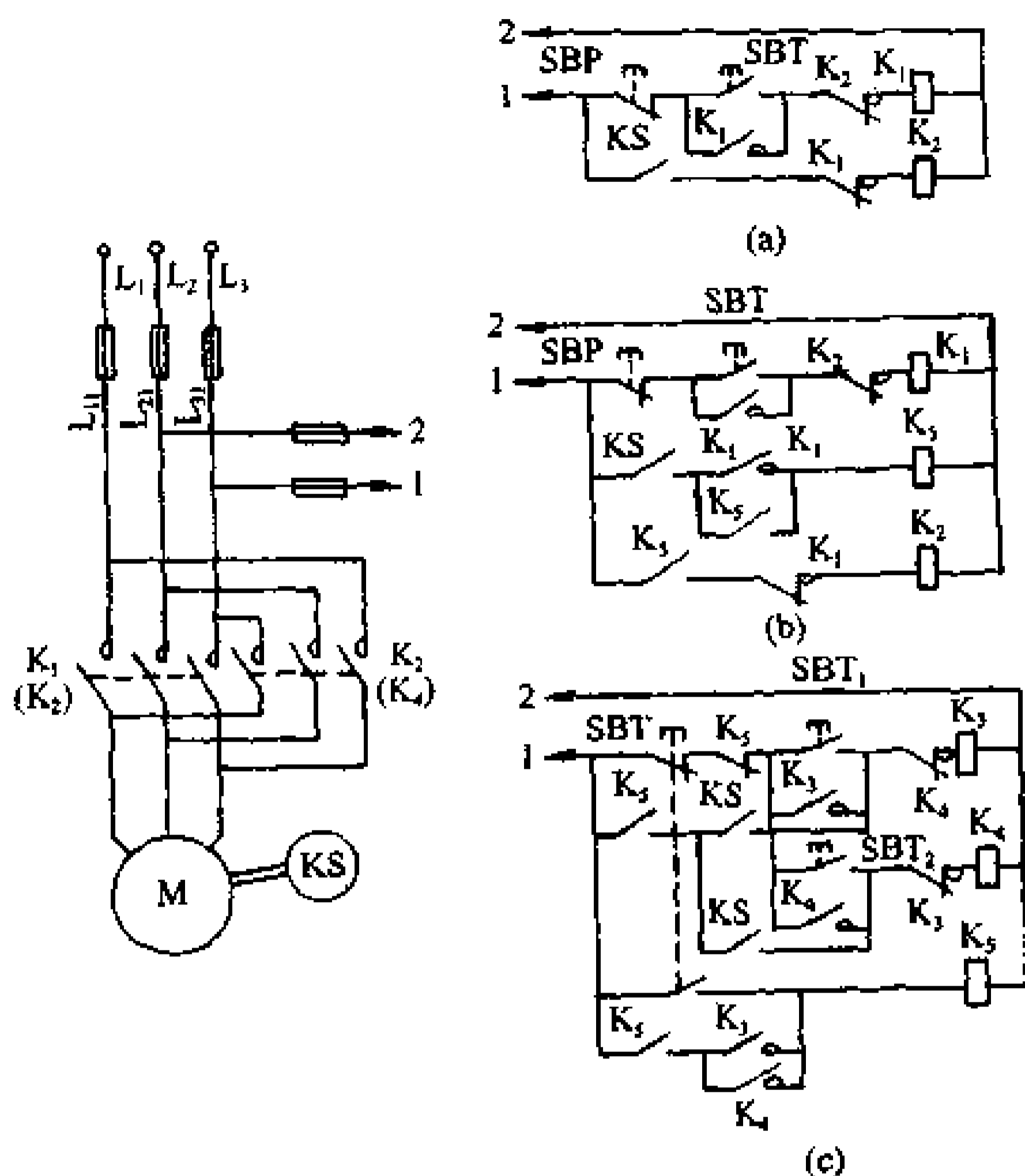
图 5-13 反接制动控制线路
