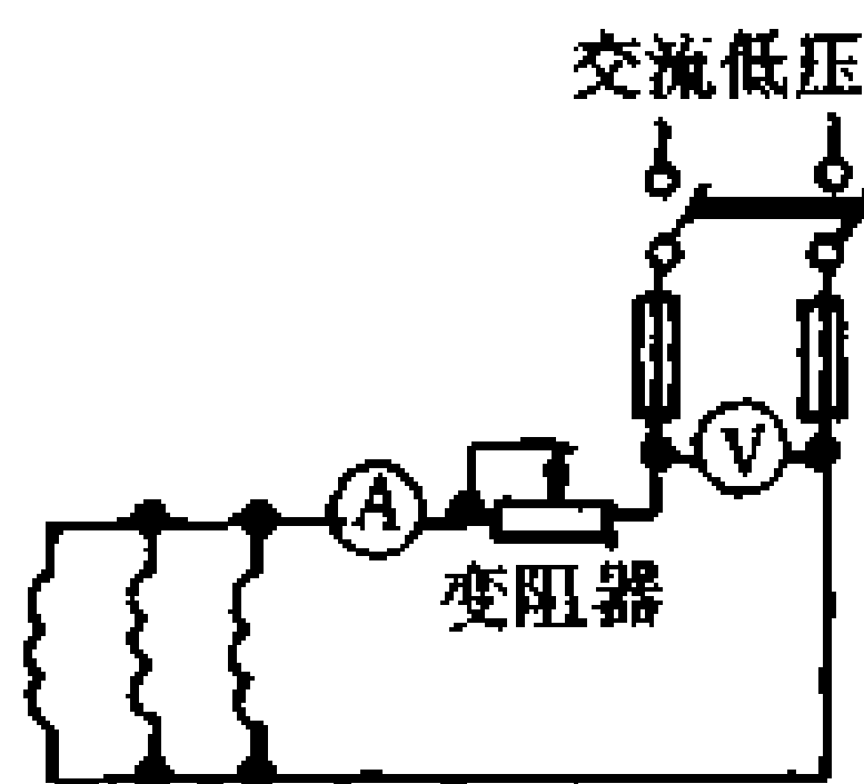
图 5-34 绕组并联干燥法
