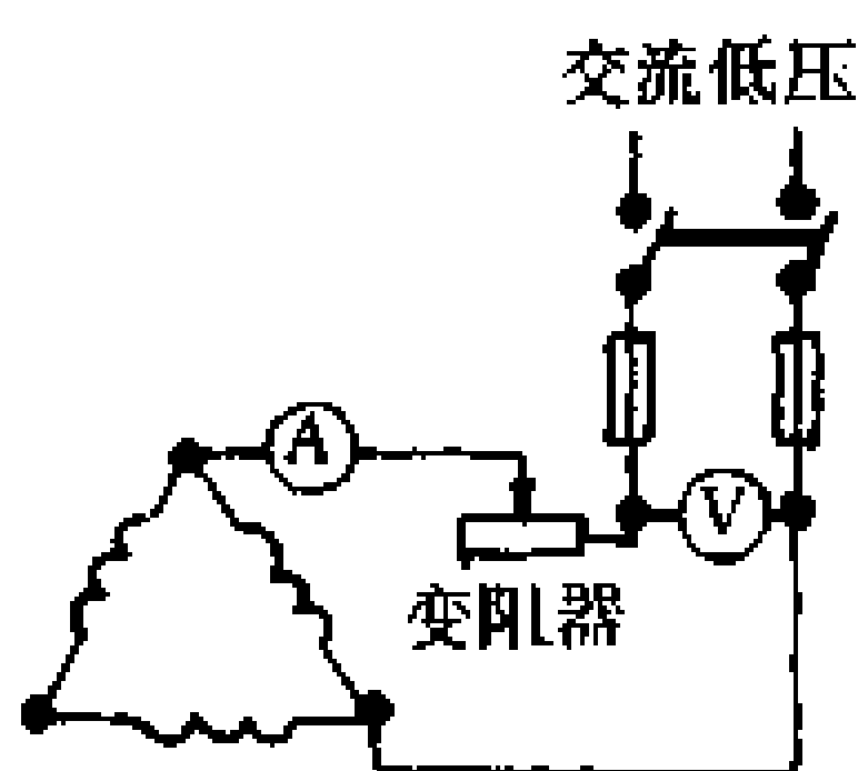
图 5-33 绕组串、并联干燥法
