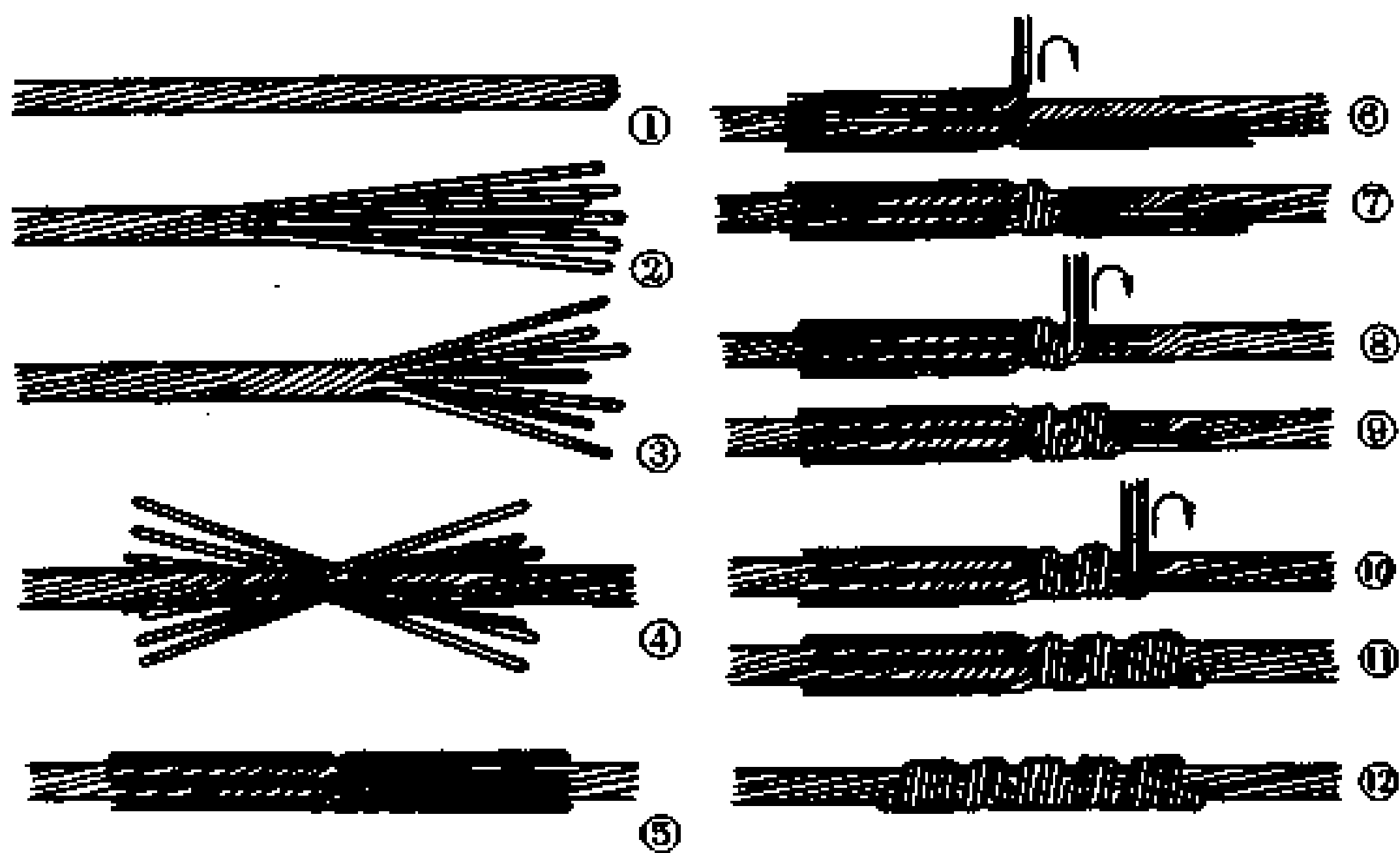
图 10-6 铝绞线的缠绕连接法
