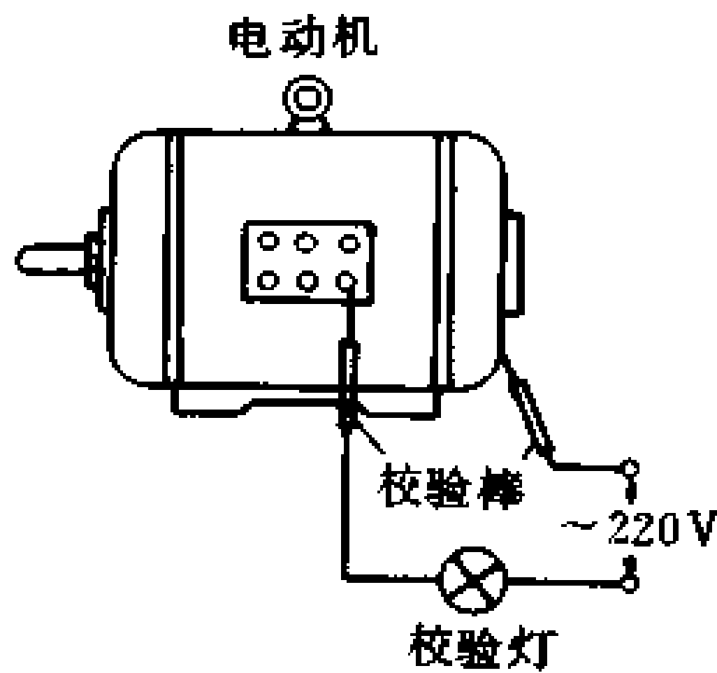
图 5-26 检查定子绕组接地的方法
