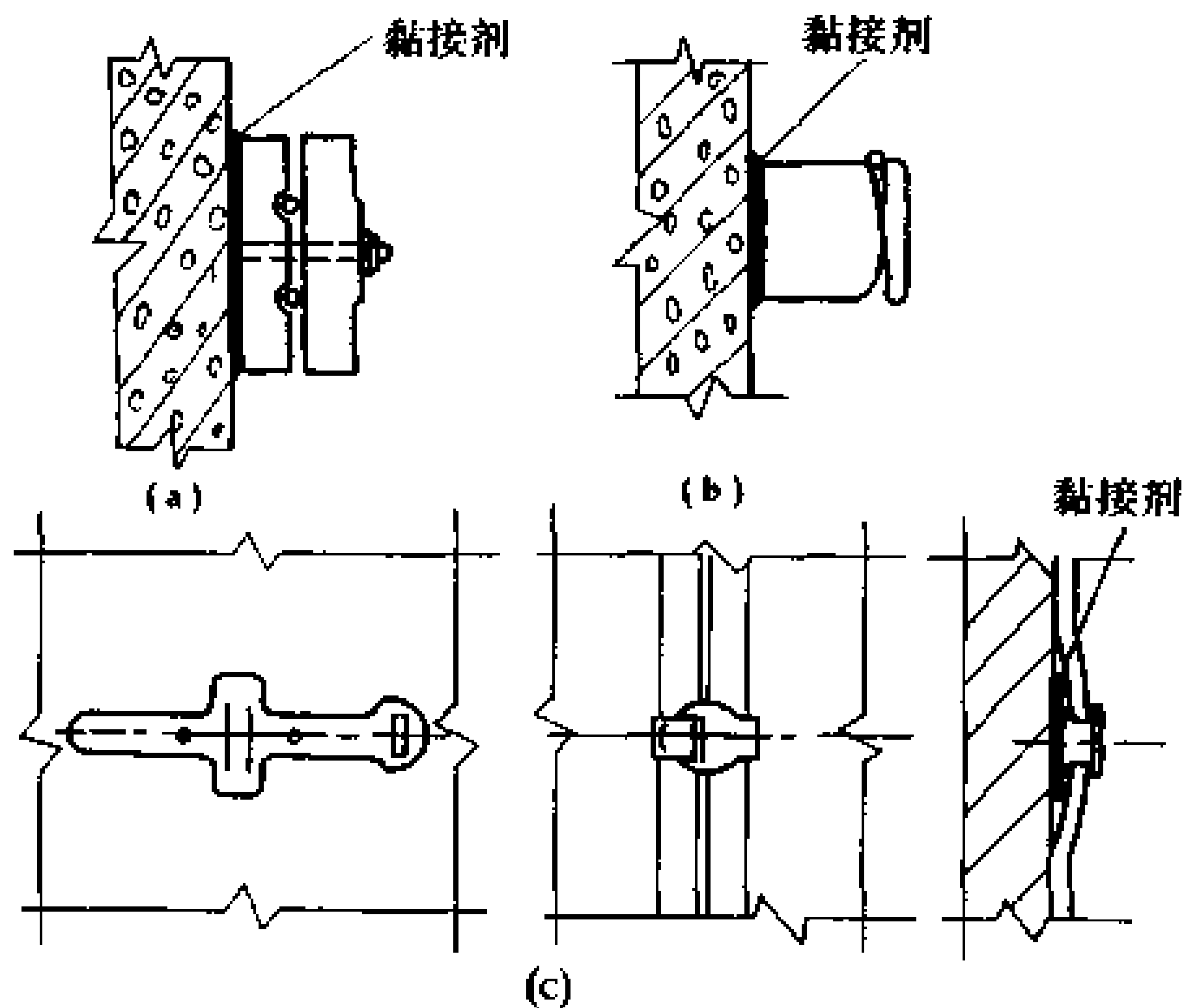
图 10-8 线夹、瓷瓶和铝片卡黏接 (a) 线夹 (b) 瓷瓶 (c) 铝片卡
