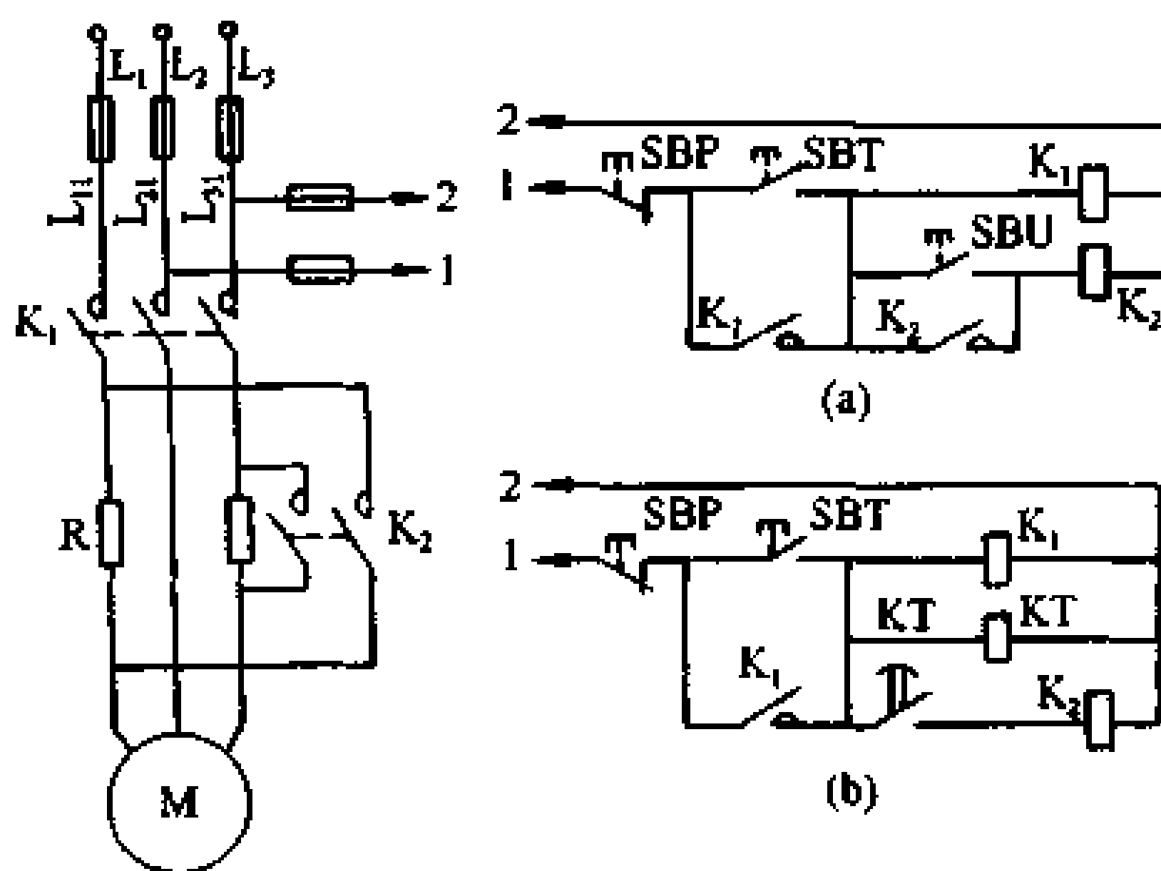
图 5-8 电阻降压起动电路
