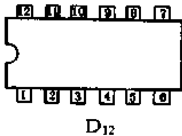
(c) 12 引线金属封装和双列直插封装
