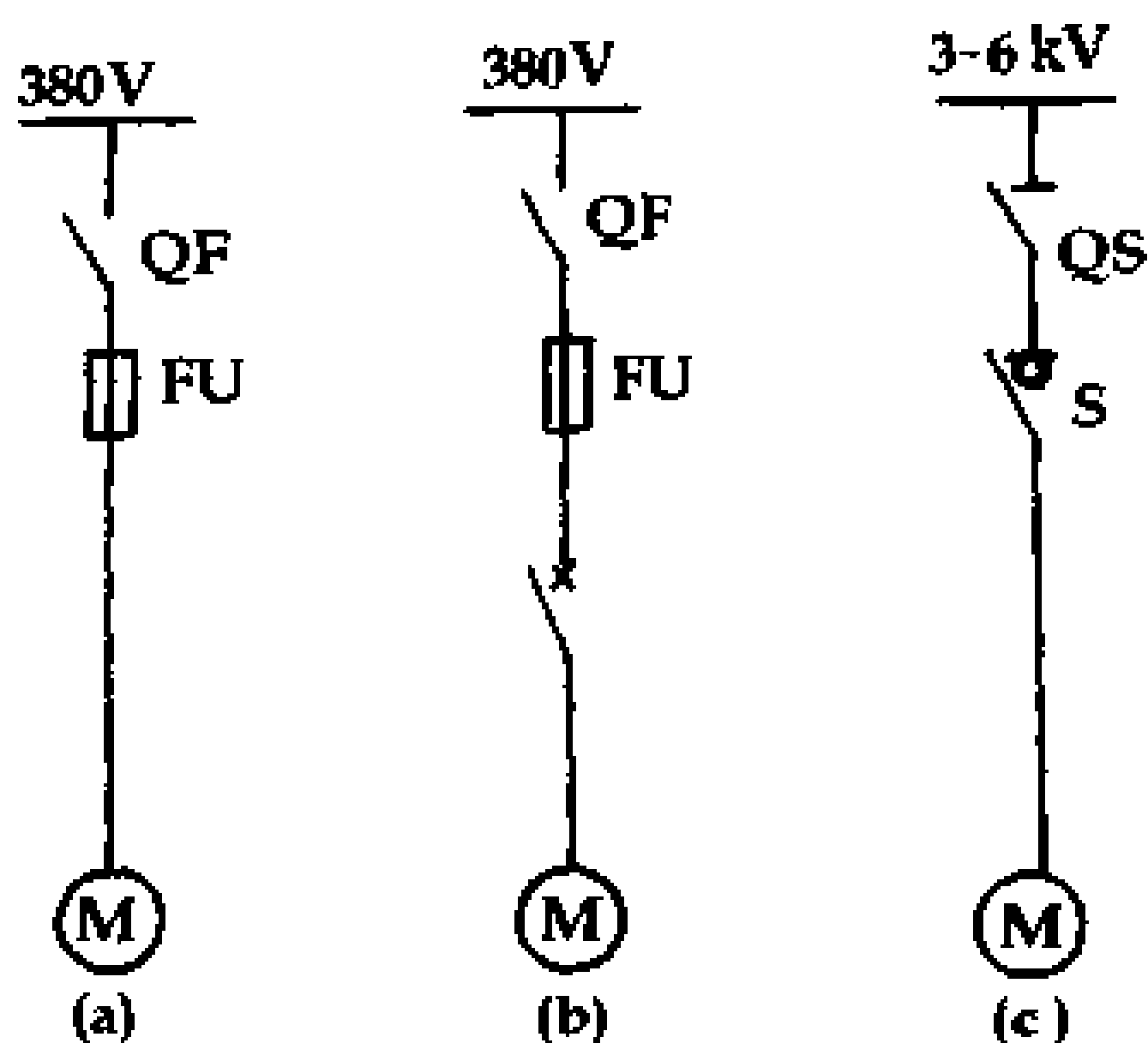
图 1-6 电动机系统图
