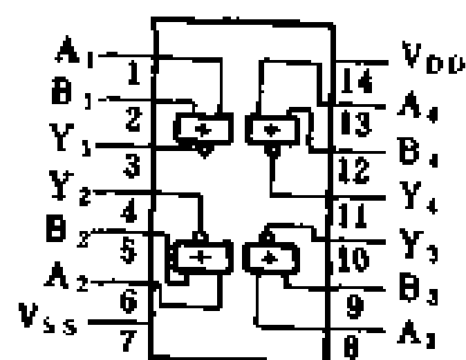
CC4001 四 2 输入或非门 Y = \overline{A + B}
