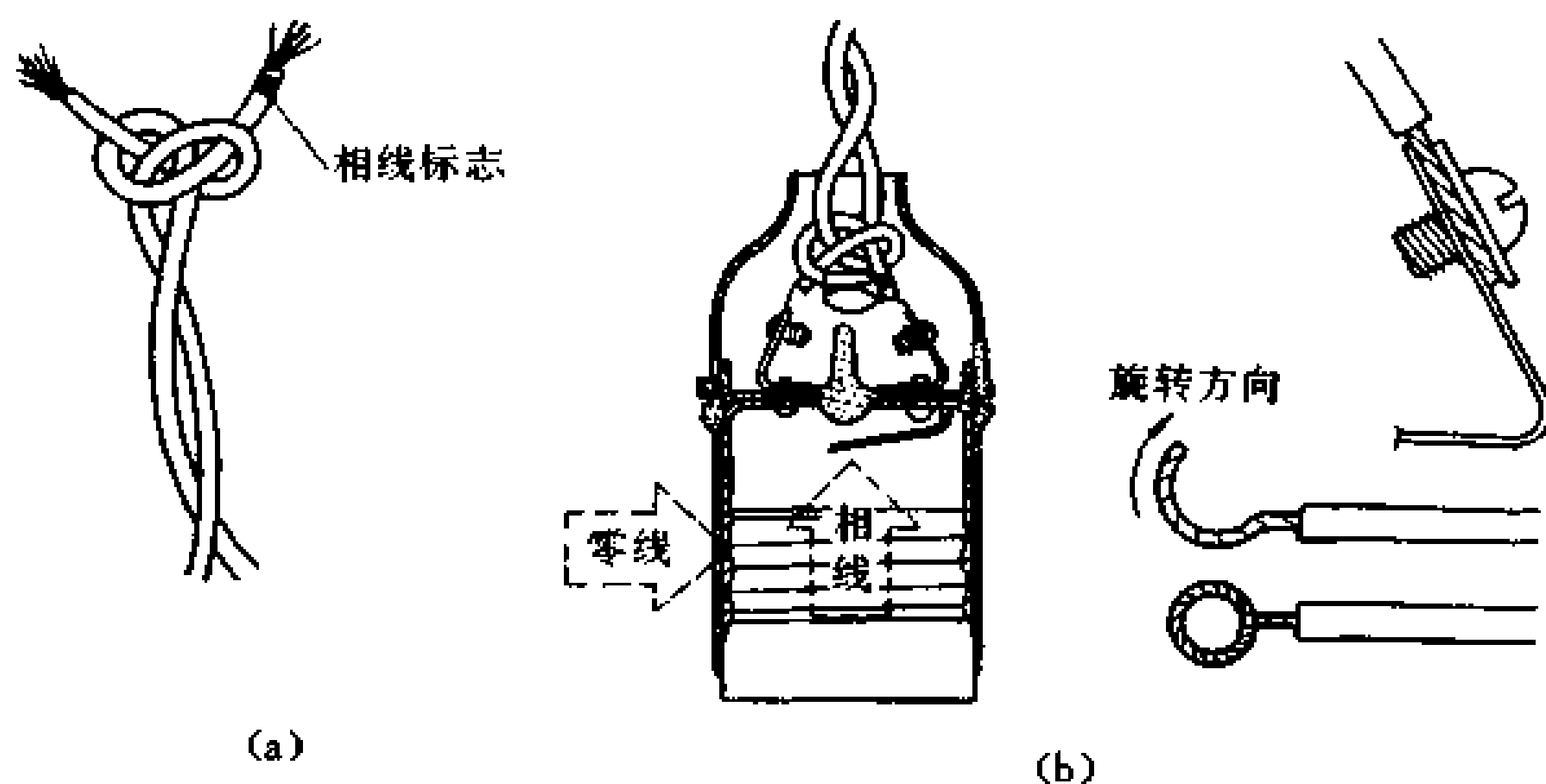
图 10-16 导线结扣、灯头接线及导线连接法
