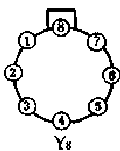
(a) 8 引线金属封装和双列直插封装
