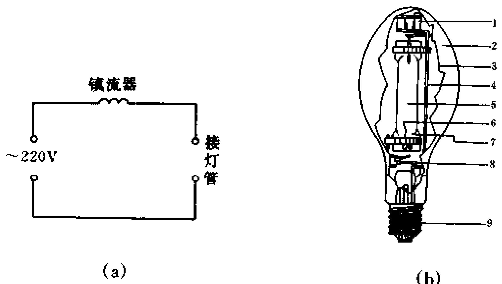
图 11-6 高压汞灯结构与接线图
