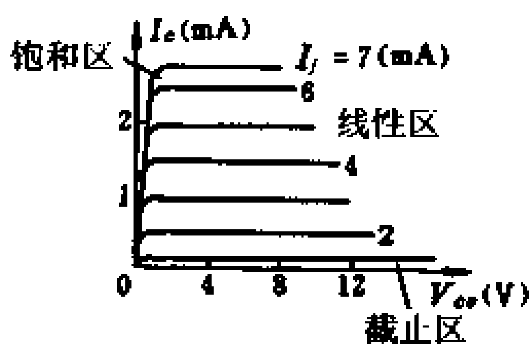
图 3-19 输出特性
