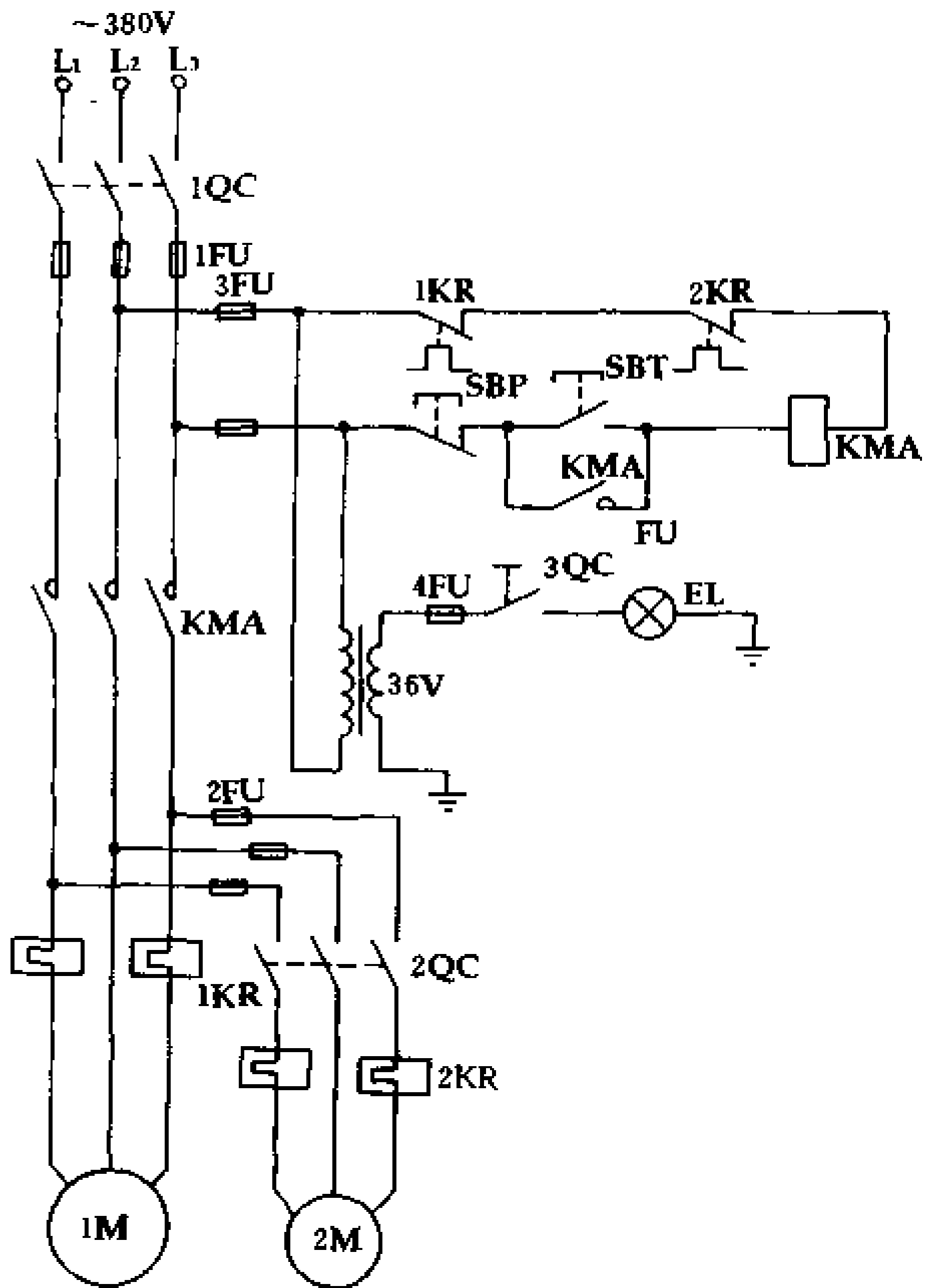
图 12-1 C620 型普通机床的控制电路图
