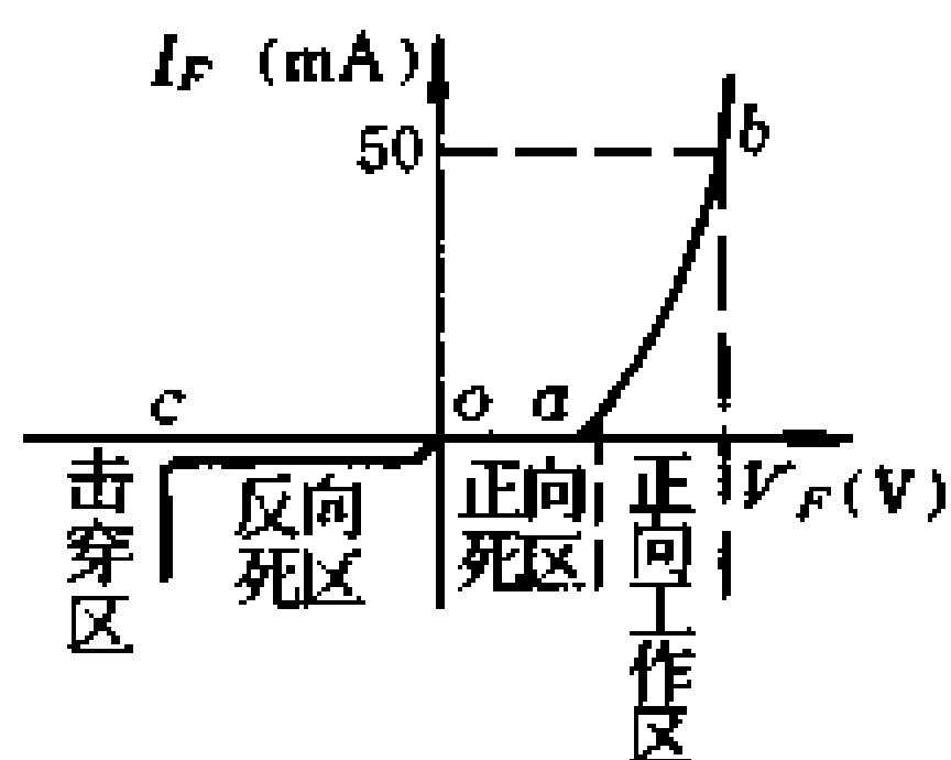
图 3-18 输入特性
