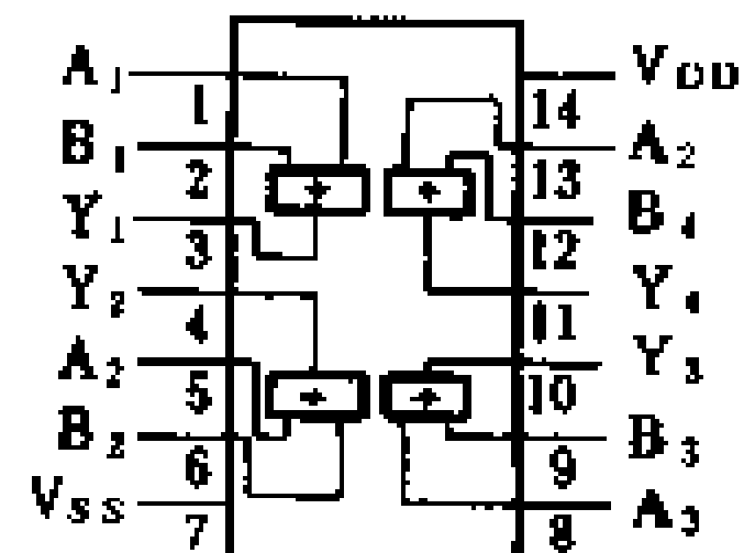
CC4071 四 2 输入或门 Y = A + B
