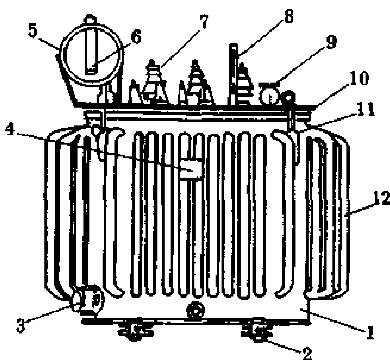
图 8-4 电力变压器的组成
