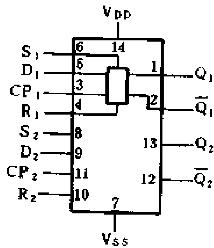
CC4013 双上升沿D触发器
