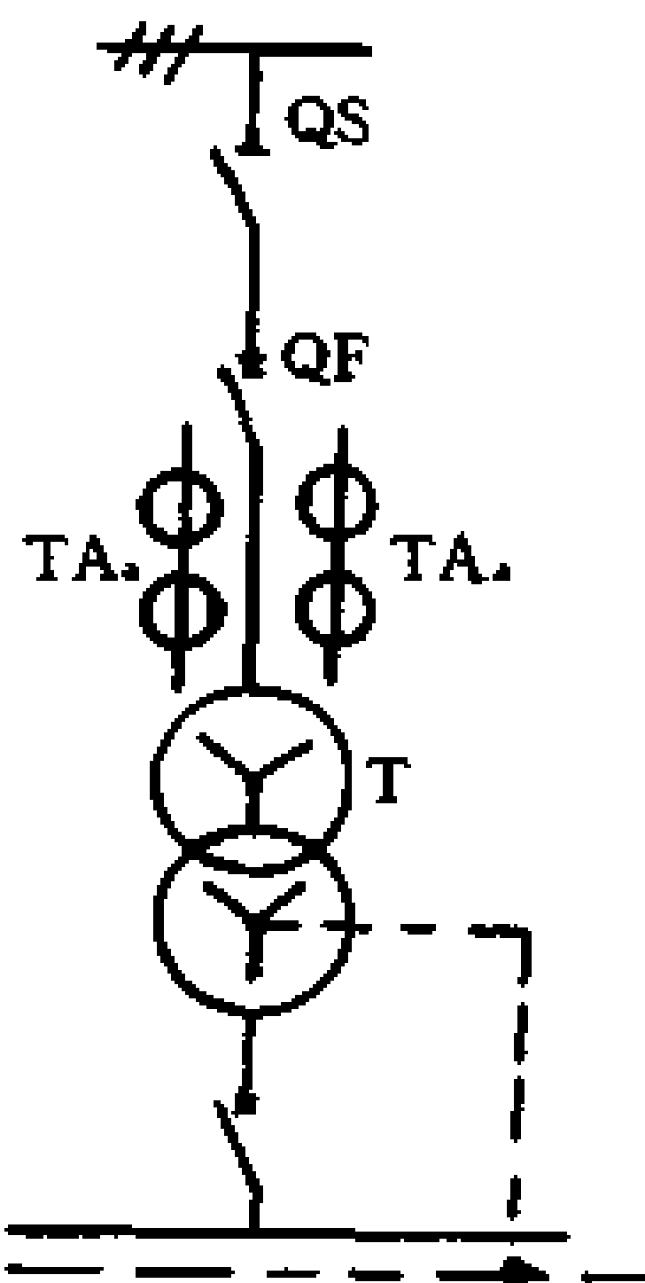
图 1-3 变电所一次回路系统图
