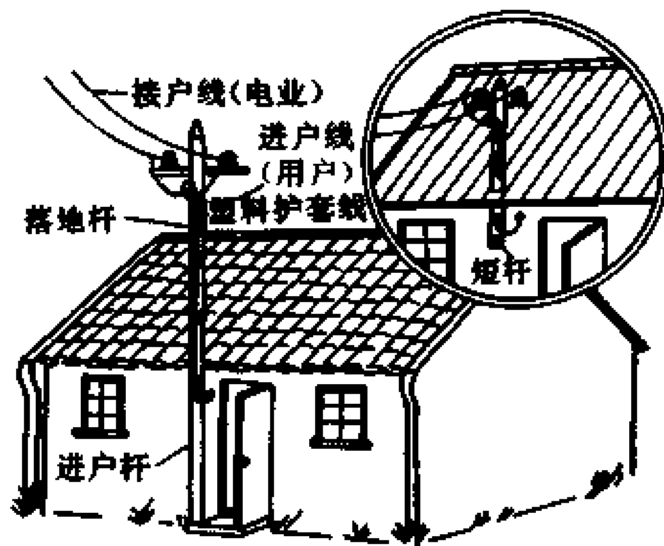
图 10-3 加装进户杆（落地杆或短杆）进户
