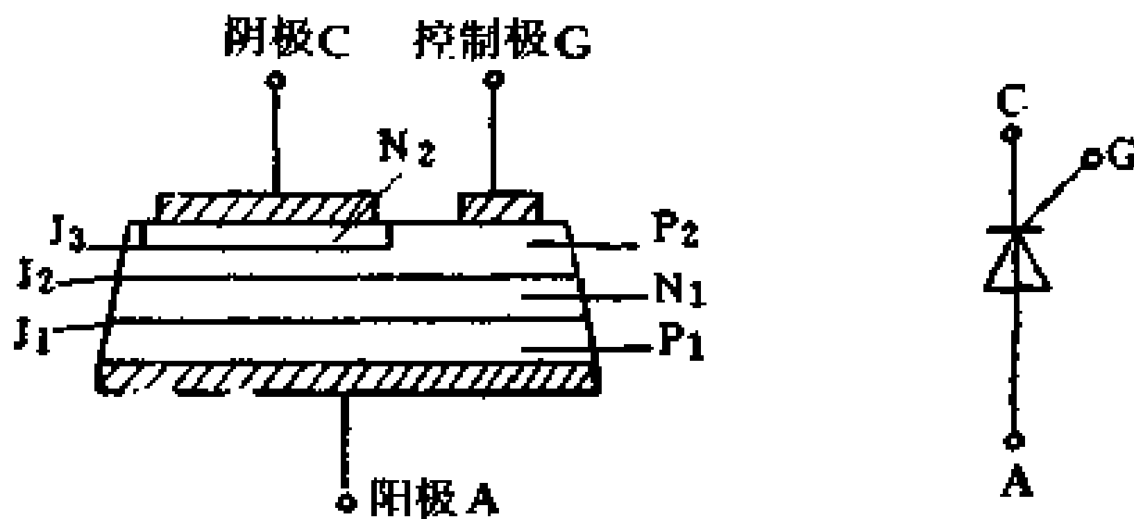
图 3-16 晶闸管的内部结构及其符号
