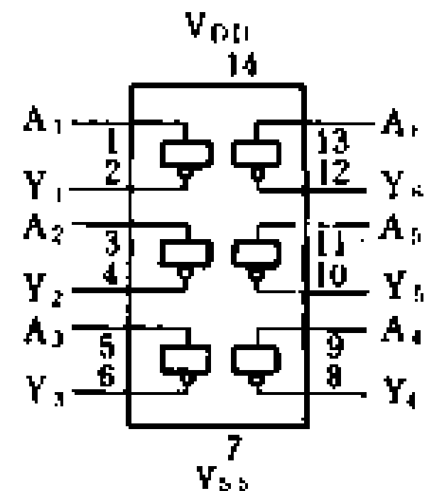
CC4069 六反相器 Y = \overline{A}
