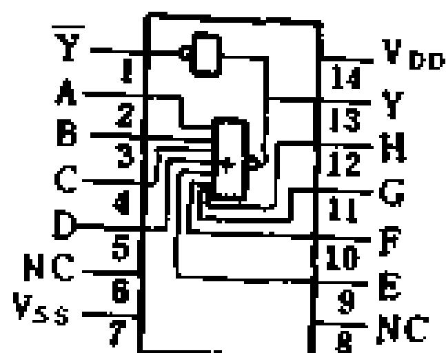
CC4078 8 输入或非/或门 Y = \overline{A + B + C + D + E + F + G + H} Y = A + B + C + D + E + F + G + H
