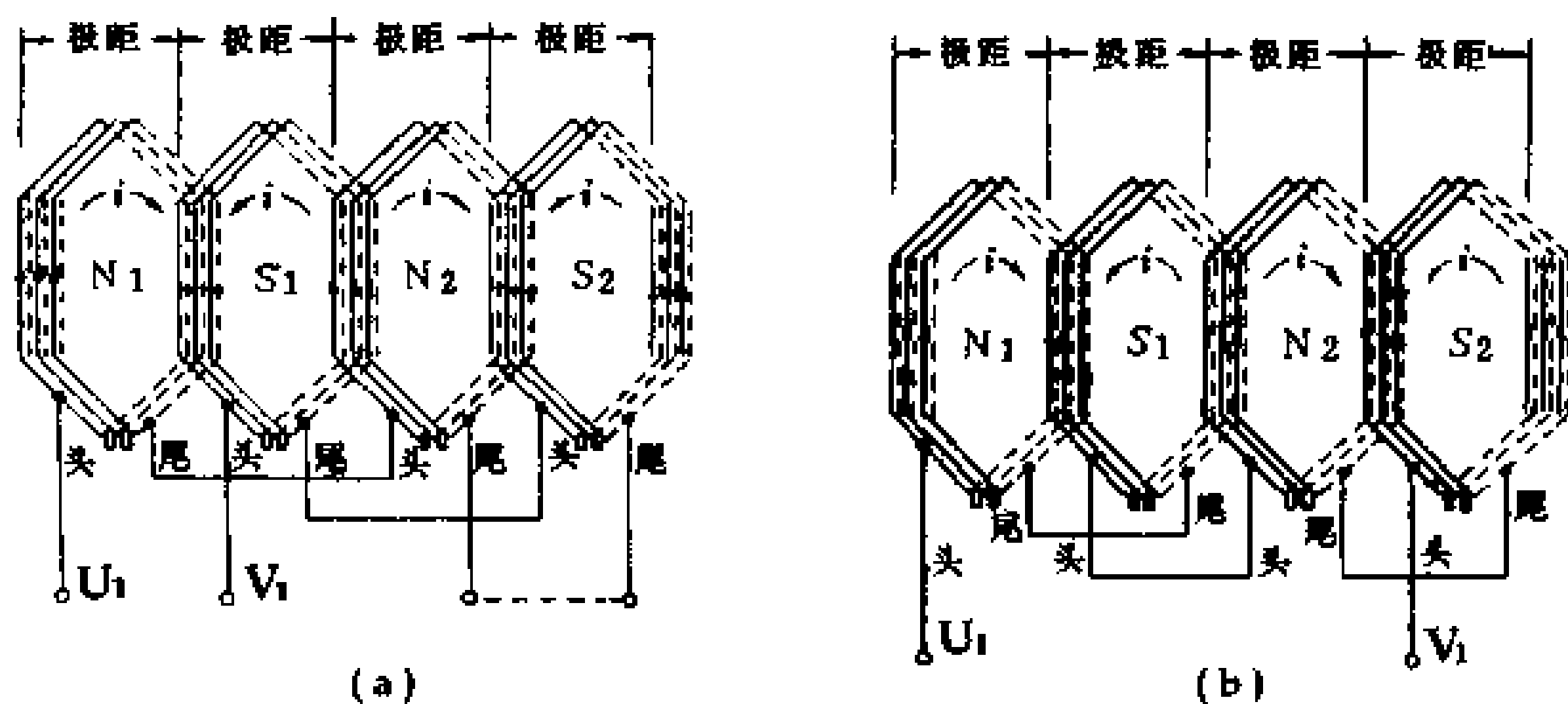
图 5-30 双层绕组的“正、反串”接法
