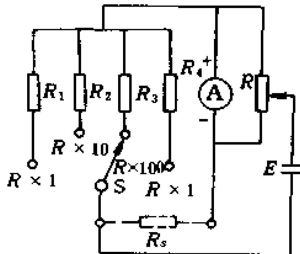
图 2-5 万用表测量电阻的实际线路
