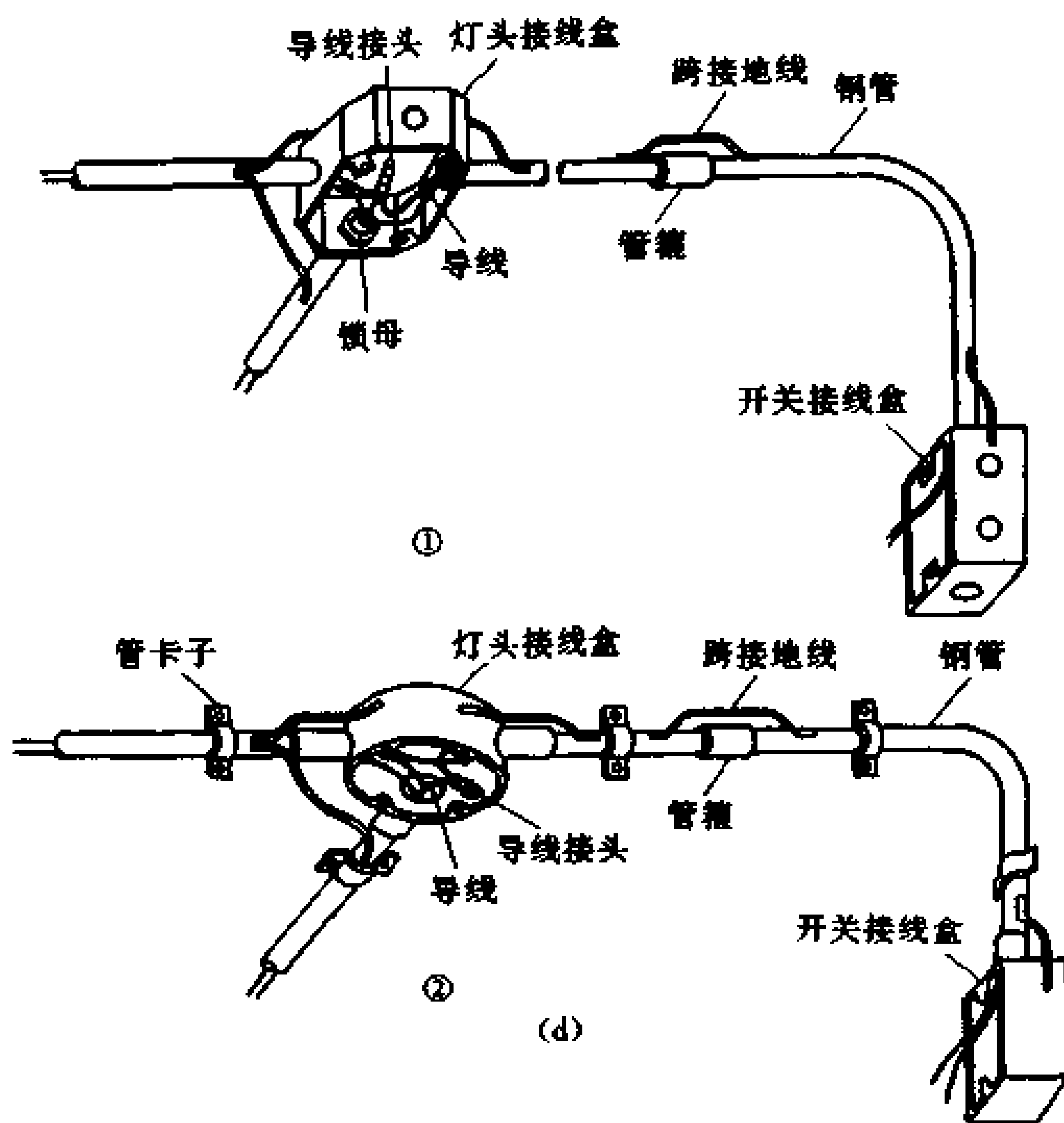
图 10-10 聚乙烯电线管和钢管暗布线 (a) 电线管的节点 (b) 暗布线示例 (1, 2, 3, 4) (c) 明、暗布线接线盒 (d) 钢管布线
