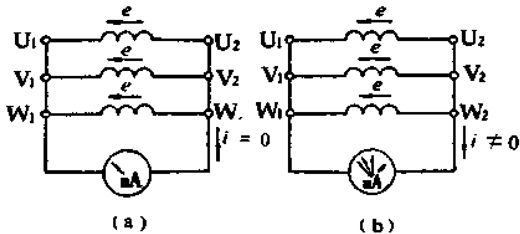
图 5-28 用万用表检查三相绕组连接 (a) 指针不动, 头尾连接正确 (b) 指针摆动, 头尾连接错误
