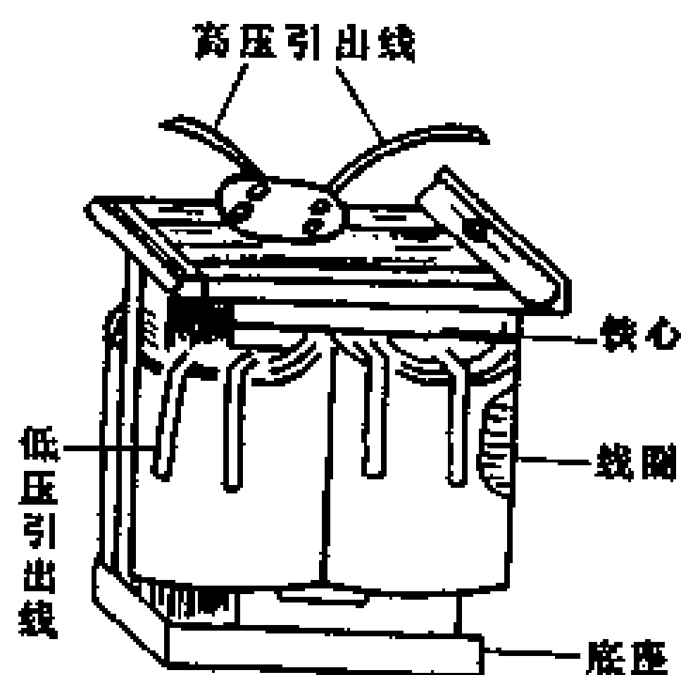
图 8-3 小功率变压器的组成
