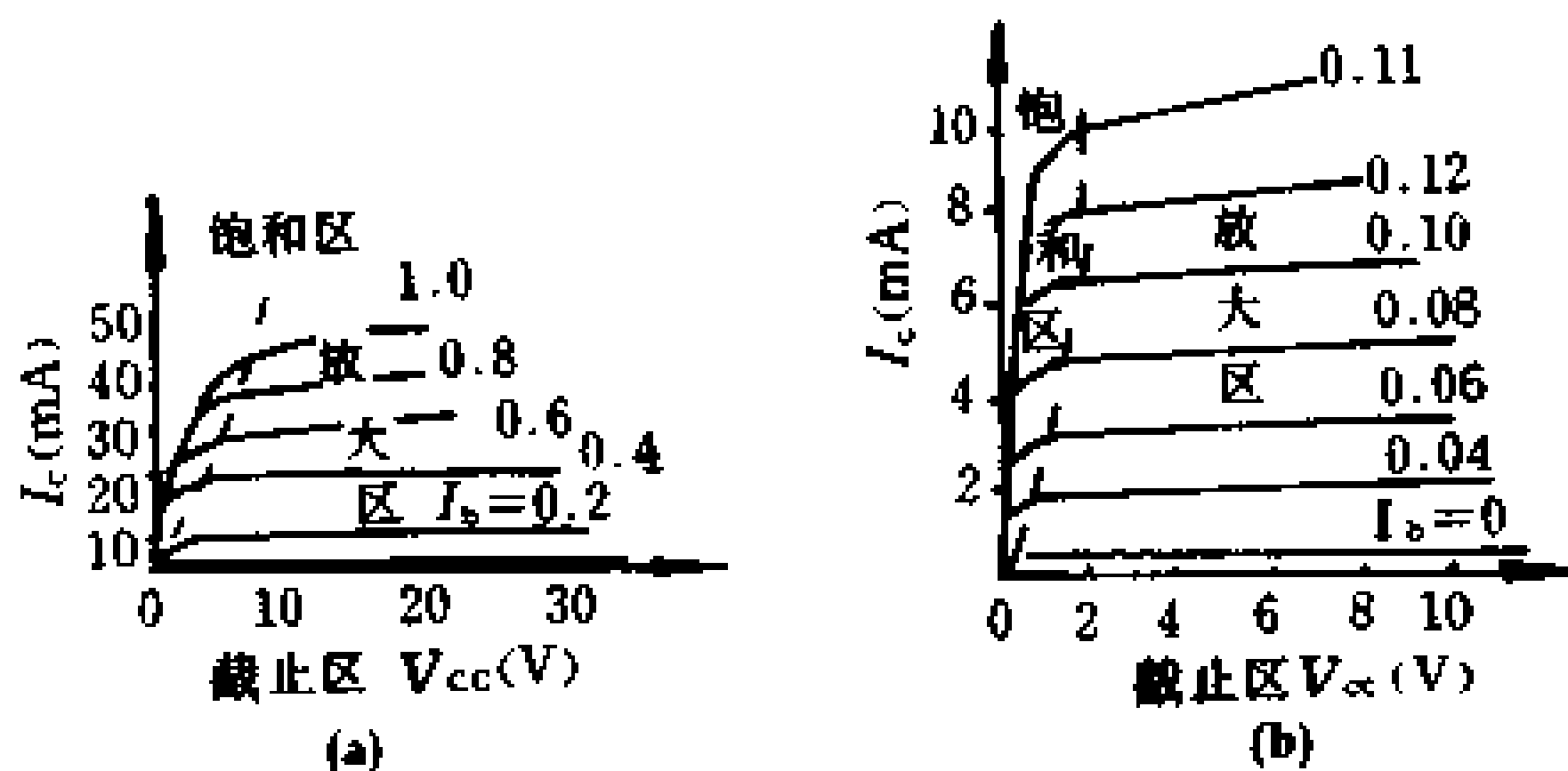
图 3-7 晶体三极管的输出特性
