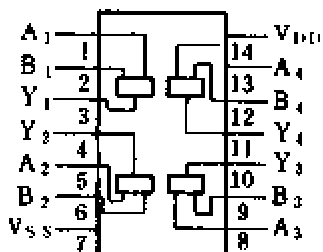
CC4081 四 2 输入与门 Y = A \cdot B
