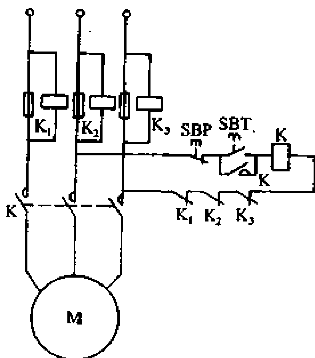
图 5-21 断丝电压保护线路
