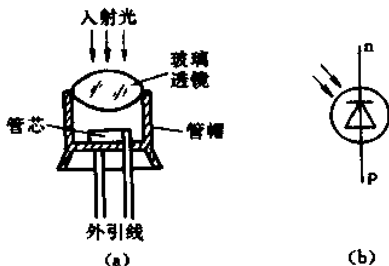
图 3-11 硅光电二极管内部结构及符号
