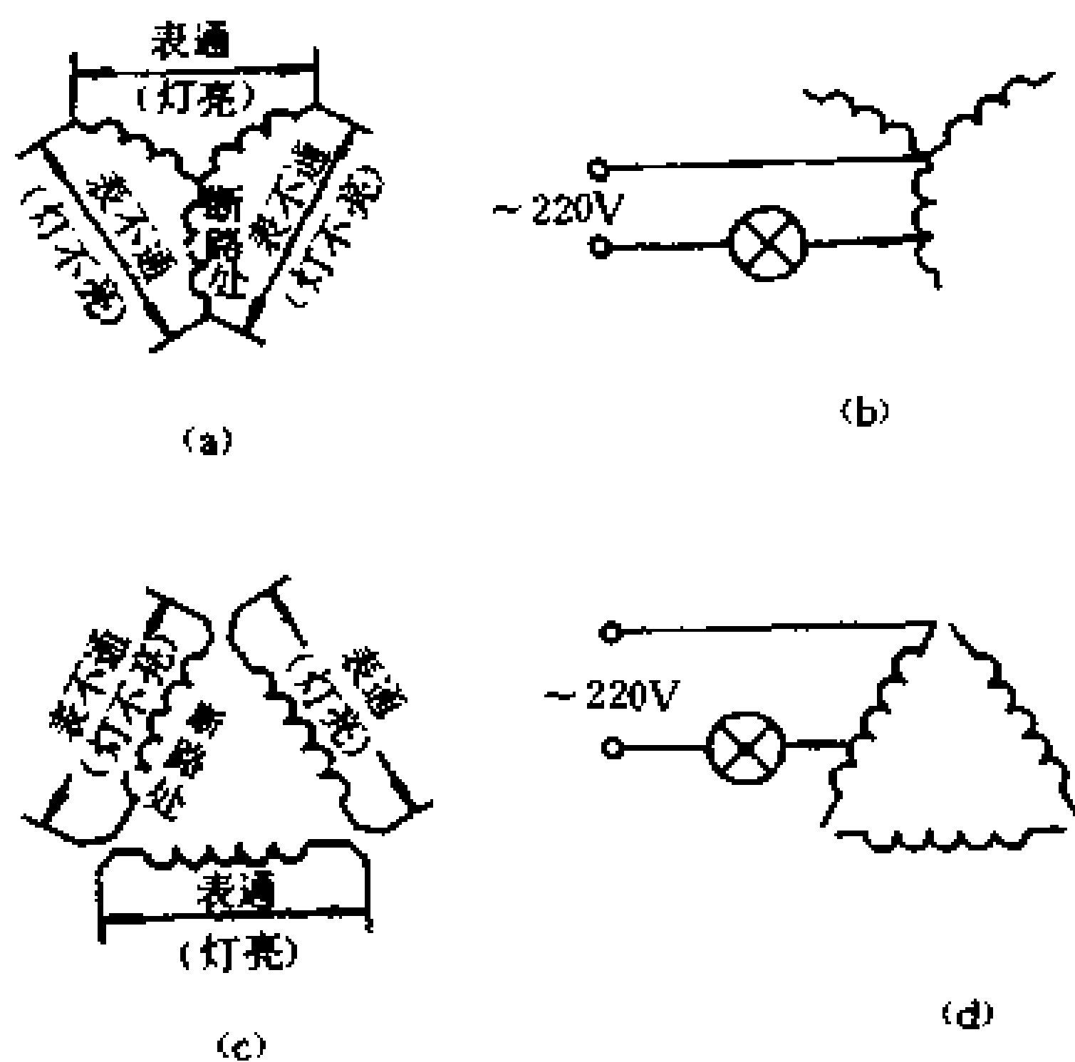
图 5-24 定子绕组断路的检查方法
