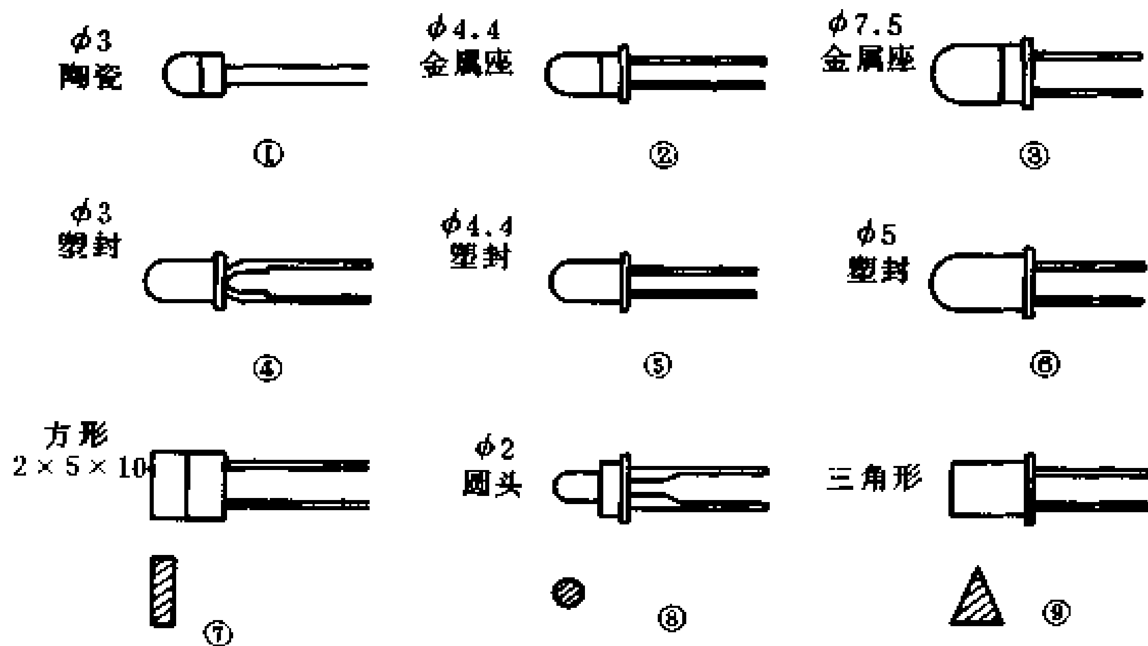
图 3-6 发光二极管的外形图
