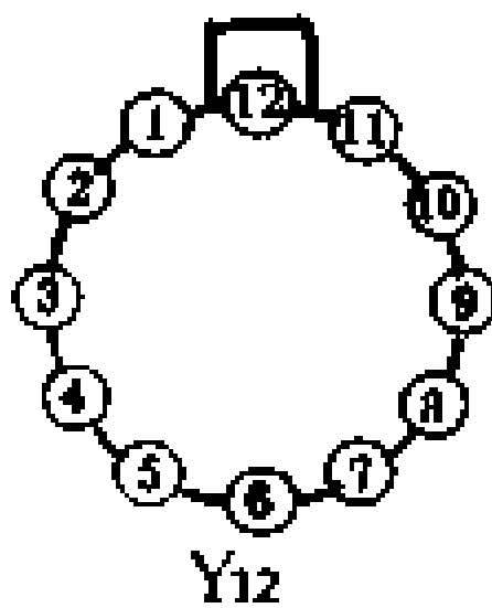
(c) 12 引线金属封装和双列直插封装
