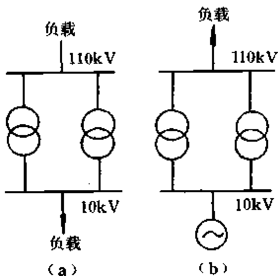
图 8-5 变压器并列运行示意图
