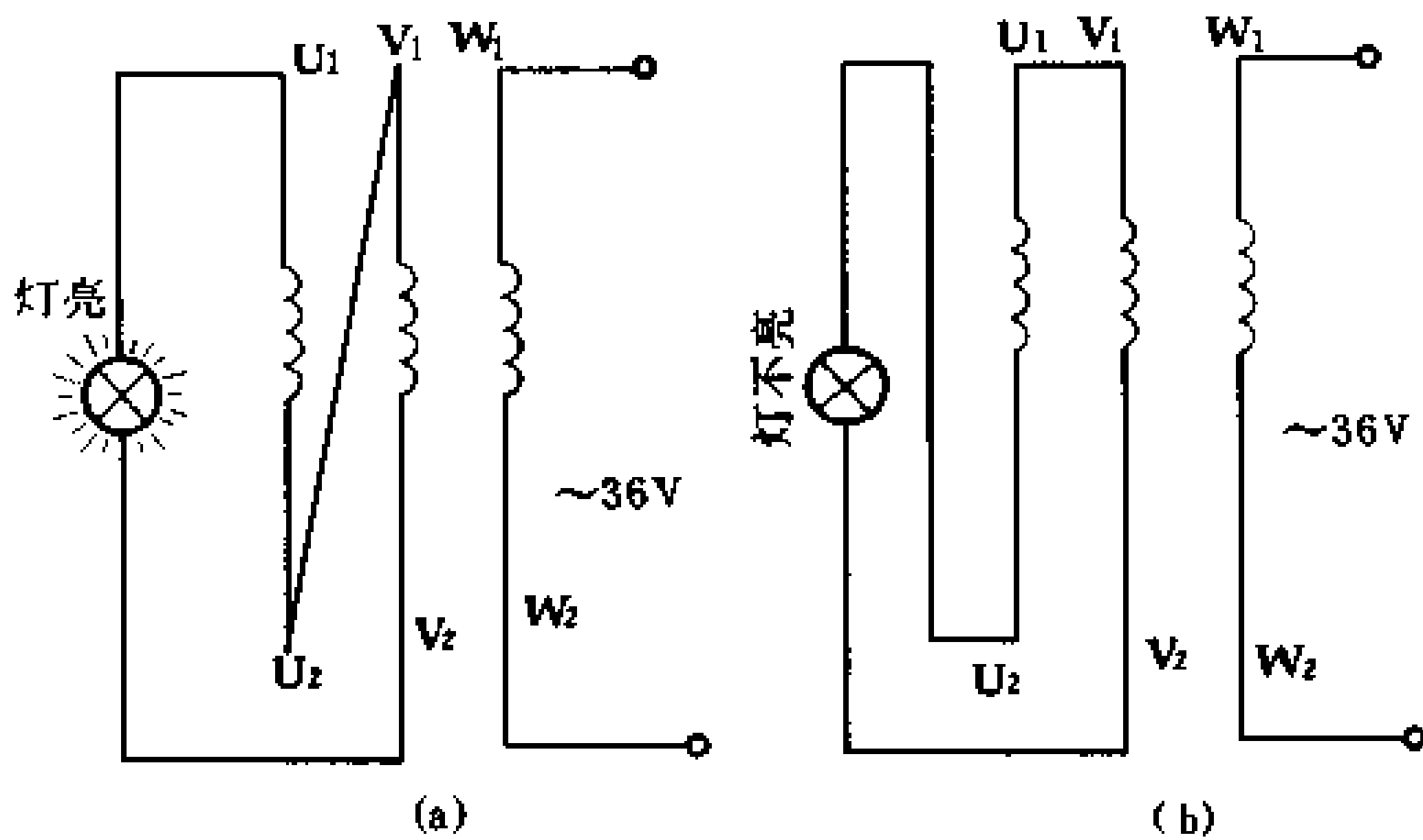
图 5-27 用灯泡检查三相绕组连接 (a) 头尾连接正确 (b) 头尾连接错误
