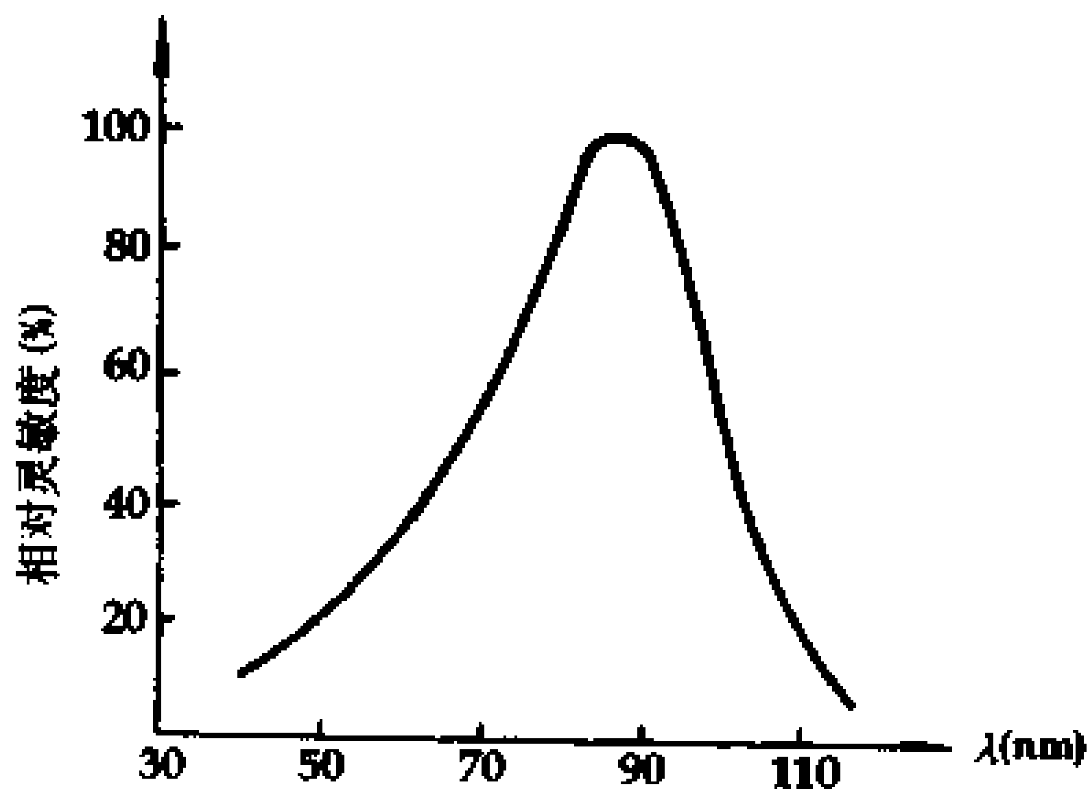
图 3-12 硅光电晶体管的波长特性曲线
