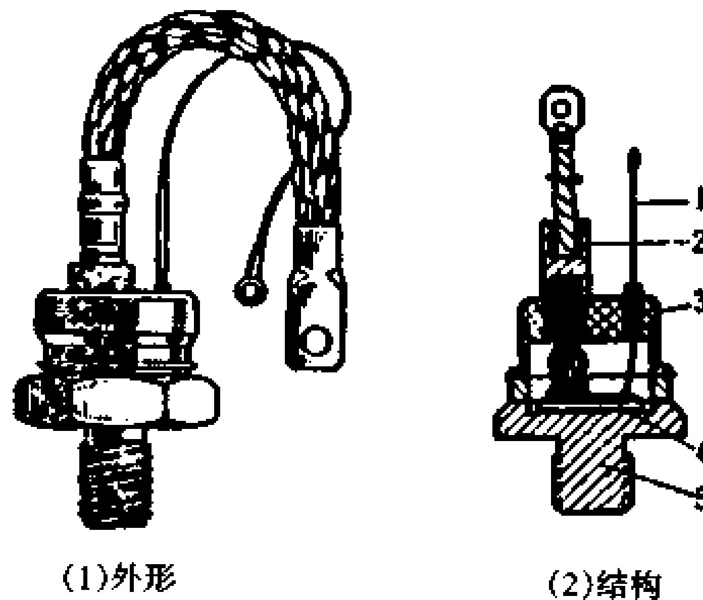
图 3-15(b) 螺栓型晶闸管
