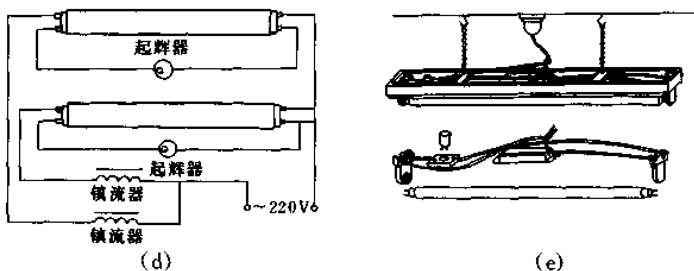
图 11-5 日光灯的安装方法及接线
