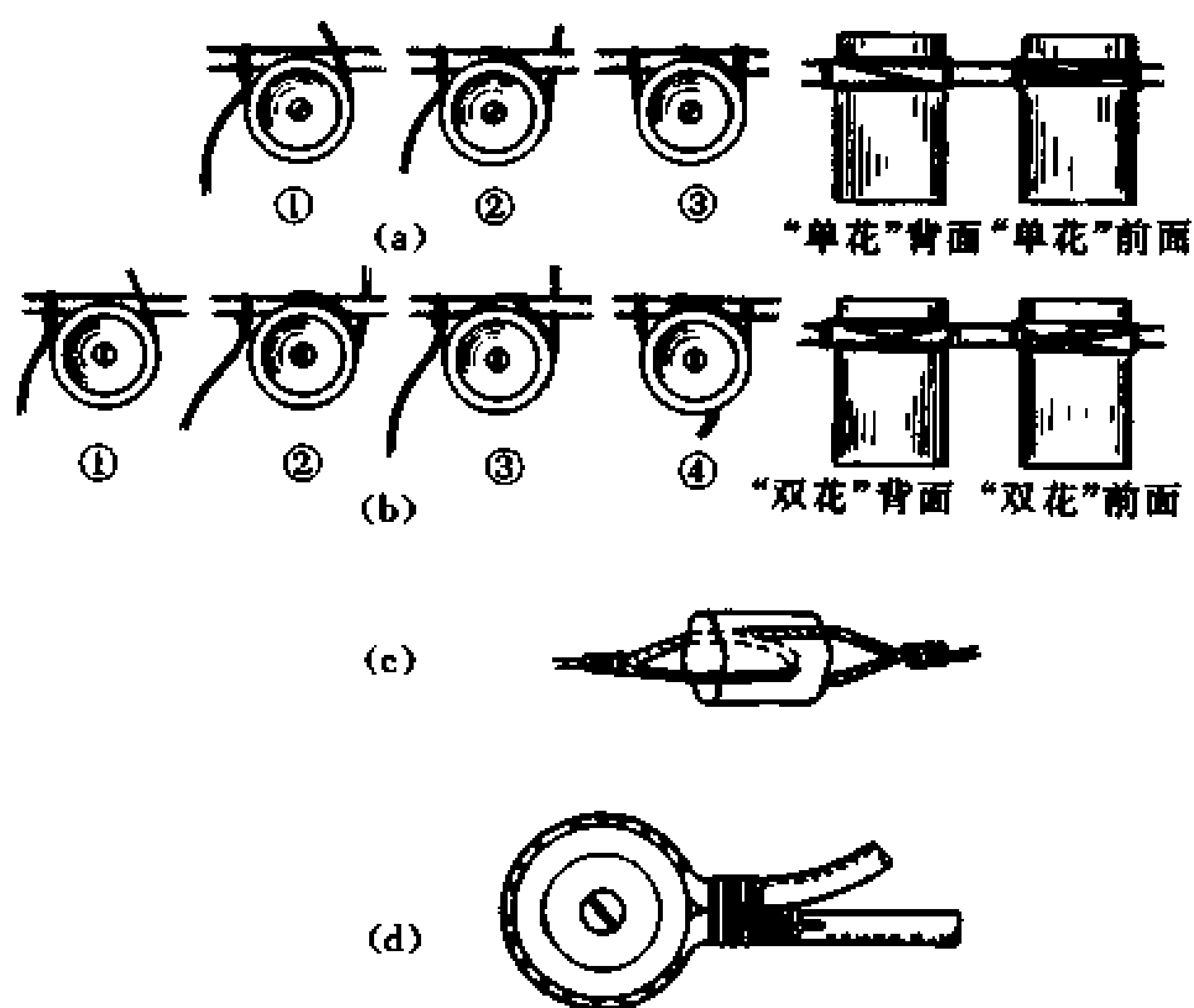
图 10-7 导线在绝缘子上的绑扎方法 (a) 瓷瓶单绑 (b) 瓷瓶双绑 (c) 隔绝缘子的绑法 (d) 导线回头绑法
