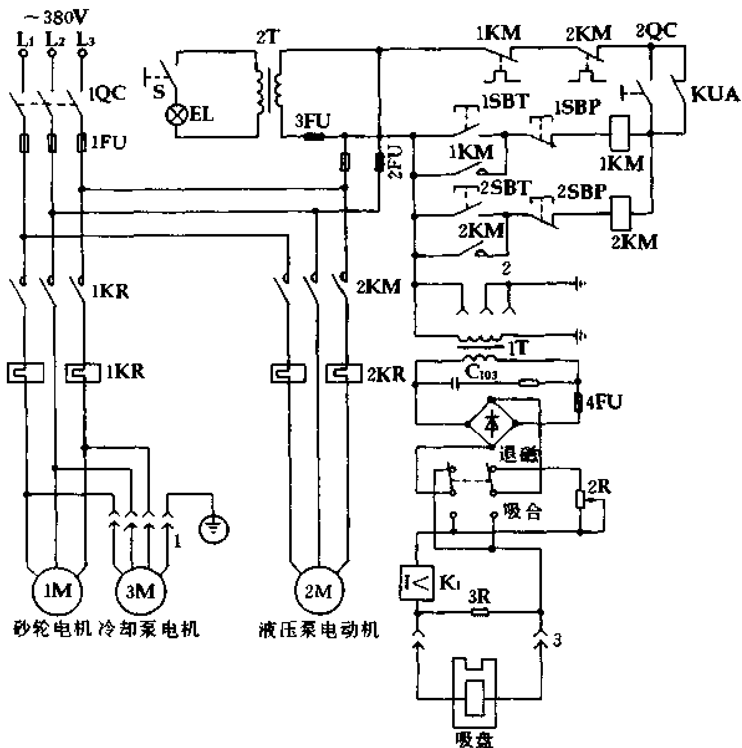
图 12-3 M7130 型平面磨床电路图
