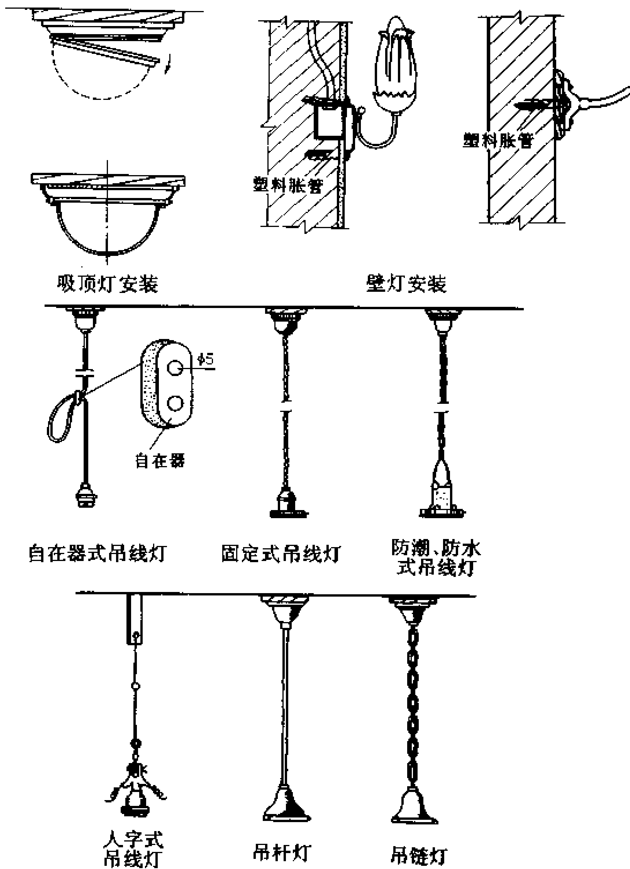
图 10-15 各种灯具安装方法
