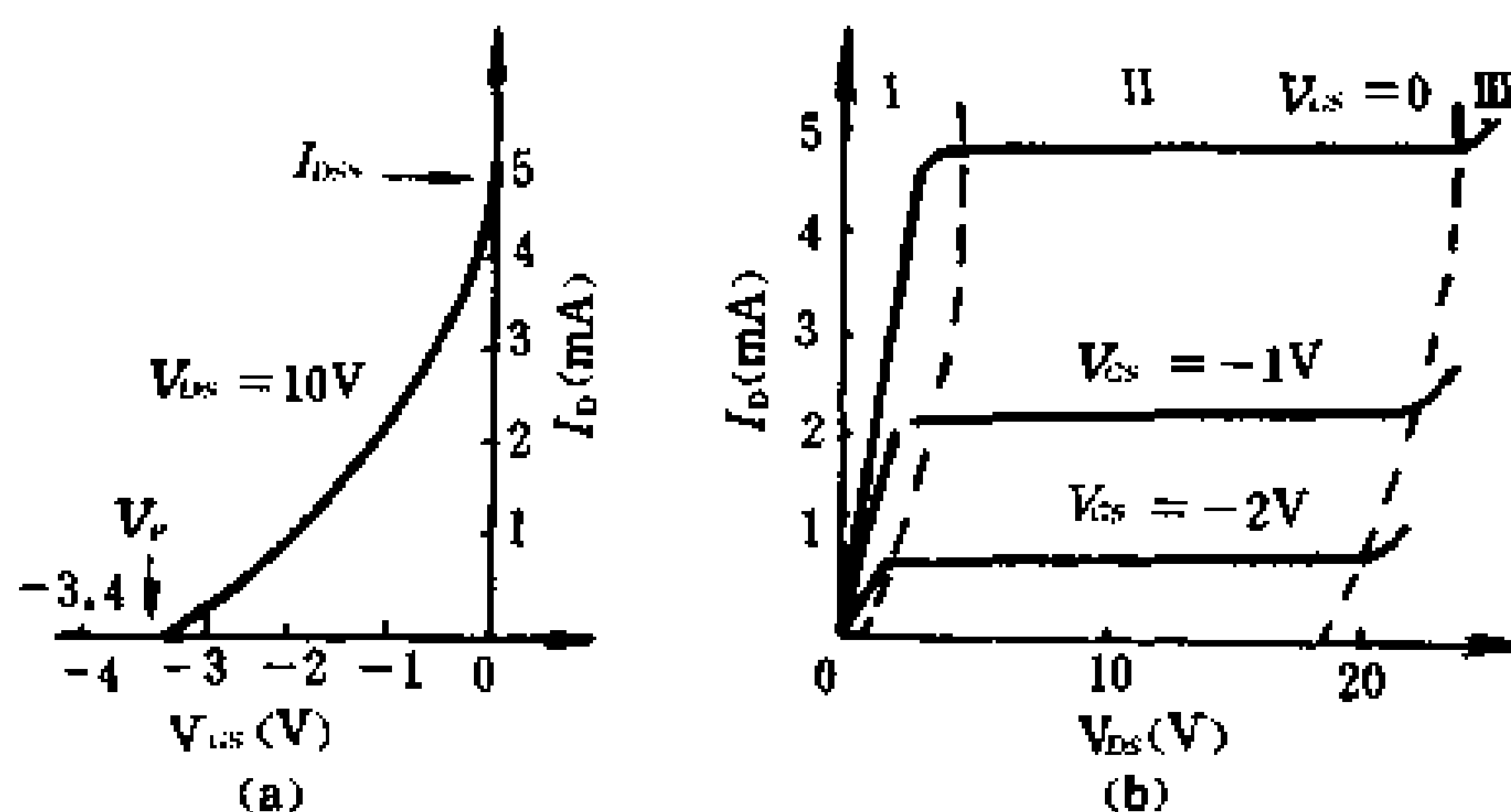
图 3-9 结构型场效应管的特性曲线
