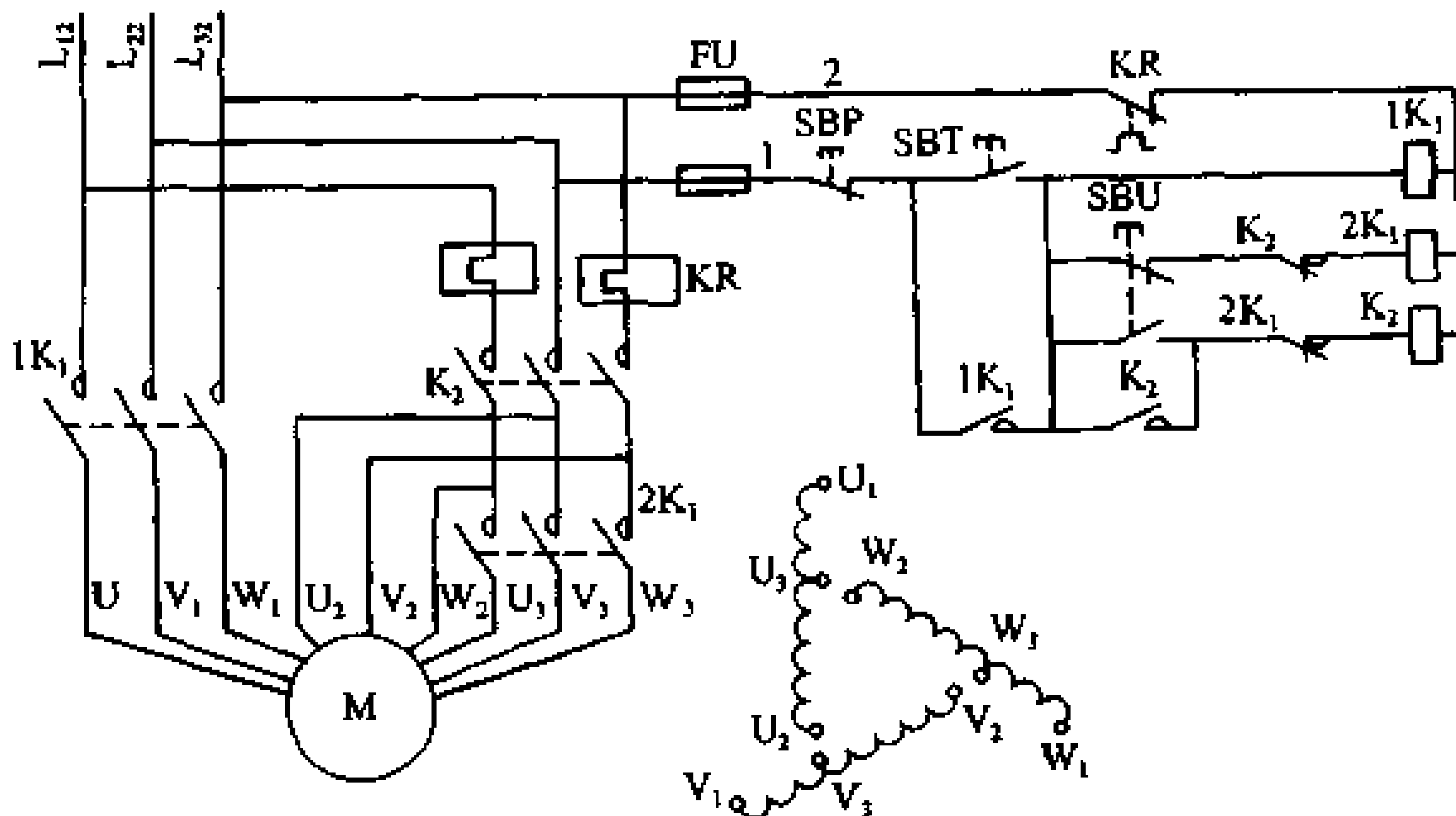
图 5-10 延边三角形降压起动电路
