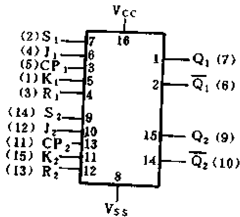
CC4027 双上升沿JK触发器
