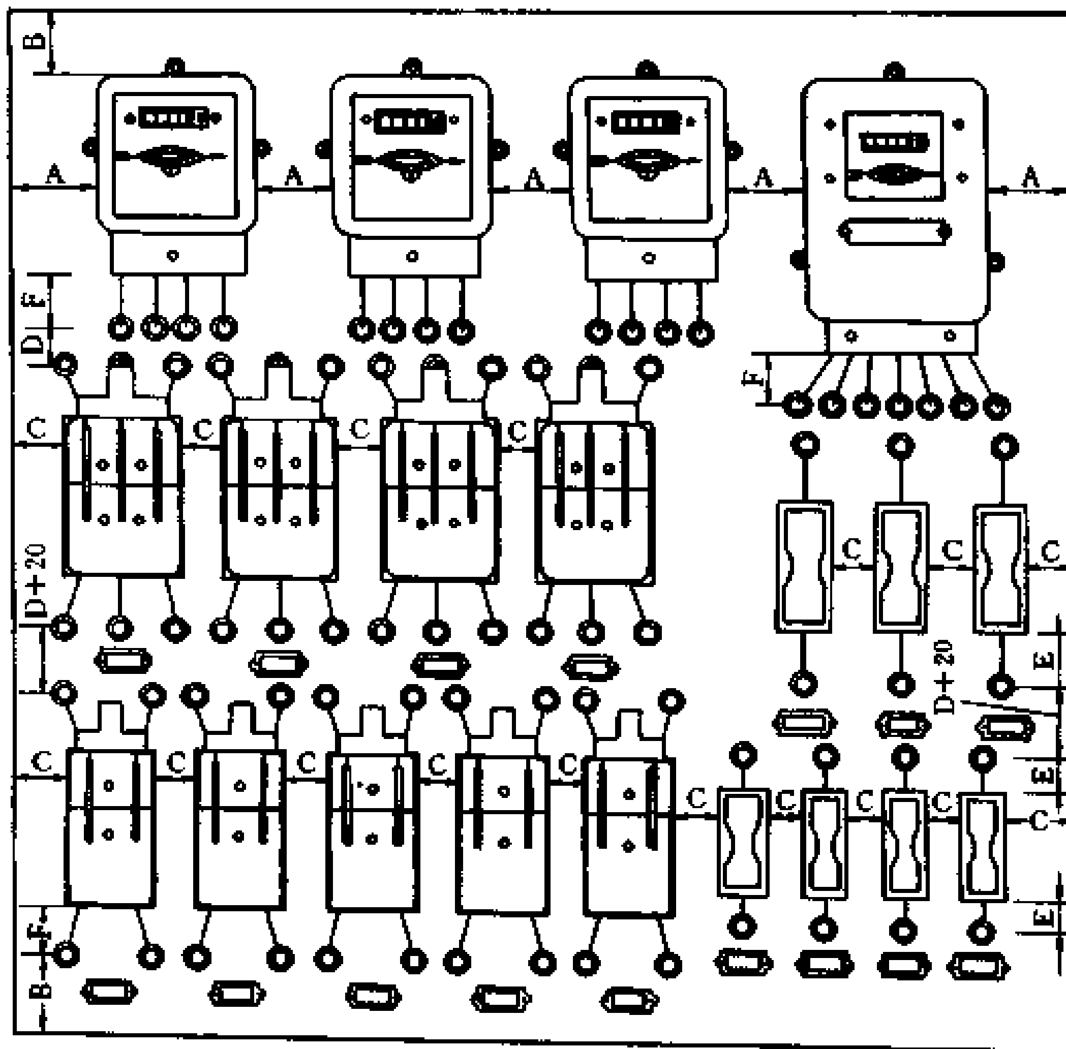
图 10-14 低压配电箱盘面电具排列图
