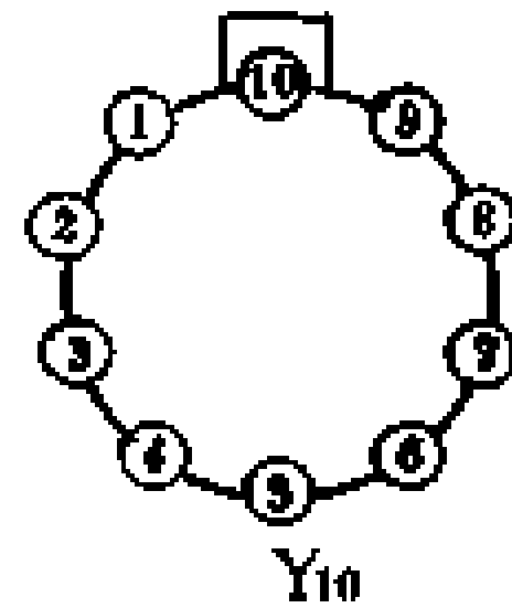
(b) 10 引线金属封装和双列直插封装
