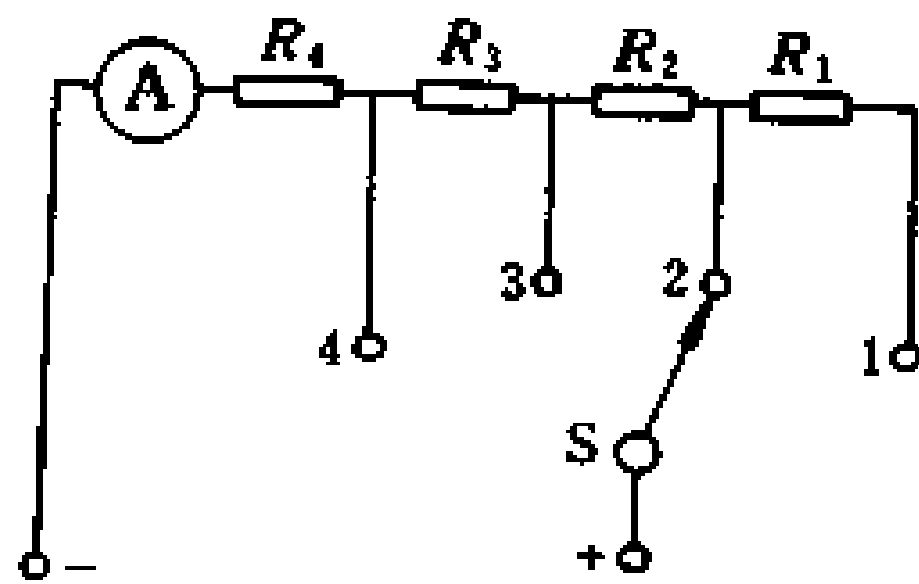
图 2-3 万用表测量直流电压的实际线路
