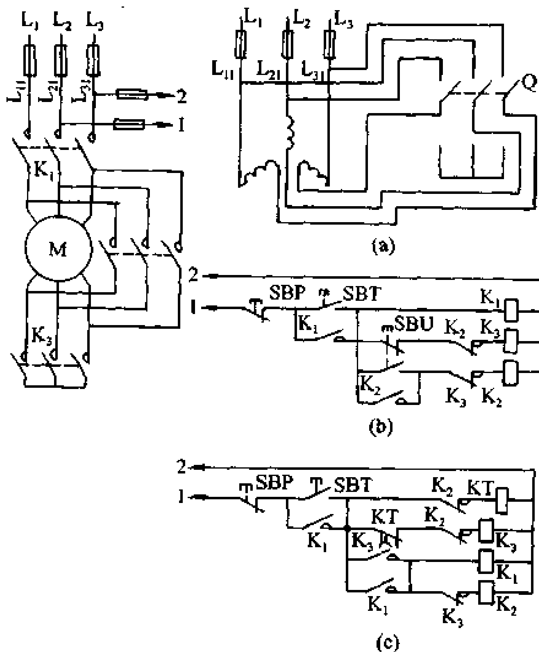
图 5-7 星-三角降压起动电路
