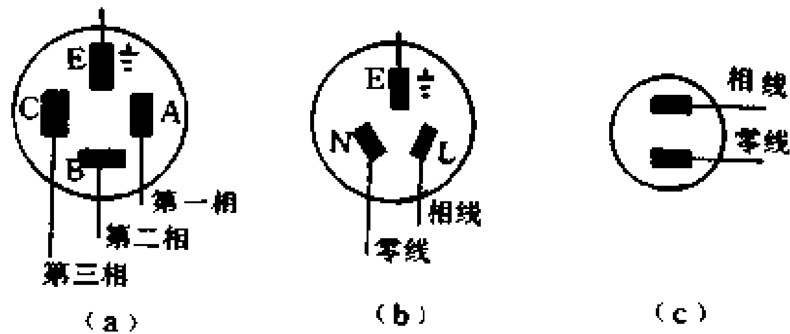
图 9-2 插座接线和标志图
