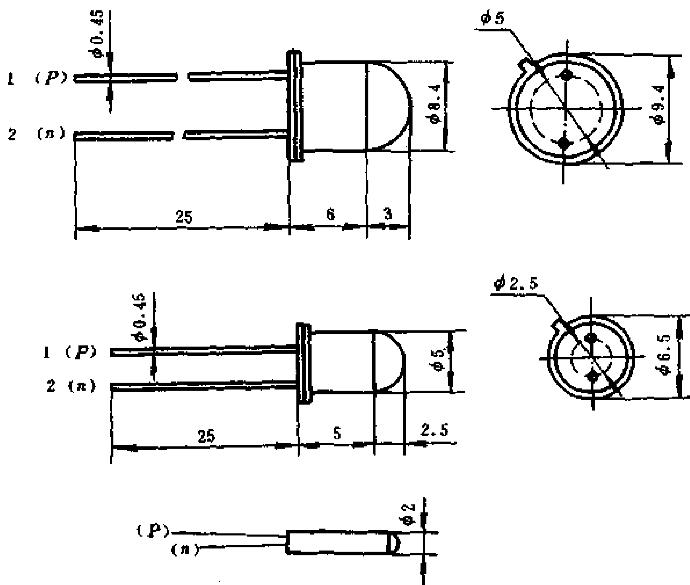
图 3-14 光电二极管外形图
