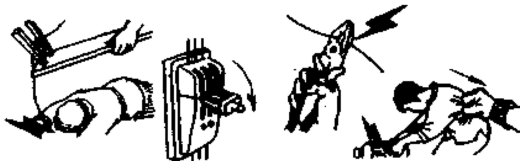
图 1-10 正确解脱触电电源的方法
