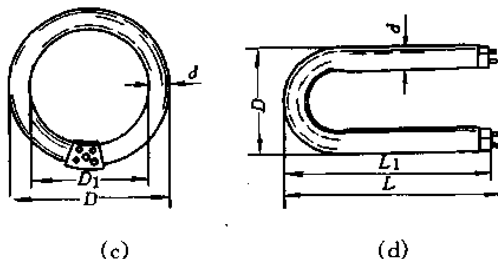
图 11-4 日光灯的结构及灯管形式
