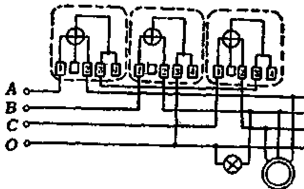
图 2-8 用三块单相电度表测量三相四线制接线图
