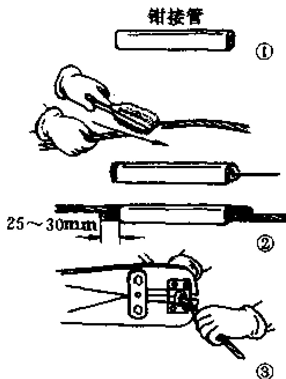
图 10-4 绞线压接方法和步骤
