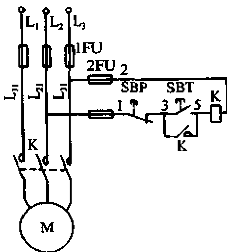
图 5-3 具有自锁的单向起动控制电路
