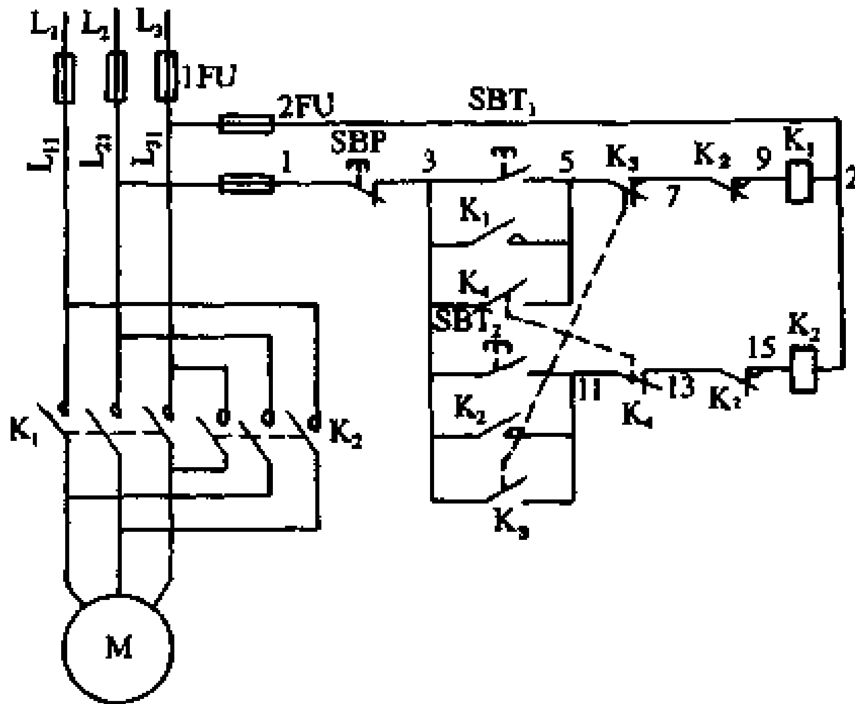
图 5-5 自动循环控制电路
