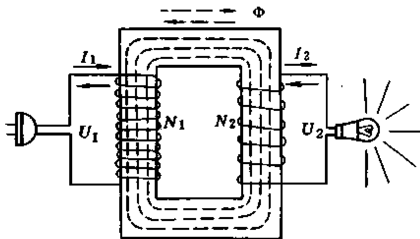
图 8-1 单相变压器原理图
