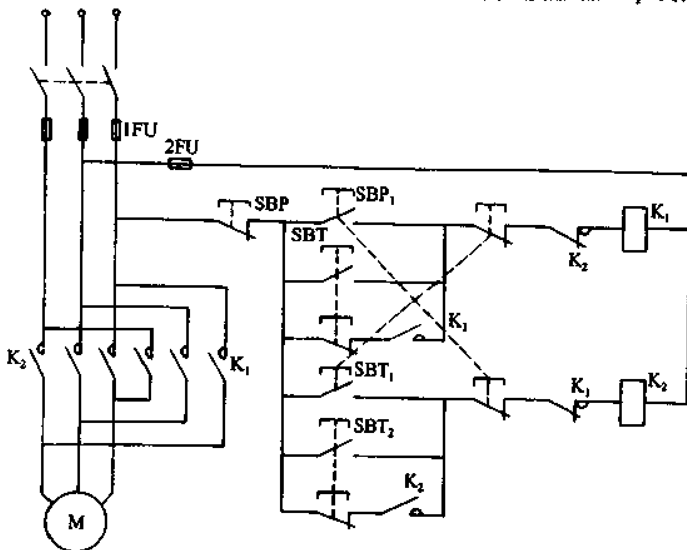
图 5-6 可逆点动、起动混合控制电路
