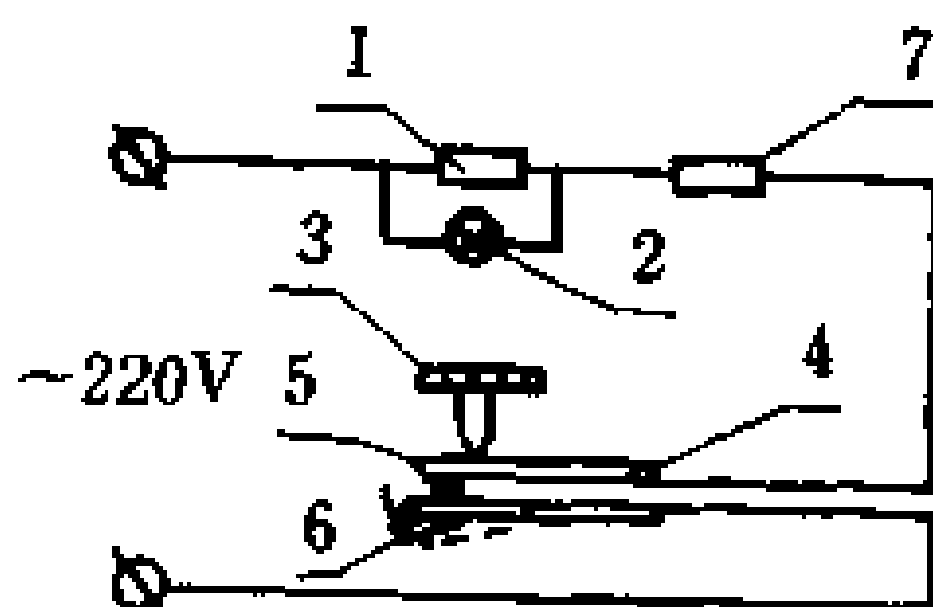
图 14-6 调温电熨斗电路原理图
