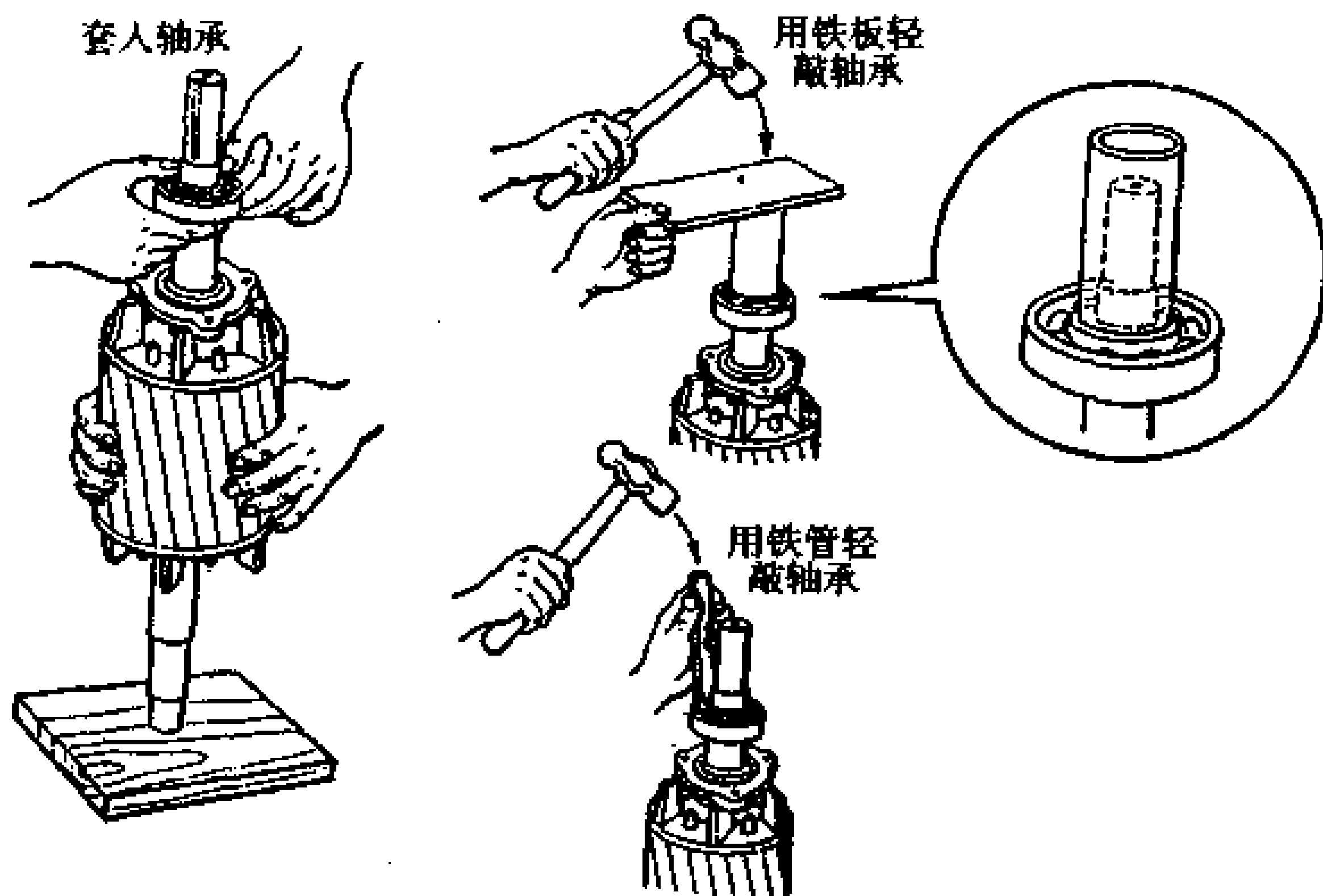
图 5-23 装配轴承的方法
