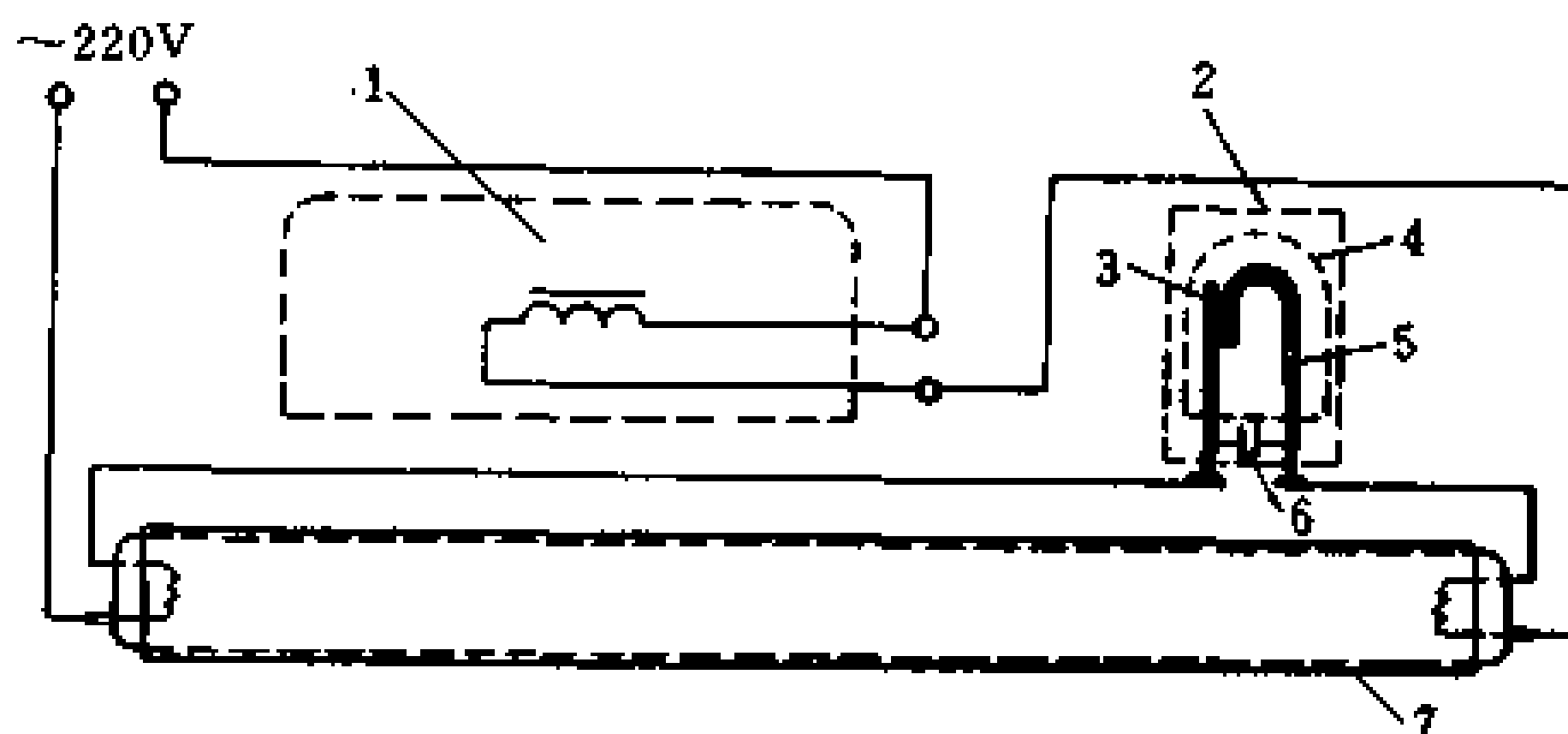
图 11-3 日光灯的原理接线图
