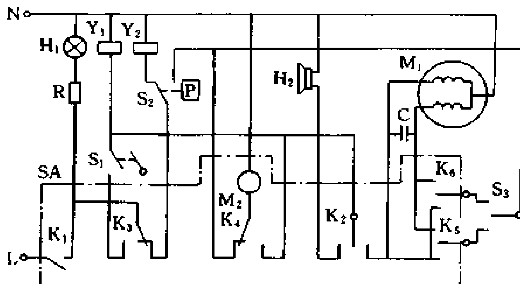
(a) 电动式程序控制器的控制电路
