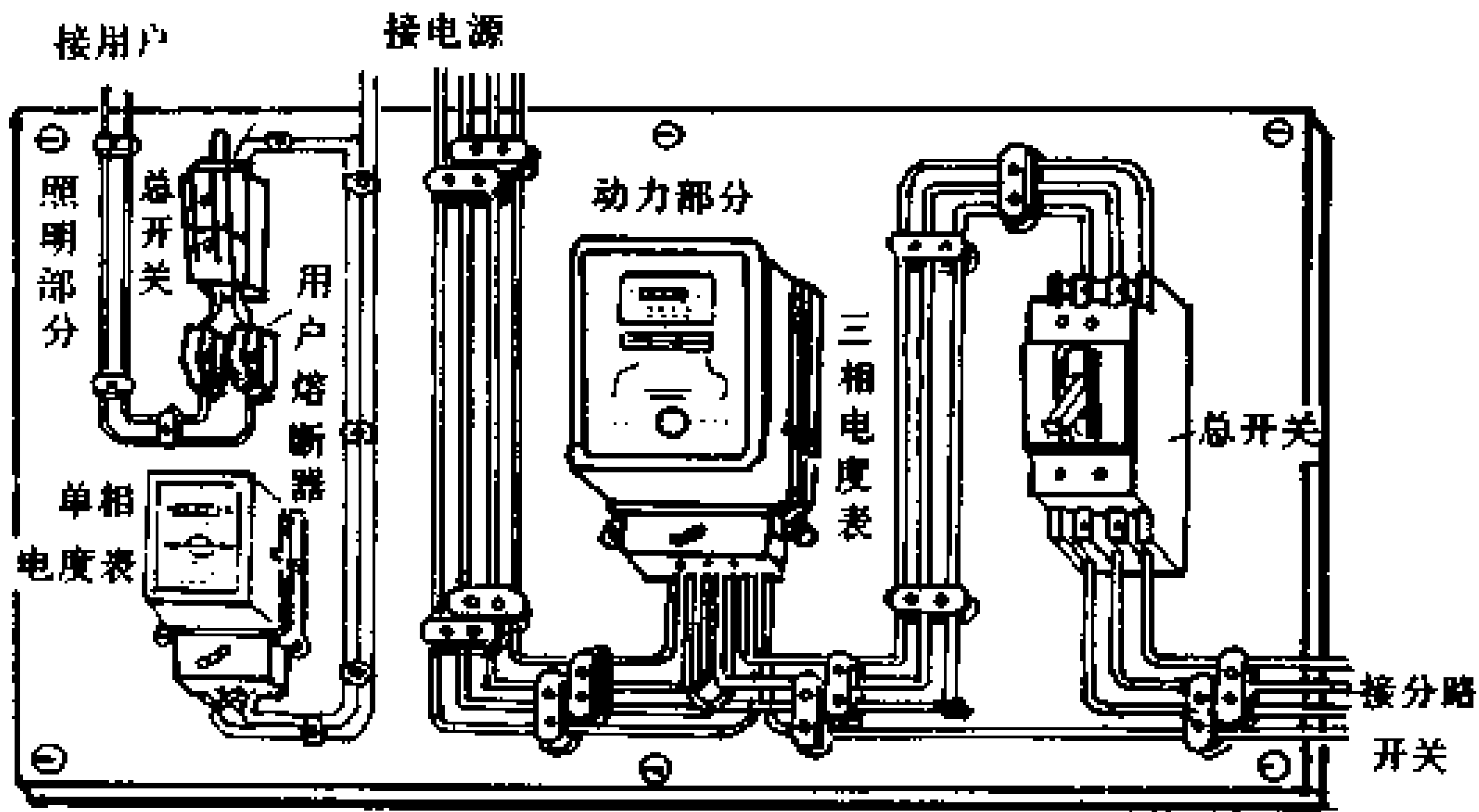
图 10-13 小容量配电箱接线示意图
