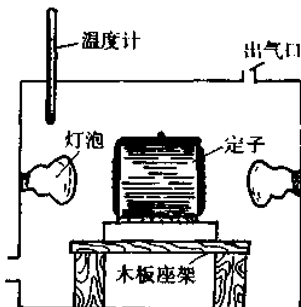
图 5-32 用灯泡烘干绕组的示意图
