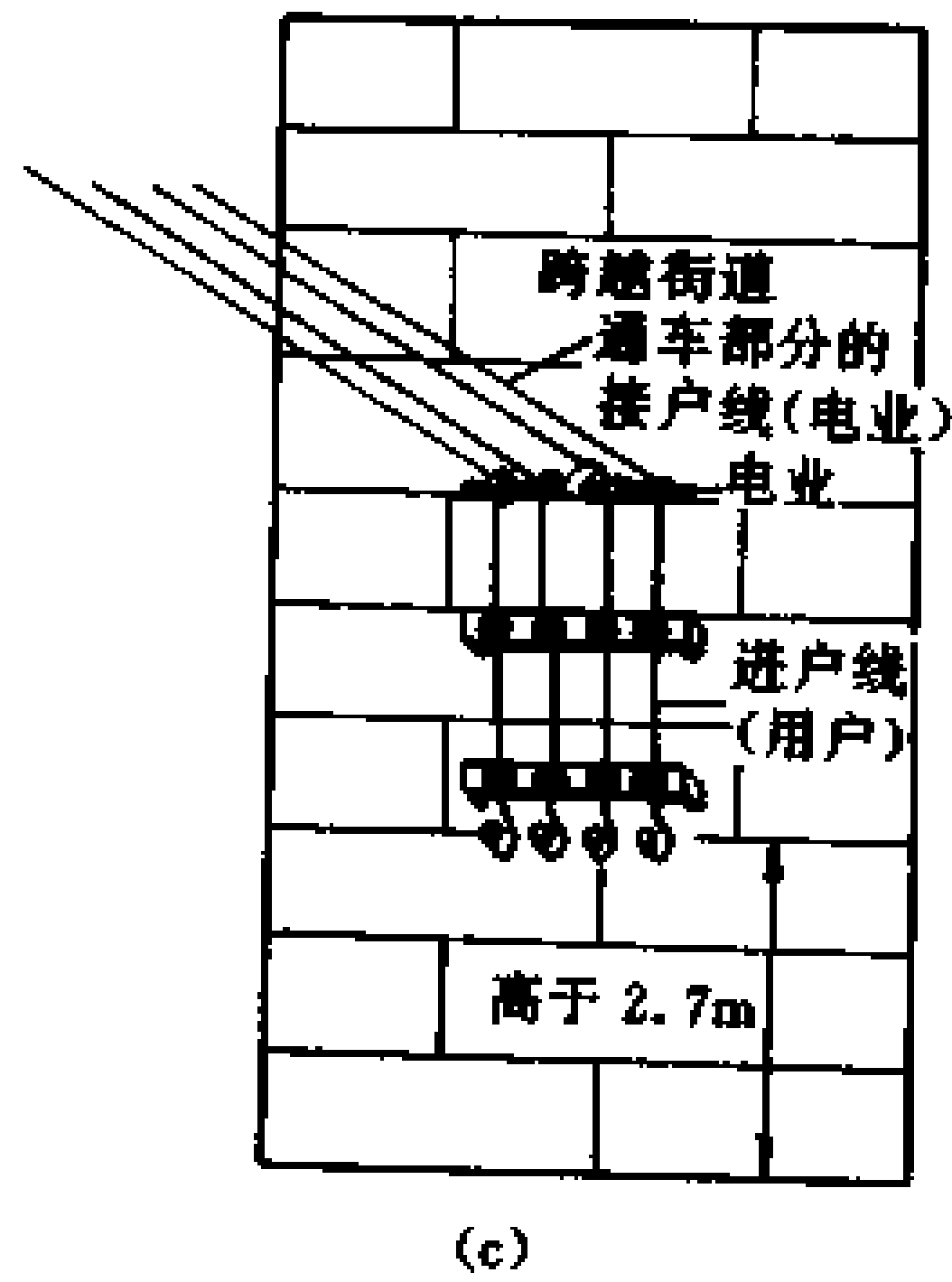
图 10-2 绝缘线穿瓷管进户
