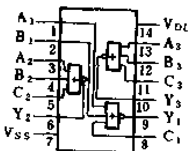
CC4025 三 3 输入或非门 Y = \overline{A + B + C}
