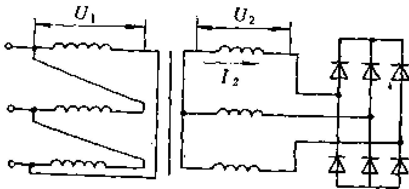
图 8-10 三相 E 形电源变压器电路图
