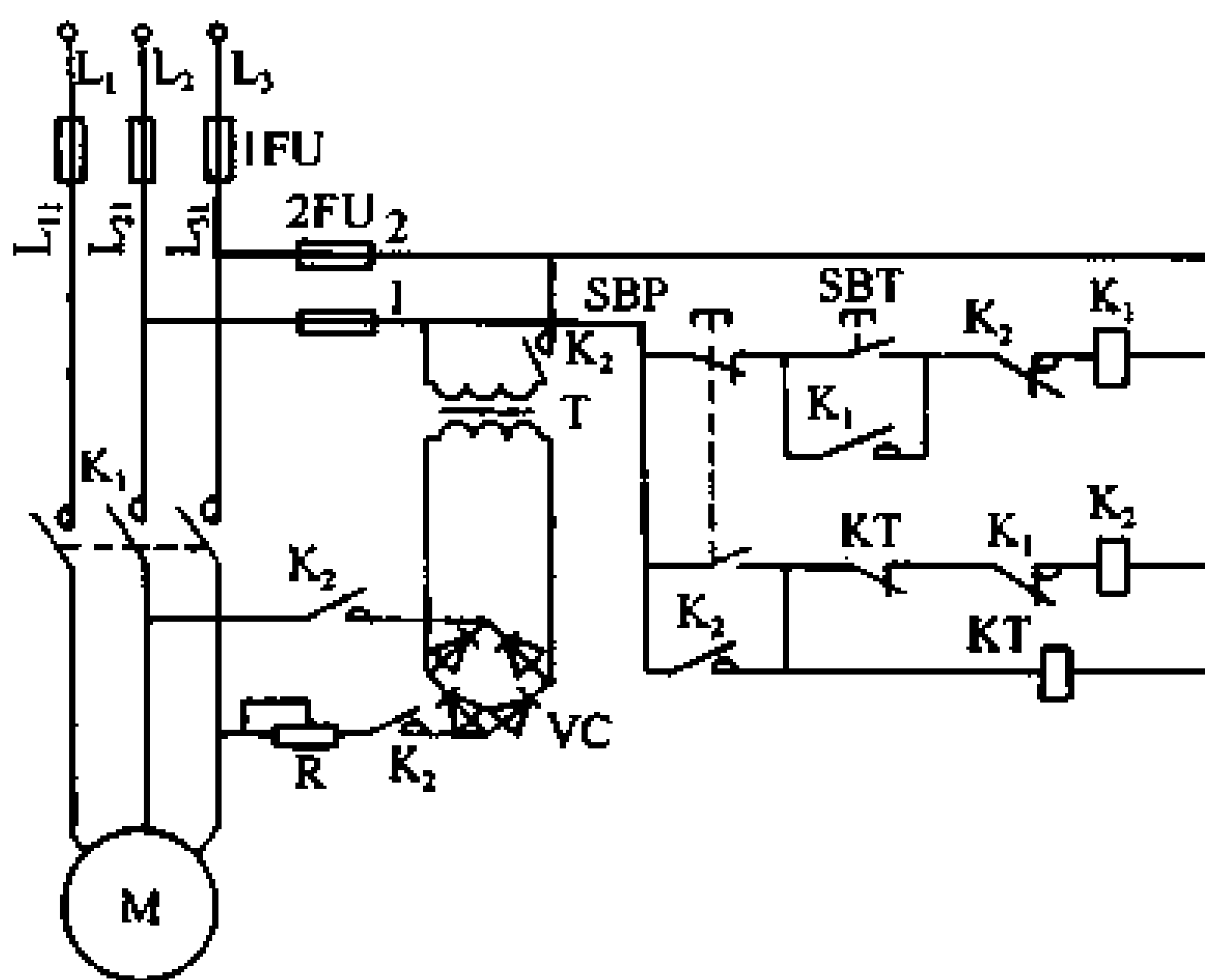
图 5-14 能耗制动控制线路
