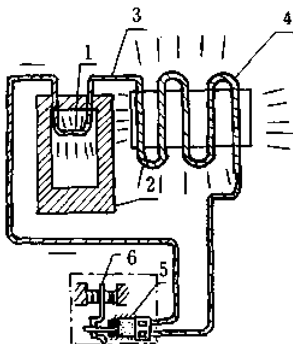
图 14-1 压缩式电冰箱制冷示意图
