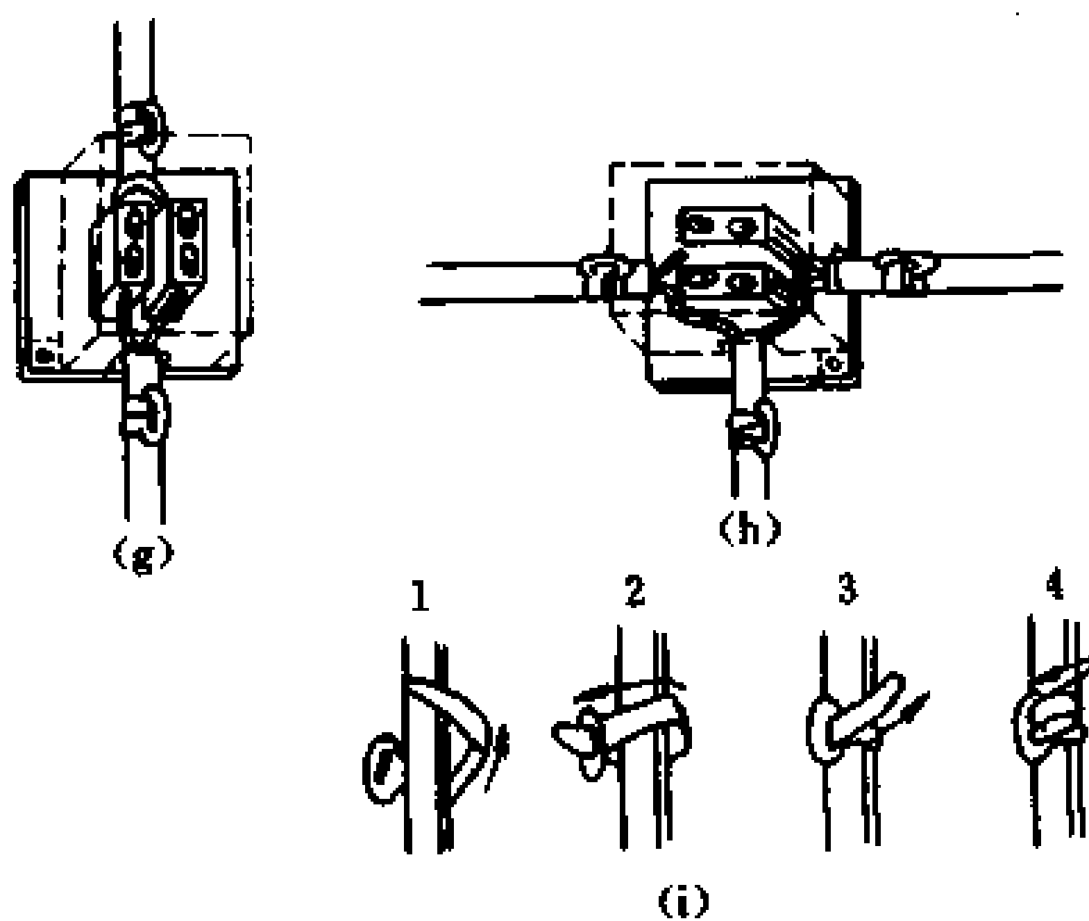
图 10-11 塑料护套管布线
