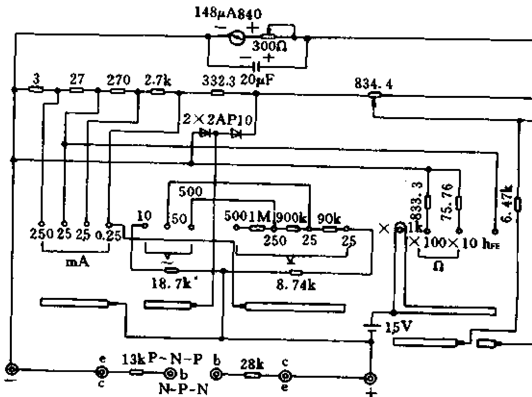
图 2-6 MF52 型万用电表接线线路图
