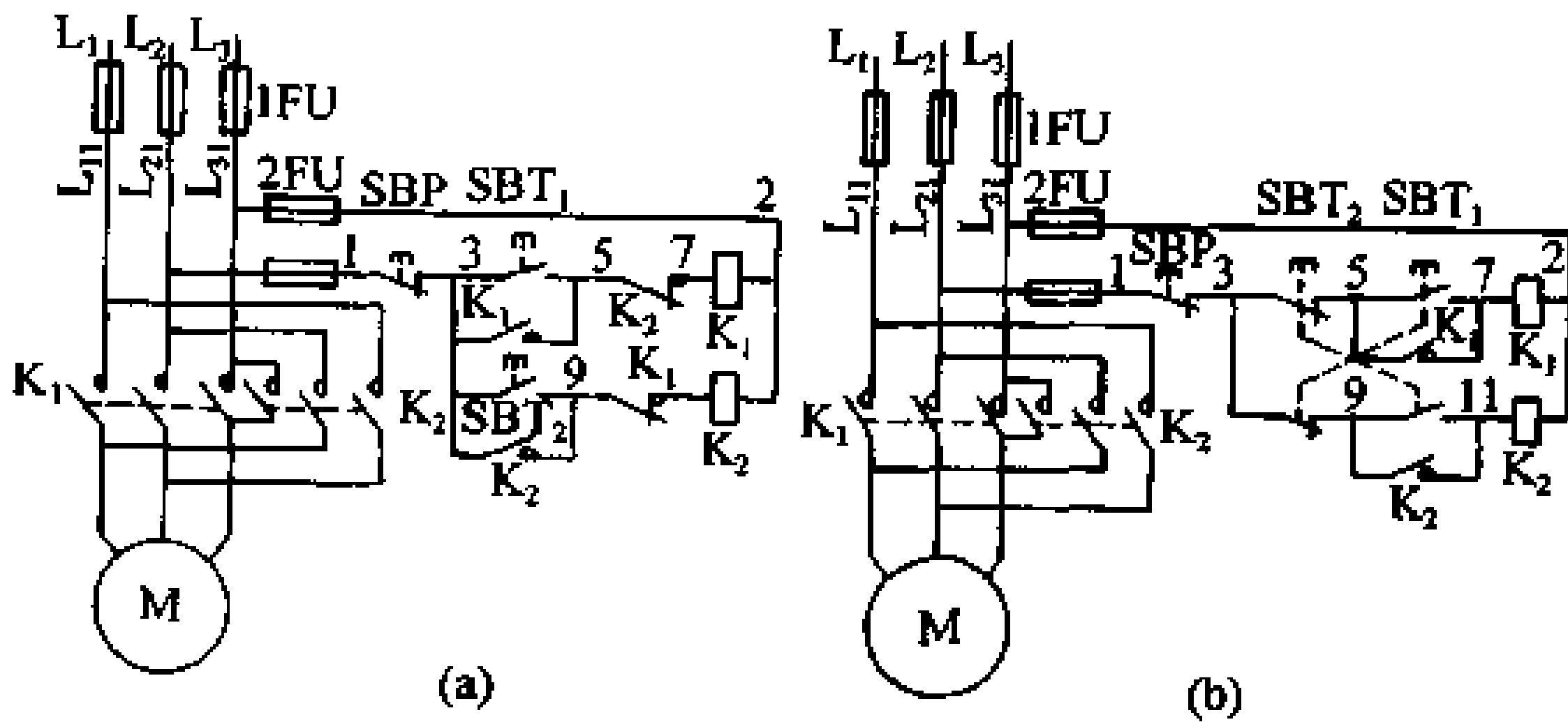
图 5-4 可逆起动控制电路
