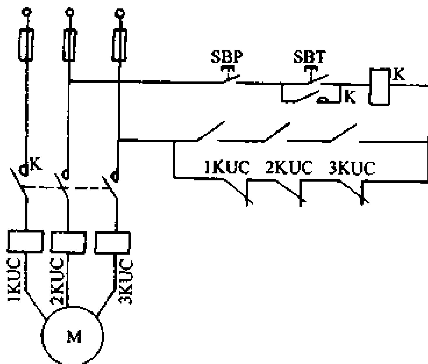
图 5-19 欠电流继电器保护线路
