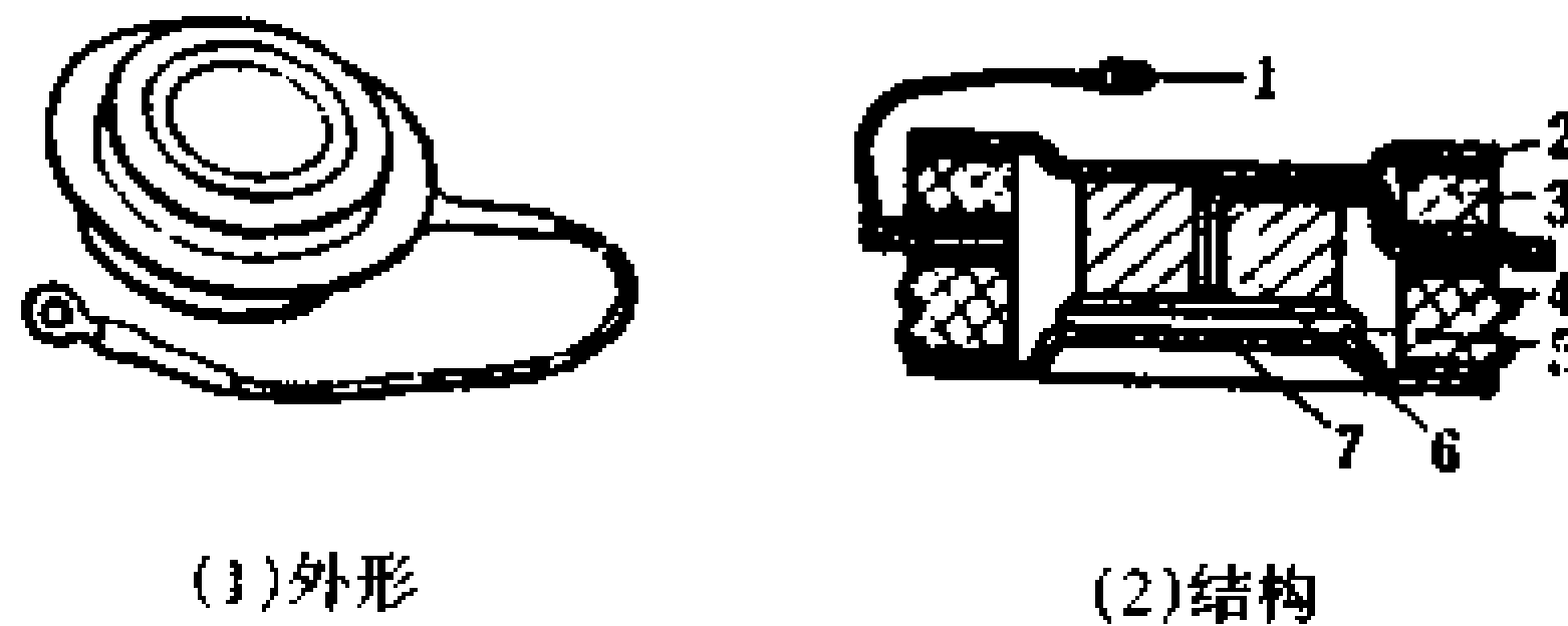
图 3-15(a) 平板型晶闸管
