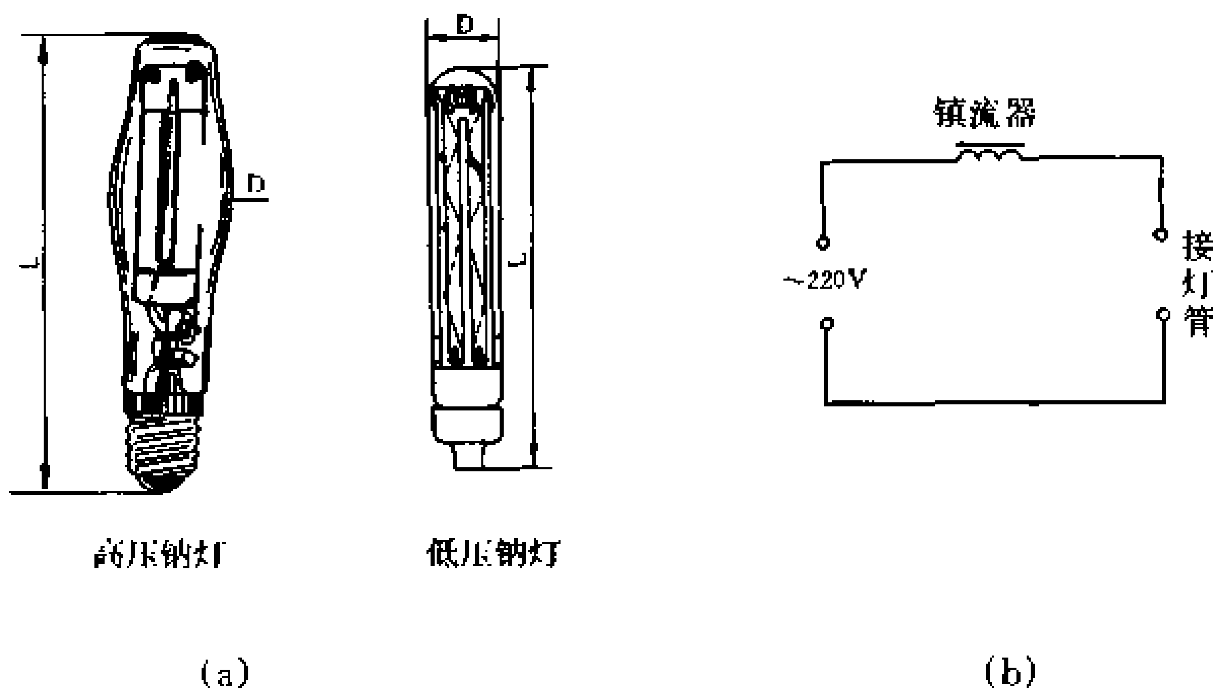
图 11-7 钠灯结构及其接线图
