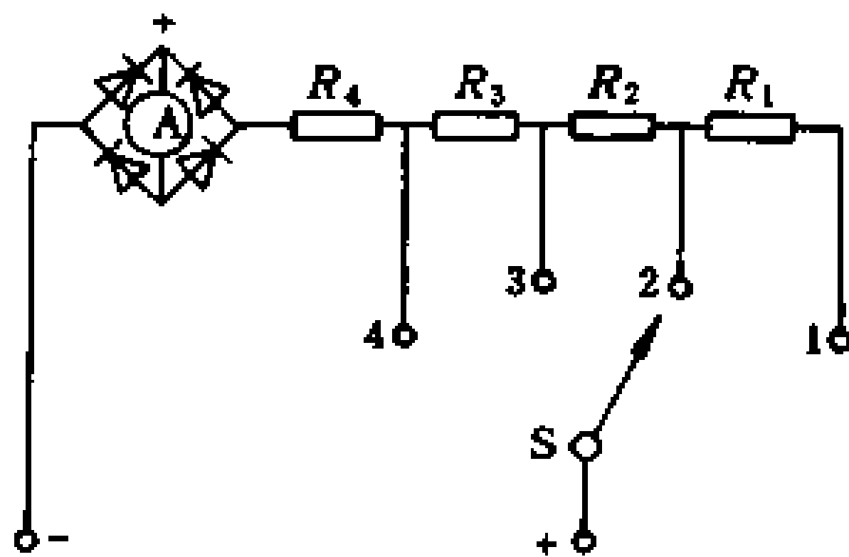
图 2-4 万用表测量交流电压的实际线路
