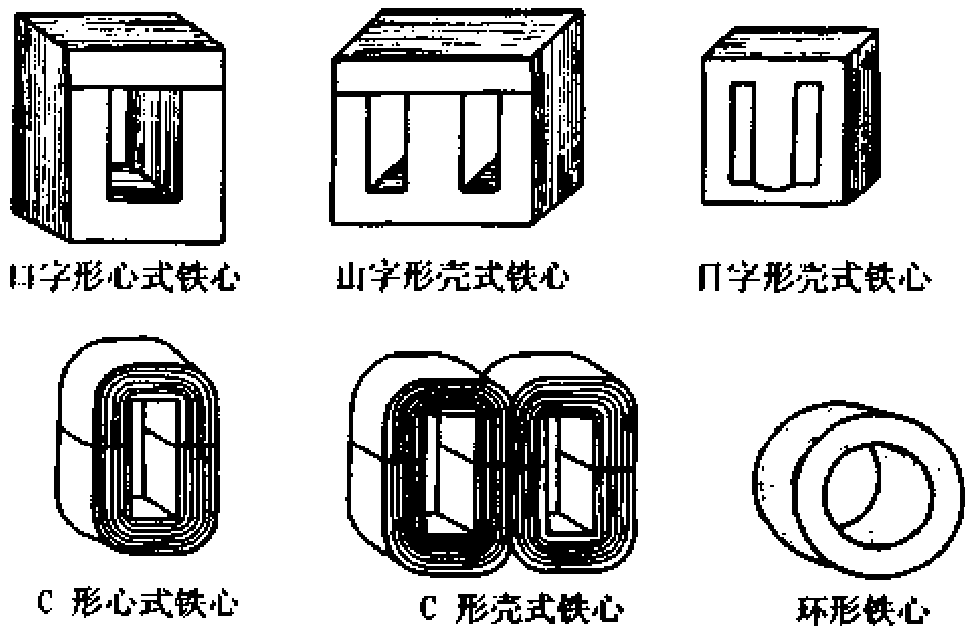
图 8-2 变压器铁心结构
