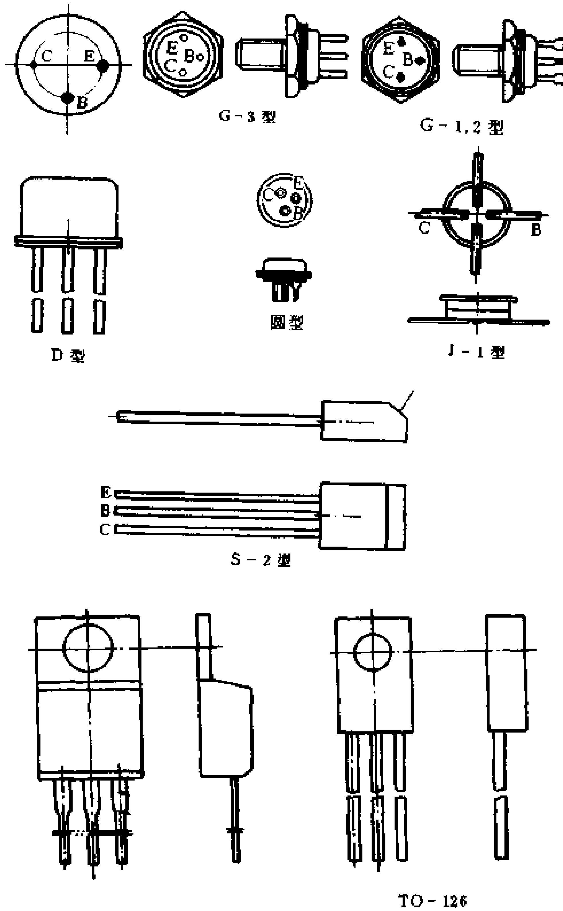
图 3-8 各类晶体三极管外形图
