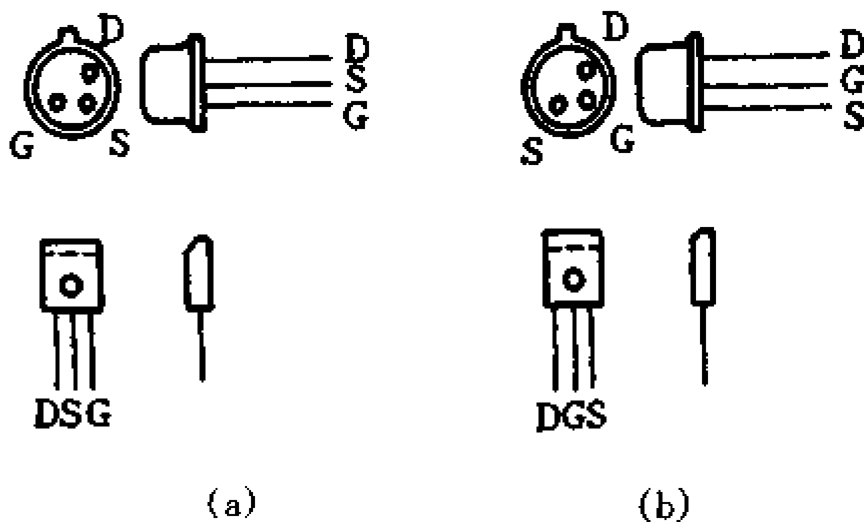
图 3-10 场效应管外形图
