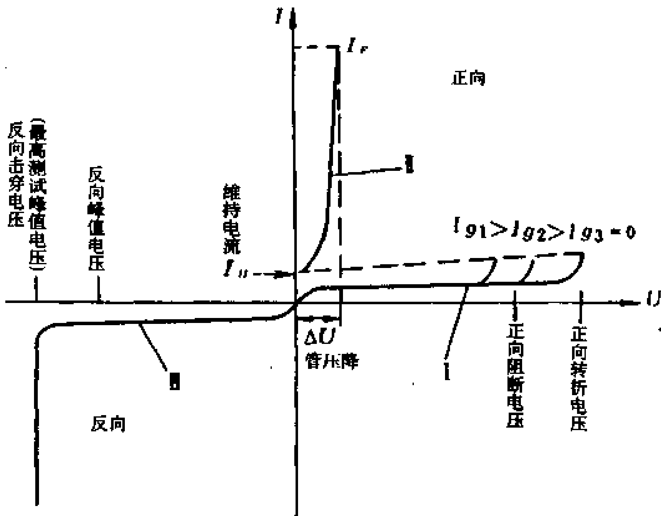
图 3-17 晶闸管的阳极伏安特性曲线
