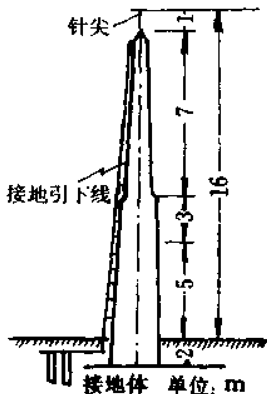
图 1-8 木杆避雷针示意图
