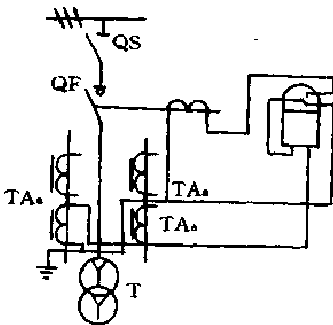
图 1-4 过电流保护二次接线原理图
