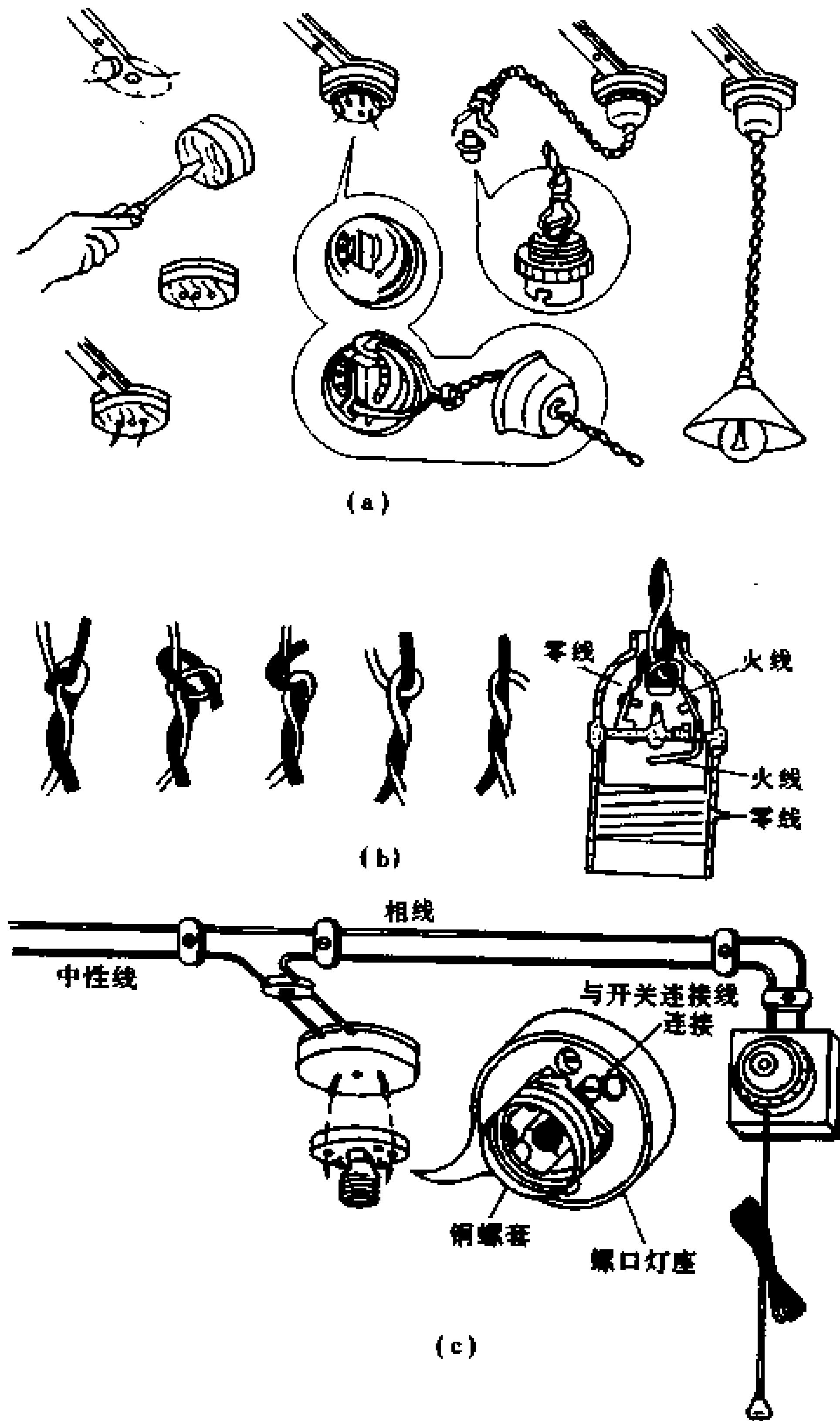
图 11-2 白炽灯的安装
