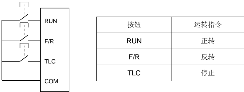
图 6-6 外控端子控制运行方式示意图
