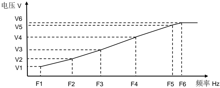
V1~V5: VF1~VF5 段电压点 F1~F5: VF1~VF5 段频率点 V6: 额定电压 F6: 额定频率
