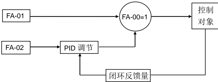
图 6-37 开环给定+PID 运行
