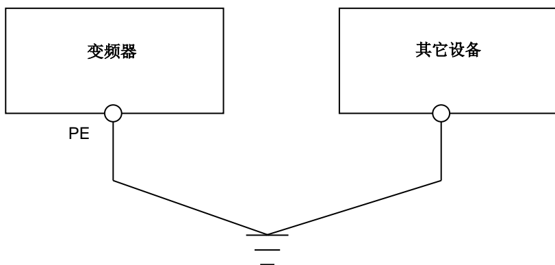
附图 2-4 共用接地极示意图
