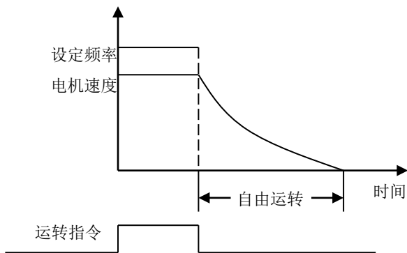
图 6-25 自由停车
