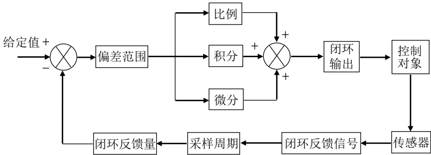
图 6-36 单一 PID 运行
