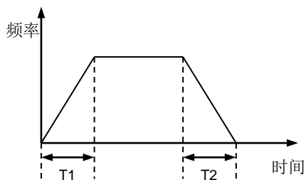
图 6-21 直线加减速
