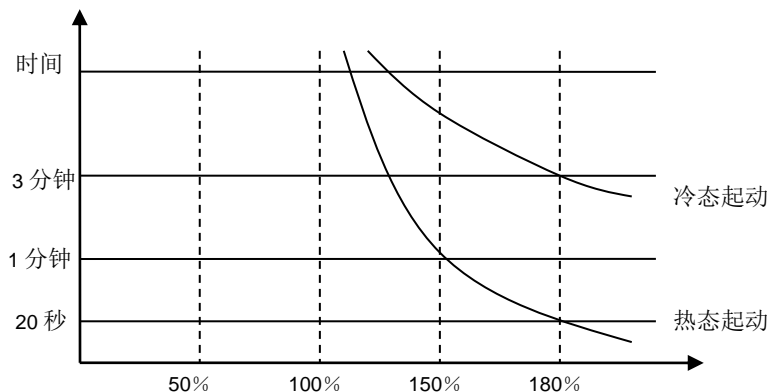
图 6-31 电子热保护
