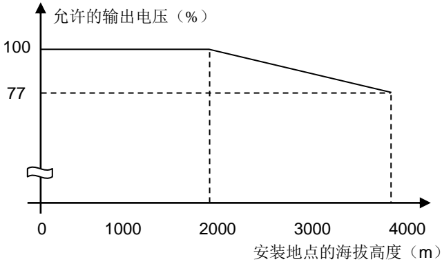
变频器额定参数随安装地点海拔高度的升高而降额
