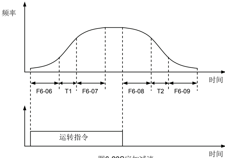
图6-23S字加减速
