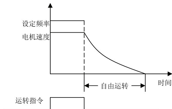
图 6-25 自由停车
