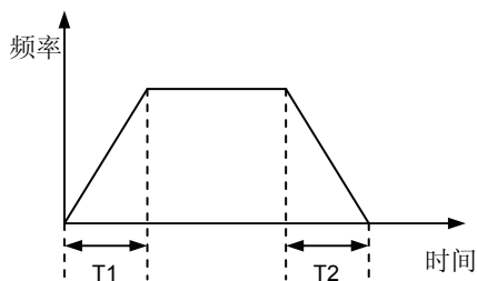
图 6-21 直线加减速
