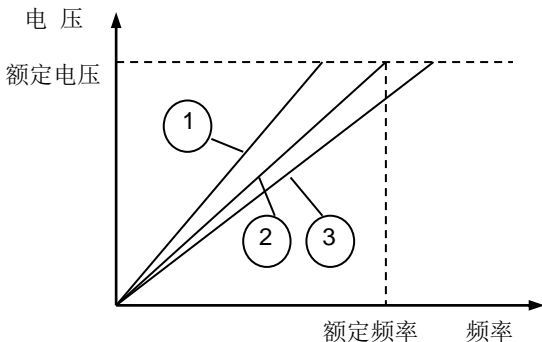
图 6-5 自动节能示意图
