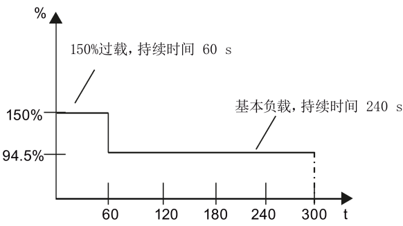
高过载模式允许的过载 (HO)
