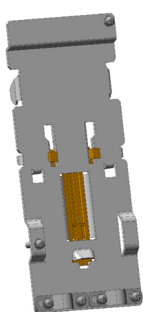
适用于外形尺寸 A 的 DIN 导轨安装件
