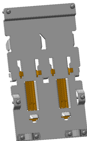
适用于外形尺寸 B 的 DIN 导轨安装件
