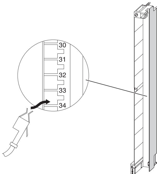
图 5-13 为带压接型端子的前连接器接线
