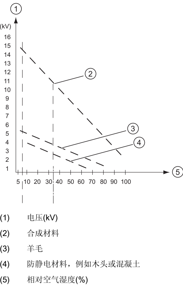
图 B-2 人体可能产生的静电电压
