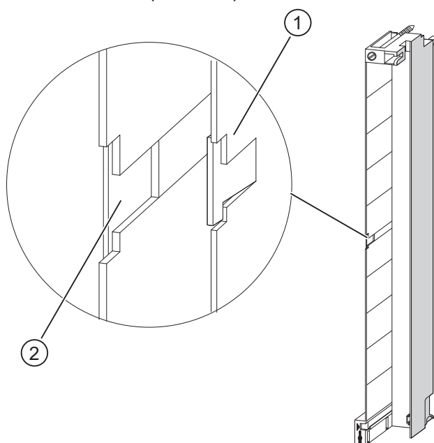
图 5-19 在前连接器上安装标签
