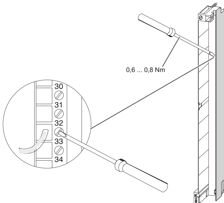
图 5-14 为带螺钉型端子的前连接器接线
