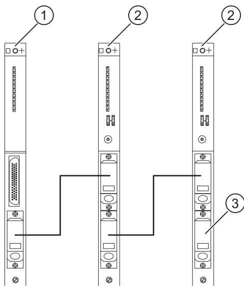
图 5-23 一个发送 IM 和两个接收 IM 之间的连接
