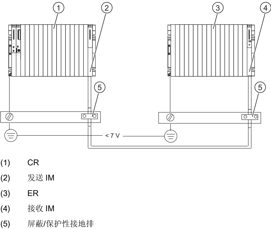
图 5-8 远程连接的屏蔽和接地连接电缆
