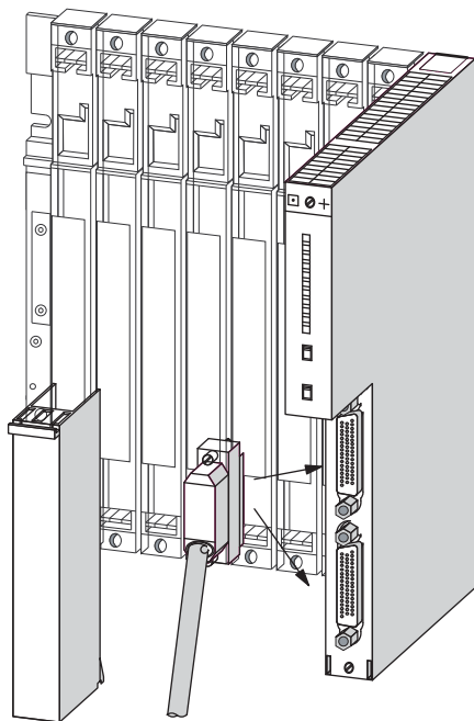
图 5-22 将连接电缆插入发送 IM
