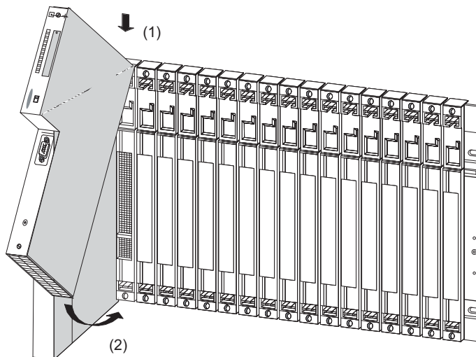
图 3-3 安装模块
