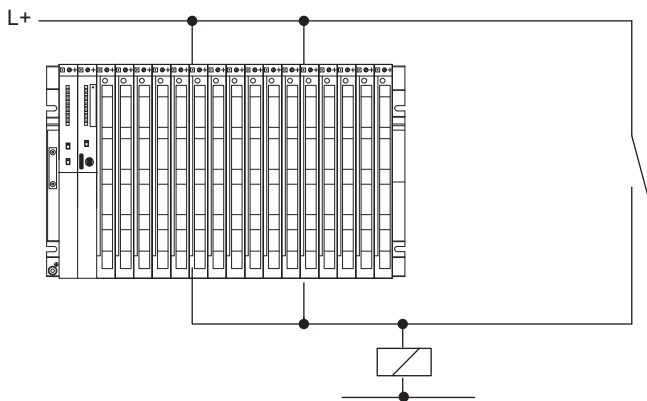
图 5-6 数字量输出(带相同额定负载电压)的并行接线
