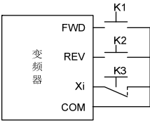
图 6-16 三线式运行模式 1
