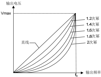
图 6-12 V/F 曲线
