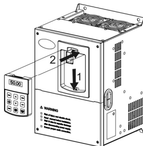
图 2-3 操作面板的安装
