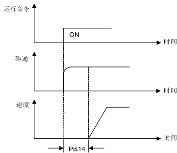
图 6-37 预激磁
