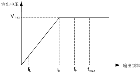
图 6-2 特性参数定义
