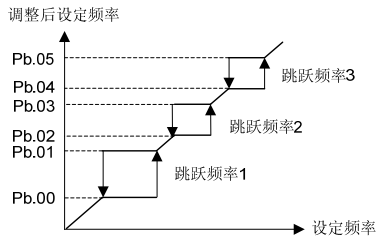
图 6-34 跳跃频率上下限
