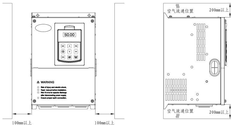
图 2-1 VY-H-4T3.7GX/5.5LX 及以上功率等级的安装方向和空间
