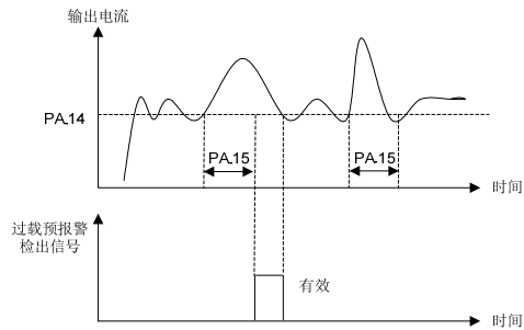
图 6-33 过载预警
