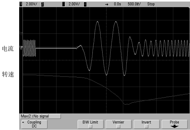
图 5 电机高速自由旋转时跟踪并降频后平滑启动
