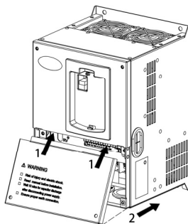
图 2-7 下盖板的安装
