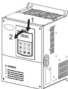
图 2-2 操作面板的拆卸
