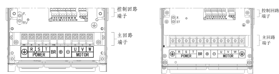
VY-H-4T3.7GX/5.5LX~VY-H-4T15GX/18.5LX 功率等级 VY-H-4T18.5GX/22LX 及以上功率等级 图 3-2 产品端子配置情况
