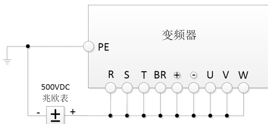
图8-1 V5-20H-4T11GX/15LX~V5-20H-4T110GX/132LX 主回路绝缘测试
