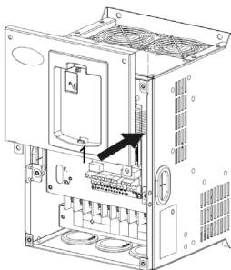
图 2-6 上盖板的安装
