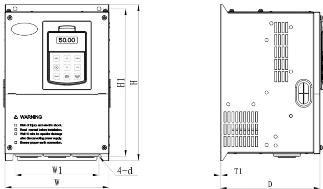
图 1-2 产品的外形和安装尺寸
