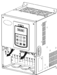
图 2-5 上盖板的拆卸
