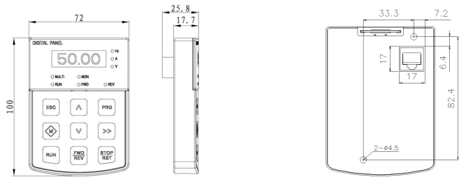
按键型操作面板（V6-DP04）
