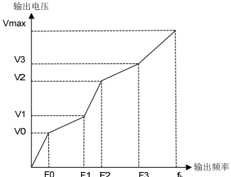
图 6-13 多段 V/F 曲线
